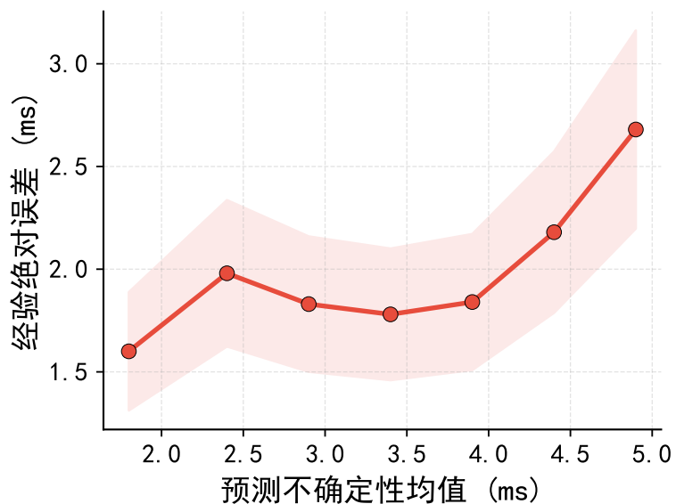
(c) 置信度校准结果
