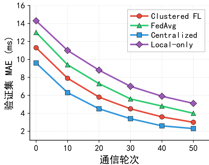
(a) 联邦训练收敛过程
