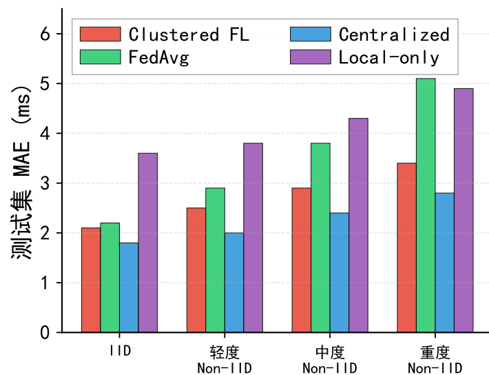
(d) 不同异构强度下的 MAE
