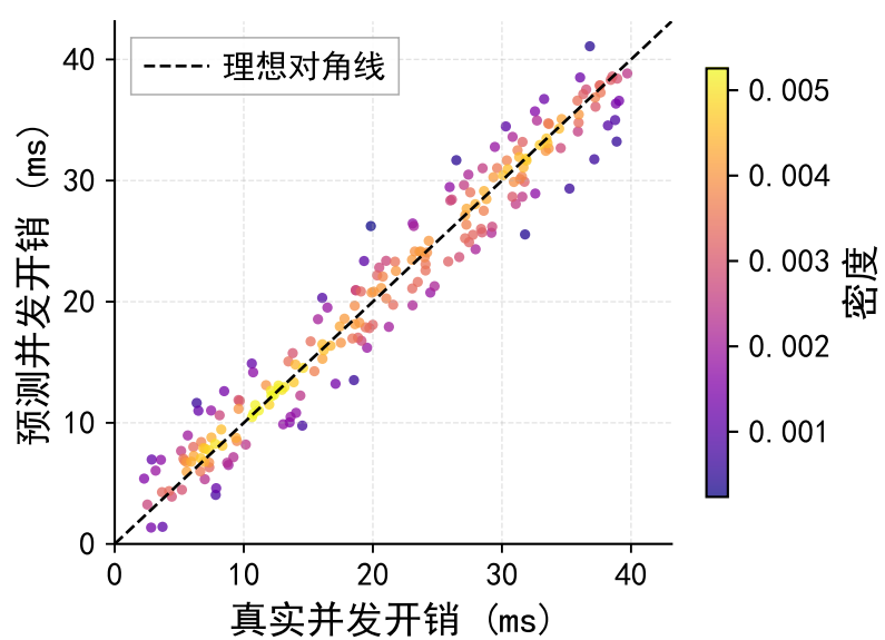
(b) 预测—真实散点密度
