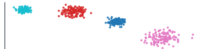
Anisotropic Blobs
