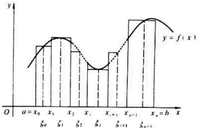
黎曼积分
