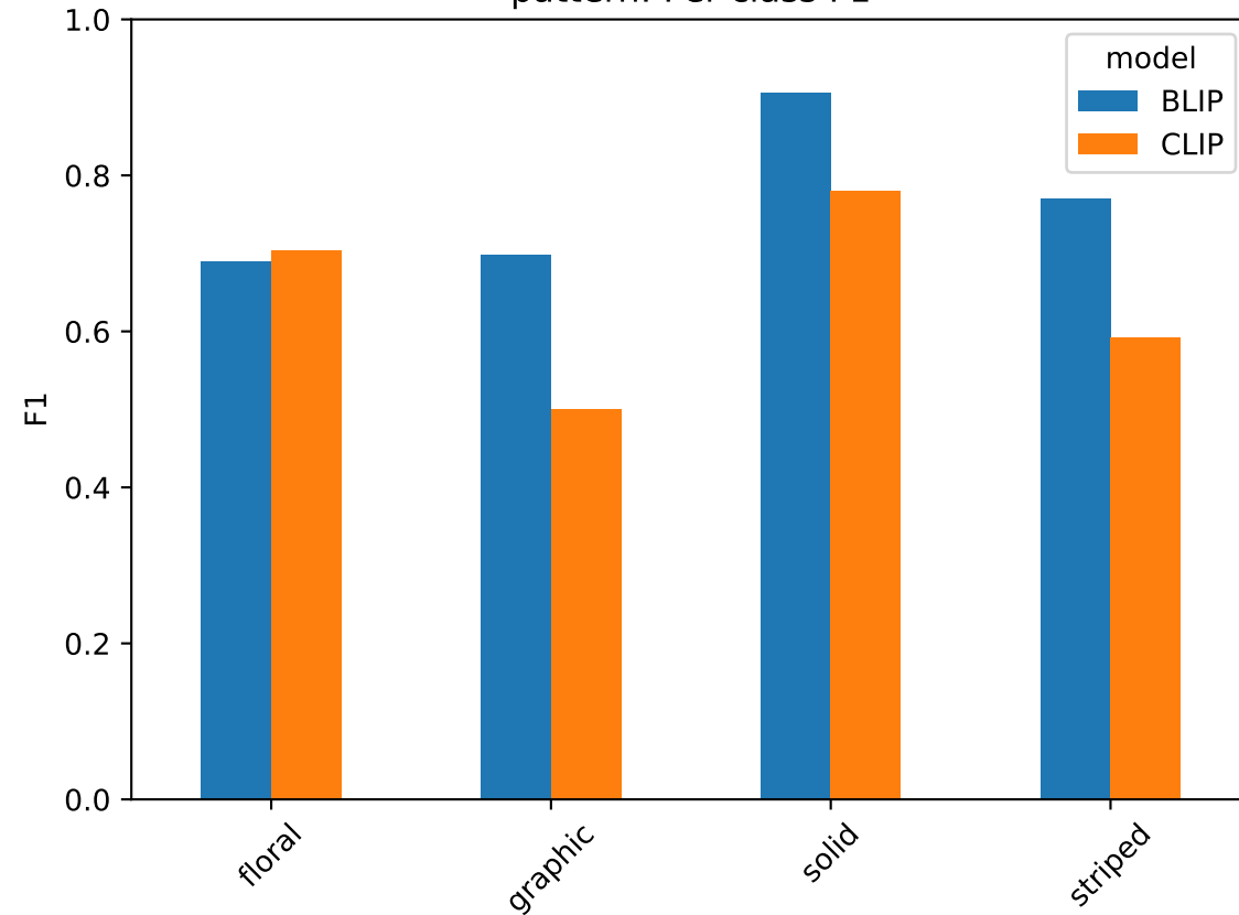
pattern: Per-class F1
