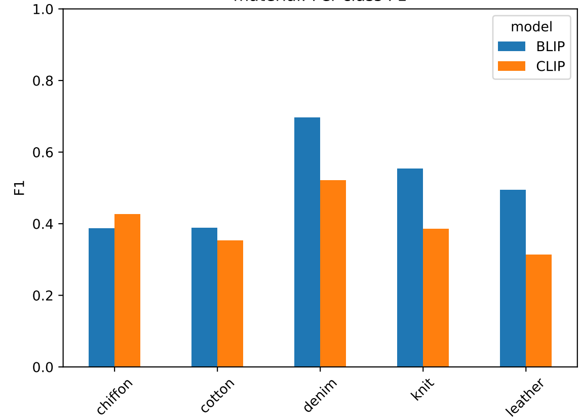
material: Per-class F1
