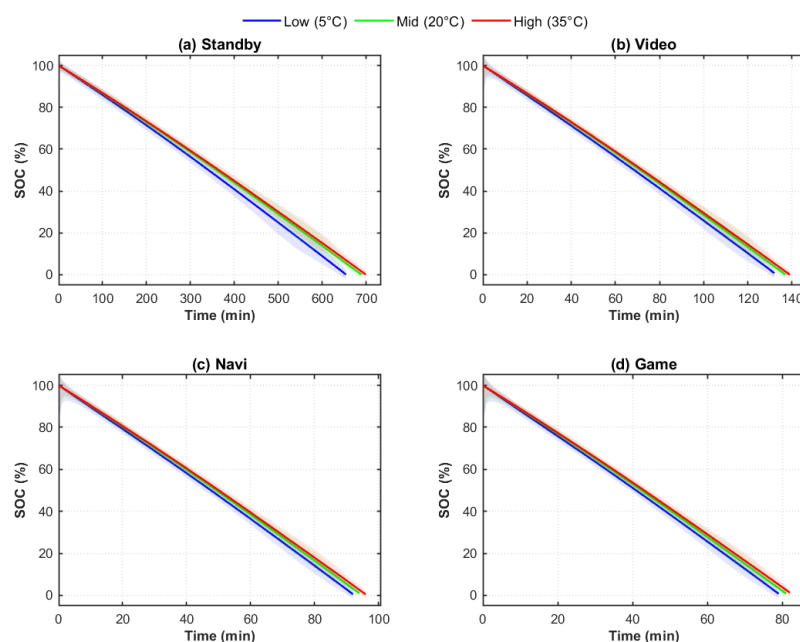
图 14: 不同温度下的 SOC 衰减曲线
