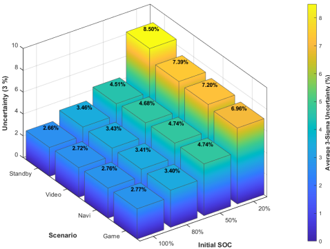
图 13: 不同场景和初始 SOC 组合下的平均 3σ 不确定性水平
