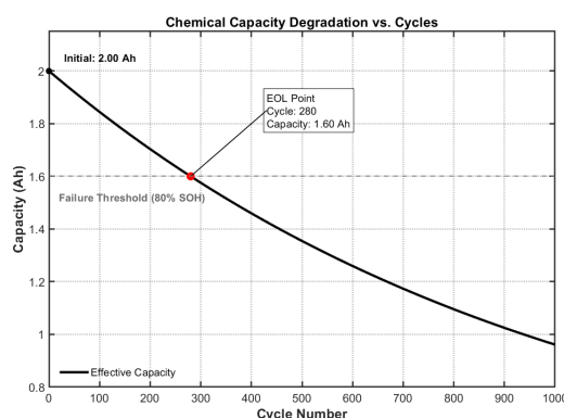
图 9: 容量和循环次数关系曲线
