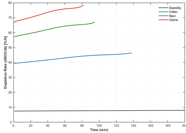
图 7: 不同使用场景下的 SOC 衰减率对比
