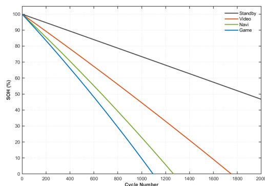
图 8: 不同使用场景下的 SOH 衰减对比
