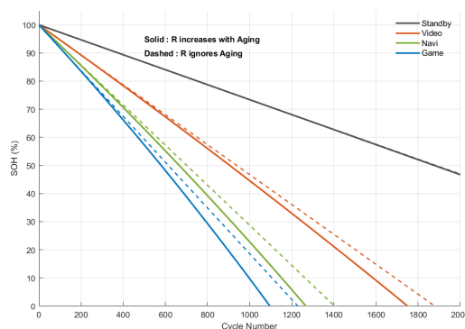
图 18: 不同内阻模型下的 SOH 衰减曲线
