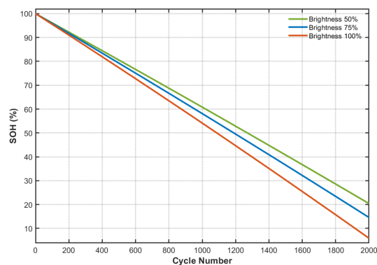
(b) 不同亮度下的 SOH 衰减曲线（待机场景）
