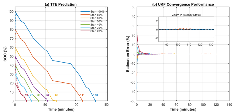
图 11: 动态场景下 Time-to-Empty Prediction 评估结果
