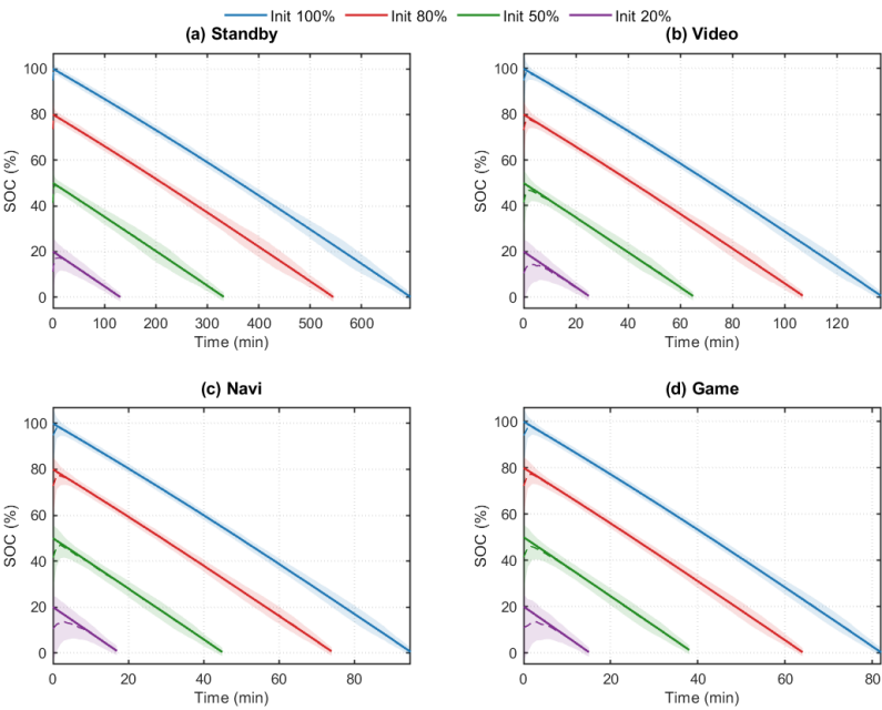
图 12: 预测模型在动态场景下的不确定性评估结果
