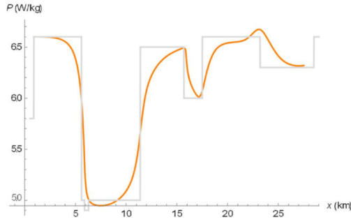
Figure 13: Actual output power
