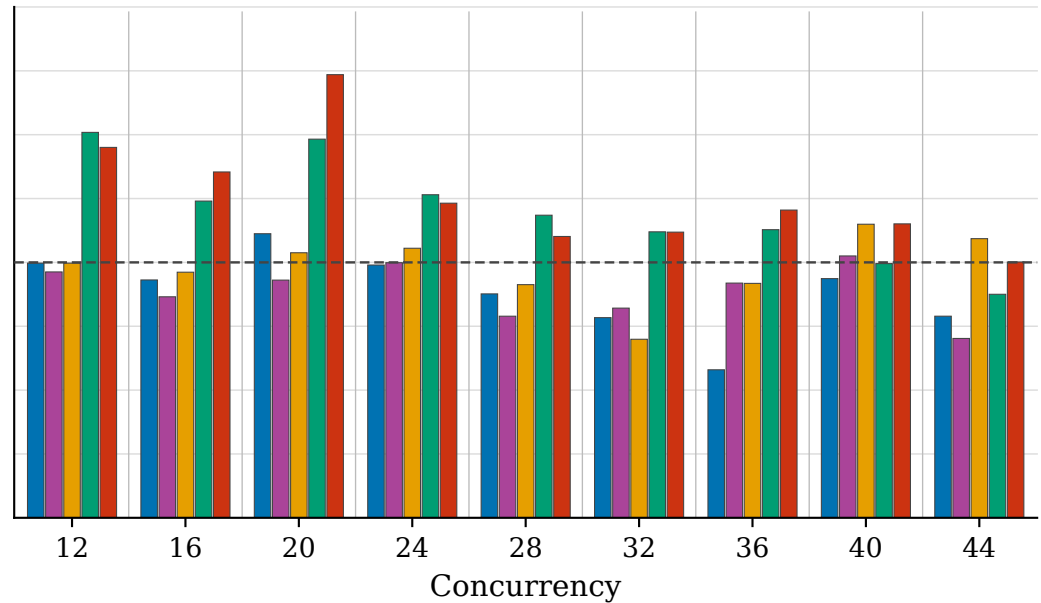
Mean TTFT
