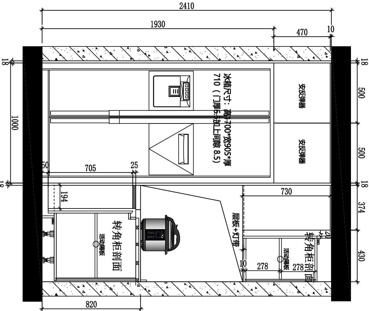
立面图 比例1:1
