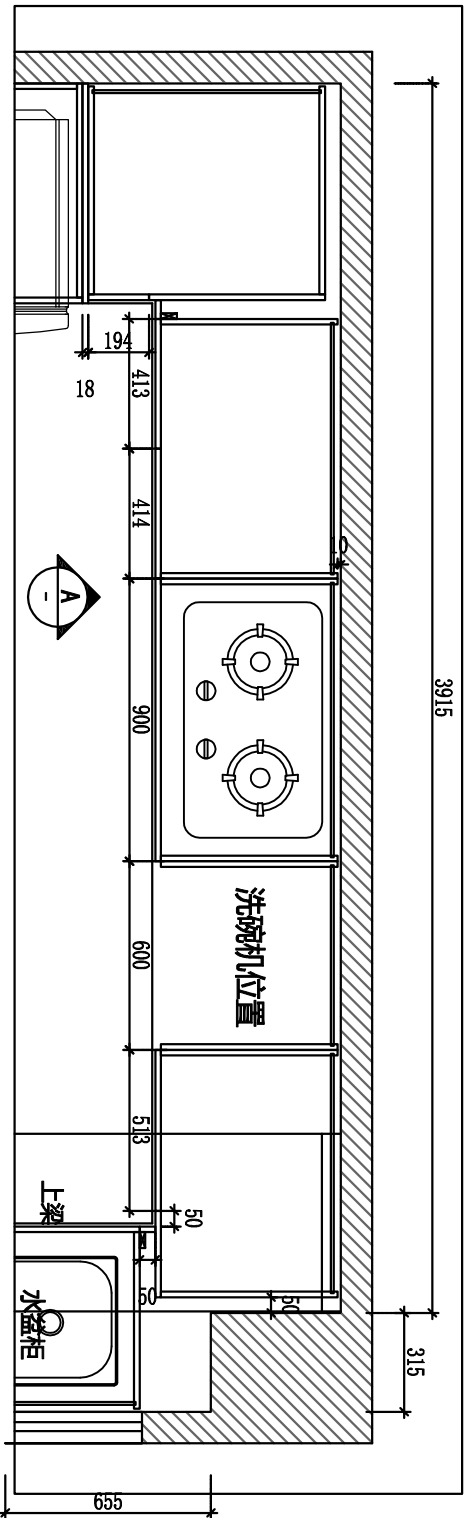
立面图 比例1:1
