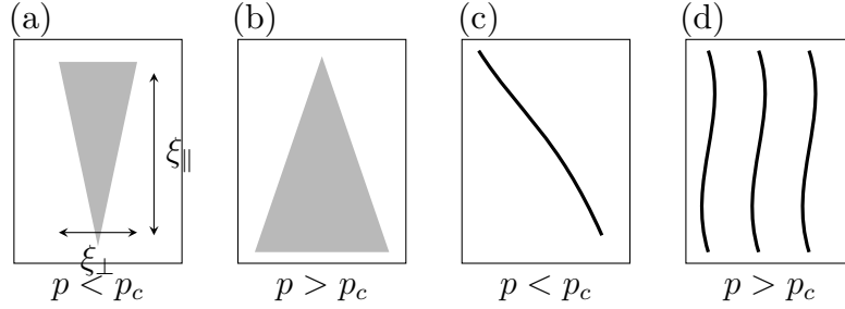
图 1.31: 临界点以下和以上, 不同初始条件的有向渗流过程中关联长度 \xi_{\parallel}, \xi_{\perp} 的图示. (a)–(d) 的说明见正文. 改绘自 Hays Hinrichsen, Non-equilibrium critical phenomena and phase transitions into absorbing states, Advances in Physics 49 (2000) 815–958.
