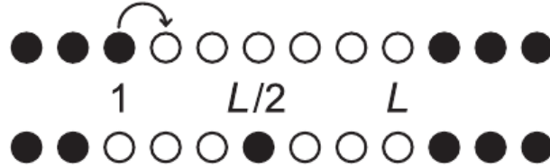
图 1.71: 两个粒子畴由空穴隔开。左畴脱附的粒子若在返回格点 1 前到达右畴格点 L ，两畴便交换物质。粒子位于 L/2 时，到达起始畴与目标畴的概率相等。
