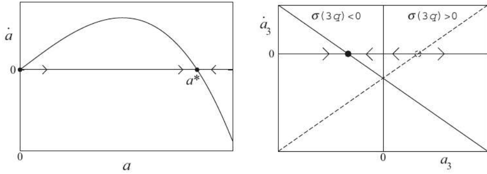
图 1.99: a(t) (见式 (7.80)) 与 a_3(t) (见式 (7.81)) 的流.
