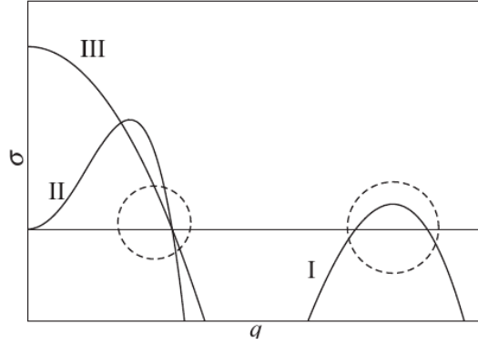
图 1.100: 模型 I、II、III 的稳定性曲线示意图; 虚线圈出的 q 区域可作弱非线性分析.
