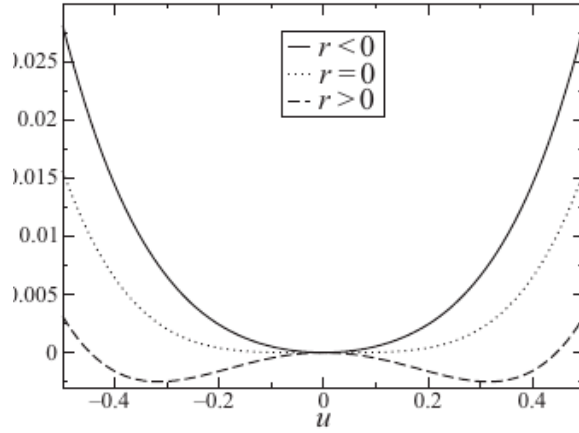
图 1.93: 负、零、正 r 时的势 V(u) ; 见式 (7.6).
