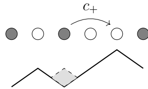
图 1.50: ASEP 到单步模型的映射. 粒子向右 (左) 移动, 对应在局域极小处沉积一个粒子 (从局域极大处蒸发一个粒子). 使粒子模型偏离平衡, 意味着在向右跳与向左跳之间制造不对称; 在表面生长模型中, 这种不对称意味着沉积与蒸发之间不平衡.
