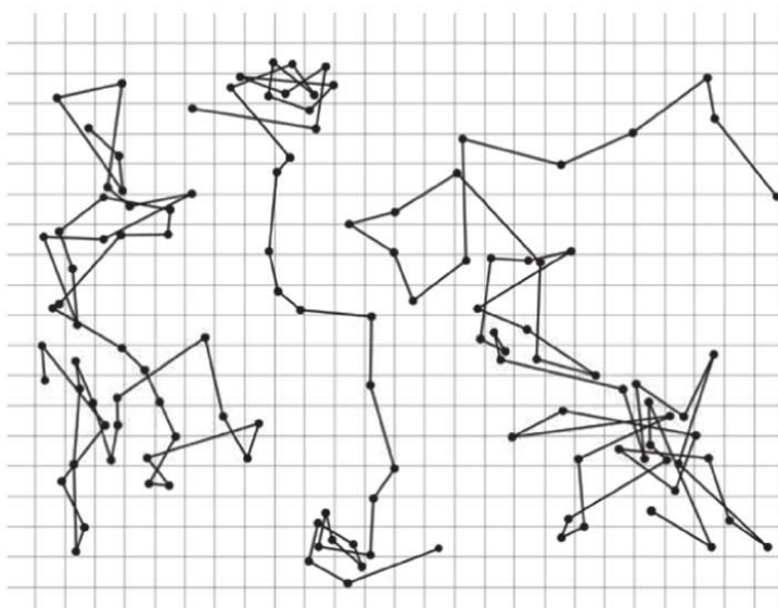
图 1.5: 显微镜下所见半径为 0.53 \mu\text{m} 的胶体粒子的三条运动轨迹。每隔 30 \text{ s} 的相继位置用直线段连接，网格间距为 3.1 \mu\text{m} 。转载自 J. B. Perrin, Les Atomes (Paris: Librairie Félix Alcan, 1913), Wikimedia Commons.
