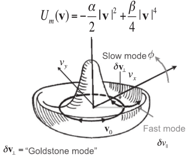
图 4.2.3: “Mexican 帽” 势；注意由极小值构成的圆环. 使速度沿环移动的涨落 \delta \mathbf{v}_\perp 是“Goldstone 模式”，不受这个“势”的回复力；相反，使速度沿帽檐上升或朝向帽顶（即沿径向）的涨落 \delta v_\parallel 是“快”模式，会因该势迅速弛豫，这只反映集群运动个体穿过摩擦介质时存在优选速率. 图中保留出版图的英文“Slow mode”与“Fast mode”标注，以避免改变三维势面的科学含义；经 Oxford University Press 许可，转载自文献 [7].
