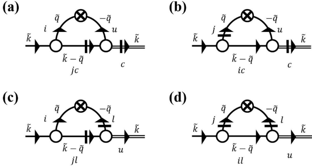
图 9.6.1: 运动方程 (9.3.1) 中线性项修正的图形表示. 转载自文献 [23].
