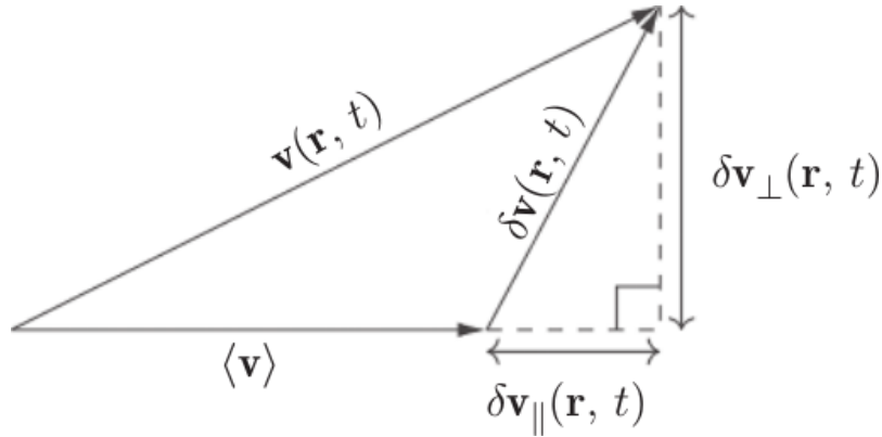
图 4.2.1: 把局域速度 \mathbf{v} 分解为其平均值 \langle \mathbf{v}(\mathbf{r}, t) \rangle \equiv v_0 \hat{\mathbf{x}}_\parallel 与偏离平均值的局域涨落 \delta \mathbf{v} . 矢量 \delta \mathbf{v} 还可进一步分解为平行于平均速度的分量 \delta v_\parallel 与投影 \delta \mathbf{v}_\perp(\mathbf{r}, t) . 经 Oxford University Press 许可, 转载自文献 [7].
