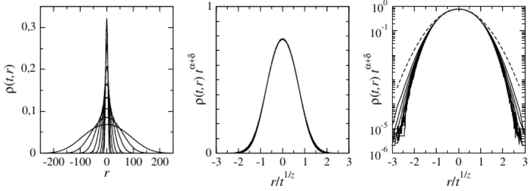
图 4.7: 左图: 临界点处, (1 + 1) 维接触过程中由单个种子生成的簇在 t = 16, 32, 64, \dots, 2048 时的扩散轮廓. 中图: 按照式 (4.81) 得到的数据坍缩. 右图: 以半对数坐标表示的同一数据坍缩. 虚线表示在 origin 处拟合的高斯分布.
