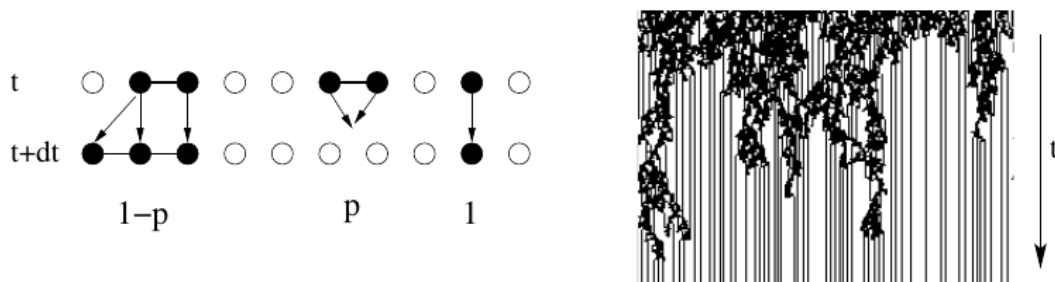
图 3.11: 1 + 1 维成对接触过程 [350]. 左图: 晶格格点可以为空 (空心圆), 也可被粒子占据 (实心圆). 被占据的格点对 (实线键) 视为活性的, 而孤立粒子保持非活性. 格点对以速率 p 湮灭; 否则, 在随机选取的空相邻格点产生一个后代. 右图: 亚临界 PCP 的模拟, 最终停在由不可移动孤立粒子组成的吸收构型.
