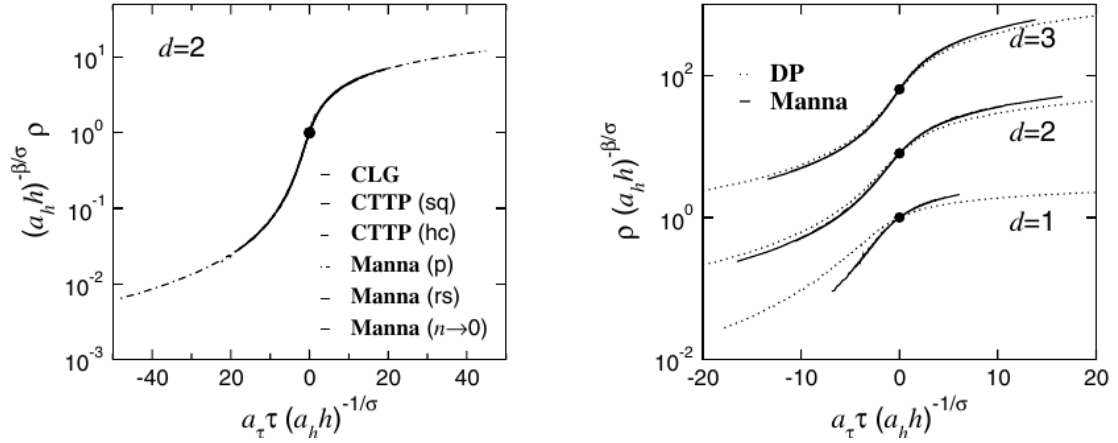
图 7.8: 不同维数中 Manna 普适类状态方程的普适标度函数 \tilde{R}(x, 1) . 曲线按照标度形式 (5.206) 绘制. 对 d = 2 , CTPP 数据来自方格 (sq) 和蜂窝 (hc) 晶格模拟. 对 Manna 模型, 图中给出原始模型 (7.56) 采用随机顺序 (rs) 与并行 (p) 更新的数据, 以及修改模型在 n \rightarrow 0 极限 (7.57) 的数据. 如左图所示, 所有曲线塌缩到同一条曲线上. 此外, 标度函数依赖维数, 并不同于 DP 的相应标度函数 (见右图). 经许可转载自文献 [433]. 版权所有 © 2004 World Scientific Publishing Company.
