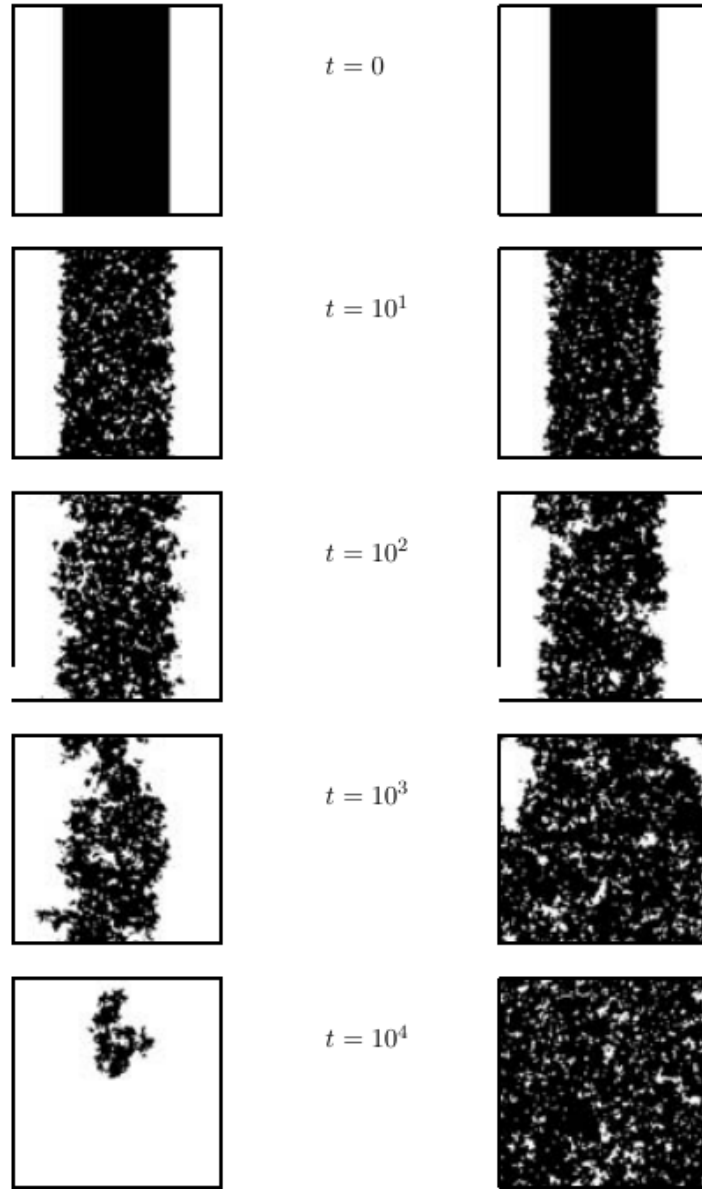
图 7.15: 通过分析界面运动估计一级相变临界点. 图中是在一级转变附近、采用周期性边界条件的三临界接触过程快照. 从一条粒子条带出发, 动力学要么被空晶格吸引 (左, p < p_c ), 要么被齐次非零粒子密度稳态吸引 (右, p > p_c ). 经 Springer Science and Business Media 许可, 转载自文献 [436].
