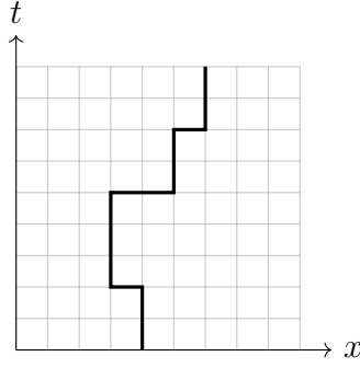
图 10.1: 沿方格晶格主轴的一条有向路径.
