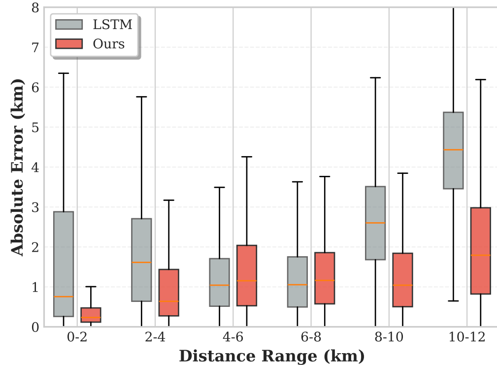
(d) Error Distribution by Range
