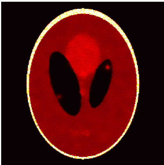
NLM
