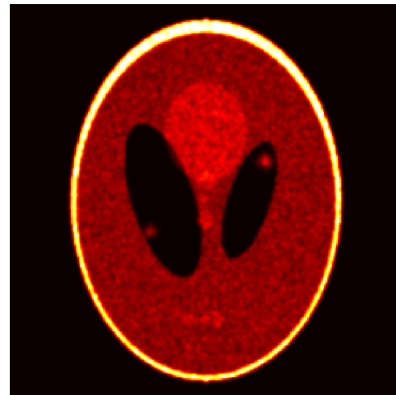
Adaptive VST-PGD
