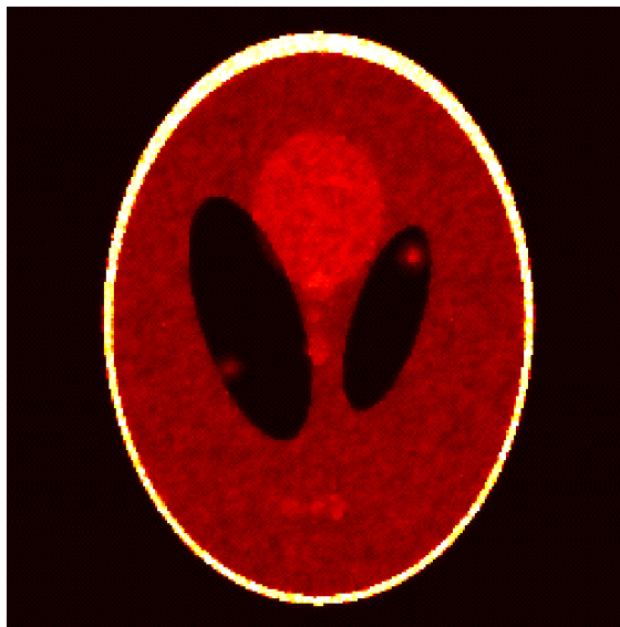
TV-GD
