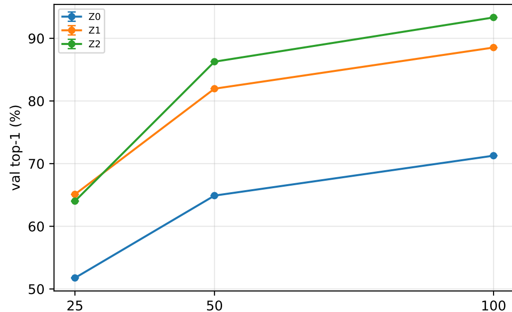
vits1k
