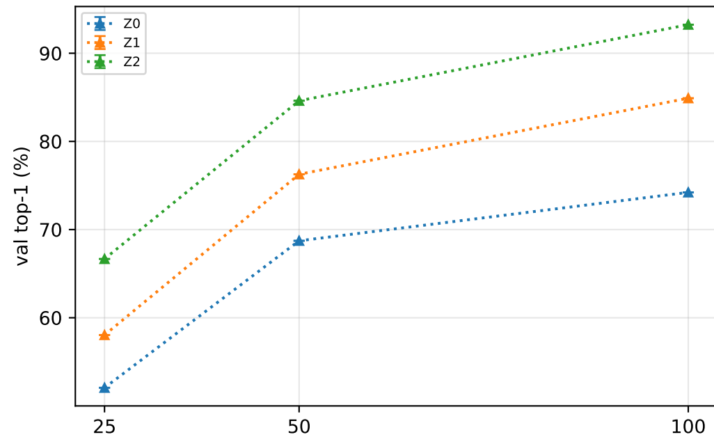
vits1k
