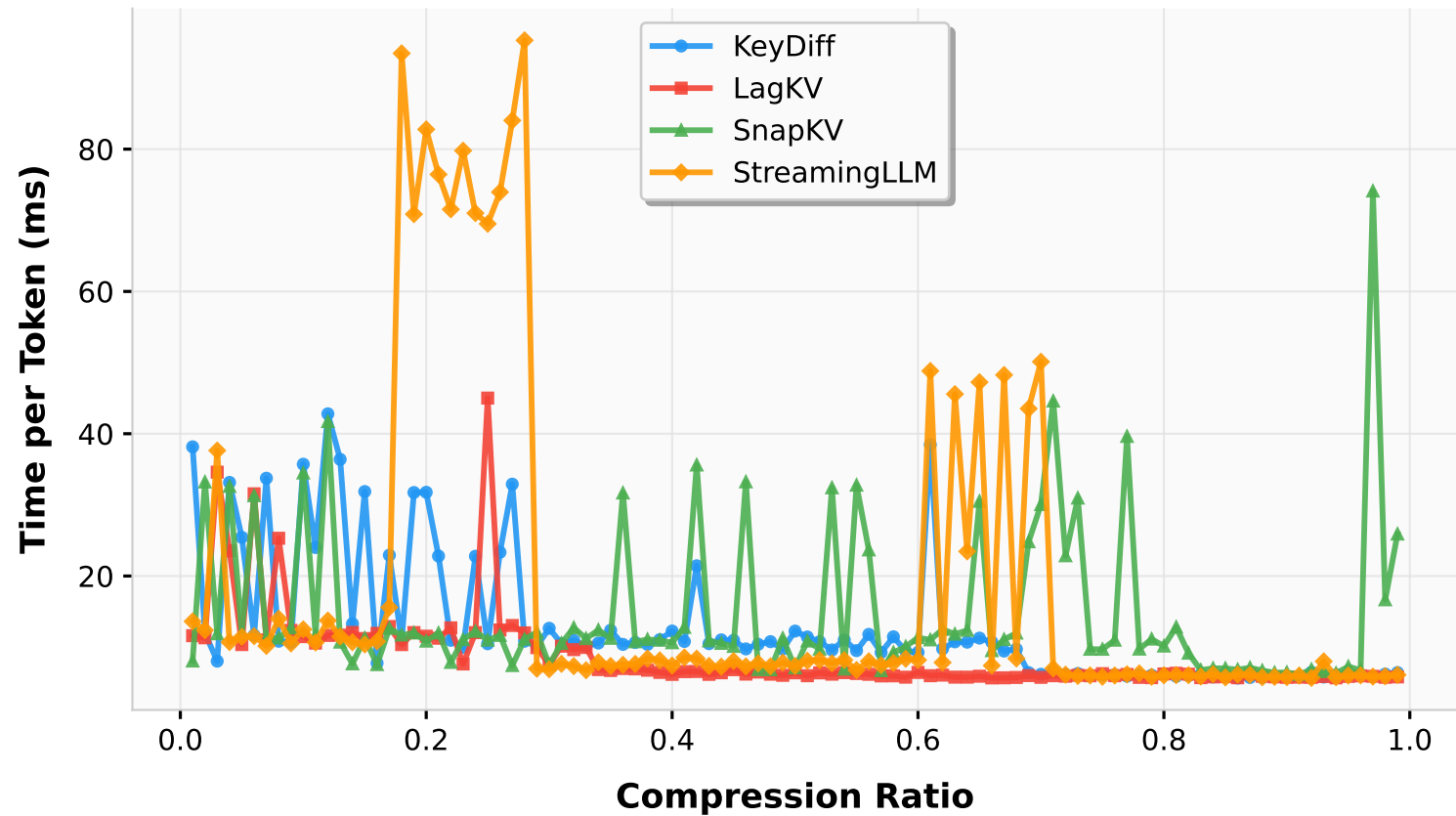
PG19 - Time per Token (ms)
