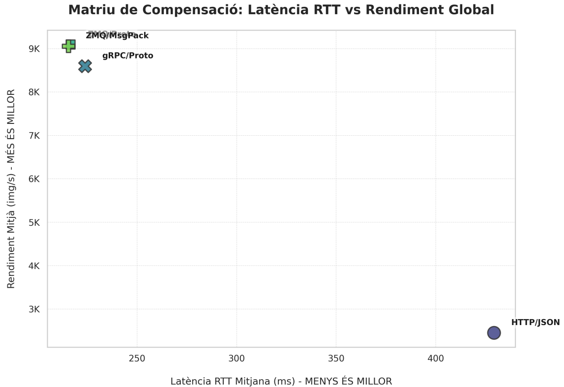
Figura 6.3: Relació de compromís ( Trade-off ) entre rendiment global i Latència RTT.
