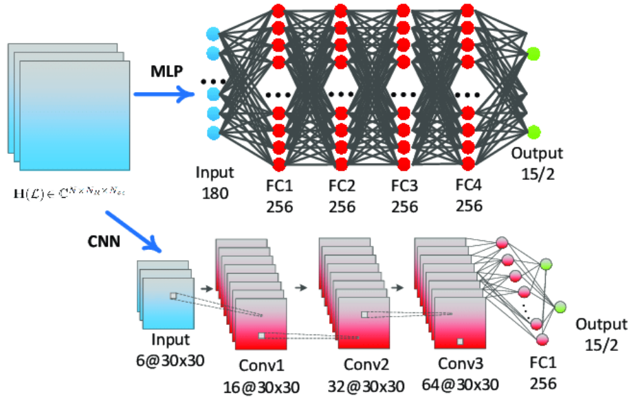
Figura 2.2: Arquitectura comparativa de xarxes MLP i CNN dissenyades per a tasques de classificació i regressió. Font: Adaptada de [1].
