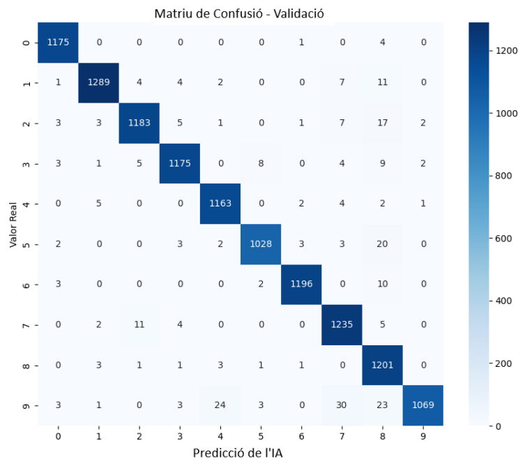
Figura 6.5: Avaluació del model fundacional: Matriu de confusió en validació.
