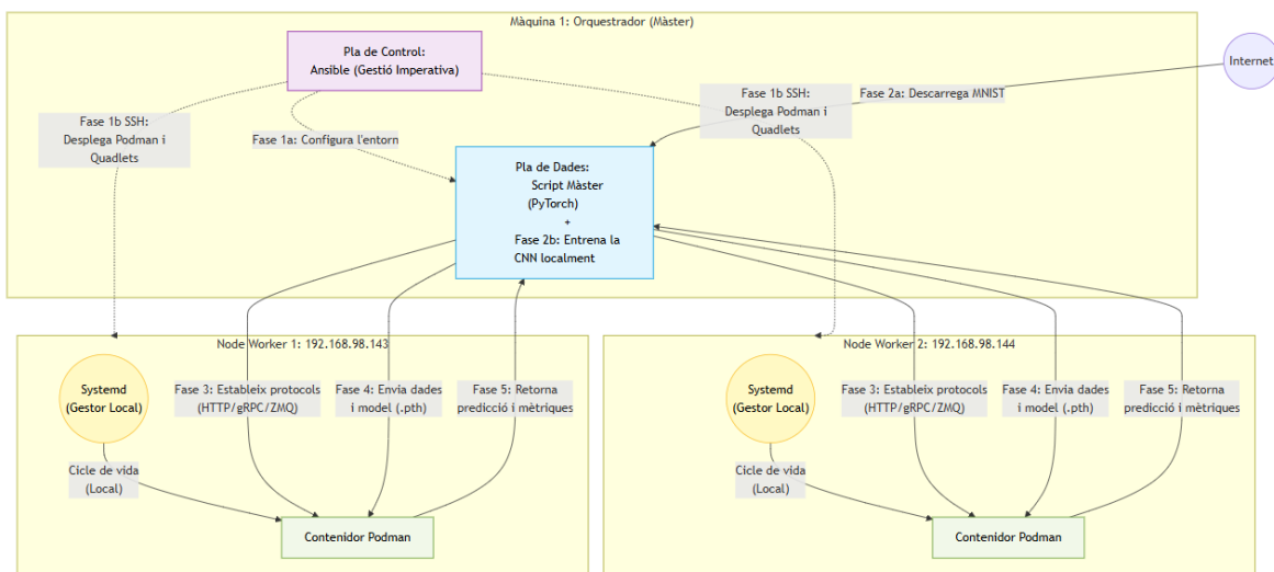
Figura 5.3: Topologia completa de la inferència d'IA sobre Systemd.
