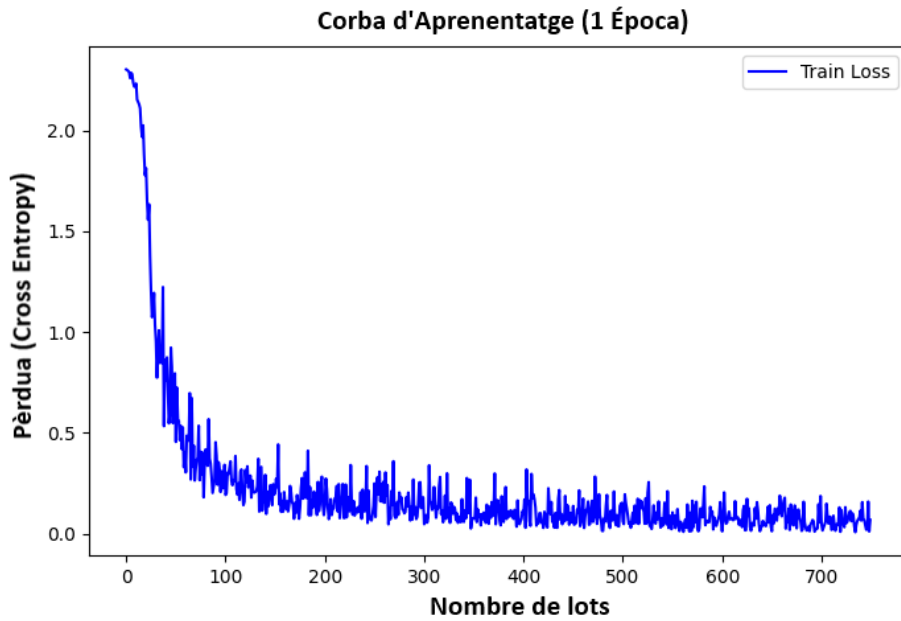
Figura 6.4: Avaluació del model fundacional: Corba de pèrdua ( Train Loss ).
