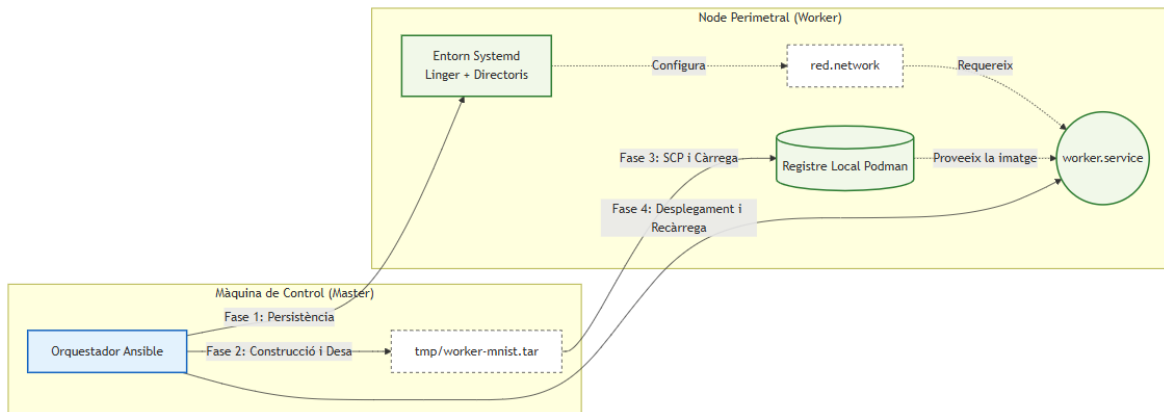
Figura 5.1: Arquitectura de l'entorn nativa amb Systemd.
