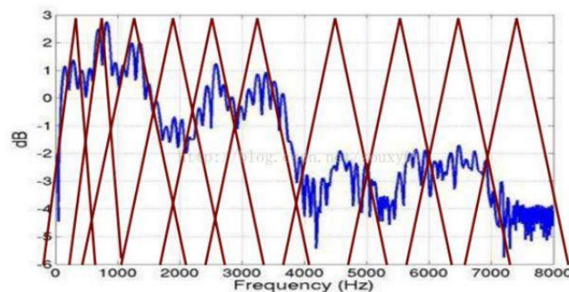
图 2. 梅尔频率倒谱的基本概念示意图。
