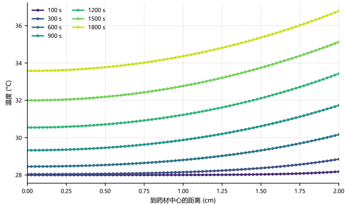
30分钟内药材径向温度分布
