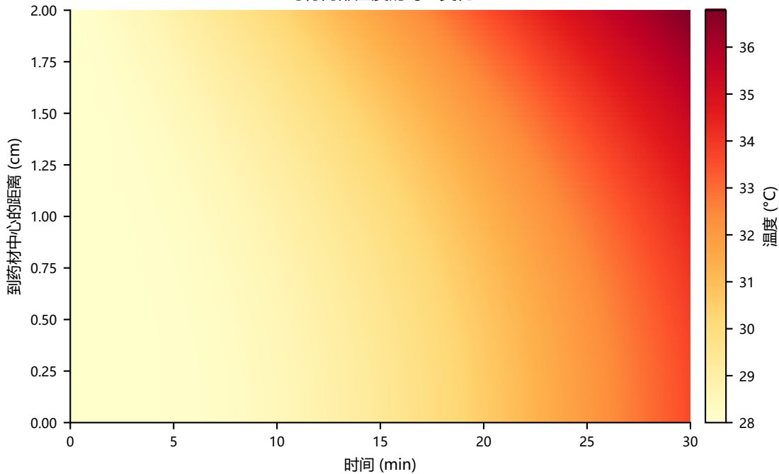
药材内部温度的时空变化
