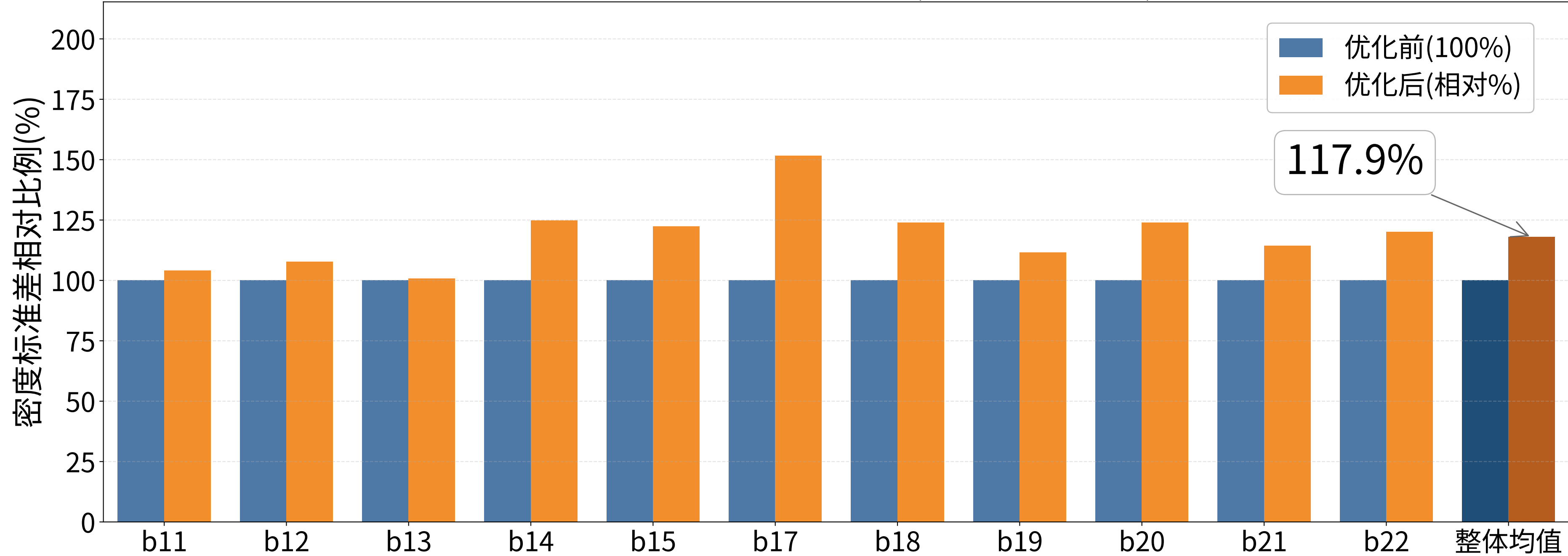
密度标准差相对比例变化(优化前=100%)
