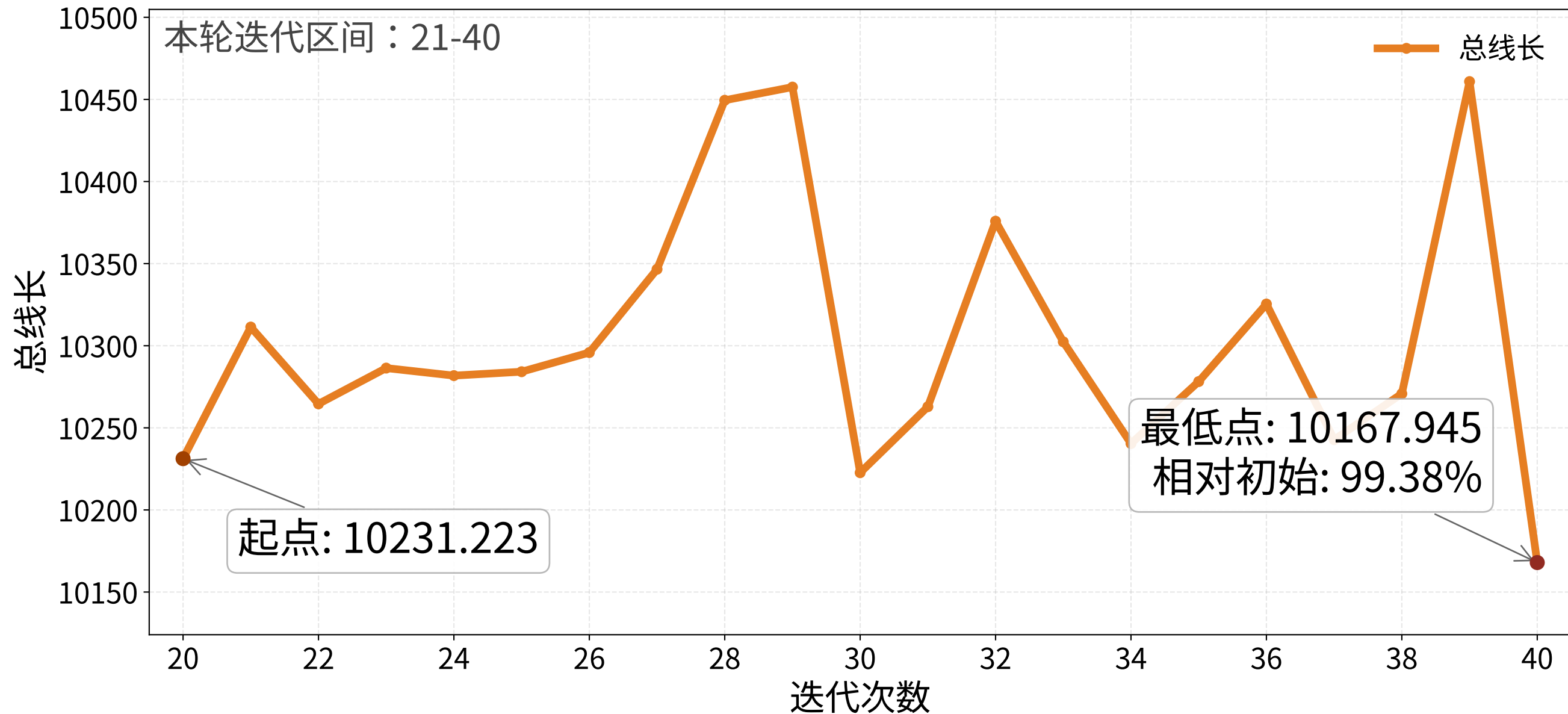
b20 第2轮模拟退火：总线长变化曲线
