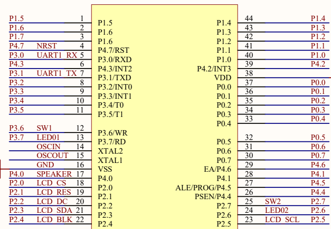
8051微处理器芯片
