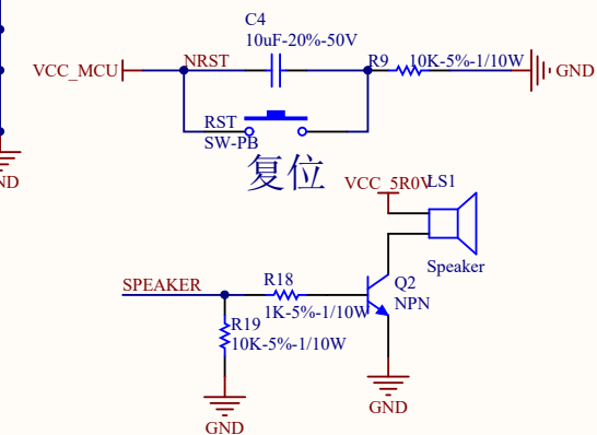
蜂鸣器
