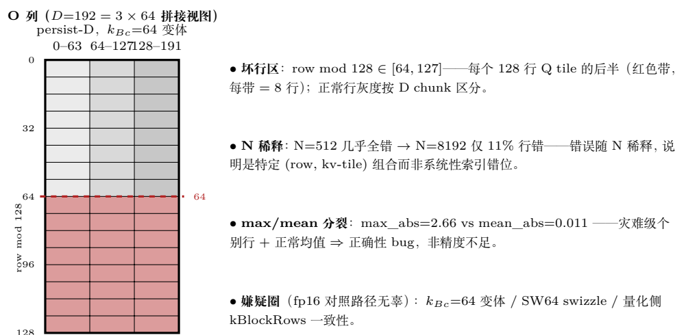
图 31.6: D=192 正确性 bug 的坏行定位 (29.7.1 节五步法的可视化): 把 O 视为 3 \times 64 列拼接, 坏行集中在 row mod 128 \in [64, 127] (每个 128 行 Q tile 的后半); N=512 几乎全错而 N=8192 仅 11% 行错 (N 稀释 \Rightarrow 特定 (row, kv-tile) 组合); max_abs=2.66 对 mean_abs=0.011 的分裂是「个别行灾难」的强信号。
