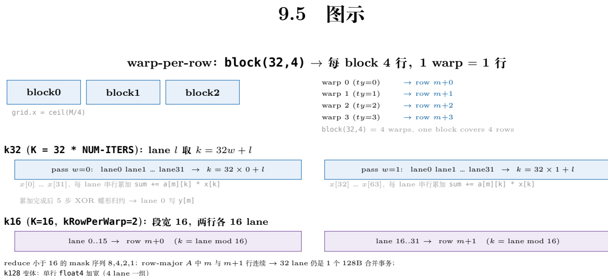
图 9.2: warp-per-row 的划分: k32 单行 32 lane 铺满、k16 双行各 16 lane 分段归约 (mask 8/4/2/1); k128 变体串行 float4 加宽。
