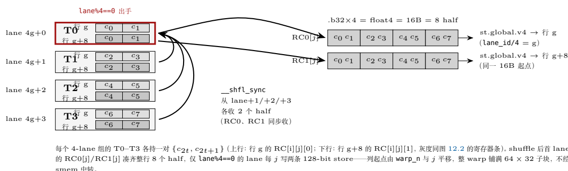
图 12.7: Epilogue shuffle 收拢与写回 (hgemm.cuh L336-382): 4-lane 组内 T0-T3 各持一对 \{c_{2t}, c_{2t+1}\} (上行 = 行 g , 下行 = 行 g+8 的寄存器对), _shfl_sync 从 \text{lane}+1/+2/+3 各收 2 个 half, 把 \text{RC}[0][j] (行 g ) 与 \text{RC}[1][j] (行 g+8 ) 各凑成 4 条 .b32 = 一条 16B float4 ; 随后仅 \text{lane}\%4==0 的 lane 出手, 行号 = \text{lane\_id}/4 = g , 两条 128-bit store 分别写行 g 与 g+8 。
