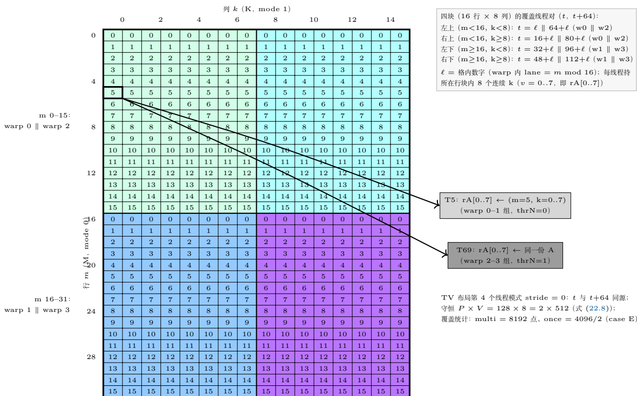
图 22.3: S \rightarrow R A 拷贝的 2 倍重复因子 (式 (22.9)、测试 case D/E): tiler (32, 16) 的 A tile ( M \times K ) 上, 每格标 warp 内 lane 号 \ell = m \bmod 16 , 格子的实际覆盖线程对为 (基址 + \ell , 基址 + 64 + \ell ), 四块的基址见右上表 (w0-w3 即 warp 0-3)。每个元素恰被 2 个 (thread, value) 对覆盖: t 与 t+64 (两个 N 方向 warp, \text{thrN} = 0/1 ) 各持同一行块 8 个连续 k 的一份寄存器拷贝——TV 布局第 4 个线程模式 stride 为 0 的几何含义, 守恒 128 \times 8 = 2 \times 512 。对照图 22.5 的 G \rightarrow S 双射网格 (每格恰一线程)。
