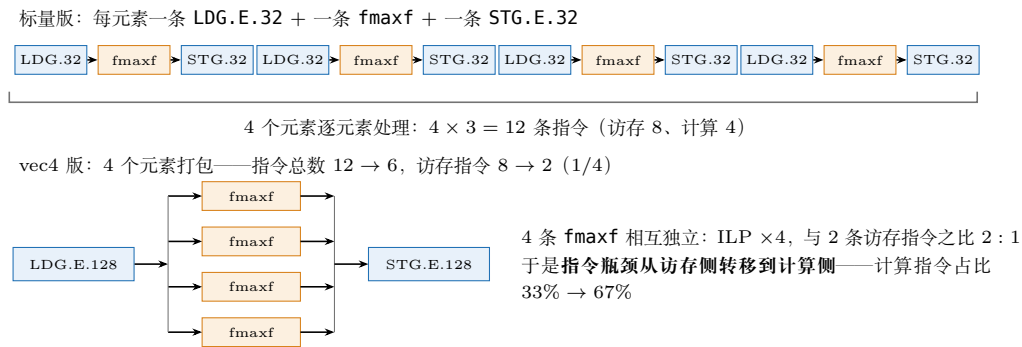
图 4.3: 标量与 vec4 的指令流对照 (relu, 以 4 个元素为例): 标量版每元素 3 条指令 ( LDG.E.32 \rightarrow fmaxf \rightarrow STG.E.32 ), 4 元素共 12 条、其中访存 8 条; vec4 版用一条 LDG.E.128 取回 4 个元素, 4 条 fmaxf 互不依赖 ( \text{ILP} \times 4 ) 后由一条 STG.E.128 写回, 总数降到 6 条、访存只剩 2 条。访存: 计算从 8:4 变为 2:4, 指令瓶颈因此从访存侧移到计算侧。
