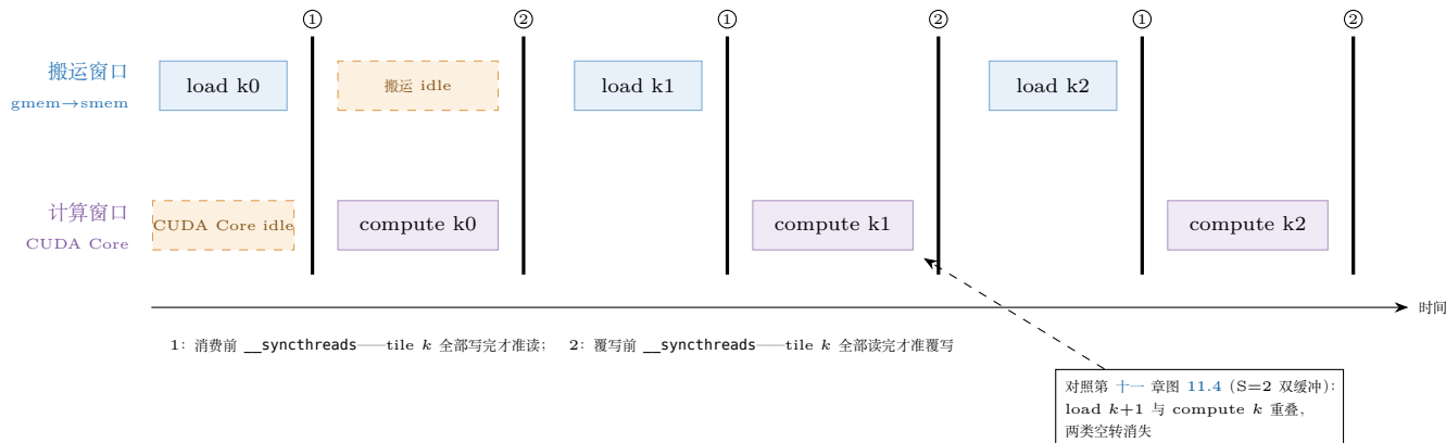
图 10.1: 单缓冲 k-slice 循环的双栅栏时序 (3 个迭代): load (蓝) → 栅栏 1 (消费前) → compute (紫) → 栅栏 2 (覆写前)。load 期间 CUDA Core 空转、compute 期间搬运单元空转——「搬一算一」串行使两个窗口无法重叠；双缓冲 (图 11.4) 正是为消除这两类空转而来的。
