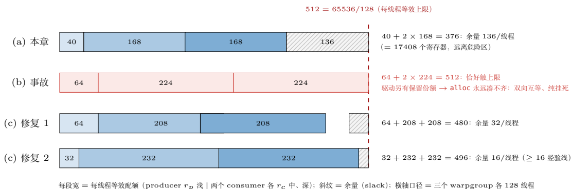
图 19.2: 65536 个寄存器按角色「切蛋糕」的三种切法 (式 19.5 与 18.3.4 节事故分析的图形化)。横轴为每线程等效配额 r_p + 2r_c \leq 512 = 65536/128 : (a) 本章 D=128 的 40 + 2 \times 168 = 376 , 余量 136/线程 (= 17408 个寄存器), 远离危险区; (b) 第 十五 章那次事故的 64 + 2 \times 224 恰好等于 512——驱动对寄存器文件另有保留份额, 有效池小于 65536, 于是 consumer 卡在 setmaxnreg 、producer 卡在等 barrier arrive, 双向互等、纯挂死 ; (c) 修复版的 480 与 496 分别留出 32 与 16 的每线程余量, 后者正是工程规则「 \geq 2048 slack」除以 128 的下界。
