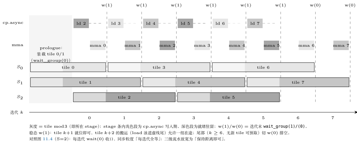
图 12.5: kStages=3 三级流水时序: 迭代 k 读 S_{k \bmod 3} (tile k )、同时预取 (k+2) \bmod 3 (tile k+2 )，三个 stage 按 tile mod 3 轮转。稳态迭代末 wait_group(1) 允许一组搬运在途; 尾部无 tile 可预取时切 wait_group(0) 排空。与图 11.4 的两级流水 (每迭代 wait(0) ) 相比, 同步粒度从「每迭代全等」放松为「保持距离即可」。
