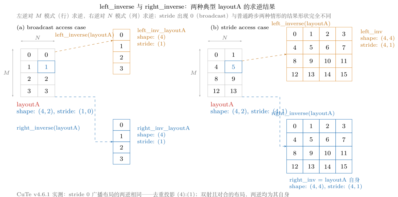
图 21.9: left_inverse / right_inverse 的两种情形 (CuTe v4.6.1 实测): stride (1,0) 广播布局两逆相同, 均为去重投影 (4):(1)——stride 为 0 的维度被投影掉, 每行只保留代表坐标 m; stride (4,1) 的双射布局两逆均为其自身 (4,4):(4,1) (该布局是对合, f \circ f = \text{id} )。重建自 @ 竹熙佳处《写给大家看的 CuTe 教程: Layout Compose & Inverse》(数值按 CuTe v4.6.1 实测校正)。
