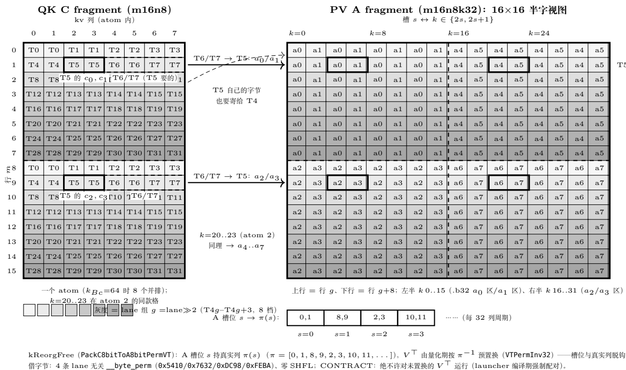
图 31.2: C→A fragment 的 lane→值映射 (lst:29-reorg-bg 的网格化)。左: QK C fragment (m16n8), 每 lane 4 值 c_0-c_3 落在行 g/g+8 的列对 \{2t, 2t+1\} ; 右: PV A fragment (m16n8k32) 的 16×16 半字视图, 格值 a_0-a_7 为 e4m3x2 半字寄存器, 四象限对应源码.b32 a_0-a_3 ; 两面板灰度同语义 (lane 组 g = \text{lane} \gg 2 , 8 档)。中: t=1 (T5) 的自然 A 需要 k \in \{4..7\} \cup \{20..23\} (行 g 与 g+8 ), 在 C 视图里属 T6/T7——纯 lane 内置换凑不齐, 即 16 SHFL + 32 PRMT (ReorgC8bitToA8bit) 的根源。下: kReorgFree 的出路——槽位持 \pi(s) 、 V^\top 预置换, 4 条 lane 无关 __byte_perm、零 SHFL。
