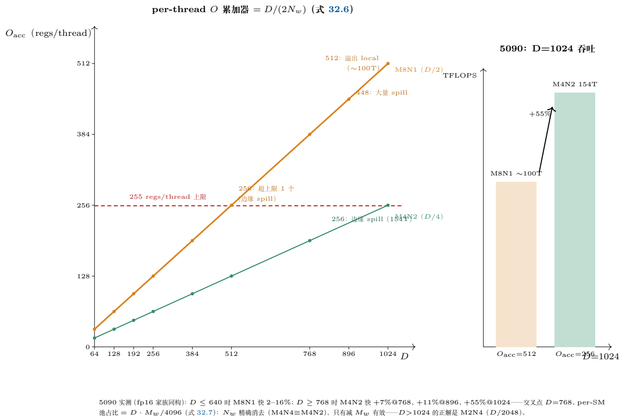
图 32.2: 寄存器墙的定量视图。左: per-thread O 累加器 = D/(2N_w) (式 32.6) ——M8N1 的 D/2 在 D=512 达 256 (超 255 上限 1 个, 边缘 spill)、 D \geq 896 大量 spill、 D=1024 溢出 local memory ( \sim 100T ); M4N2 的 D/4 同点仅 256 (154T)。右: 5090 实测 D=1024 吞吐对比 (+55%)。下: per-SM 池占比 D \cdot M_w / 4096 (式 32.7) 中 N_w 精确消去——加 N-warp 不降总量, D > 1024 只能走 M2N4。
