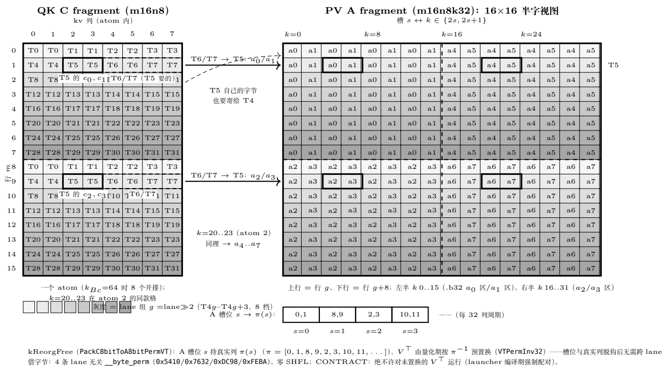
图 30.2: C→A fragment 的 lane→值映射 (lst:29-reorg-bg 的网格化)。左: QK C fragment (m16n8), 每 lane 4 值 c_0-c_3 落在行 g/g+8 的列对 \{2t, 2t+1\} ; 右: PV A fragment (m16n8k32) 的 16×16 半字视图, 格值 a_0-a_7 为 e4m3x2 半字寄存器, 四象限对应源码.b32 a_0-a_3 ; 两面板灰度同语义 (lane 组 g=\text{lane}\gg 2 , 8 档)。中: t=1 (T5) 的自然 A 需要 k \in \{4..7\} \cup \{20..23\} (行 g 与 g+8 ), 在 C 视图里属 T6/T7——纯 lane 内置换凑不齐, 即 16 SHFL + 32 PRMT (ReorgC8bitToA8bit) 的根源。下: kReorgFree 的出路——槽位持 \pi(s) 、 V^T 预置换, 4 条 lane 无关 __byte_perm、零 SHFL。
