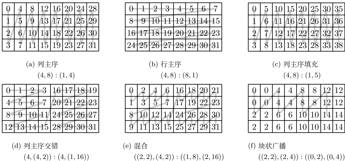
图 W.3: 与形状 (4, 8) 相容的布局示例, 绘制为 4 \times 8 矩阵。这些布局使用整数步幅与层次形状 (hierarchical shapes) 来定义对数据张量有用的函数。浅色线条沿布局偏移的总体顺序勾勒。
