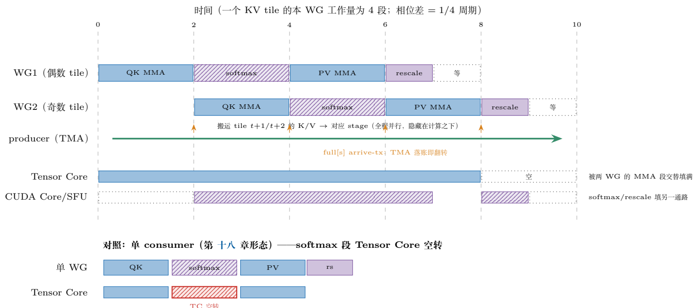
图 19.4: 双 consumer 的相位交错时序 (18.4.6 节统计性交错的图形化)。上: WG1/WG2 各按「QK MMA → softmax → PV MMA → rescale」四段推进自己的 KV tile 子序列，两 WG 相位差 1/4 周期——WG1 处于 MMA 段时 WG2 大概率处于 softmax/rescale 段；producer 的 TMA 全程并行，落账即 arrive-tx 翻转 full[s] 。中: Tensor Core 与 CUDA Core/SFU 两条资源条被两路计算交替填满（同步 mma.sync 做不到 WG 内重叠，靠两路独立流在硬件调度器上统计性交错）。下: 单 consumer (第 18 章形态) 的对照——softmax 段 Tensor Core 只能空转，这正是第二个 consumer 要填的洞。
