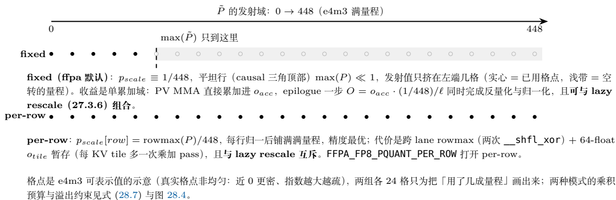
图 28.2: fixed 与 per-row 两种 p_{scale} 策略的发射域利用率 (27.3.5 节)。上: fixed 的 p_{scale} \equiv 1/448 是编译期常数, 平坦行的 \max(P) \ll 1 使发射值只占量程左端一小段, 其余量程空转——换来的是单累加域与「可与 lazy rescale 组合」; 下: per-row 用 \text{rowmax}(P)/448 把每一行拉满, 精度最优, 代价是跨 lane rowmax 归约与 64-float 的 o_{tile} 暂存, 且与 lazy rescale 互斥。
