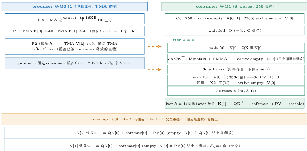
图 18.3: FA2 TMA + WS 的 producer/consumer 双流水时序 ( S_k=2, S_v=1, D=64 )。producer 的 P2 每轮先发 V 再预取 K; consumer 的 empty 释放点 (K 在 QK 后、V 在 PV 后) 决定了每个 stage 的可覆盖窗口。
