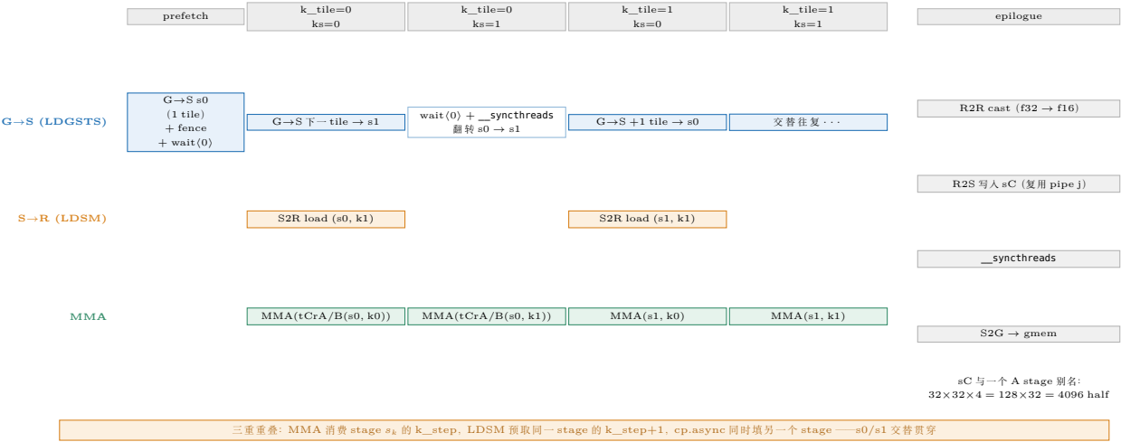
图 25.4: CuTe HGEMM 的 k_{\text{stage}} = 2 流水时序（含寄存器双缓冲）。上：G \rightarrow S（LDGSTS）；中：S \rightarrow R（LDSM）；下：MMA。MMA 消费 stage s_k 的 k_step 时，LDSM 预取同一 stage 的 k_step+1 ， cp.async 同时填另一个 stage——三重重叠；左端 prefetch 一个 tile，右端 epilogue（ R2R \rightarrow R2S \rightarrow S2G ， sC 与一个 A stage 别名： 32 \times 32 \times 4 = 128 \times 32 = 4096 half）。
