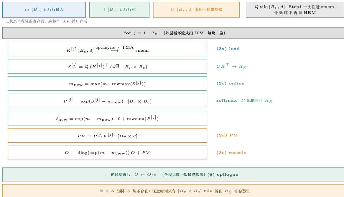
图 16.3: Attention 分块计算: 单个 Q 块 ( B_r 行) 流式扫过全部 T_c 个 KV 块 ( B_c \times d ), 每块依次执行 S[j] \rightarrow P[j] \rightarrow P[j]V[j] , 并把 (m, \ell, O) 三状态按式 16.12–16.17 联动更新, 循环结束后统一除 \ell 。步骤编号对齐 flash_attn.cuh L48–59 的执行流程。
