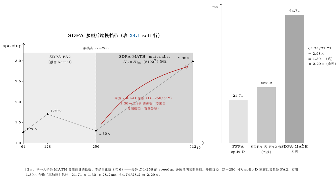
图 34.1: 参照系视角看表 34.1 的 self 行。左: SDPA 参照随 D 换挡——FA2 只覆盖 D \leq 256 , 更大 D 静默落到 MATH (materialize N_q \times N_{kv} 矩阵); 四个 speedup 点 (1.26/1.70/1.30/2.98×) 落在换挡带上, D=512 的跳变与 kernel 无关。右: D=512 的 2.98× 归因——以 D=256 同家族 (split-D、FA2 参照) 实测 1.30× 为真加速估计, MATH 参照自身再慢 \times 2.29 : 「3×」的大头是参照低效 (坑 6)。
