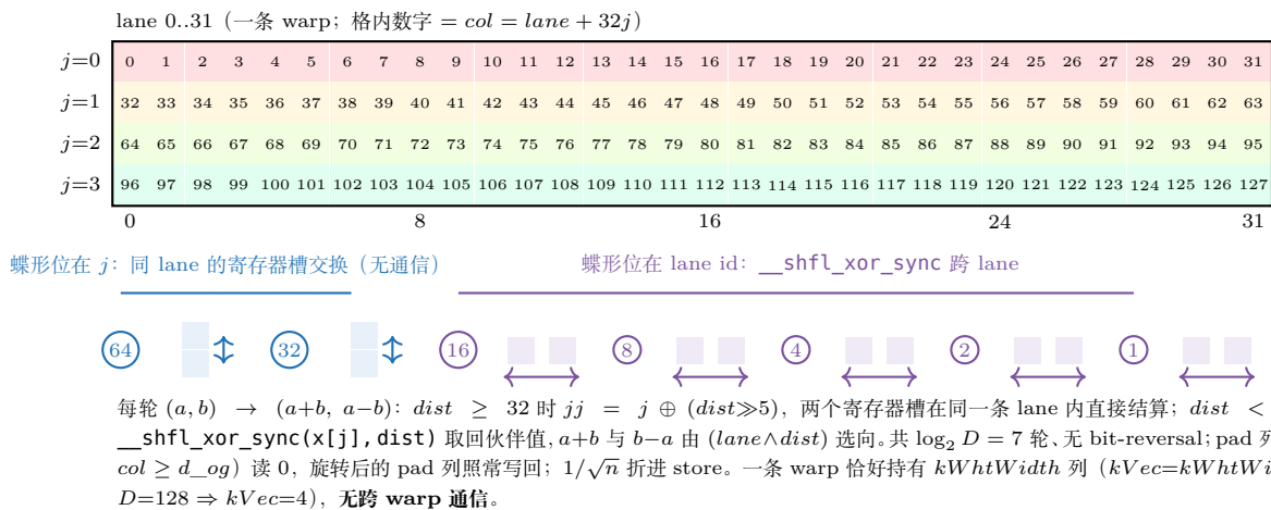
图 29.4: radix-2 蝶形的距离二分 (hadamard.cuh L40-92, 本例 D=128 、 kWhtWidth=D )。上: 列归属—— j 是寄存器槽、lane 是 warp 内线程, 格内数字 \text{col} = \text{lane} + 32j 满足索引律, 右下角 127 = \text{size} - 1 ; 一条 warp 覆盖整行 128 列。下: 七轮的「距离阶梯」—— \text{dist} \geq 32 的 bit 落在 j 上 (同 lane 两个寄存器槽直接加减, 无通信), \text{dist} < 32 的 bit 落在 lane id 上 ( __shfl_xor_sync 跨 lane); 每轮一个 bit, 1/\sqrt{n} 折进 store。
