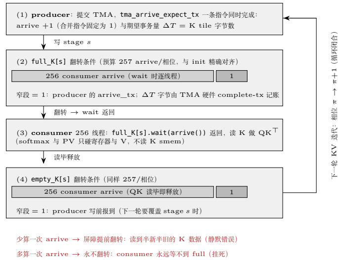
图 18.1: 固定 stage s 上 full/empty 两张屏障的相位收支循环 (式 18.5 与式 18.6 的图形化)。每轮 KV 迭代: producer 提交 TMA 时用 tma_arrive_expect_tx 一条指令完成「 arrive + 1 」与「声明 \Delta T 」两件事, TMA 硬件搬完后自动 complete-tx 记账; consumer 256 线程在 full_K[s].wait() 时各贡献一份 arrive ( 256 + 1 + tx 构成翻转条件), 读毕 K 再各 arrive 一次释放 empty_K[s] , producer 下一轮写前补上第 257 份。两边的 arrive 预算都是 257/轮, 与 init 值精确对齐——多算一次挂死、少算一次静默错。窄段为可读放大, 实际只占 1/257 。
