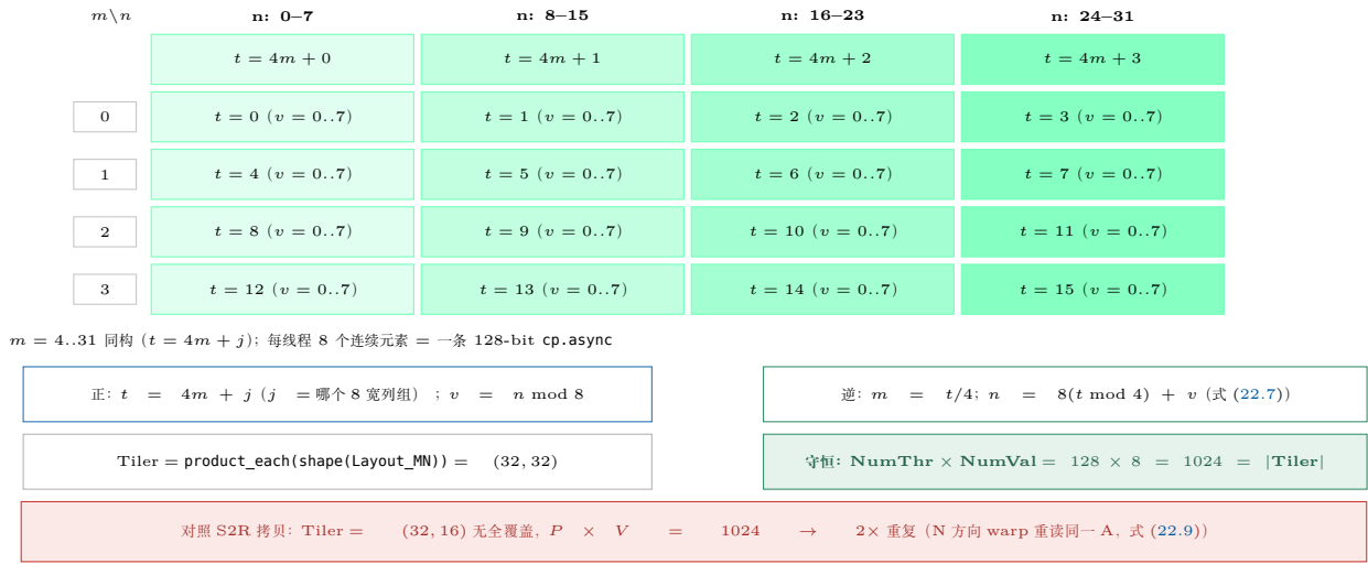
图 22.5: thread×value 网格：G→S 拷贝把 32 × 32 的 tile 划成 t = 4m + j 的网格，每个线程搬 8 个连续元素（一条 128-bit cp.async）。同一划分用 MN 语言或 TV 语言描述是等价的（式 (22.6) 与式 (22.7)）；本章测试 case A/B 对 1024 个 (t, v) 对与 4096 个坐标逐一核对了这两组公式。
