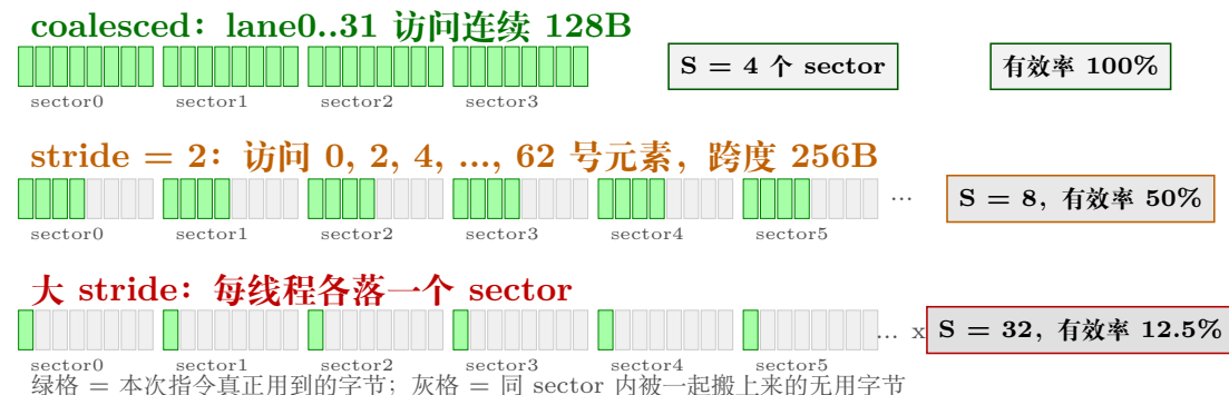
图 4.1: coalescing 与非合并访存对比 (fp32, 每格 4B, 一个 sector 8 格 32B): coalesced 一条指令落 4 个 sector 有效率 100%; stride=2 落 8 个、50%; 大 stride 每线程各占一个 sector、仅 12.5%——事务粒度是 32B sector, 无用字节照样从 HBM 搬上来。
