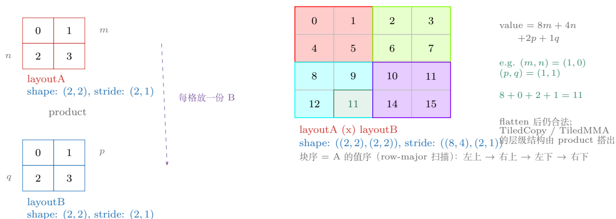
图 21.10: layout product: A 的每个坐标位放一份 B 的拷贝 (块偏移 = A 的线性序号 \times size(B)), 得到嵌套布局 ((2,2), (2,2)):((8,4), (2,1))。行值 0,1,4,5 / 2,3,6,7 / ... 的「块拷贝拼接」排布即 product 的几何签名——它不是 row-major。重建自 @ 竹熙佳处《写给大家看的 CuTe 教程: Layout Product & Divide》。
