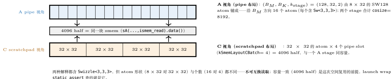
图 22.4: epilogue scratchpad: 同一块 4096 half 的 smem、两种布局视图 (hgemm.cuh L1001)。上条带是 A 的 pipe 解释——(128,32) 的 stage 按 8 \times 32 的 SW128 atom 沿 B_M 切成 16 段; 下条带是 C 的 scratchpad 解释—— 32 \times 32 的 atom \times 4 个 pipe slot ( kSmemLayoutCBatch = 4)。中间那条带是两者共用的地址带： sC 拿到的只是 sA(_, _, ismem_read).data() 这个裸指针，没有 Tensor 类型转换，重复的只是「同一段地址的两种读法」。
