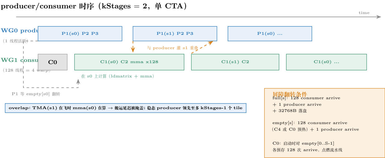
图 15.4: producer/consumer 时序: C0 预热点燃流水线；此后 producer 的 TMA 提交与 consumer 的 ldmatrix+mma 在不同 stage 上重叠，搬运延迟被计算掩盖；稳态 producer 领先至多 kStages-1 个 tile。
