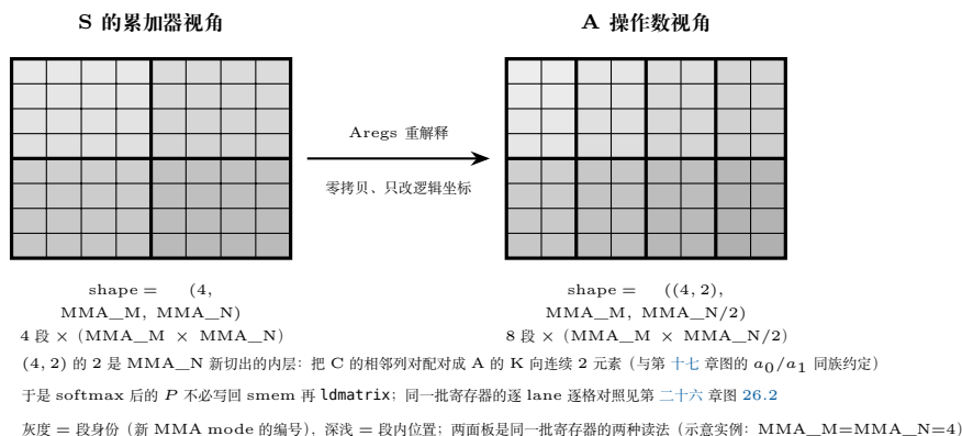
图 20.3: 零拷贝的寄存器重解释 (19.4.3 节 quote 块中 convert_layout_acc_Aregs (L300–305) 的模式级示意)。左: S 的累加器 layout 是 (MMA=4, MMA\_M, MMA\_N) ——4 个 MMA 重复段, 每段 MMA\_M \times MMA\_N ; 右: 同一批寄存器被读成 ((4, 2), MMA\_M, MMA\_N/2) ——沿 MMA\_N 切一刀得到 (2, MMA\_N/2) , 切出的 2 与原来的 4 配对成新的 8 段 MMA mode, 正是 PV 的 A 操作数所需的「K 向连续 2 元素」(与第 十七 章旗舰图的 a_0/a_1 配对同族)。数据一个比特都没动: 只是坐标重排, softmax 后的 P 因此不需要写回 smem 再 ldmatrix 。
