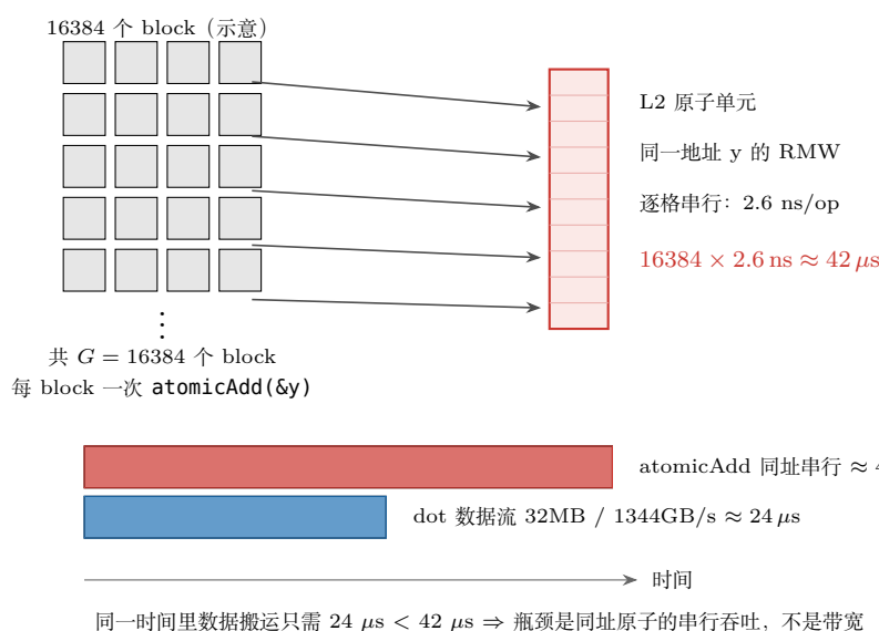
图 3.5: 全局原子串行化的几何证据： G = 16384 个 block 的 atomicAdd 全部汇入同一地址 y 的 L2 原子单元窄队列逐格串行（ 2.6\text{ ns/op} ，共约 42\mu\text{s} ），长于 dot 本身的数据流时间（约 24\mu\text{s} ）。
