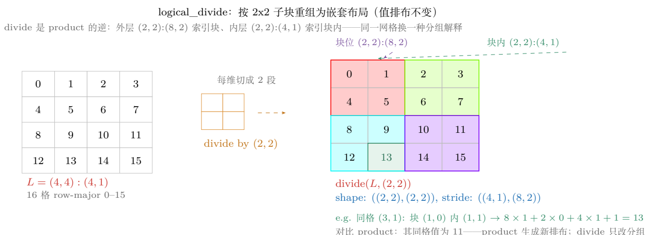
图 21.11: logical_divide: 按 2 \times 2 子块把 (4,4):(4,1) 重组为 ((2,2), (2,2)):((4,1), (8,2)) (CuTe 实测的 zipped 形式: 块内 mode 在前、块位 mode 在后)——值排布不变 (仍 row-major), 改变的只是索引方式 (一组 (4,1) 索引块内、一组 (8,2) 索引块位)。与上图对比: 同物理格 (3,1) 的 product 值为 11 (新排布), divide 后仍为 13 (原排布)。重建自同上文。
