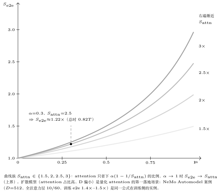
图 34.2: 端到端摊销曲线族 (式 34.3): 单算子 S_{\text{attn}} 换算到管线收益由 attention 占比 \alpha 封顶。 \alpha=0.3 、 S_{\text{attn}}=2.5x 时只剩 1.22x; \alpha \rightarrow 1 的渐近线即 S_{\text{attn}} 。
