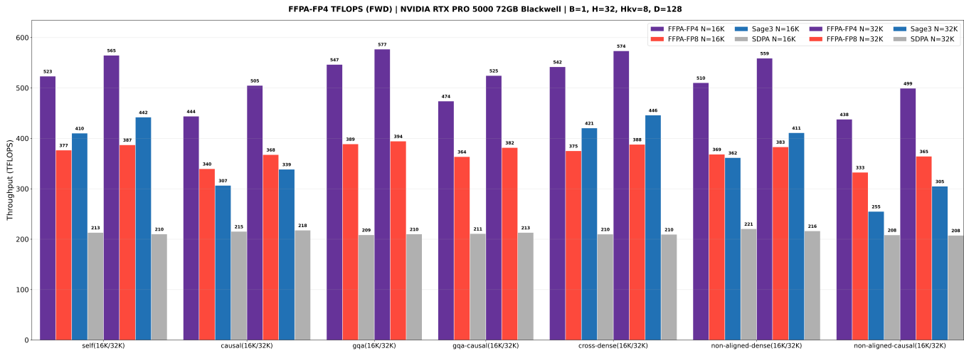
图 34.6: 本机 PRO 5000 复测 (fp4, 同形状, bench_fp4.py, 2026-09-16): FFPA-FP4 (紫) 在所有场景领先; Sage3 在 GQA 行缺席 (不支持), causal 行其 rel_err 达 0.59 (早期行 e2m1 噪声无 hybrid 抑制) 而 FFPA-FP4 为 0.14。
