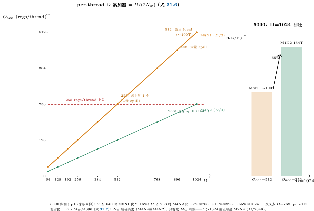
图 31.2: 寄存器墙的定量视图。左: per-thread O 累加器 = D/(2N_w) (式 31.6) ——M8N1 的 D/2 在 D=512 达 256 (超 255 上限 1 个, 边缘 spill)、 D \geq 896 大量 spill、 D=1024 溢出 local memory (~100T); M4N2 的 D/4 同点仅 256 (154T)。右: 5090 实测 D=1024 吞吐对比 (+55%)。下: per-SM 池占比 D \cdot M_w / 4096 (式 31.7) 中 N_w 精确消去——加 N-warp 不降总量, D > 1024 只能走 M2N4。
