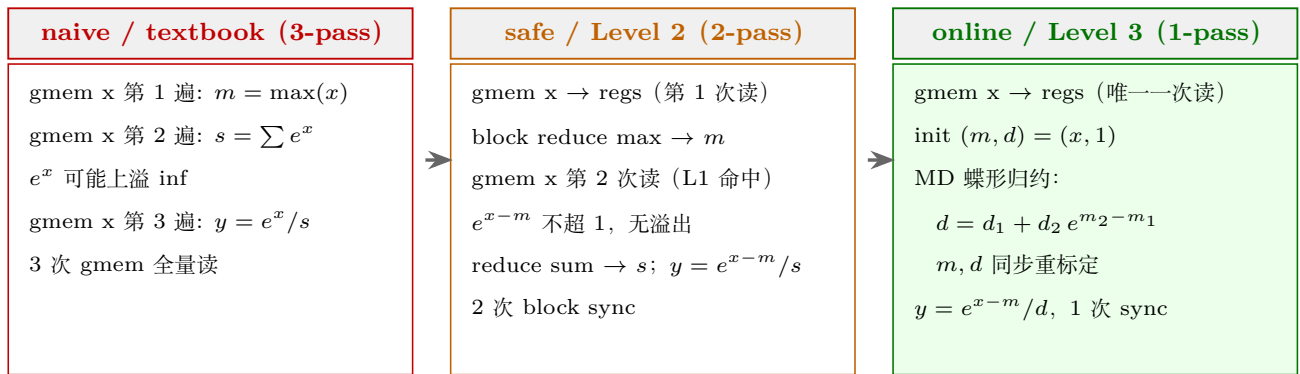
图 5.3: Softmax 三级递进的 3-pass \rightarrow 2-pass \rightarrow 1-pass 数据流：左为教科书三遍扫描（无 max 减法， e^x 可能上溢）；中为 safe 版两次归约；右为 online 版 (m, d) 状态一次融合归约。
