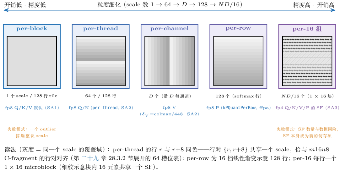
图 28.1: 量化粒度谱系五联图 (表 28.2 的可视化, 缩略网格为 16 行 \times 16 列)。从左到右: per-block 整块共享 1 个 scale; per-thread 按 C-fragment 行对 \{r, r+8\} 分档 (128 行块共 8 \times 8 = 64 个, 零 shuffle 消费); per-channel 沿 D 每通道一个; per-row 每 softmax 行一个 (128 个); per-16 每行一个 1 \times 16 microblock (NVFP4 的 SF)。顶部双向轴是整条谱系的 trade-off: 粒度越细精度越高, 但 scale 的存储、传递与消去开销同步上涨, 且必须与 MMA 的 fragment 布局对齐——谱系两端的失败模式分别是对 outlier 的脆弱性与 SF 自身的访存账。
