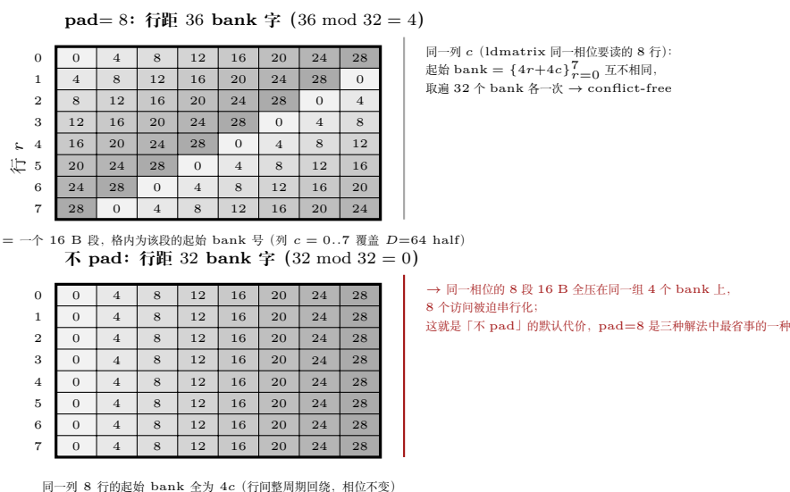
图 17.3: pad=8 与不 pad 的 ldmatrix bank 相位对照 (16.4.2 节 smem 三段布局中 pad 分析的图形化)。上: k\text{SmemStride} = D + \text{pad} = 72 half 时一行 144 B = 36 bank 字, 第 r 行相对第 0 行整体错开 36r \bmod 32 = 4r 个 bank; 任一行 c (ldmatrix 同一相位读的 8 行) 的起始 bank 为 \{4r + 4c\} , 取遍 32 个 bank 各一次——8 段 16 B 恰好铺满全部 bank, conflict-free。下: 不 pad 时行距 128 B = 32 bank 字, 整周期回绕后 8 行起始 bank 全为 4c , 同一相位的 8 段 16 B 压在同一组 4 个 bank 上串行化。格内数字为「该 16 B 段的起始 bank 号」, 灰度按 bank 号每 4 个一档。
