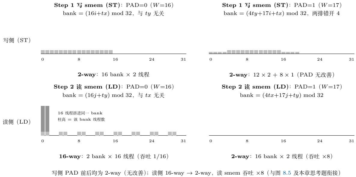
图 8.4: bank 占用直方图 (2 指令 \times 2 配置，每格为 32 bank 的线程计数，取 i = j = 0 的一条指令)：写侧 (ST) PAD=0 与 PAD=1 都是每 bank 至多 2 线程——写侧 PAD 前后无改善；读侧 (LD) PAD=0 时 32 线程挤进 2 个 bank (16-way，深灰柱)，PAD=1 后 tx 每加 1 bank 前进 4，16 个 bank 各 2 线程 (2-way)。图 8.5 讲「步长 64B \rightarrow 68B 为何打破对齐」，本图给出两指令两配置的完整占用结果。
