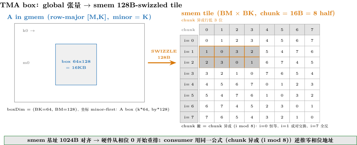
图 15.3: TMA box: descriptor 以 minor-first 坐标指定 64 × 128 的 2D 搬运块，落盘时按 SWIZZLE_128B 原子（16B chunk 号与行低 3 位 XOR）重排；smem 基址 1024B 对齐保证硬件从相位 0 开始重排，consumer 的软件公式才能按零相位逆推。
