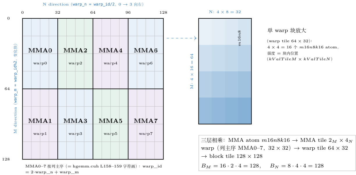
图 12.6: MMA warp 2 \times 4 排布 (左, 128 \times 128 block tile, 浅色 = warp 身份): MMA0–7 按列主序——N 向 MMA0/2/4/6、M 向 MMA1/3/5/7 ( \text{warp\_m} = \text{warp\_id} \% 2 变化快), 与 hgemma.cuh L158–159 原字符画一致; 每 warp 块内 4 \times 4 个 m16n8 atom 小格。右: 单 warp 块放大 (warp tile 64 \times 32 , 蓝深 = atom 块内位置); 侧栏三层记号 B_M = 16 \cdot 2 \cdot 4 、 B_N = 8 \cdot 4 \cdot 4 。
