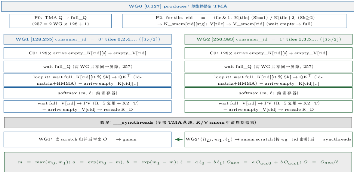
图 19.5: FA3 双 consumer 的角色图: WG0 单线程提交 TMA, 并按 cid = tile \& 1 把 K/V 投递到两个独立 bank; WG1/WG2 各自遍历一半 KV tile、维护独立 partial 与独立流水; 收尾在 smem scratch 上做一次稳定归并后由 WG1 写出。
