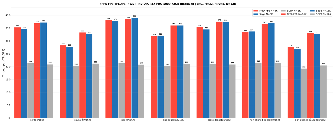
图 34.5: 本机 PRO 5000 复测 (fp8, D=128 fp16, H32/Hkv8, bench_fp8.py 默认 preset, 2026-09-16): 七个场景 \times 8K/16K。与 Sage 总体打平、互有胜负 (self 8K FFPA +2.0%, gqa 16K Sage +1.4%, 最差差 2.6%); 与 5090 图的形态一致, 绝对 TFLOPS 低 \sim 15\% (SM 数与功耗包络差异)。
