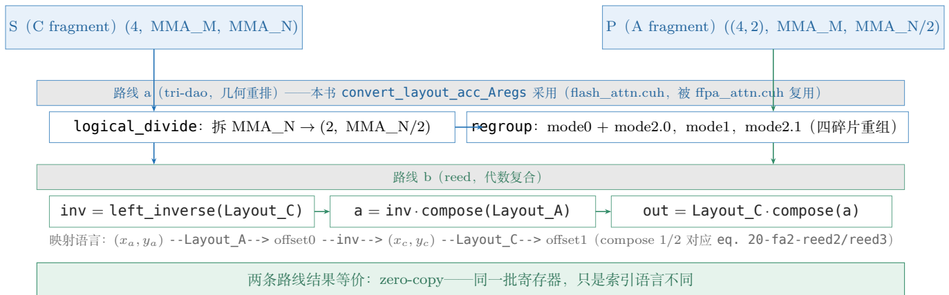
图 21.5: FA2 的 P 矩阵布局转换: tri-dao 的几何重排与 reed 的代数复合两条路线, 结果等价。本书 flash_attn.cuh 的 convert_layout_acc_Aregs (被 fpa_attn.cuh 复用) 采用的是几何路线。
