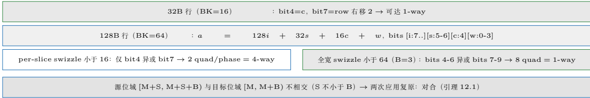
图 13.6: XOR 位运算示意: 源位域 (行号低位) 经右移 S 异或到目标位域 (chunk 号)。行宽决定「有多少行号位能进入 bank 位 [2,7)」, 从而决定可达到的最小冲突度; 源/目标位域不相交 ( S \geq B ) 保证对合性 (引理 12.1)。
