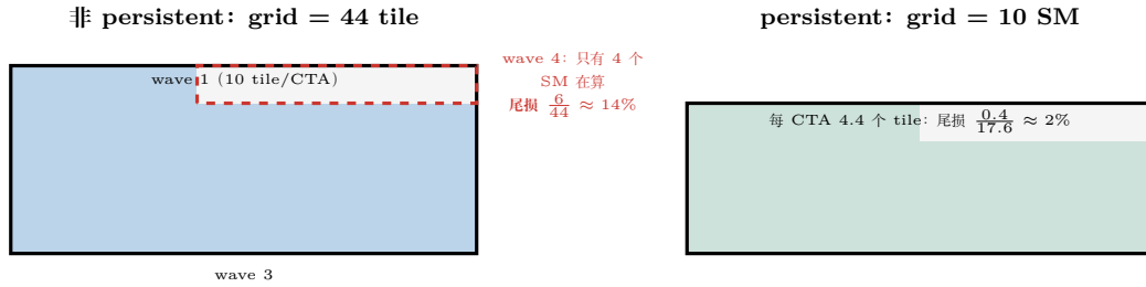
图 28.5: wave 量化尾损示意 (10 个 SM、44 个 tile 的缩小模型)。左: 非 persistent launch 按整 wave 调度, 最后一个 wave 只有 4 个 SM 在算, 其余空转满一个 tile 时长; 右: persistent CTA 把 grid 收缩到 SM 数, 每个 CTA 串行处理 \lceil 44/10 \rceil 或 \lfloor 44/10 \rfloor 个 tile, 不均衡被压缩到最后一个 tile 的零头。真实场景 (110 SM, H=32/N=8192 ) dense 收益 +2%~6%; causal 反向 ——tile 负载前轻后重, 线性分配会把重 tile 固定在同一批 CTA 上 (实测 -9% ~ -21%), 此时必须回退全量 grid 让硬件调度器自然均衡。
