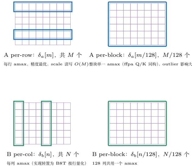
图 30.2: 四种 scale 粒度组合 (上排 A, 下排 B)。蓝框 = A 侧 scale 统计范围, 绿框 = B 侧。粒度越粗, scale 存储/查表越省 (per \times per-block 每 tile 只查两个标量), 但 outlier 的影响越大——一个大值会放大整块的量化步长, 其余小值全部落入低精度区间。四种组合在 API 里是一个枚举, 主 kernel 用 if constexpr 编译期剔除, 运行时零分支开销。
