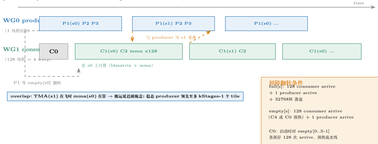
图 15.4: producer/consumer 时序: C0 预热启动流水线; 此后 producer 的 TMA 提交与 consumer 的 ldmatrix+mma 在不同 stage 上重叠, 搬运延迟被计算掩盖; 稳态 producer 领先至多 kStages-1 个 tile。
