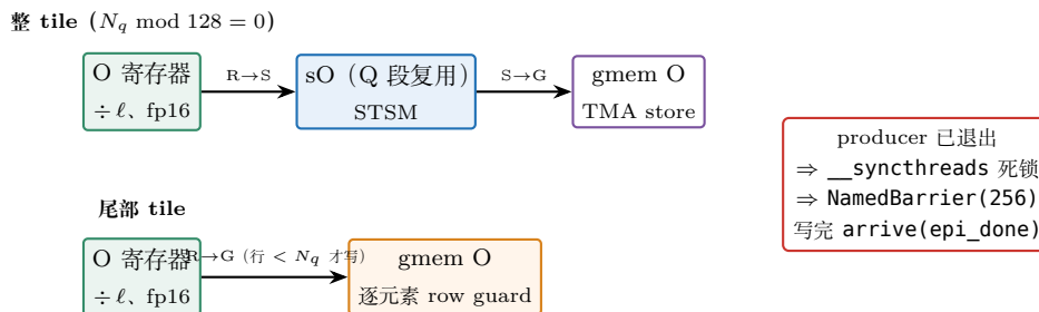
图 28.6: Epilogue 双路径。整 tile 走 R \rightarrow S \rightarrow G : STSM 把 O fragment 写进 (已闲置的) Q smem 段, NamedBarrier 后由一个线程发射 TMA store——与装载对称的「反向 TMA 全链」。尾部 tile 行数不足 128, STSM/TMA 的整块写会越界, 退化为带行 guard 的 R \rightarrow G 。
