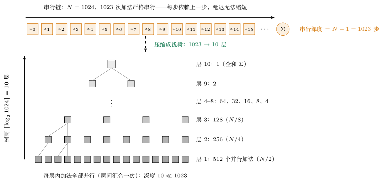
图 3.1: 串行依赖链与二叉归约树对照 ( N = 1024 )：上半为串行链——1023 次加法严格依序，无论启动多少线程延迟都无法隐藏；下半为两两相加的归约树——树高 \lceil \log_2 N \rceil = 10 层，每层内加法全部并行（灰度自底向上随节点数减半渐浅）。深度从 N-1 压缩到 \log_2 N ，代价是「谁跟谁相加」成为必须显式约定的结构信息。
