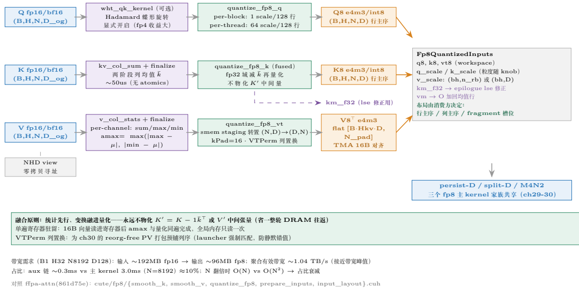
图 35.5: fp8 前处理链全景: 三泳道 (Q/K/V) 各自的统计 → 变换 → 量化 kernel 与输出 workspace 布局。smoothing 与量化融合在同一 kernel 内 (无中间落盘); V^T 的列 pad 兼顾 TMA 16B 对齐与置换写。
