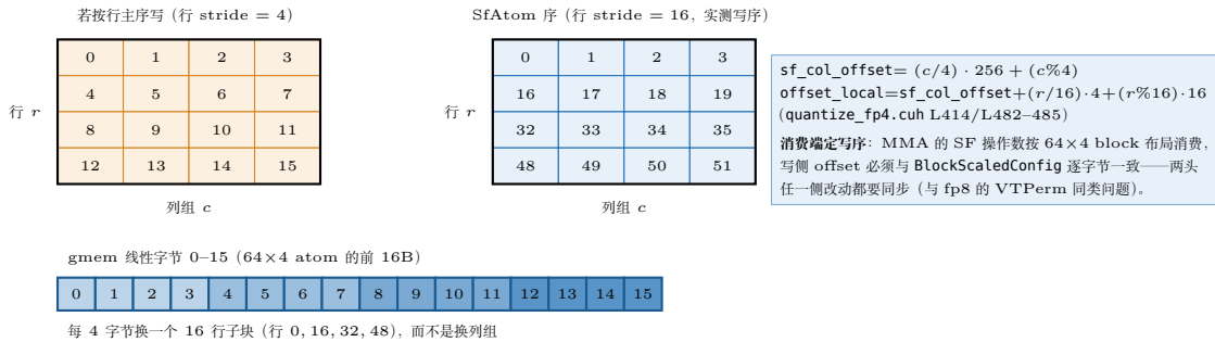
图 38.3: SF 字节的写序由消费端决定 ( V^T 量化链)。同一 (r, c) 单元格在行主序假设下偏移 4r + c , 在 SfAtom 序下偏移 16r + c : 每 4 个列组构成 64 \times 4 的 256B atom, atom 内按 16 行子块交错。写侧 (sf_col_offset/offset_local) 与 MMA 的 BlockScaledConfig 必须逐字节一致。
