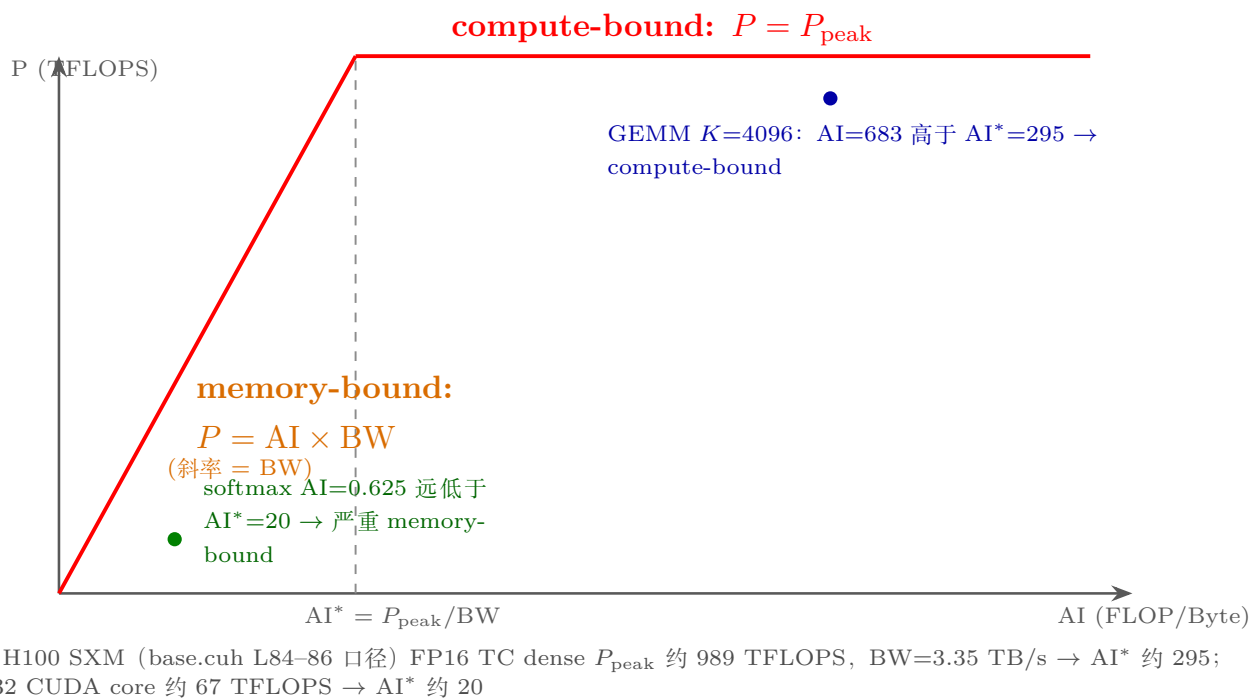
图 2.3: Roofline 模型: P = \min(P_{\text{peak}}, AI \times BW) , 脊点 AI^* = P_{\text{peak}}/BW 。GEMM K=4096 ( AI=683 ) 落在计算屋顶, softmax ( AI=0.625 ) 落在带宽斜线区。
