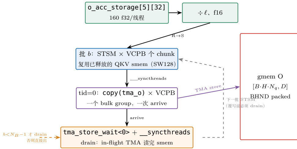
图 29.3: epilogue 的批量写出协议 (D=320: 5 个 v_chunk 一批, VCPB = k_V \text{ChunksPerBatch} )。O 累加器除以 \ell 转 f16 后, STSM 把每 chunk 的 128 \times 64 分量暂存进复用的 QKV smem; tid=0 对批内所有 chunk 发 TMA store 并提交一个 bulk group。灰色回边是 drain race 的约束: 下一批的 STSM 要覆写同一段 smem, 必须等 in-flight TMA 读完 (tma_store_wait<0> 只对发射线程有意义, 配套 __syncthreads 让全 CTA 对齐; 末批免等直接收尾)。对比 WS 教学版的逐元素寄存器直写 gmemo: 指令数从每线程 32C 次标量 store 降到 VCPB 次 STSM + 一次 bulk 提交。
