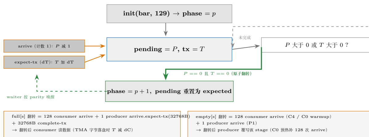
图 14.6: mbarrier 状态机: arrive 与 tx 两个独立的计数条件同时归零才翻转相位; 翻转瞬间原子地重置 pending 为 expected。下半部分给出 full[s] 与 empty[s] 各自的翻转条件。
