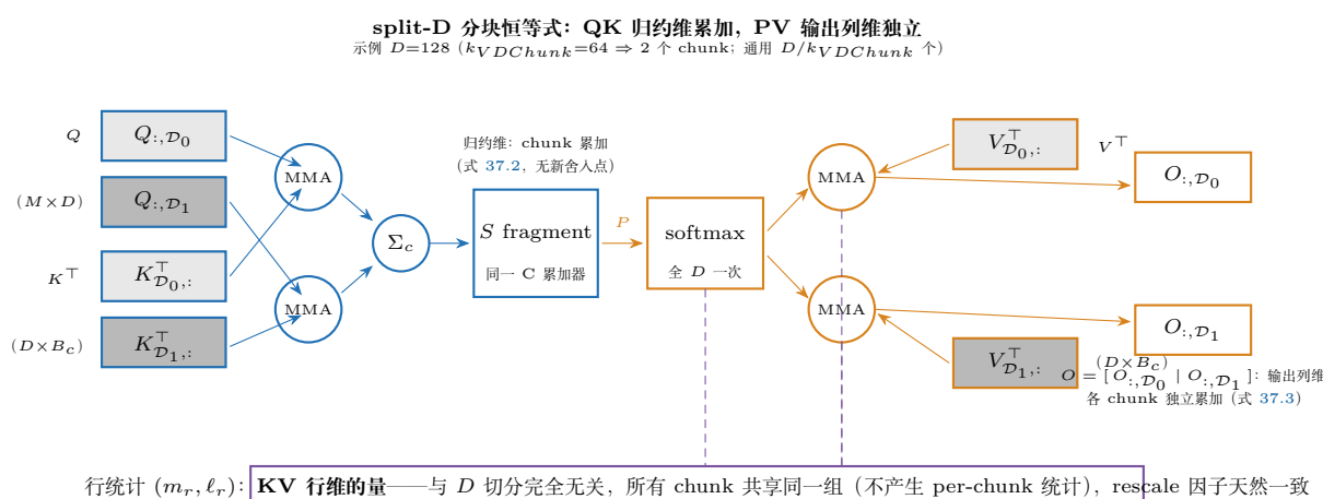
图 37.1: split-D 分块恒等式的数据流 (30.3.1 节)。QK 侧： D 是归约维，各 chunk 的 Q_{:, \mathcal{D}_c} K_{\mathcal{D}_c, :}^\top 累加进同一个 S fragment (式 37.2, f32/s32 累加，不引入新舍入点)；PV 侧： D 是输出列维，各 chunk 独立累加出 O_{:, \mathcal{D}_c} 列段 (式 37.3)，无任何合并。softmax 的行统计 ( m_r, \ell_r ) 是 KV 行维的量——与 D 切分完全无关，所有 chunk 共享同一组 (灰色 = chunk 身份，两图同语义)。
