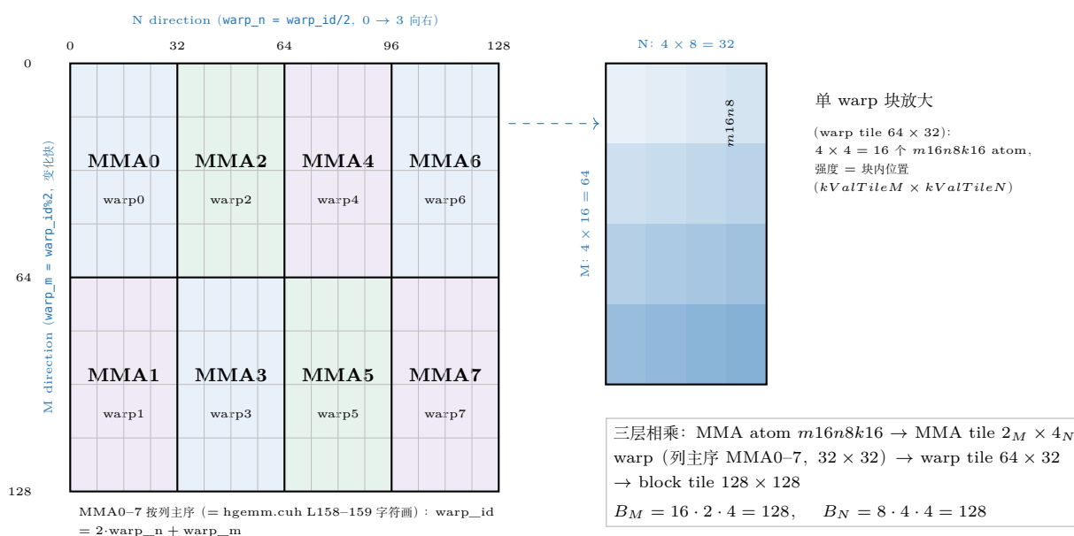
图 12.6: MMA warp 2 \times 4 排布 (左, 128 \times 128 block tile, 浅色 = warp_id): MMA0–7 按列主序——N 向 MMA0/2/4/6、M 向 MMA1/3/5/7 ( \text{warp\_m} = \text{warp\_id} \% 2 变化快); 每 warp 块内 4 \times 4 个 m16n8 atom 小格。右: 单 warp 块放大 (warp tile 64 \times 32 , 蓝深 = atom 块内位置); 侧栏三层记号 B_M = 16 \cdot 2 \cdot 4 、 B_N = 8 \cdot 4 \cdot 4 。
