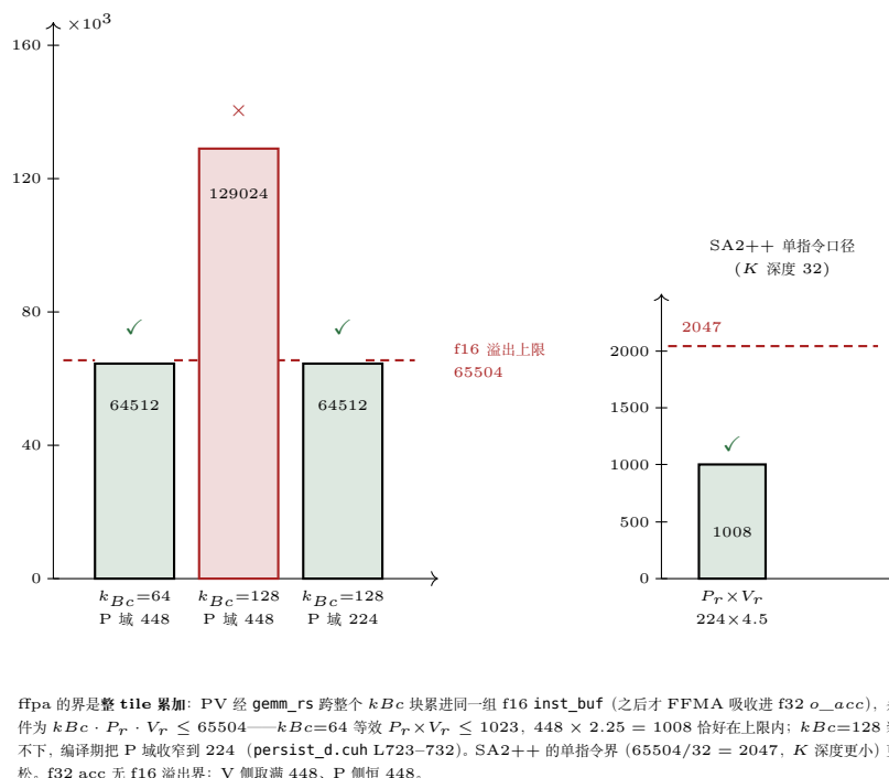
图 36.1: f16 PV 累加器的整 tile 域预算 (式 36.4)。条形为 kBc \times P_r \times V_r : kBc=64 与「 kBc=128 + P 域自动收窄到 224」都恰为 64512, 接近 65504 上限; kBc=128 且 P 仍 448 则 129024 约 2 倍超限。右: SA2++ 按单条 MMA ( K=32 ) 核算的界 2047 更松 ( P_r=224, V_r=4.5 双侧收紧)。f32 acc 路径无此约束。
