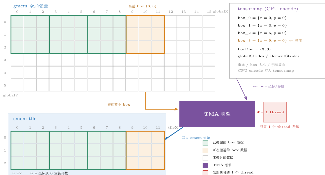
图 24.5: TMA copy 数据流：全局张量按 3 \times 3 box 切分（绿 = 已搬完、橙 = 搬运中），各 box 起始坐标与张量描述由 CPU encode 进 tensormap ，TMA 引擎据此定位整块搬运。发起与搬运分离——单线程发起拷贝指令，box 内全部元素由 TMA 引擎异步搬入 smem ；数据落地后改用 tile 局部坐标，与全局坐标脱钩。重建自 @ 竹熙佳处《写给大家看的 CuTe 教程：TMA Copy》。
