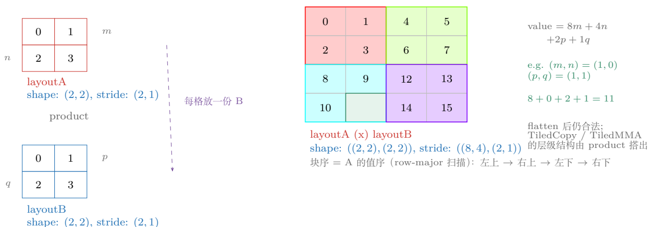
图 21.10: layout product: A 的每个坐标位放一份 B 的拷贝 (块偏移 = A 的线性序号 \times size(B)), 得到嵌套布局 ((2,2), (2,2)) : ((8,4), (2,1)) 。行值 0, 1, 4, 5 / 2, 3, 6, 7 / ... 的「块拷贝拼接」排布即 product 的几何特征——它不是 row-major。重建自 @ 竹熙佳处《写给大家看的 CuTe 教程: Layout Product & Divide》。
