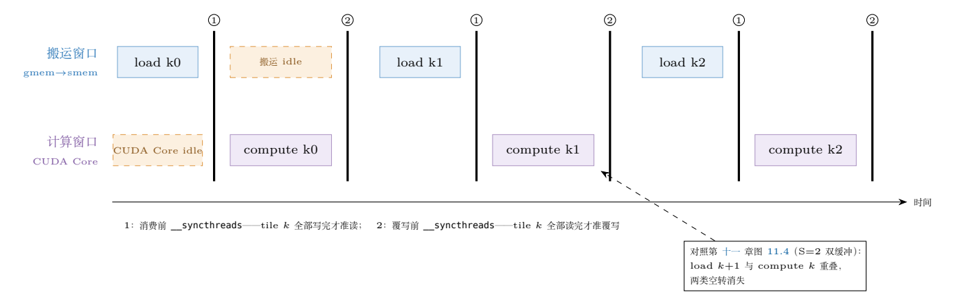
图 10.1: 单缓冲 k-slice 循环的双栅栏时序 (3 个迭代): load (蓝) → 栅栏 1 (消费前) → compute (紫) → 栅栏 2 (覆写前)。load 期间 CUDA Core 空转、compute 期间搬运单元空转——「搬一算一」串行使两个窗口无法重叠; 双缓冲 (图 11.4) 正是为消除这两类空转而设计。
