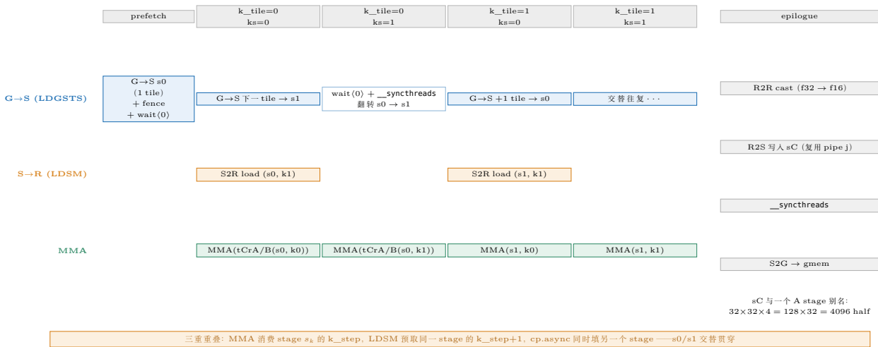
图 25.4: CuTe HGEMM 的 k_{\text{stage}} = 2 流水时序 (含寄存器双缓冲)。上: G \rightarrow S (LDGSTS); 中: S \rightarrow R (LDSM); 下: MMA。MMA 消费 stage s_k 的 k_step 时, LDSM 预取同一 stage 的 k_step+1 , cp.async 同时填另一个 stage——三重重叠; 左端 prefetch 一个 tile, 右端 epilogue ( R2R \rightarrow R2S \rightarrow S2G , sC 与一个 A stage 别名: 32 \times 32 \times 4 = 128 \times 32 = 4096 half)。
