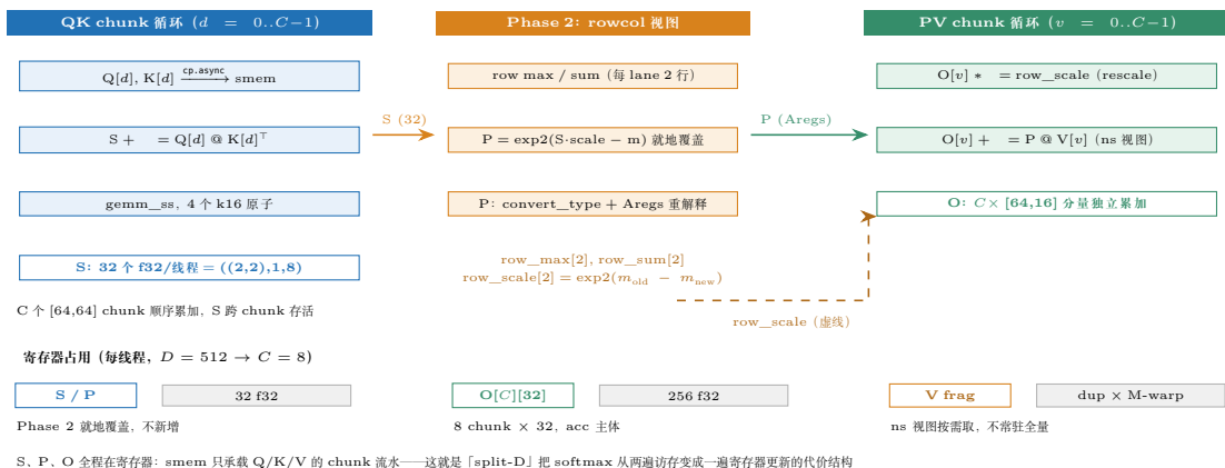
图 27.5: 双 TiledMma 的数据流: QK 沿 D 累加成 S (32 寄存器跨 chunk 存活), softmax 就地覆盖为 P , Aregs 重解释后交给 PV; O 的每个 chunk 分量独立 rescale 与累加, row_scale (虚线) 耦合两个循环。底部为寄存器占用: S/P 32、 O[C][32] 共 256 ( C=8 )、V fragment 按 M-warp 重复——smem 只承载 Q/K/V 的 chunk 流水。
