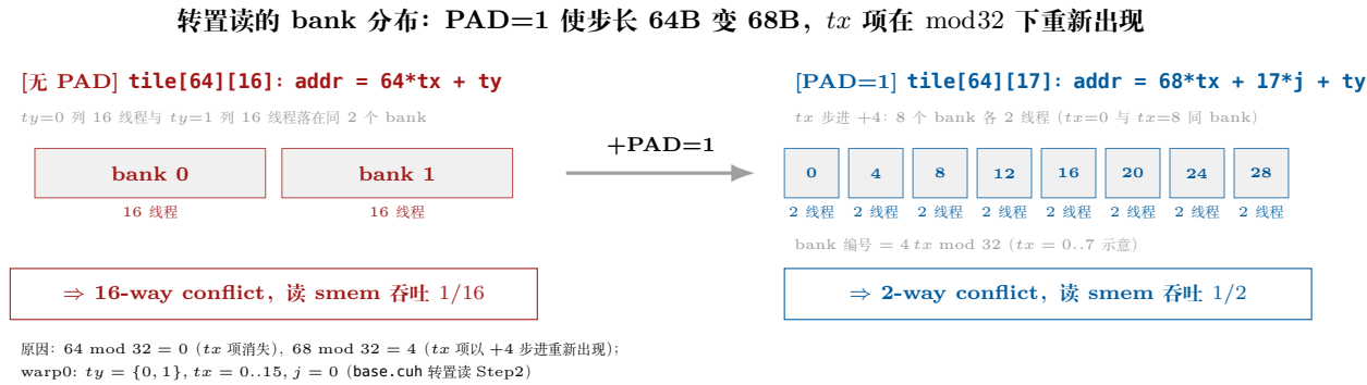
图 8.5: bank conflict vs padding—PAD=1 使步长 64B 变为 68B, tx 项在 mod 32 下重新出现, 16-way 冲突降为 2-way (读 smem 吞吐 1/16 → 1/2)。
