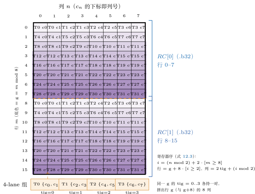
图 12.3: C fragment ( m16 \times n8 ) 寄存器布局 (式 12.3): 行 m = g = \text{lane} \gg 2 (底色 8 档, 行 0-7 与 8-15 由同批 lane 重复覆盖), 列对由 \text{tig} = \text{lane} \% 4 决定; RC[0] 装行 0-7、RC[1] 装行 8-15。底部: 4-lane 组内 \text{tig} = 0..3 各持一对 \{c_{2t}, c_{2t+1}\} , 拼齐一行 8 个 half——11.4.6 节 epilogue shuffle 的出发点。
