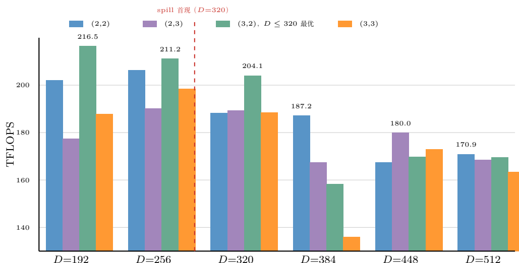
图 29.4: K/V 流水深度解耦实验 ( B=1/H=32/N=8192 , PRO 5000, 成对同轮)。 D \leq 320 : (S_K, S_V)=(3,2) 一致最优, 绿色系柱全面领先; D \geq 384 : 最优回落到 (2,2)/(2,3), (3,3) 在 D=384 降至 136.0 (比 (2,2) 低 27%)。红色虚线是分界: 恰在寄存器 spill 首次出现处 (表 见下, D=320 全组合 spill、 D \leq 256 零 spill)。
