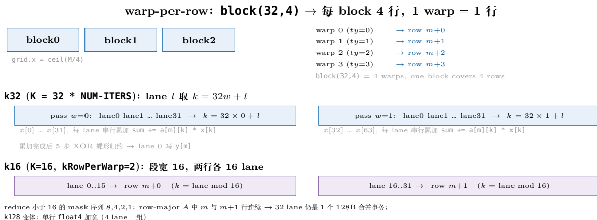
图 9.2: warp-per-row 的划分: k32 单行 32 lane 铺满、k16 双行各 16 lane 分段归约 (mask 8/4/2/1); k128 变体串行 float4 加宽。
