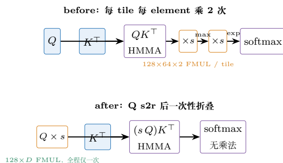
图 28.1: softmax scale 融合的数据流对照。上：传统路径，S 从 QK GEMM 出来后在 softmax 的 max/exp 两个 pass 各乘一次 s = \text{scale} \cdot \log_2 e ；下：融合路径， s 在 Q s2r 后一次性乘进 A-fragment (persist-D 使 Q 对整个 KV 循环不变)，HMMA 直接输出 log2 域分数，softmax 循环体内零 FMUL。等价性由式 (28.7)/(28.8) 保证；代价是 s \odot Q 的一次 fp16 重舍入。
