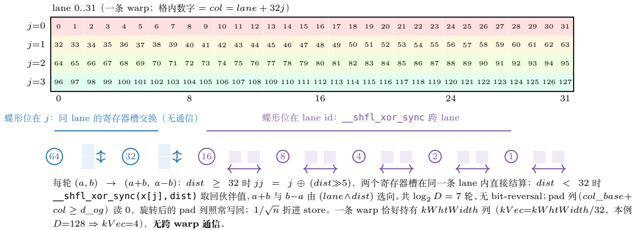
图 35.4: radix-2 蝶形的距离二分 (本例 D=128 、 kWhWidth=D )。上: 列归属—— j 是寄存器槽、lane 是 warp 内线程, 格内数字 col = lane + 32j 满足索引律, 右下角 127 = \text{size} - 1 ; 一条 warp 覆盖整行 128 列。下: 七轮的 距离二分 —— dist \geq 32 的 bit 落在 j 上 (同 lane 两个寄存器槽直接加减, 无通信), dist < 32 的 bit 落在 lane id 上 ( __shfl_xor_sync 跨 lane); 每轮一个 bit, 1/\sqrt{n} 折进 store。
