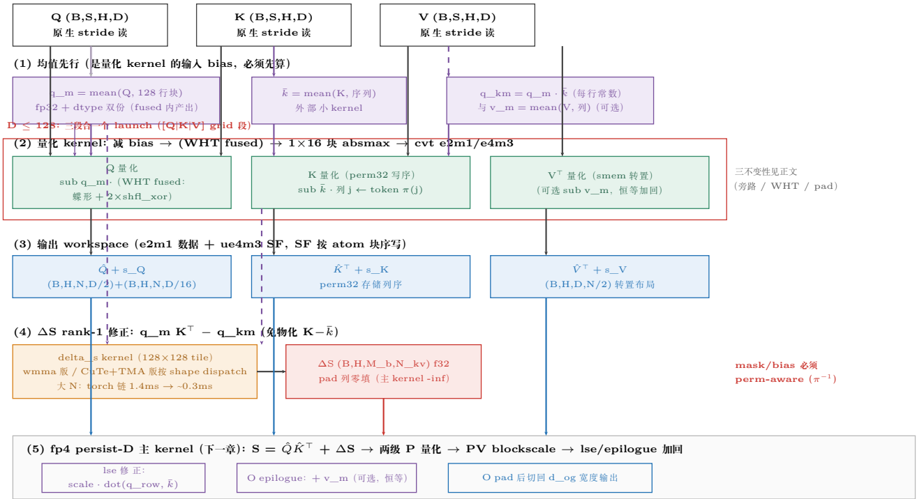
图 38.6: fp4 前处理链数据流 ( D \leq 128 走 fused 单 launch 路径): \bar{k}/q_m 均值先行的原因是它们是量化 kernel 的输入 bias; hadamard 下 q_m^{rot} 在 fused kernel 内同时产出。
