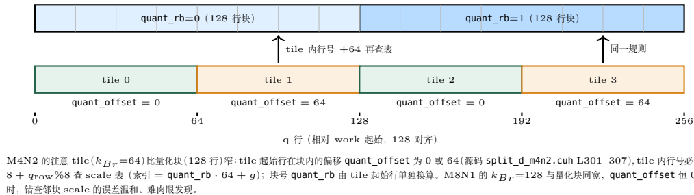
图 37.3: 量化 128 行块与 M4N2 注意 tile ( k_{Br}=64 ) 的错位关系。tile 1/3 的起始行落在量化块内的偏移 64 处, 其行号需先加 quant_offset 再查 per-thread scale 表; tile 0/2 偏移为 0。M8N1 的 k_{Br}=128 与量化块同宽, 不存在该映射。
