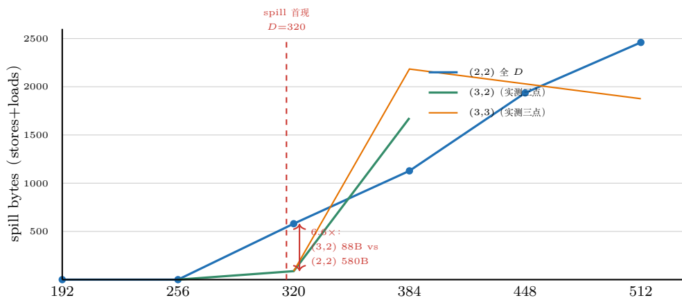
图 29.5: 寄存器溢出随 D 的增长 (nvcc -Xptxas -v, -O2, sm_120a, 各组合显式实例化)。 D \leq 256 全组合零 spill; D=320 (红色虚线) 是分水岭——所有组合达到 255 寄存器上限并开始溢出, 且 (3,2)/(3,3) 的 88 B 与 (2,2) 的 580 B 相差 6.6 倍, 与 TFLOPS 排序 (204.1 对 188.3) 完全同序; D \geq 384 后 spill 基线过千, stages 加深进一步推高溢出 ((3,2) 1676 B、(3,3) 2184 B, 均高于 (2,2)), 流水掩蔽收益被抵消, 最优组合回落 (2,2)。
