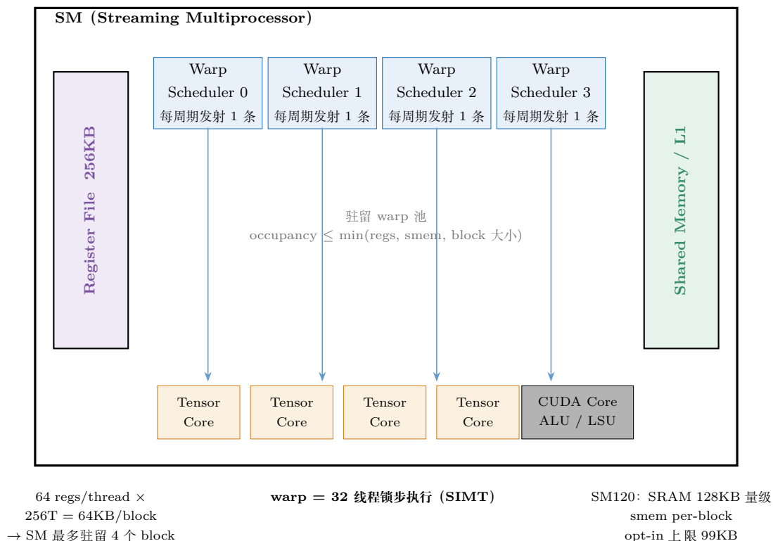
图 2.1: SM 内部结构示意 (Blackwell sm_120 口径): 顶部 4 个 warp scheduler (各每周期发射 1 条指令), 左侧 256KB 寄存器文件与右侧 smem/L1 共池 SRAM 共同钳制驻留 block 数, 底部 4 个 Tensor Core 与 CUDA Core 阵列执行发射来的指令。
