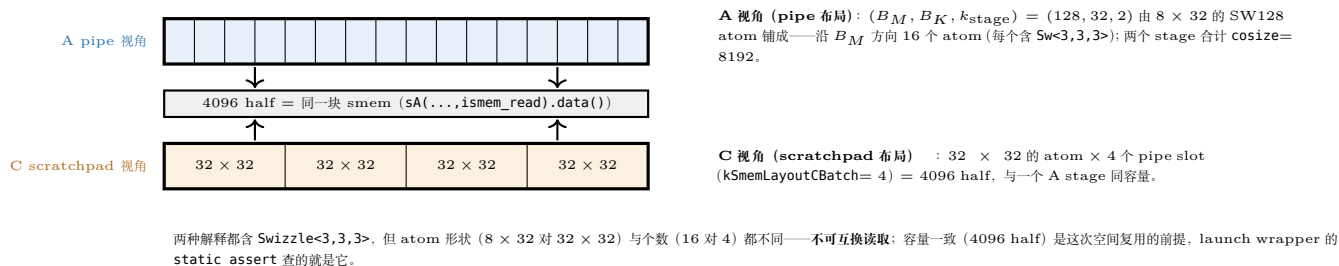
图 22.4: epilogue scratchpad：同一块 4096 half 的 smem、两种布局视图。上条带是 A 的 pipe 解释—— (128, 32) 的 stage 按 8 \times 32 的 SW128 atom 沿 B_M 切成 16 段；下条带是 C 的 scratchpad 解释—— 32 \times 32 的 atom \times 4 个 pipe slot ( kSmemLayoutCBatch=4 )。中间那条带是两者共用的地址带：sC 拿到的只是 sA(_,_,ismem_read).data() 这个裸指针，没有 Tensor 类型转换，重复的只是「同一段地址的两种读法」。
