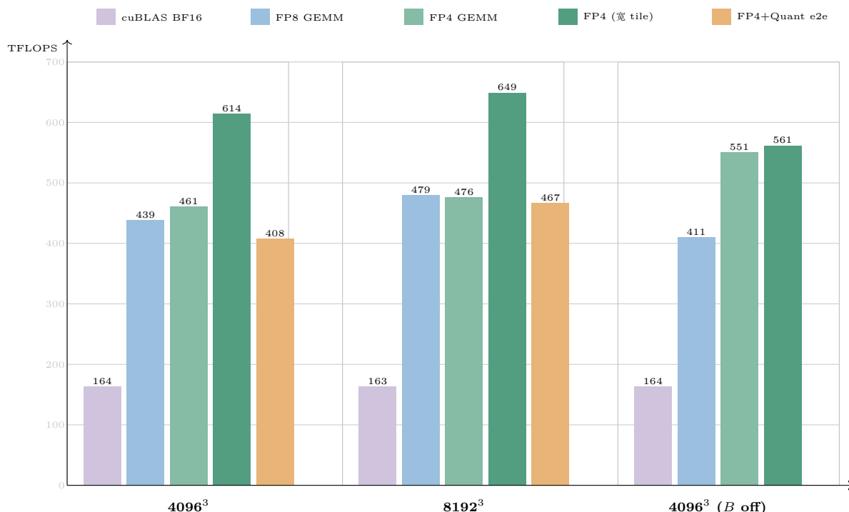
图 33.6: NVFP4 GEMM vs cuBLAS BF16 (PRO 5000, 越高越好)。三条读法：其一， kernel-only 口径下 FP4 只比 FP8 快 6 ~ 40%——库默认档 ( 128^2/s4 , 柱取口径: 4096^3 取扫描表 461 T, 8192^3 取默认档实测 476 T) 只快 6%, 宽 tile 档才快 40%, 远不是比特数暗示的 2\times ; 原因是本 kernel 走 bf16 输出、f32 累加, 且 BK=64 让 K 方向的算术强度下降 (表 33.1 的两条固定约束); 其二, 宽 tile ( 128\times 256 ) 是本章最大的单项收益 (+31%, 33.9.4 节), 也是 --bench 标准行在 MNK \geq 4096 上的自适应选择; 其三, e2e 口径下 FP4 反超 FP8 ( 4096^3 : 408 vs 187 T; 8192^3 : 467 vs 315 T) ——量化的写出字节数只有 FP8 的一半, B 侧重构后这个差距进一步扩大 (33.9.3 节); 第三组 ( B 离线) FP4 的 e2e 回到 551~561 T (FP8 为 411 T), 是各自 kernel 的 91 ~ 93%。
