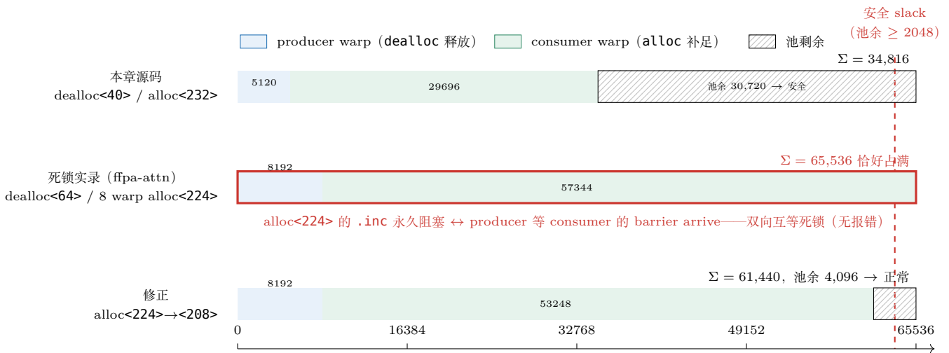
图 15.1: setmaxnreg 的 CTA 寄存器池三配置对照 (式 15.4, 每 SM 寄存器文件共 65,536 个 32-bit 寄存器): 条形按 \sum_w 32r_w 堆叠 producer (dealloc 释放) 与 consumer (alloc 补足) 两段, 红色虚线为工程安全界 (池余 \geq 2048 )。① 本章源码 dealloc<40>/alloc<232> : 5120 + 29696 = 34816 , 池余 30720, 安全; ② ffpa-attn 调优实录的死锁配置 dealloc<64> + 8 \text{ warp} \times \text{alloc<224>} : 8192 + 57344 = 65536 恰好占满——有效池 < 65536 , .inc 永远凑不齐而阻塞在 setmaxnreg 上, 与 producer 等 barrier arrive 形成双向互等死锁; ③ alloc 降到 208: 总 61440、池余 4096, 恢复正常。
