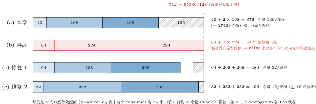
图 19.2: 65536 个寄存器按角色分配的三种方案 (式 19.5 与 18.3.4 节事故分析的图形化)。横轴为每线程等效配额 r_p + 2r_c \leq 512 = 65536/128 : (a) 本章 D=128 的 40 + 2 \times 168 = 376 , 余量 136/线程 (= 17408 个寄存器), 远离危险区; (b) 第 15 章那次事故的 64 + 2 \times 224 恰好等于 512——驱动对寄存器文件另有保留份额, 有效池小于 65536, 于是 consumer 卡在 setmaxnreg 、producer 卡在等 barrier arrive, 双向互等导致挂死 ; (c) 修复版的 480 与 496 分别留出 32 与 16 的每线程余量, 后者正是工程规则「 \geq 2048 slack」除以 128 的下界。
