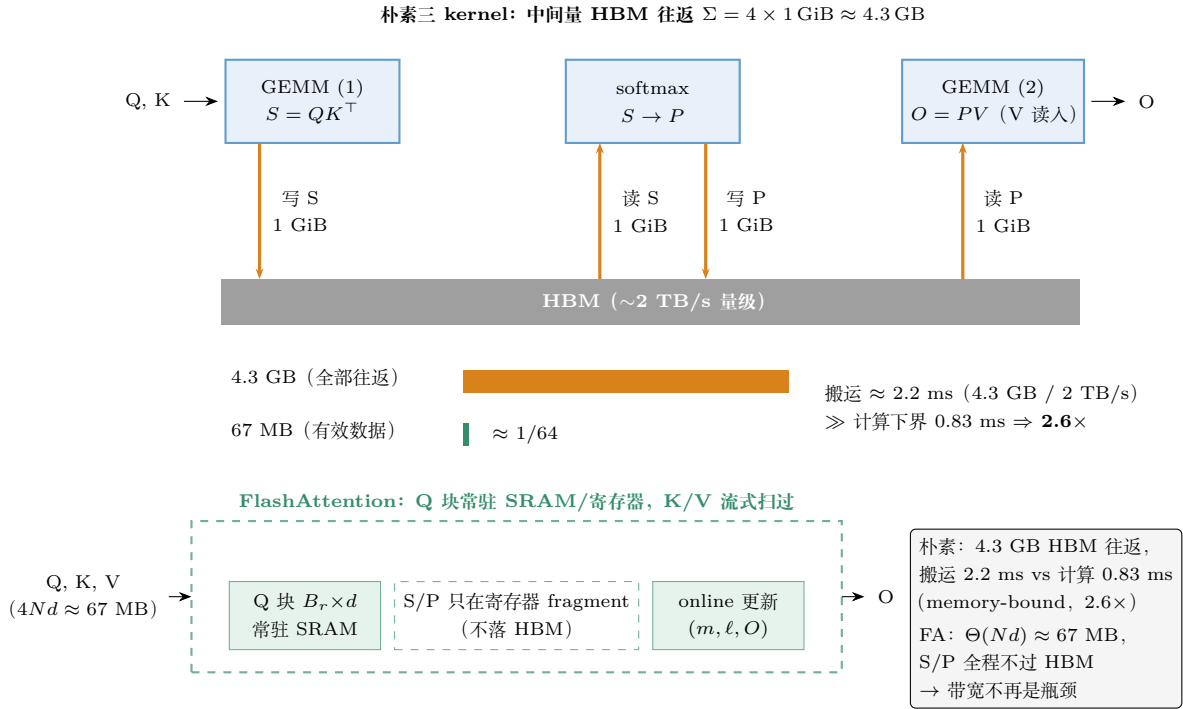
图 16.2: 朴素 attention 与 FlashAttention 的 HBM 往返流量对比 (15.3.3 节, B=1 、 H=32 、 N=4096 、 d=64 ): 上行三个 kernel 之间, S 与 P (各 \approx 1 \text{ GiB} ) 必须经 HBM 往返——写 S 、读 S 、写 P 、读 P 共 4 \times 1 \text{ GiB} \approx 4.3 \text{ GB} , 而有效数据 ( Q, K, V 读入 + O 写出) 只有 \approx 67 \text{ MB} , 占全部流量的 1/64 ; 按 2 \text{ TB/s} 乐观带宽, 仅搬运就要 \approx 2.2 \text{ ms} , 已是 0.83 \text{ ms} 计算下界的 2.6 倍——kernel 落在 memory-bound 区。下行 FlashAttention 把 S 、 P 限制在 SRAM/寄存器 fragment 里 (虚线框), HBM 只传输 Q, K, V 输入与 O 输出 ( \Theta(Nd) , 式 16.9 的另一端), 中间量全程不过 HBM。
