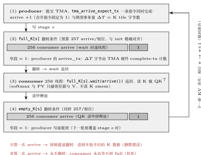
图 18.1: 固定 stage s 上 full/empty 两张屏障的相位循环（式 18.5 与式 18.6 的图形化）。每轮 KV 迭代：producer 提交 TMA 时用 tma_arrive_expect_tx 一条指令完成「arrive +1」与「声明 \Delta T 」两件事，TMA 硬件搬完后自动 complete-tx 计数；consumer 256 线程在 full_K[s].wait() 时各贡献一份 arrive（256 + 1 + tx 构成翻转条件），读毕 K 再各 arrive 一次释放 empty_K[s] ，producer 下一轮写前补上第 257 份。两边的 arrive 预算都是 257/轮，与 init 值精确对齐——多算一次挂死、少算一次静默错。窄段为可读放大，实际只占 1/257。
