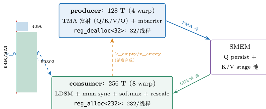
图 28.2: WS 双角色架构与 setmaxnreg 寄存器再分配。左：SM 寄存器池按式 (28.9) 重新切分，producer 只留 32/线程，consumer 分到 232/线程；中：producer 只发 TMA、consumer 只算；右：smem 是两者的交接面。实线箭头是数据流 (TMA 写入 \rightarrow LDSM 读出)，虚线箭头是 mbarrier 控制流 (full = 数据就绪、empty = 消费完成)，两者构成 §28.4.3 的握手协议。
