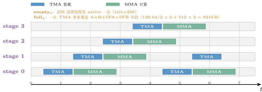
图 33.4: 四级流水的时序示意（ BN 取 128 的默认档；本卡 k_{Stages} 可用到 8~10 级，见 33.9.4 节扫描表）。与第三十一章图 31.2 的结构差别在 MMA 块的宽度：FP4 的一个 stage 只有一跳原子（ BK=64 ），K 方向不再有内层循环，MMA 块相对 TMA 块更窄——这意味着流水线对 TMA 延迟的容忍度更低，是 BN 翻倍的收益来源之一（ BN 翻倍 = MMA 块宽翻倍，而 TMA 字节数只增加 B 与 SFB 的部分）。
