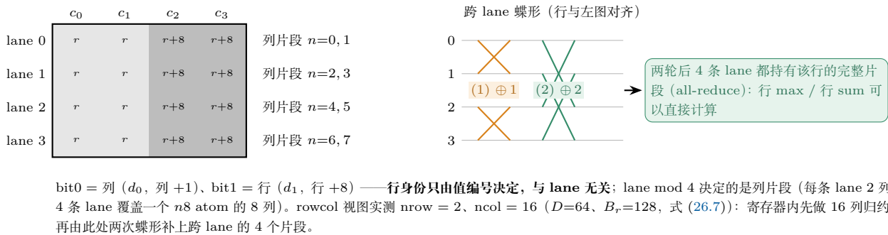
图 26.1: convert_layout_acc_rowcol 的两层拆解 (式 (26.6)–(26.7))。左: quad 内 4 条 lane 的 4 个寄存器 c_0..c_3 —— 两档灰度标出「行身份」: c_0, c_1 属行 r 、 c_2, c_3 属行 r+8 ; 右侧标出该 lane 覆盖的列片段 (由 \text{lane} \bmod 4 决定)。值编号的 bit0 是列偏移、bit1 是行 +8, 所以同一行的 8 列散落在 quad 的 4 条 lane 上。右: 两次 __shfl_xor_sync 的蝶形——第一轮并 (0,1) 与 (2,3) (步长 1), 第二轮并 (0,2) 与 (1,3) (步长 2), 两轮后每条 lane 都持有该行的完整片段, 行 max / 行 sum 可以就地计算。
