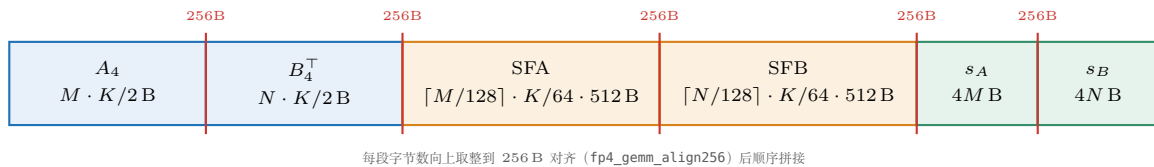
图 33.5: fp4_gemm_bf16 一次性 workspace 的六段布局 ( fp4_gemm.cuh 的 fp4_gemm_workspace_size )。 A_4 与 B_4^T 是量化产物 (4bit/元素); SFA/SFB 的行数按 128 向上取整——每个 512B 原子覆盖 128 行 \times 64 个 K 元素; s_A/s_B 是 level-1 的行/列 scale ( M/N 个 float)。每段字节数向上取整到 256B ( fp4_gemm_align256 ) 后顺序拼接。
