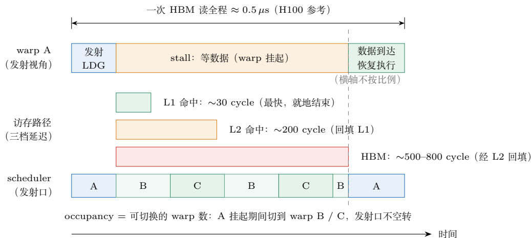
图 2.6: 一次访存的全程与延迟隐藏 (蓝 = 发射/执行, 橙 = 等待/过渡延迟, 绿 = 命中与恢复, 红 = 直达 HBM 的最长延迟)
