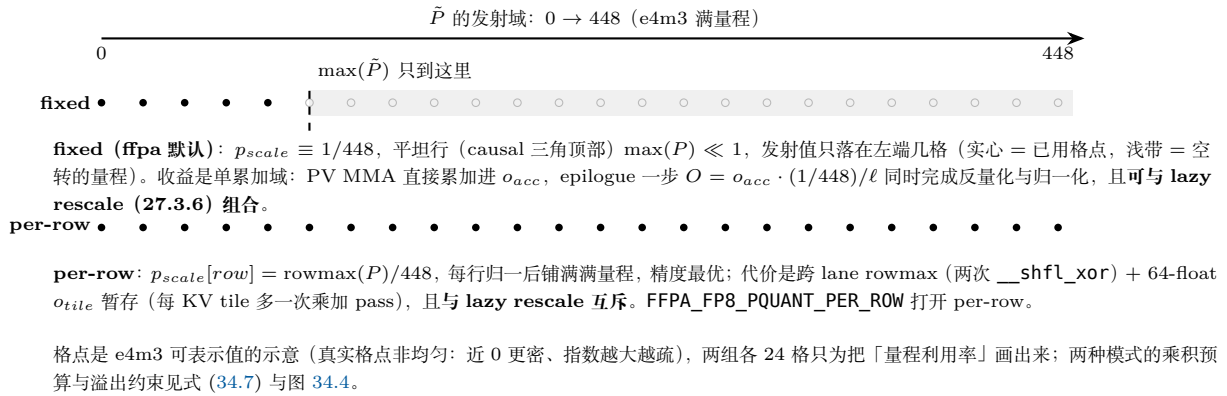
图 34.2: fixed 与 per-row 两种 p_{scale} 策略的发射域利用率 (27.3.5 节)。上: fixed 的 p_{scale} \equiv 1/448 是编译期常数, 平坦行的 \max(P) \ll 1 使发射值只占量程左端一小段, 其余量程空转——换来的是单累加域与「可与 lazy rescale 组合」; 下: per-row 用 \text{rowmax}(P)/448 使每一行铺满量程, 精度最优, 代价是跨 lane rowmax 归约与 64-float 的 o_{tile} 暂存, 且与 lazy rescale 互斥。
