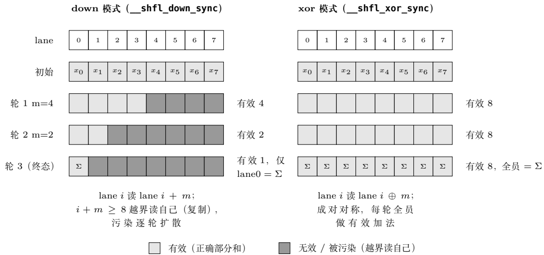
图 3.3: down 与 xor 两种 shuffle 逐轮对比 ( W=8 , 与图 3.2 同尺度, 灰 20 = 有效 / 灰 80 = 无效污染): down 模式 lane i 读 lane i + m , 越界者读自己 (复制), 有效 lane 数逐轮减半 ( 4 \rightarrow 2 \rightarrow 1 ), 终态仅 lane0 持正确全和; xor 模式成对对称、每轮全员有效, 终态 8 个 lane 全部持有 \Sigma (all-reduce) ——block 归约的广播步骤因此不再需要。
