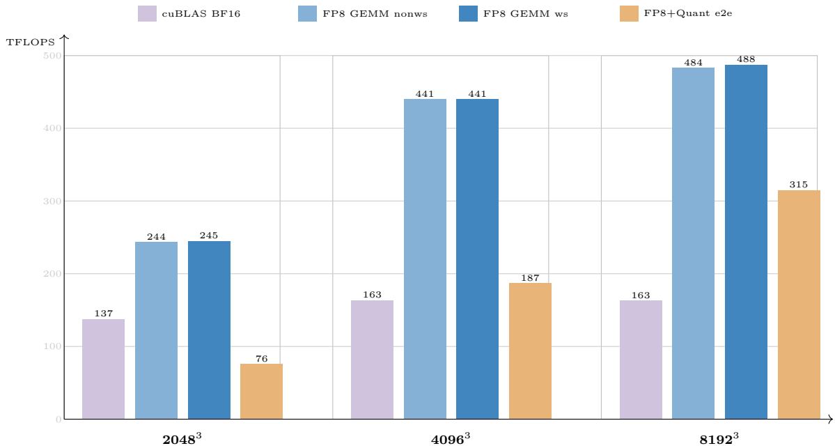
图 31.4: FP8 GEMM vs cuBLAS BF16 (PRO 5000, 越高越好; 默认档 128 \times 256/s2 )。三个规律: kernel-only 随 shape 增大从 1.77\times 升到 2.99\times ——宽 tile 需要足够多的 tile 填满 110 个 SM, 2048^3 的 128 \times 256 grid 只有 128 个 CTA (35.8.4 节末的波次量化); e2e 的形状敏感度更陡: 2048^3 反而低于 cuBLAS ( 0.55\times ), 因为量化是 O(MK+NK) 的带宽型工序, GEMM 变小时它的占比线性放大 (35.8.2 节); WS 全程略优于 non-WS (寄存器有余量, setmaxnreg 有让渡空间, 35.6 节), 但差距远小于 attention 大 D 场景。图中 e2e 柱是「全链路量化」的保守口径; 权重 B 离线量化后 e2e 回到 226/411/429 T (35.8.3 节)。
