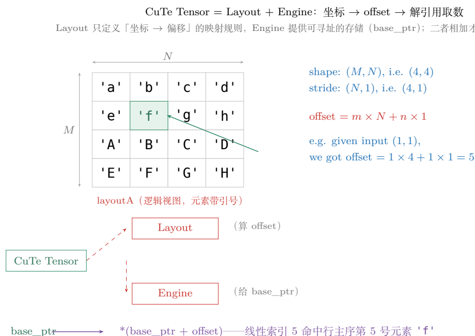
图 21.6: CuTe Tensor 的寻址分工: Layout 负责「坐标 \rightarrow offset」的代数——shape 限定输入范围、stride 决定各 mode 步长; Engine 只持有 base_ptr 。(1,1) \rightarrow 5, 命中行主序 ((4,4):(4,1), 列连续) 第 5 号元素 f。重建自 @ 竹熙佳处《写给大家看的 CuTe 教程: Layout Compose & Inverse》。
