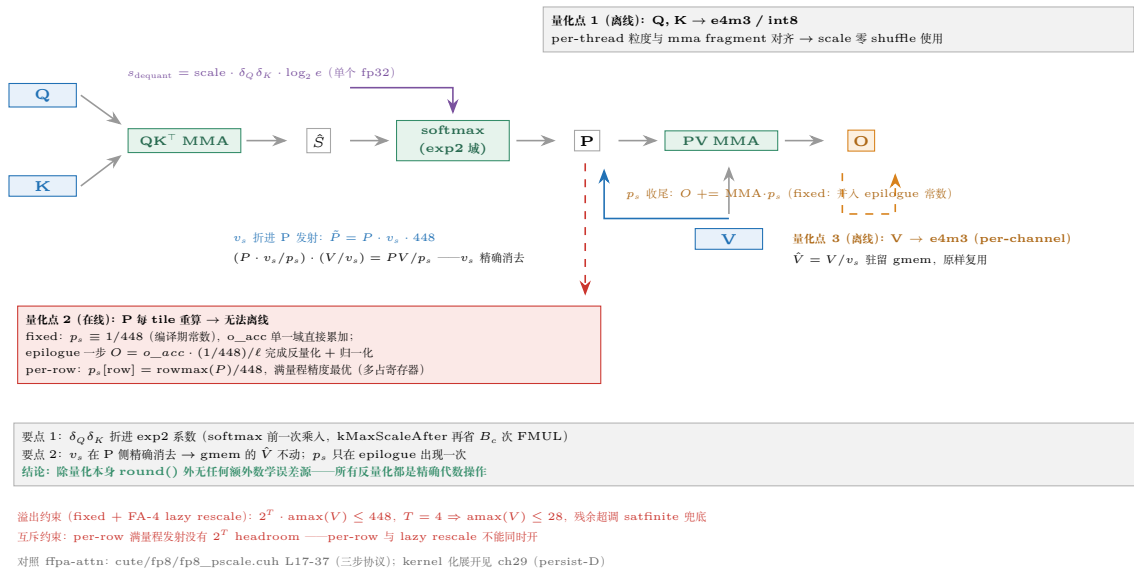
图 34.6: attention 的三个量化点与 scale 流向: \delta_Q \delta_K 折进 exp2 系数 (式 34.4)、 v_s 在 P 侧精确消去 (式 34.5)、 p_{\text{scale}} 在 epilogue 一步收尾。
