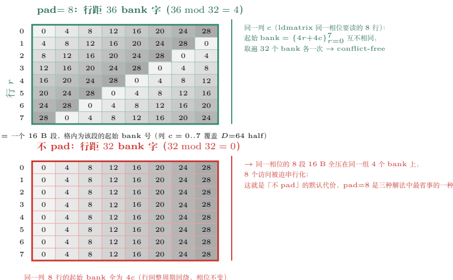
图 17.3: pad=8 与不 pad 的 ldmatrix bank 相位对照 (16.4.2 节 smem 三段布局中 pad 分析的图形化)。上: kSmemStride = D + \text{pad} = 72 half 时一行 144 B = 36 bank 字, 第 r 行相对第 0 行整体错开 36r \bmod 32 = 4r 个 bank; 任一行 c (ldmatrix 同一相位读的 8 行) 的起始 bank 为 \{4r+4c\} , 取遍 32 个 bank 各一次——8 段 16 B 恰好铺满全部 bank, conflict-free。下: 不 pad 时行距 128 B = 32 bank 字, 整周期回绕后 8 行起始 bank 全为 4c , 同一相位的 8 段 16 B 压在同一组 4 个 bank 上串行化。格内数字为「该 16 B 段的起始 bank 号」, 灰度按 bank 号每 4 个一档。
