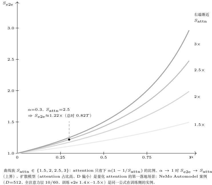
图 40.2：端到端摊销曲线族（式 40.3）：单算子 S_{\text{attn}} 换算到管线收益由 attention 占比 \alpha 决定上界。 \alpha=0.3 、 S_{\text{attn}}=2.5\times 时只剩 1.22\times ； \alpha \rightarrow 1 的渐近线即 S_{\text{attn}} 。
