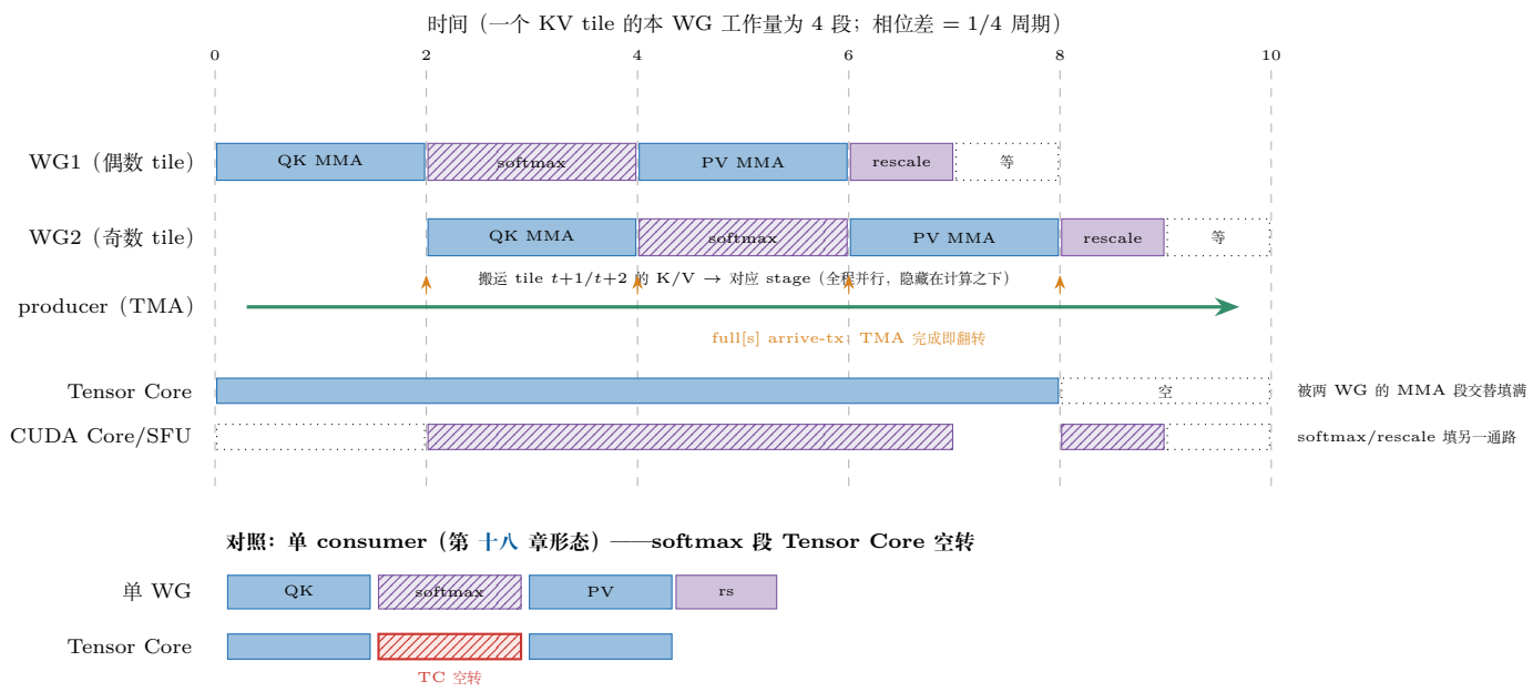
图 19.4: 双 consumer 的相位交错时序 (18.4.6 节统计性交错的图形化)。上: WG1/WG2 各按「QK MMA → softmax → PV MMA → rescale」四段推进自己的 KV tile 子序列, 两 WG 相位差 1/4 周期——WG1 处于 MMA 段时 WG2 大概率处于 softmax/rescale 段; producer 的 TMA 全程并行, 完成即 arrive-tx 翻转 full[s] 。中: Tensor Core 与 CUDA Core/SFU 两条资源条被两路计算交替填满 (同步 mma.sync 做不到 WG 内重叠, 靠两路独立流在硬件调度器上统计性交错)。下: 单 consumer (第 十八 章形态) 的对照——softmax 段 Tensor Core 只能空转, 这正是第二个 consumer 要填补的空档。
