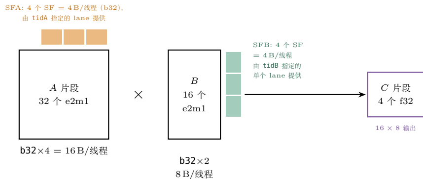
图 33.2: SM120_16x8x64_TN_VS 一条指令的操作数明细。数据侧共 16 + 8 = 24 B/线程, SF 侧 8 B/线程——SF 的字节数达到数据的 1/3。注意 SF 的「字节数/线程」与「SF 数/线程」是一回事 (ue4m3 是 1 字节), 但哪些 lane 的字节作数由指令的 tidA/tidB 选择器决定, 这就是 SF 的寄存器 fragment 必须由 CuTe 的 partition_fragment_sfa 从权威布局推导、而不能手写的原因。
