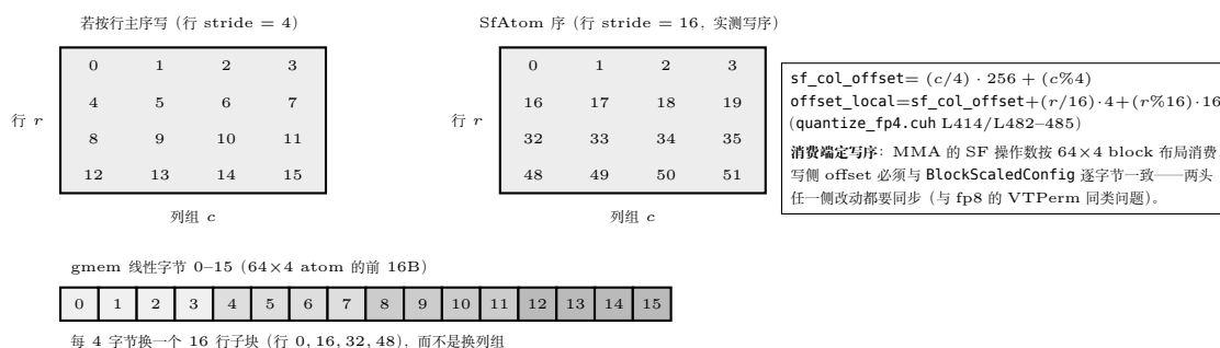
图 33.3: SF 字节的写序由消费端决定 ( V^T 量化链)。同一 (r, c) 单元格在行主序假设下偏移 4r + c , 在 SfAtom 序下偏移 16r + c : 每 4 个列组构成 64 \times 4 的 256B atom, atom 内按 16 行子块交错。写侧 (sf_col_offset/offset_local) 与 MMA 的 BlockScaledConfig 必须逐字节一致。
