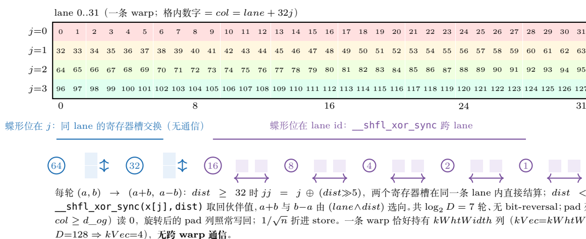
图 30.4: radix-2 蝶形的距离二分（ hadamard.cuh L40–92，本例 D=128 、 kWhtWidth=D ）。上：列归属—— j 是寄存器槽、lane 是 warp 内线程，格内数字 col = lane + 32j 满足索引律，右下角 127 = size - 1 ；一条 warp 覆盖整行 128 列。下：七轮的「距离阶梯」—— dist \geq 32 的 bit 落在 j 上（同 lane 两个寄存器槽直接加减，无通信）， dist < 32 的 bit 落在 lane id 上（ __shfl_xor_sync 跨 lane）；每轮一个 bit， 1/\sqrt{n} 折进 store。
