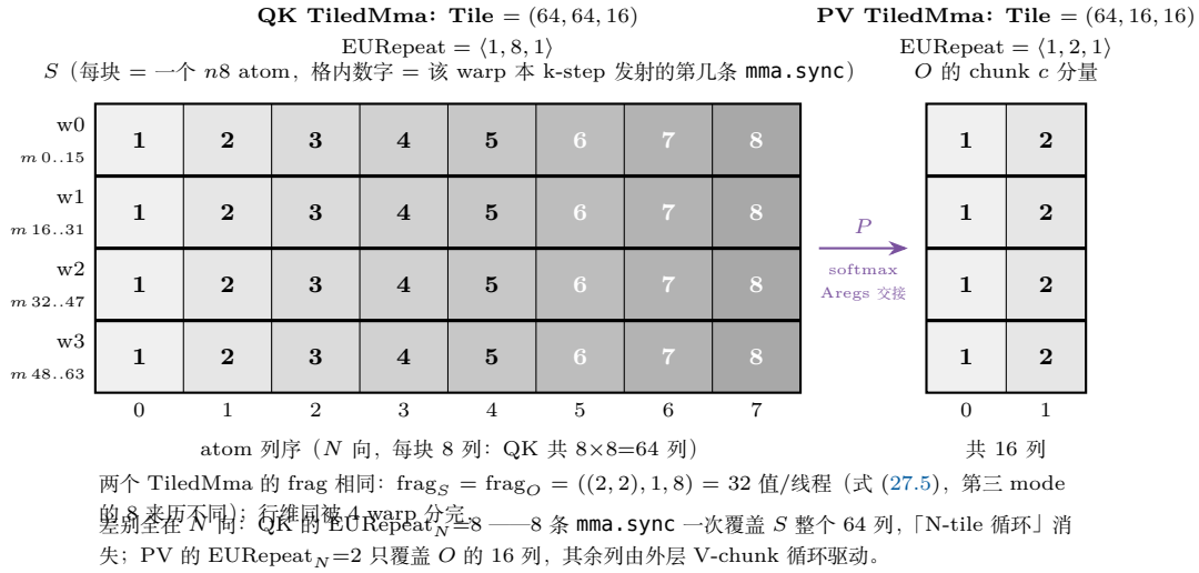
图 27.1: 双 TiledMma 的 Tile 分工 (ffpa_attn_.cu L52–58, 式 (27.2)–(27.3))。左: QK 的输出 S[64, 64] ——4 个 warp 各占 16 行 ( \text{AtomLayout} 的 M 分量 4), 列向 8 个 n8 atom 由同一线程在一个 k-step 里连发 8 条 mma.sync 覆盖 (灰度 8 档标识 atom 身份, 格内数字为发射序); 右: PV 的输出 O 只有一个 chunk 分量 [64, 16] (2 个 atom、2 条 mma.sync )。中间箭头是 26.3.3 节的交接: S 经 softmax 与 Aregs 零拷贝重解释成 P , 作为 PV 的 A 操作数——共享的正是左侧那批 S 寄存器。
