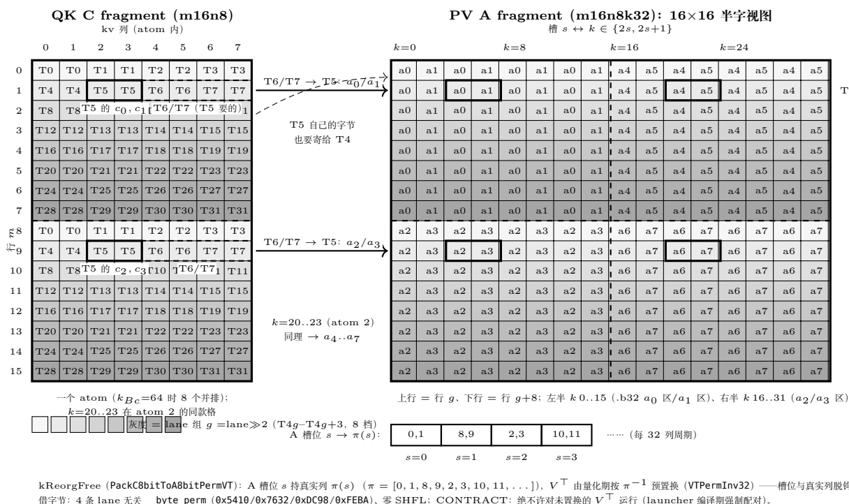
图 31.2: C→A fragment 的 lane→值映射 (lst:29-reorg-bg 的网格化)。左: QK C fragment (m16n8), 每 lane 4 值 c_0-c_3 落在行 g/g+8 的列对 \{2t, 2t+1\} ; 右: PV A fragment (m16n8k32) 的 16×16 半字视图, 格值 a_0-a_7 为 e4m3x2 半字寄存器, 四象限对应源码.b32 a_0-a_3 ; 两面板灰度同语义 (lane 组 g = \text{lane} \gg 2 , 8 档)。中: t=1 (T5) 的自然 A 需要 k \in \{4..7\} \cup \{20..23\} (行 g 与 g+8 ), 在 C 视图里属 T6/T7——纯 lane 内置换凑不齐, 即 16 SHFL + 32 PRMT (ReorgC8bitToA8bit) 的根源。下: kReorgFree 的出路——槽位持 \pi(s) 、 V^T 预置换, 4 条 lane 无关 __byte_perm、零 SHFL。
