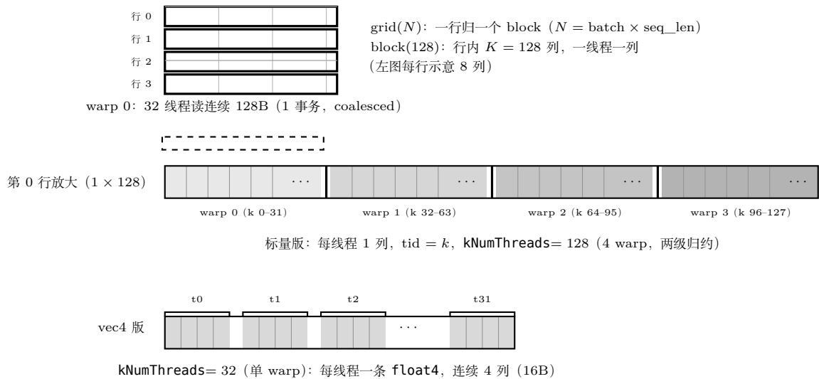
图 7.2: one-row-one-block 行划分: 上, N \times K 矩阵每行归一个 block ( grid( N ) ); 中, 单行放大为 1 \times 128 条带, 4 个 warp 各占 32 列 (各一档灰度), warp 0 的 32 线程读连续 128B, 单事务合并; 下, vec4 版改为 32 线程、每线程一条 float4 (连续 4 列), 指令数降为 1/4。
