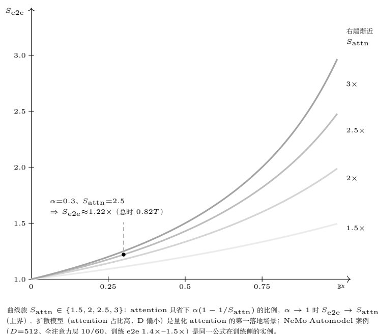
图 35.2: 端到端摊销曲线族 (式 35.3): 单算子 S_{\text{attn}} 换算到管线收益由 attention 占比 \alpha 封顶。 \alpha=0.3 、 S_{\text{attn}}=2.5\times 时只剩 1.22x; \alpha \rightarrow 1 的渐近线即 S_{\text{attn}} 。
