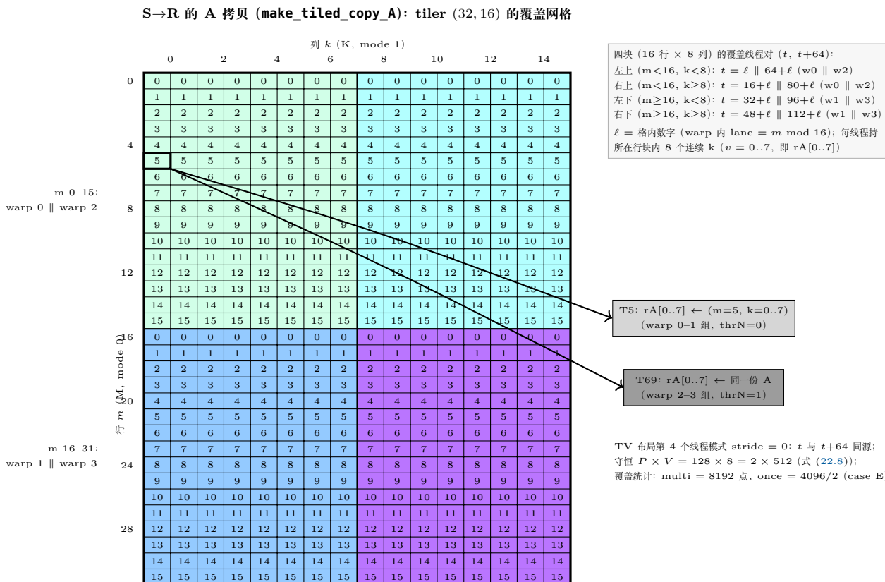
图 22.3: S→R A 拷贝的 2 倍重复因子 (式 (22.9)、测试 case D/E): tiler (32, 16) 的 A tile ( M \times K ) 上, 每格标 warp 内 lane 号 \ell = m \bmod 16 , 格子的实际覆盖线对为 (基址 +\ell , 基址 +64+\ell ), 四块的基址见右上表 (w0-w3 即 warp 0-3)。每个元素恰被 2 个 (thread, value) 对覆盖: t 与 t+64 (两个 N 方向 warp, thrN = 0/1) 各持同一行块 8 个连续 k 的一份寄存器拷贝——TV 布局第 4 个线程模式 stride 为 0 的几何含义, 守恒 128 \times 8 = 2 \times 512 。对照图 22.5 的 G→S 双射网格 (每格恰一线程)。
