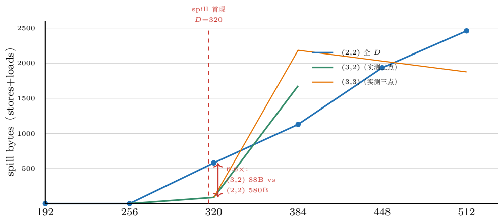
图 29.5: 寄存器溢出随 D 的增长 (nvcc -Xptxas -v, -O2, sm_120a, 各组合显式实例化)。 D \leq 256 全组合零 spill; D=320 (红色虚线) 是分水岭——所有组合达到 255 寄存器上限并开始溢出, 且 (3,2)/(3,3) 的 88B 与 (2,2) 的 580B 相差 6.6 倍, 与 TFLOPS 排序 (204.1 对 188.3) 完全同序; D \geq 384 后 spill 基线过千, stages 加深进一步推高溢出 ((3,2) 1676B、(3,3) 2184B, 均高于 (2,2)), 流水掩蔽收益被抵消, 最优组合回落 (2,2)。
