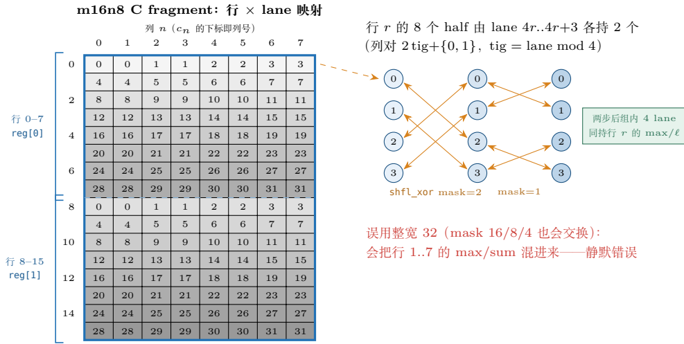
图 17.2: m16n8 C fragment 的行 × lane 映射与 \text{warp\_reduce}<4> 的宽度依据。左: 行 r 与 r+8 的 8 个列元素同由 lane 4r..4r+3 持有 ( \text{tig} = 0..3 各一对), 行 0-7 走 \text{reg}[0] 、行 8-15 走 \text{reg}[1] ; 右: 组内两步 XOR 蝶形 ( \text{mask } 2 \rightarrow \text{mask } 1 ) 后 4 个 lane 同持该行归约值。若误用整宽 32, \text{mask } 16/8/4 的交换会把别的行的值混进来——这是 3c 步最典型的静默错误。
