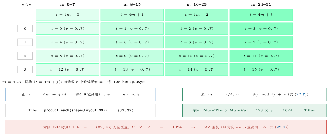
图 22.5: thread×value 网格: G \rightarrow S 拷贝把 32 \times 32 的 tile 划成 t = 4m + j 的网格, 每个线程搬 8 个连续元素 (一条 128-bit cp.async )。同一划分用 MN 语言或 TV 语言描述是等价的 (式 (22.6) 与式 (22.7))。
