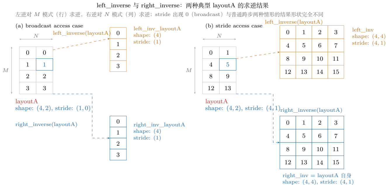
图 21.9: left_inverse / right_inverse 的两种情形 (CuTe v4.6.1 实测): stride (1, 0) 广播布局两逆相同, 均为去重投影 (4):(1)——stride 为 0 的维度被投影掉, 每行只保留代表坐标 m; stride (4, 1) 的双射布局两逆均为其自身 (4, 4):(4, 1) (该布局是对合, f \circ f = \text{id} )。重建自 @ 竹熙佳处《写给大家看的 CuTe 教程: Layout Compose & Inverse》(数值按 CuTe v4.6.1 实测校正)。
