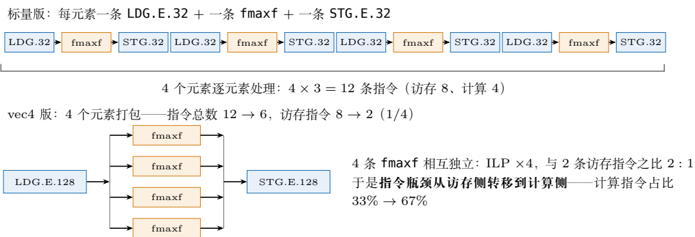
图 4.3: 标量与 vec4 的指令流对照(relu, 以 4 个元素为例): 标量版每元素 3 条指令 ( LDG.E.32 \rightarrow fmaxf \rightarrow STG.E.32 ), 4 元素共 12 条、其中访存 8 条; vec4 版用一条 LDG.E.128 取回 4 个元素, 4 条 fmaxf 互不依赖 ( ILP \times 4 ) 后由一条 STG.E.128 写回, 总数降到 6 条、访存只剩 2 条。访存: 计算从 8:4 变为 2:4, 指令瓶颈因此从访存侧移到计算侧。
