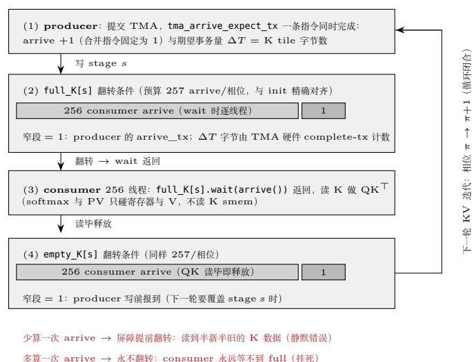
图 18.1: 固定 stage s 上 full/empty 两张屏障的相位收支循环（式 18.5 与式 18.6 的图形化）。每轮 KV 迭代：producer 提交 TMA 时用 tma_arrive_expect_tx 一条指令完成「arrive +1」与「声明 \Delta T 」两件事，TMA 硬件搬完后自动 complete-tx 计数；consumer 256 线程在 full_K[s].wait() 时各贡献一份 arrive（256 + 1 + tx 构成翻转条件），读毕 K 再各 arrive 一次释放 empty_K[s] ，producer 下一轮写前补上第 257 份。两边的 arrive 预算都是 257/轮，与 init 值精确对齐——多算一次挂死、少算一次静默错。窄段为可读放大，实际只占 1/257。
