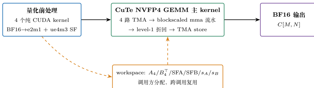
图 33.1: fp4_gemm_bf16 全链路。与第三十一章(图 31.1)同构,唯一的结构差异是 workspace 里多出两份 SF: A 侧的 SFA 是 \lceil M/128 \rceil \cdot (K/64) 个 512B 原子, B 侧的 SFB 同理。SF 不是「辅助数据」,它是 MMA 指令的操作数——主 kernel 必须为它单独开一条 TMA 通道、一块 smem、一个寄存器 fragment (33.4 与 33.5 节)。
