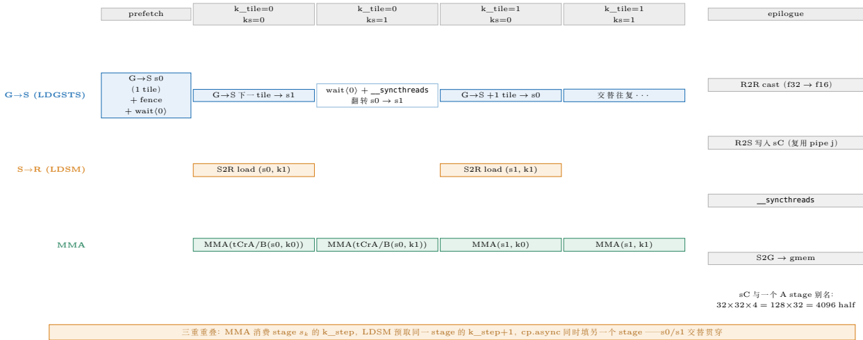
图 25.4: CuTe HGEMM 的 k_{\text{stage}} = 2 流水时序（含寄存器双缓冲）。上：G→S (LDGSTS)；中：S→R (LDSM)；下：MMA。MMA 消费 stage s_k 的 k_{\text{step}} 时，LDSM 预取同一 stage 的 k_{\text{step}}+1 ， cp.async 同时填另一个 stage——三重重叠；左端 prefetch 一个 tile，右端 epilogue ( R2R \rightarrow R2S \rightarrow S2G , sC 与一个 A stage 别名: 32 \times 32 \times 4 = 128 \times 32 = 4096 half)。
