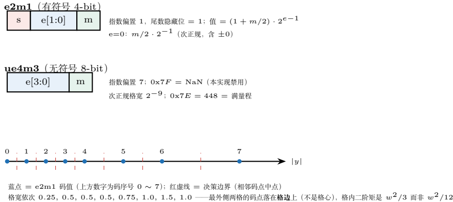
图 32.2: NVFP4 的两个 4-bit 类型。上: e2m1 位域与数轴 (格宽随量级翻倍, 最外侧两格「码点在格边」是误差模型里最大的一项贡献, 见 32.5 节); 下: ue4m3 位域 (scale 专用, 量程 [2^{-9}, 448] , 0 \times 7F 是 NaN)。
