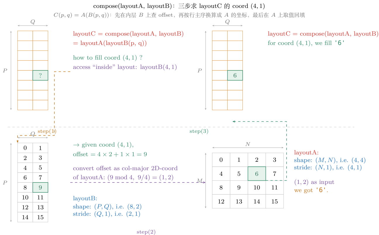
图 21.7: \text{compose}(A, B) 的三步求值: 先查内层 B 得 \text{offset} , 再按外层 A 的 \text{shape} 把 \text{offset} 换算回坐标, 最后查 A 得最终值。例: C(4, 1) \rightarrow B(4, 1) = 9 \rightarrow (9 \bmod 4, 9 \div 4) = (1, 2) \rightarrow A(1, 2) = 6 回填 C 。重建自同上文。
