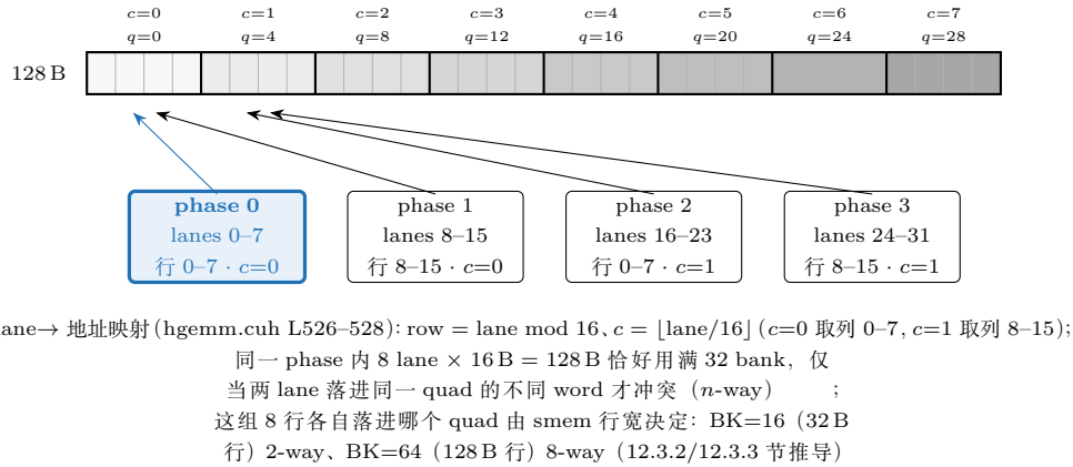
图 13.1: bank/phase 硬件模型 (12.3.1 节): 32 bank \times 4 B 一拍最多交付 128 B, 任一连续 128 B 地址窗切成 8 个 16 B chunk, chunk c 占一个 quad (起始 bank q = 4 \lfloor a/16 \rfloor \bmod 32 , 同 quad 同灰度)。warp 的 32 lane 按 phase 分 4 组依次服务, ldmatrix.x4 的 4 个 8 \times 8 矩阵正对应 4 个 phase: phase p 由 lanes 8p \dots 8p+7 按 \text{row} = \text{lane} \bmod 16, c = \lfloor \text{lane}/16 \rfloor 提供地址 (高亮 phase 0 = lanes 0-7 读行 0-7 的 chunk 0; phase 0/1 同读 chunk 0, phase 2/3 同读 chunk 1)。phase 内是否冲突取决于该组 8 行落进的 quad 分布——12.3.2/12.3.3 节按行宽推导 2-way/8-way、以及图 13.2 的三档 swizzle 对比, 都建立在这个机制底座上。
