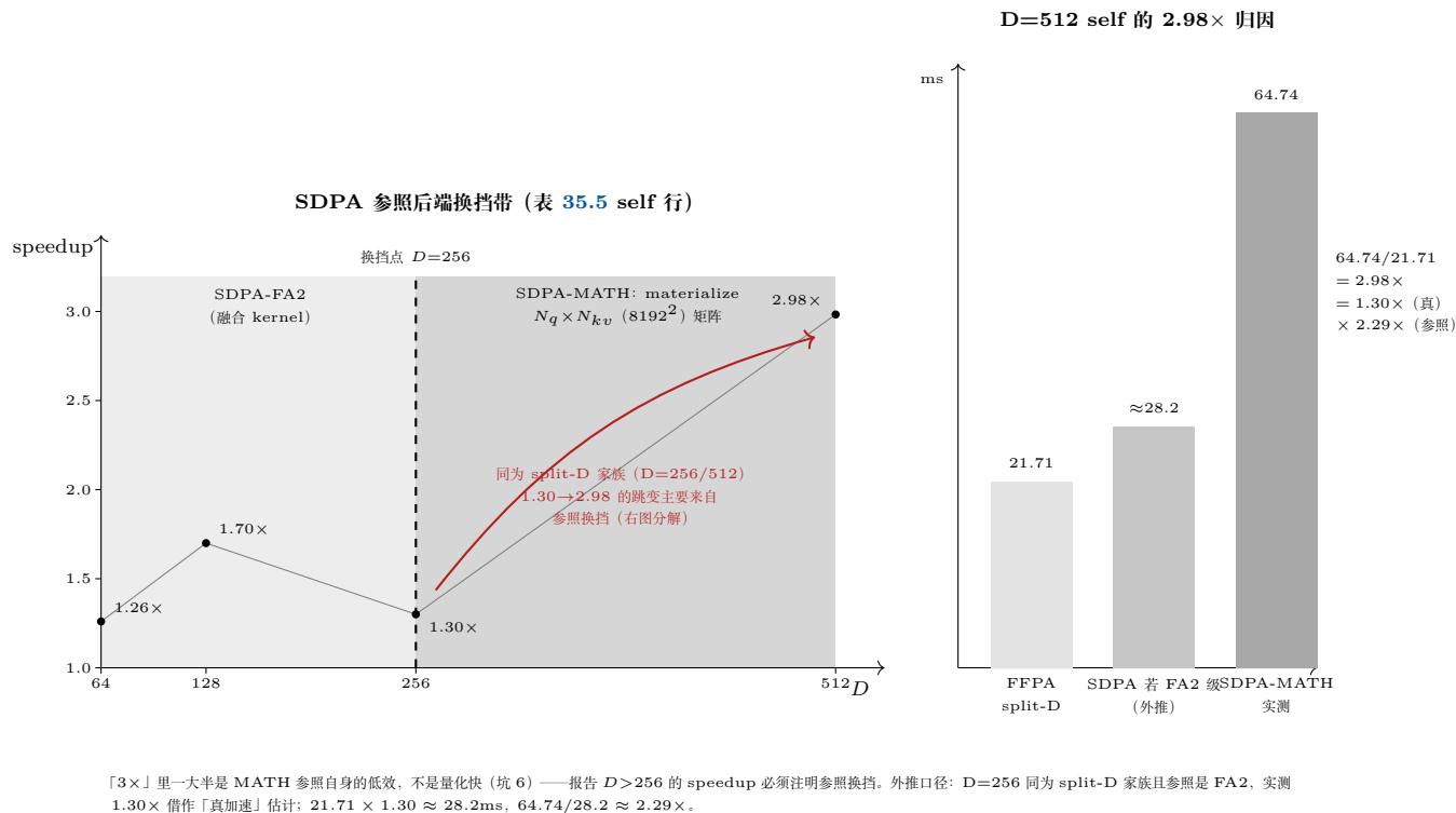
图 35.1: 参照系视角看表 35.5 的 self 行。左: SDPA 参照随 D 换挡——FA2 只覆盖 D \leq 256 , 更大 D 静默落到 MATH (materialize N_q \times N_{kv} 矩阵); 四个 speedup 点 (1.26/1.70/1.30/2.98 \times ) 落在换挡带上, D=512 的跳变与 kernel 无关。右: D=512 的 2.98 \times 归因——以 D=256 同家族 (split- D 、FA2 参照) 实测 1.30 \times 为真加速估计, MATH 参照自身再慢 \times 2.29 : 「3 \times 」的大头是参照低效 (坑 6)。
