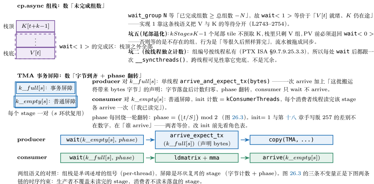
图 26.4: 两种异步等待语义的时间线对照 (flash_attn.cuh 与 ffpa_attn.cuh 的 TMA 版)。上：cp.async 组栈——提交顺序 V[t] (栈底) \rightarrow K[t+k-1] (栈顶)， wait < 1 > 停在「除栈顶 K 之外全部完成」，尾部 kStagesK-1 个 tile 必须退回 wait < 0 > (坑五)；每处 wait 后跟一次 __syncthreads() (坑二：组计数按线程私有)。中下：TMA 的事务计数——每个 stage 一对 k\_full[s] (事务屏障，producer 单线程 arrive_and_expect_tx ) 与 k\_empty[s] (普通屏障，init = kConsumerThreads )，phase 由 [t/S] \bmod 2 现算；最下一行是两条流水链的时序。
