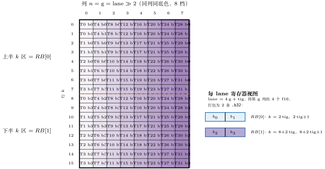
图 12.2: B fragment ( k16 \times n8 ) 寄存器布局, 式 12.2 的网格化 (图 12.1 的 B 侧对照图): 列 n = g = \text{lane} \gg 2 (同列同底色 8 档), 行 k 按 b_0 \rightarrow 2 \text{tig} , b_1 \rightarrow 2 \text{tig}+1 , b_2/b_3 再 +8 分布。右: 每 lane 4 个 f16 打包为 RB[0]/RB[1] 两条 .b32。与 A 对照: A 按行分、B 按列分。
