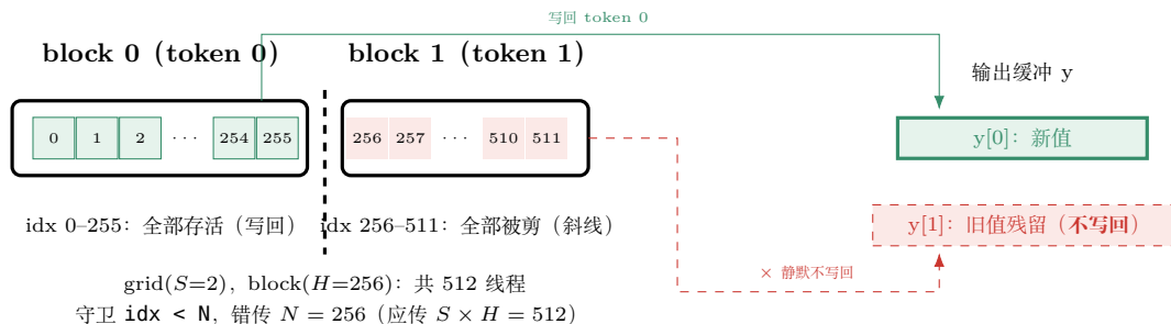
图 5.4：坑一「 N 传错语义」的静默丢输出：grid( S=2 )、block( H=256 ) 时正确应传 N = S \times H = 512 ；若按「每 token 长度」错传 N = 256 ， \text{idx} < N 守卫线落在 block 0/block 1 边界上，block 1 的全部线程（idx 256–511，斜线格）被剪掉，token 1 的输出缓冲残留旧值——不报错、不崩溃（见 4.6 节勘误一）。
