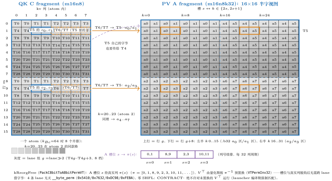
图 36.2: C→A fragment 的 lane→值映射。左: QK C fragment (m16n8), 每 lane 4 值 c_0-c_3 落在行 g/g+8 的列对 \{2t, 2t+1\} ; 右: PV A fragment (m16n8k32) 的 16x16 半字视图, 格值 a_0-a_7 为 e4m3x2 半字寄存器, 四象限对应源码.b32 a_0-a_3 ; 两面板灰度同语义 (lane 组 g = \text{lane} \gg 2 , 8 档)。中: t=1 (T5) 的自然 A 需要 k \in \{4..7\} \cup \{20..23\} (行 g 与 g+8 ), 在 C 视图里属 T6/T7——纯 lane 内置换无法拼出, 即 16 SHFL + 32 PRMT (ReorgC8bitToA8bit) 的根源。下: kReorgFree 的出路——槽位持 \pi(s) 、 V^\top 预置换, 4 条 lane 无关 __byte_perm、零 SHFL。
