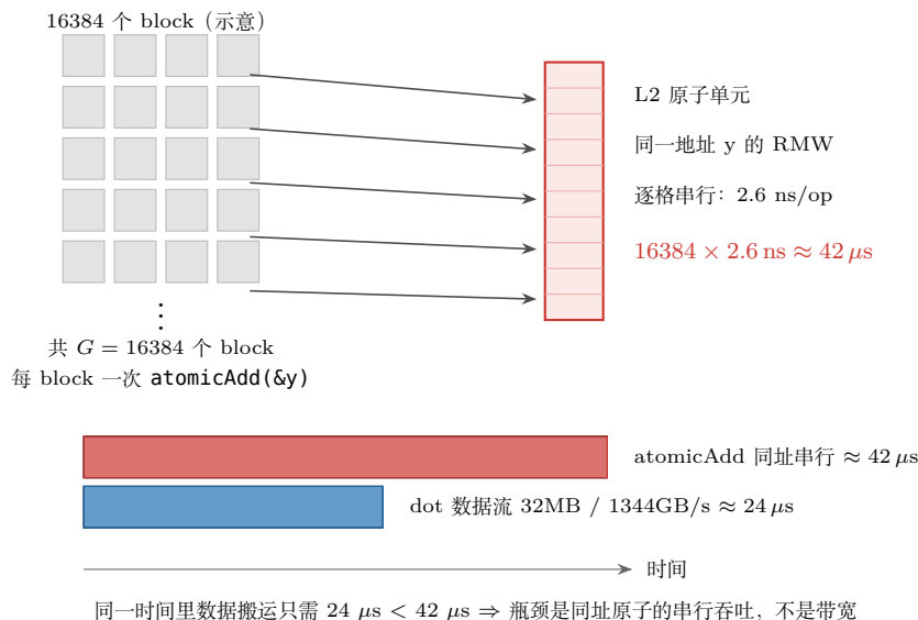
图 3.5: 全局原子串行化的量化证据: G = 16384 个 block 的 atomicAdd 全部汇入同一地址 y 的 L2 原子单元窄队列逐格串行 (2.6 ns/op, 共约 42 \mu\text{s} ), 长于 dot 本身的数据流时间 (约 24 \mu\text{s} )。
