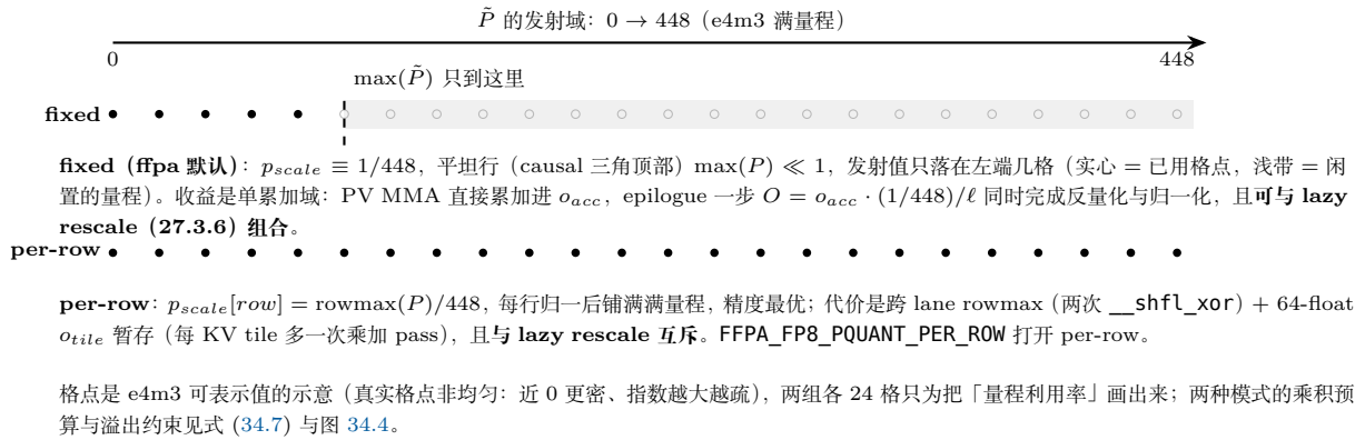
图 34.2: fixed 与 per-row 两种 p_{scale} 策略的发射域利用率 (27.3.5 节)。上: fixed 的 p_{scale} \equiv 1/448 是编译期常数, 平坦行的 \max(P) \ll 1 使发射值只占量程左端一小段, 其余量程闲置——换来的是单累加域与「可与 lazy rescale 组合」; 下: per-row 用 \text{rowmax}(P)/448 使每一行铺满量程, 精度最优, 代价是跨 lane rowmax 归约与 64-float 的 o_{tile} 暂存, 且与 lazy rescale 互斥。
