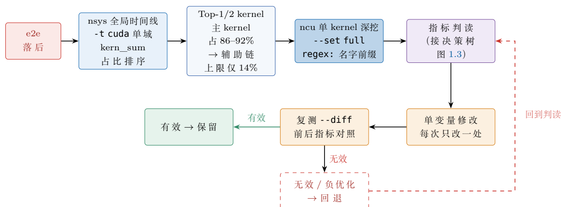
图 1.1: nsys → ncu → 单变量修改 → 复测 --diff 的闭环工作流：nsys 先给全局占比与优化预算（主 kernel 占 86–92%，辅助链上限仅 14%，对应 §1.8 例一）；ncu 只深挖 Top-1/2 kernel；每次只改一处，复测后无效立即回退、回到指标判读。配色：红 = 问题起点，蓝 = 采集/分析链，紫 = 判读决策点，橙 = 修改/复测动作，绿 = 有效保留，红虚线 = 无效回退。
