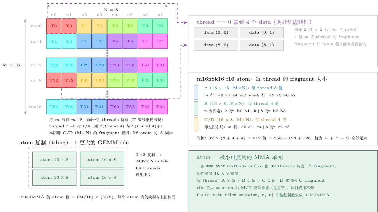
图 23.4: m16n8k16 atom 的 C fragment thread-value 映射: thread t 持行 t/4 与 t/4+8 、列 2(t \bmod 4) 与 2(t \bmod 4)+1 共 4 值——行 m 与 m+8 由同组线程重复持有。三个操作数每线程 A 8 值 / B 4 值 / C 4 值, 守恒式 32 \times (8+4+4) = 512 。更大的 tile 只是 atom 沿 M/N 的复制堆叠, thread-value 规律不变—— make_tiled_mma 的构造基础。重建自 @ 竹熙佳处《写给大家看的 CuTe 教程: tiled mma》。
