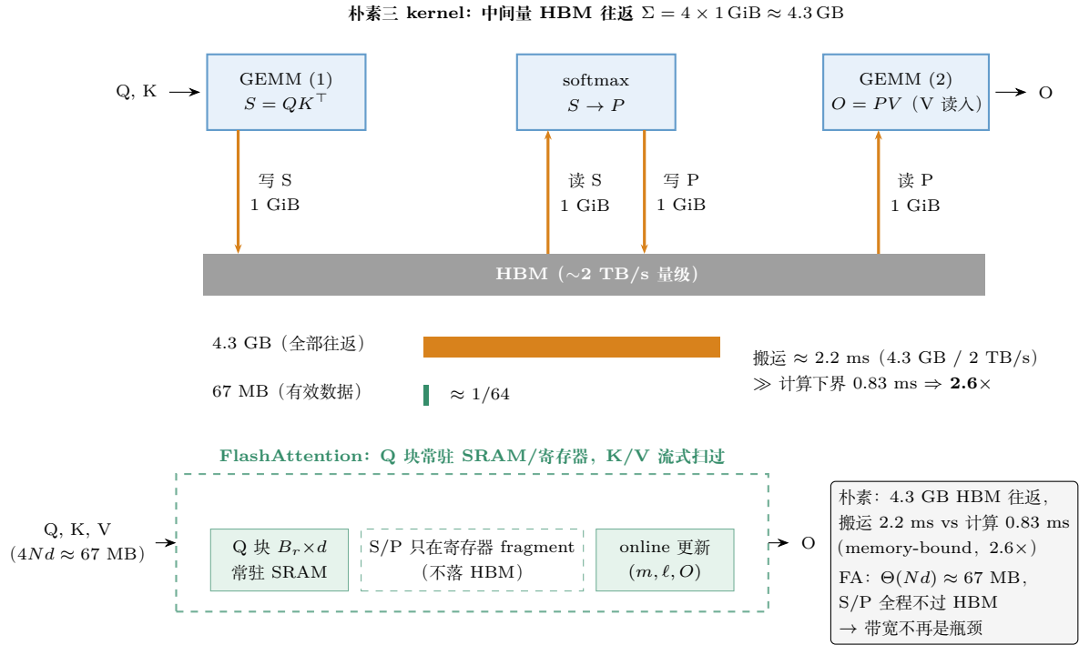
图 16.2: 朴素 attention 与 FlashAttention 的 HBM 往返流量对比 (15.3.3 节, B=1, H=32, N=4096, d=64 ): 上行三个 kernel 之间, S 与 P (各 \approx 1 \text{ GiB} ) 必须经 HBM 往返——写 S 、读 S 、写 P 、读 P 共 4 \times 1 \text{ GiB} \approx 4.3 \text{ GB} , 而有效数据 ( Q, K, V 读入 + O 写出) 只有 \approx 67 \text{ MB} , 占全部流量的 1/64 ; 按 2 \text{ TB/s} 乐观带宽, 仅搬运就要 \approx 2.2 \text{ ms} , 已是 0.83 \text{ ms} 计算下界的 2.6 倍——kernel 落在 memory-bound 区。下行 FlashAttention 把 S, P 限制在 SRAM/寄存器 fragment 里 (虚线框), HBM 只传输 Q, K, V 输入与 O 输出 ( \Theta(Nd) , 式 16.9 的另一端), 中间量全程不过 HBM。
