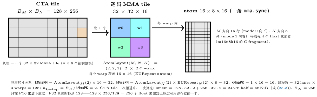
图 25.1: 本章实际配置的三层 tile 金字塔 (式 (25.2) 与式 (25.4)): 外层 CTA tile 128 \times 256 一次搬进 smem、一次算完 (F16 累加; F32 累加时 B_N 降到 128); 中层逻辑 MMA tile 32 \times 32 \times 16 被 \text{AtomLayout}(2, 2, 1) 切成 2 \times 2 个 warp (每个 warp 覆盖 16 \times 16 , 由 \text{EURepeat} \times \text{atom} 堆出); 内层 atom 16 \times 8 \times 16 就是一条 mma.sync 。CuTe 的层层 partition 都是这座金字塔上的「塔尖到塔基」坐标换算。
