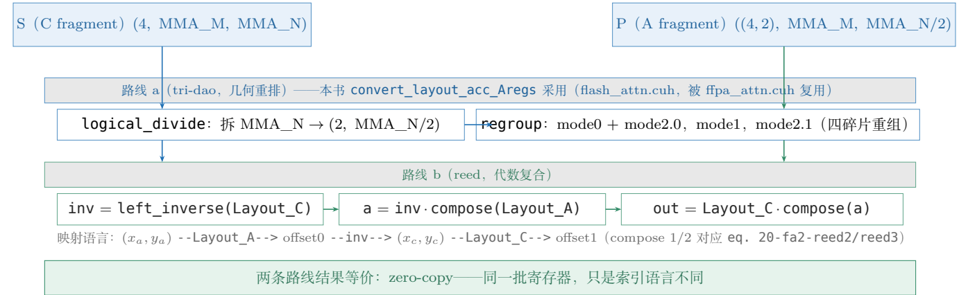
图 21.5: FA2 的 P 矩阵布局转换: tri-dao 的几何重排与 reed 的代数复合两条路线, 结果等价。本书 flash_attn.cuh 的 convert_layout_acc_Aregs (被 fpa_attn.cuh 复用) 采用的是几何路线。
