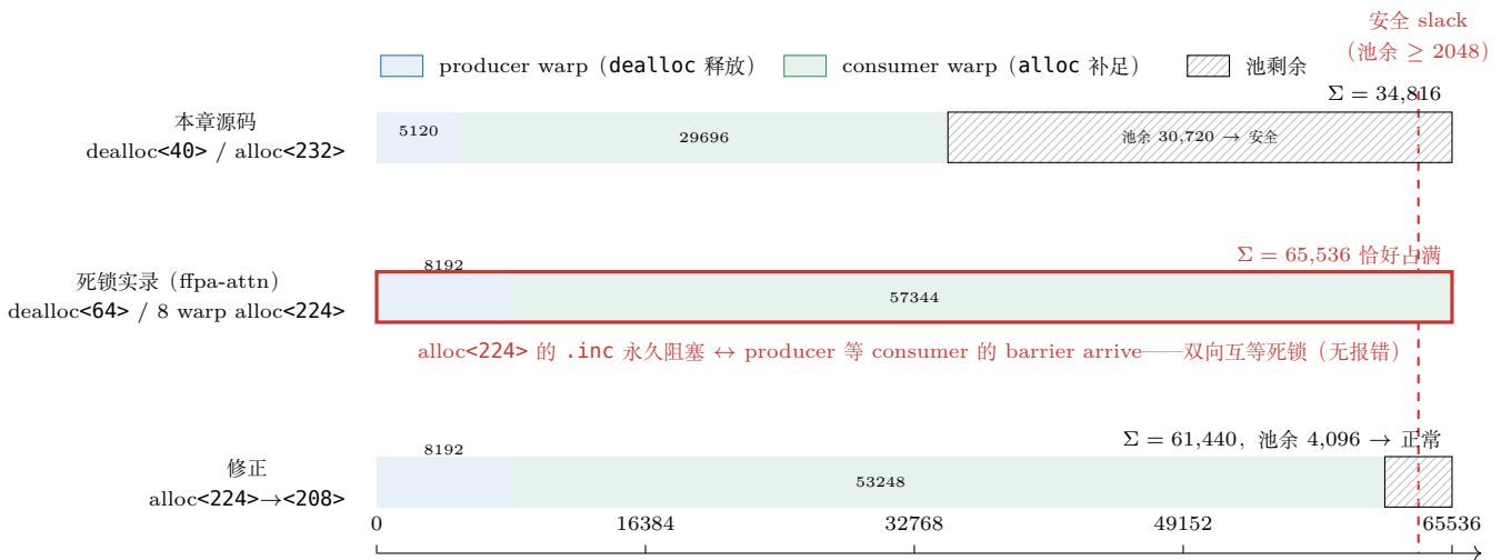
图 15.1: setmaxnreg 的 CTA 寄存器池三配置对照 (式 15.4, 每 SM 寄存器文件共 65,536 个 32-bit 寄存器): 条形按 \sum_w 32r_w 堆叠 producer ( dealloc 释放) 与 consumer ( alloc 补足) 两段, 红色虚线为工程安全界 (池余 \geq 2048 )。① 本章源码 dealloc<40>/alloc<232> : 5120 + 29696 = 34816 , 池余 30720, 安全; ② ffpa-attn 调优实录的死锁配置 dealloc<64> + 8 warp \times alloc<224> : 8192 + 57344 = 65536 恰好占满——有效池 < 65536 , .inc 永远凑不齐而阻塞在 setmaxnreg 上, 与 producer 等 barrier arrive 形成双向互等死锁; ③ alloc 降到 208: 总 61440、池余 4096, 恢复正常。
