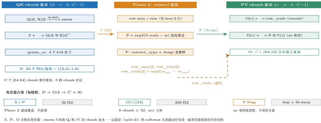
图 27.5: 双 TiledMma 的数据流: QK 沿 D 累加成 S (32 寄存器跨 chunk 存活), softmax 就地覆盖为 P , Aregs 重解释后交给 PV; O 的每个 chunk 分量独立 rescale 与累加, row_scale (虚线) 耦合两个循环。底部为寄存器占用: S/P 32、 O[C][32] 共 256 ( C=8 )、 V fragment 按 M-warp 重复——smem 只承载 Q/K/V 的 chunk 流水。
