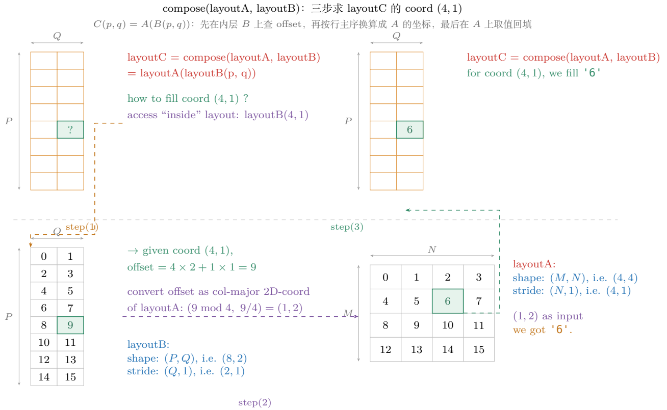
图 21.7: compose(A, B) 的三步求值: 先查内层 B 得 offset, 再按外层 A 的 shape 把 offset 换算回坐标, 最后查 A 得最终值。例: C(4, 1) \rightarrow B(4, 1) = 9 \rightarrow (9 \bmod 4, 9 \div 4) = (1, 2) \rightarrow A(1, 2) = 6 回填 C 。重建自同上文。
