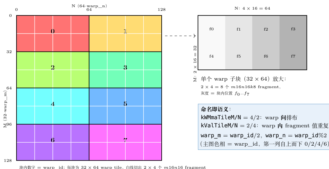
图 11.2: 128 \times 128 block tile 的三层分解: 外层按 4 \times 2 切 8 个 32 \times 64 warp 子块 (色相 = warp_id, B_M = 16 \times 4 \times 2 , B_N = 16 \times 2 \times 4 ); 每子块内再摆 2 \times 4 = 8 个 m16n16k8 fragment (右: 放大图, 灰度 = 块内位置)。侧栏: kWMmaTileM/N 表 warp 间排布、 kValTileM/N 表 warp 内 fragment 值重复, 名字即语义。
