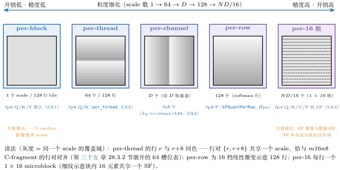
图 34.1: 量化粒度谱系五联网络 (表 34.2 的可视化, 缩略网格为 16 行 \times 16 列)。从左到右: per-block 整块共享 1 个 scale; per-thread 按 C-fragment 行对 \{r, r+8\} 分档 (128 行块共 8 \times 8 = 64 个, 零 shuffle 消费); per-channel 沿 D 每通道一个; per-row 每 softmax 行一个 (128 个); per-16 每行一个 1 \times 16 microblock (NVFP4 的 SF)。顶部双向轴是整条谱系的 trade-off: 粒度越细精度越高, 但 scale 的存储、传递与消去开销同步上涨, 且必须与 MMA 的 fragment 布局对齐——谱系两端的失败模式分别是对 outlier 的脆弱性与 SF 自身的访存账。
