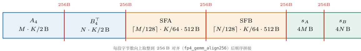
图 33.5: fp4_gemm_bf16 一次性 workspace 的六段布局 ( fp4_gemm.cuh 的 fp4_gemm_workspace_size )。 A_4 与 B_4^T 是量化产物 (4bit/元素); SFA/SFB 的行数按 128 向上取整——每个 512B 原子覆盖 128 行 × 64 个 K 元素; s_A/s_B 是 level-1 的行/列 scale ( M/N 个 float)。每段字节数向上取整到 256B ( fp4_gemm_align256 ) 后顺序拼接。
