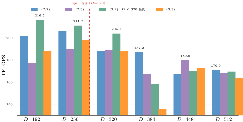
图 29.4: K/V 流水深度解耦实验 ( B=1/H=32/N=8192 , PRO 5000, 成对同轮)。 D \leq 320 : (S_K, S_V)=(3,2) 一致最优, 绿色系柱全面领先; D \geq 384 : 最优回落到 (2,2)/(2,3), (3,3) 在 D=384 崩至 136.0 (比 (2,2) 低 27%)。红色虚线是分界: 恰在寄存器 spill 首次出现处 (表 见下, D=320 全组合 spill、 D \leq 256 零 spill)。
