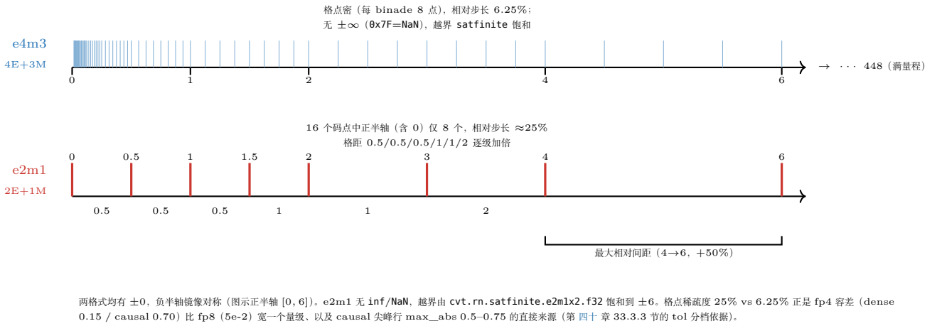
图 38.1: e2m1 vs e4m3 的格点数轴 (同一 [0, 6] 区间)。上: e4m3 每个 binade 8 个格点、相对步长 6.25%，满量程 \pm 448 ；下: e2m1 正半轴全部格点仅 \{0, 0.5, 1, 1.5, 2, 3, 4, 6\} 、相对步长约 25%，[4, 6] 段相对间距最大 (+50%)。fp4 的容差天然比 fp8 宽一个量级的格式层根源。
