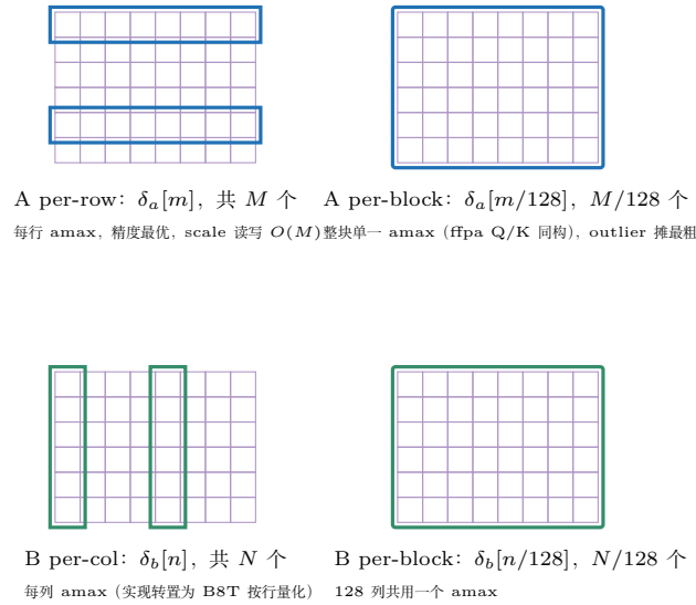
图 30.2: 四种 scale 粒度组合（上排 A，下排 B）。蓝框 = A 侧 scale 统计范围，绿框 = B 侧。粒度越粗，scale 存储/查表越省（per \times per-block 每 tile 只查两个标量），但 outlier 的「毒性」越大——一个大值会把整块的步长撑爆，其余小值全部挤进低位。四种组合在 API 里是一个枚举，主 kernel 用 if constexpr 编译期剔除，运行时零分支开销。
