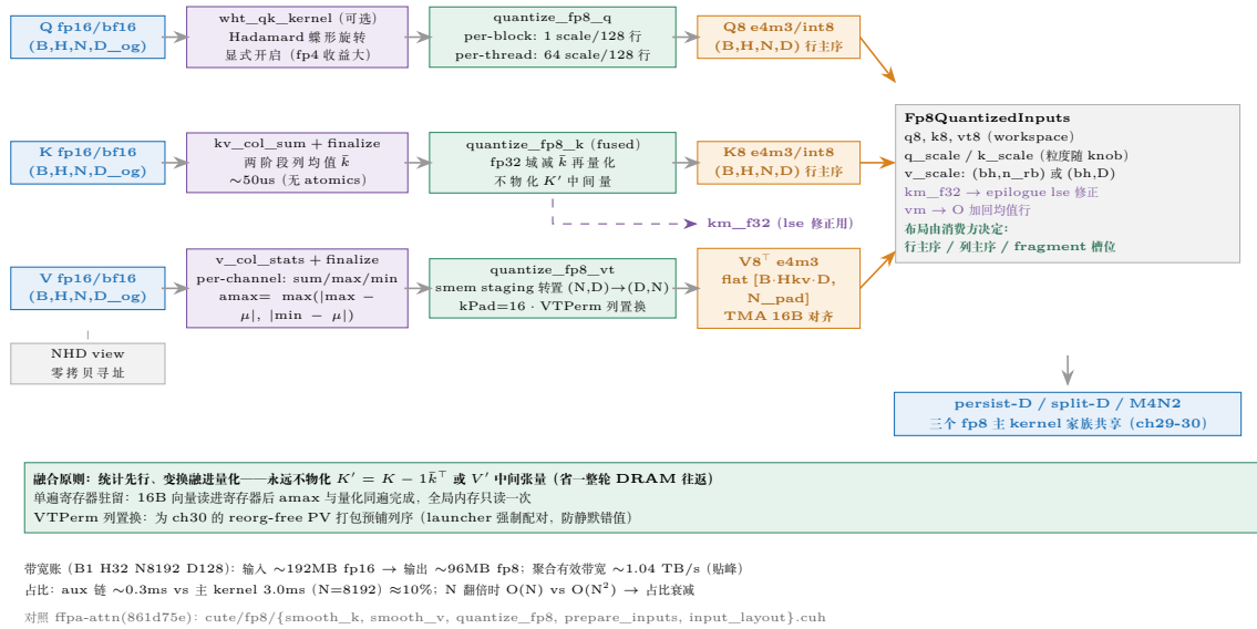
图 35.5: fp8 前处理链全景: 三泳道 (Q/K/V) 各自的统计 \rightarrow 变换 \rightarrow 量化 kernel 与输出 workspace 布局。smoothing 与量化融合在同一 kernel 内 (无中间落盘); V^T 的列 pad 兼顾 TMA 16B 对齐与置换写。
