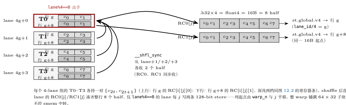
图 12.7: Epilogue shuffle 收拢与写回: 4-lane 组内 T0-T3 各持一对 \{c_{2t}, c_{2t+1}\} (上行 = 行 g 、下行 = 行 g+8 的寄存器对), __shfl_sync 从 \text{lane}+1/+2/+3 各收 2 个 half, 把 \text{RC0}[j] (行 g ) 与 \text{RC1}[j] (行 g+8 ) 各凑成 4 条 .b32 = 一条 16B float4 ; 随后仅 \text{lane}\%4==0 的 lane 出手, 行号 = \text{lane\_id}/4 = g , 两条 128-bit store 分别写行 g 与 g+8 。
