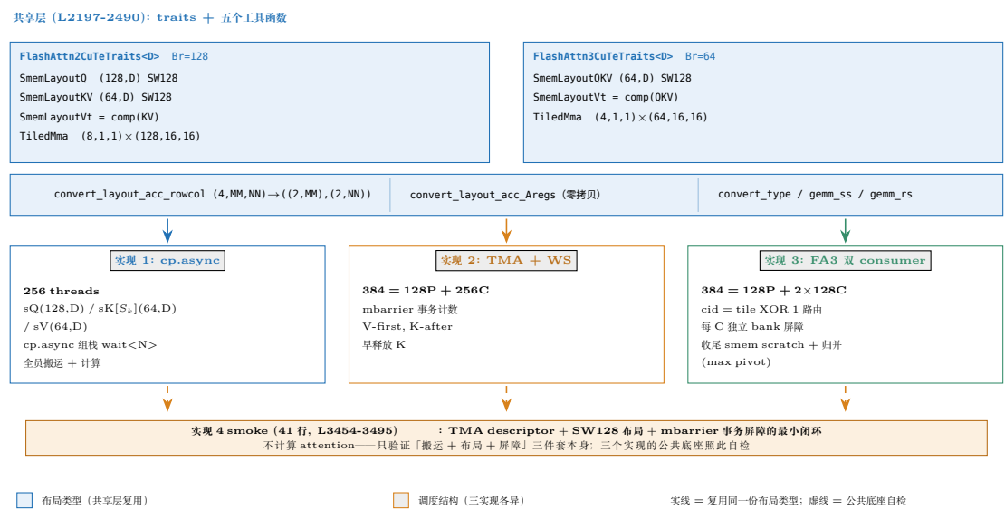
图 26.5: CuTe 块的四层结构: 共享 traits 与五个工具函数 (上), 三个 attention 实现 (中), 以及 41 行的 TMA 搬运自检 (底)。实线箭头表示「同一份布局类型被三种调度结构复用」, 虚线表示三个实现共用实现 4 的底座自检。
