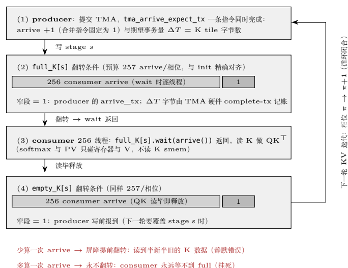
图 18.1: 固定 stage s 上 full/empty 两张屏障的相位收支循环（式 18.5 与式 18.6 的图形化）。每轮 KV 迭代：producer 提交 TMA 时用 tma_arrive_expect_tx 一条指令完成「arrive +1」与「声明 \Delta T 」两件事，TMA 硬件搬完后自动 complete-tx 记账；consumer 256 线程在 full_K[s].wait() 时各贡献一份 arrive（256 + 1 + tx 构成翻转条件），读毕 K 再各 arrive 一次释放 empty_K[s] ，producer 下一轮写前补上第 257 份。两边的 arrive 预算都是 257/轮，与 init 值精确对齐——多算一次挂死、少算一次静默错。窄段为可读放大，实际只占 1/257。
