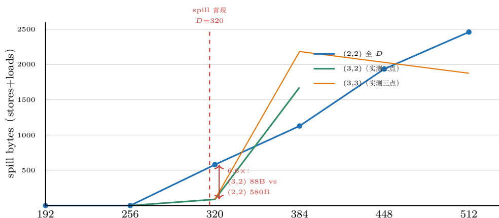
图 29.5: 寄存器溢出随 D 的增长 (nvcc -Xptxas -v, -O2, sm_120a, 各组合显式实例化)。 D \leq 256 全组合零 spill; D=320 (红色虚线) 是分水岭——所有组合顶到 255 寄存器上限并开始溢出, 且 (3,2)/(3,3) 的 88 B 与 (2,2) 的 580 B 相差 6.6 倍, 与 TFLOPS 排序 (204.1 对 188.3) 完全同序; D \geq 384 后 spill 基线过千, stages 加深进一步推高溢出 ((3,2) 1676 B、(3,3) 2184 B, 均高于 (2,2)), 流水掩蔽收益被吞掉, 最优组合回落 (2,2)。
