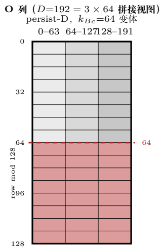
图 36.6: D=192 正确性 bug 的坏行定位 (29.7.1 节五步法的可视化)：把 O 视为 3 \times 64 列拼接，坏行集中在 \text{row mod } 128 \in [64, 127] (每个 128 行 Q tile 的后半)；N=512 几乎全错而 N=8192 仅 11% 行错 (N 稀释 \Rightarrow 特定 (row, kv-tile) 组合)；max_abs=2.66 对 mean_abs=0.011 的分裂是「个别行灾难」的强信号。
