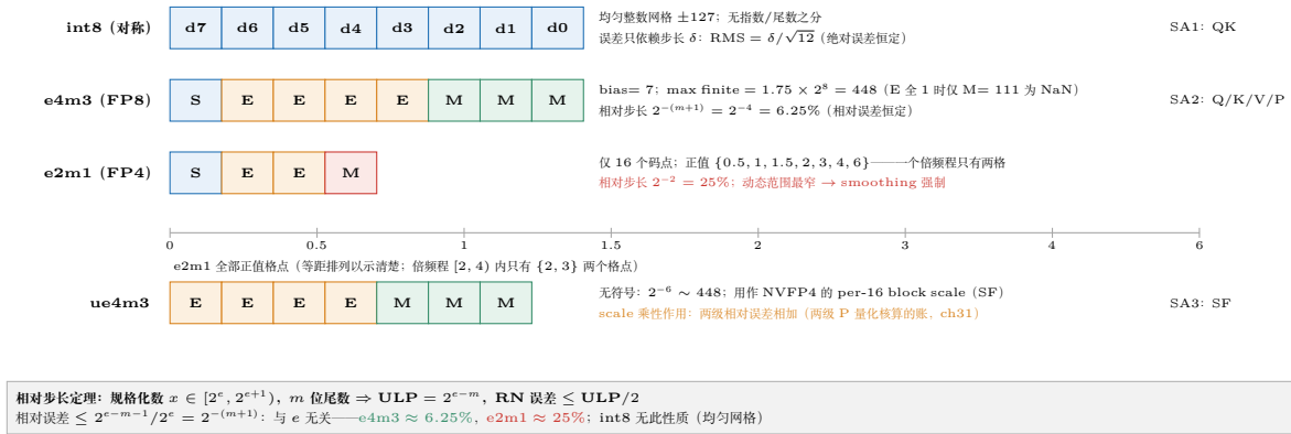
图 34.5: 四种量化格式的位域与值域对照 (int8 / e4m3 / e2m1 / ue4m3)。e4m3 的指数全 1 时仅 M=111 编码 NaN, 故满量程 448; e2m1 全部 16 个码点在数轴上标出, 直观呈现「一个倍频程内只有两格」。
