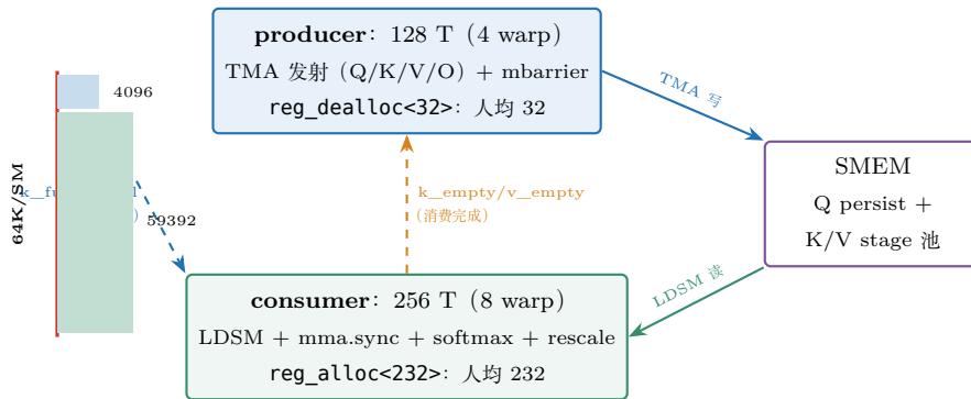
图 28.2: WS 双角色架构与 setmaxnreg 寄存器再分配。左: SM 寄存器池按式 (28.9) 重新切分, producer 只留 32/线程, consumer 拿 232/线程; 中: producer 只发 TMA、consumer 只算; 右: smem 是两者的交接面。实线箭头是数据流 (TMA 写入 \rightarrow LDSM 读出), 虚线箭头是 mbarrier 控制流 (full = 数据就绪、empty = 消费完成), 两者构成 §28.4.3 的握手协议。
