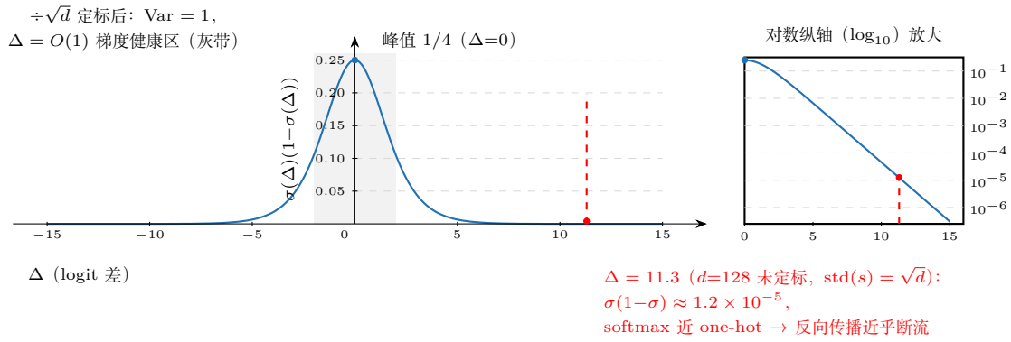
图 16.1: 1/\sqrt{d} 定标的饱和论证 (15.3.2 节, 式 16.6): sigmoid 梯度 \sigma(\Delta)(1-\sigma(\Delta)) 的峰值 1/4 在 \Delta = 0 ; 除以 \sqrt{d} 后 \text{Var} = 1 、 \Delta = O(1) (灰带), 梯度处于健康敏感区。不定标时 \text{std}(s) = \sqrt{d} (式 16.5), d = 128 即 \Delta \approx 11.3 , 梯度跌到 \approx 1.2 \times 10^{-5} ——线性纵轴上贴地, 右侧对数纵轴面板可见其仍在 10^{-5} 量级 (红点, 恰在 10^{-5} 网格线上方), softmax 近 one-hot、反向传播近乎断流。曲线偶对称, \Delta = -11.3 同理。
