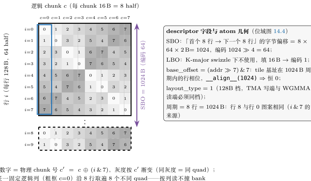
图 14.3: 128B swizzle 的 atom 几何与 WGMMMA descriptor 字段对应 (13.4.5 节): atom 为 8 行 \times 8 chunk (每 chunk 16B, 即 8 \times 64 half), TMA 写入后物理 chunk 号 c' = c \oplus (i \& 7) ——固定逻辑列 (粗框 c=0 ) 沿行取遍 8 个 quad, 按列读不撞 bank; 周期 8 行 = 1024B (行 8 与行 0 同图案), 对应 SBO = 1024B (编码 64)、base_offset 为 tile 基址在周期内的行相位 ( __align__(1024) 时恒 0)。位域编码见图 14.4; CuTe 的 SW128 原子视角 (第二十四章图 24.4) 与本章互为对照。
