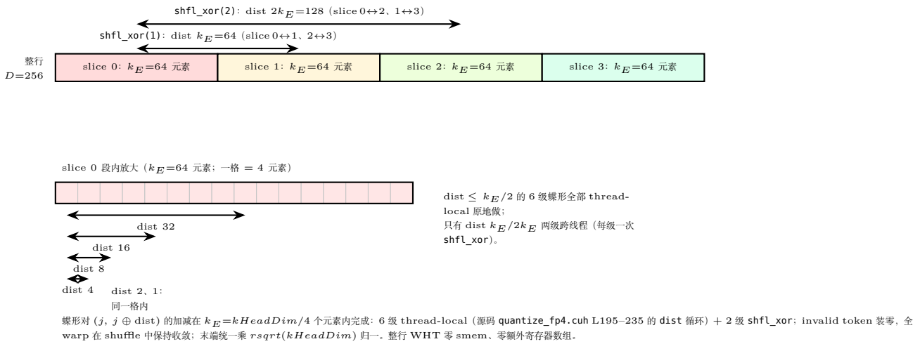
图 38.4: fused WHT 的蝶形距离分层 ( D=256 , 4 线程一 token、每线程 k_E=64 连续元素)。距离 < k_E 的 6 级蝶形全在 thread-local 数组内; dist k_E 与 2k_E 两级各用一次 shfl_xor(1)/shfl_xor(2) 跨 slice 交换——零 smem、零额外寄存器数组。
