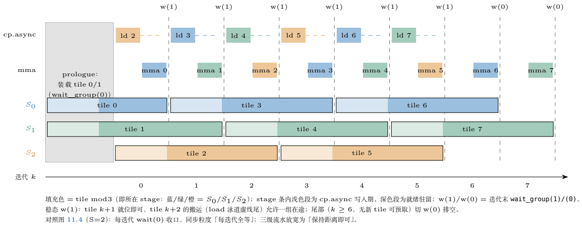
图 12.5: kStages= 3 三级流水时序: 迭代 k 读 S_{k \bmod 3} (tile k )、同时预取 (k+2) \bmod 3 (tile k+2 ) , 三个 stage 按 tile mod 3 轮转。稳态迭代末 wait_group(1) 允许一组搬运在途; 尾部无 tile 可预取时切 wait_group(0) 排空。与图 11.4 的两级流水 (每迭代 wait(0)) 相比, 同步粒度从「每迭代全等」放松为「保持距离即可」。
