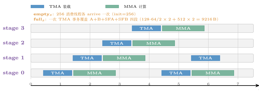
图 33.4: 四级流水的时序示意（ BN 取 128 的默认档；本卡 kStages 可用到 8~10 级，见 33.9.4 节扫描表）。与第三十一章图 31.2 的结构差别在 MMA 块的宽度：FP4 的一个 stage 只有一跳原子（ BK=64 ），K 方向不再有内层循环，MMA 块相对 TMA 块更窄——这意味着流水线对 TMA 延迟的容忍度更低，是 BN 翻倍的收益来源之一（ BN 翻倍 = MMA 块宽翻倍，而 TMA 字节数只涨 B 与 SFB 的部分）。
