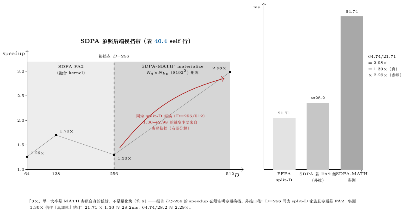
图 40.1: 参照系视角看表 40.4 的 self 行。左: SDPA 参照随 D 换挡——FA2 只覆盖 D \leq 256 , 更大 D 静默落到 MATH (materialize N_q \times N_{kv} 矩阵); 四个 speedup 点 (1.26/1.70/1.30/2.98×) 落在换挡带上, D=512 的跳变与 kernel 无关。右: D=512 的 2.98× 归因——以 D=256 同家族 (split-D、FA2 参照) 实测 1.30× 为真加速估计, MATH 参照自身再慢 \times 2.29 : 「3×」的大头是参照低效 (坑 6)。
