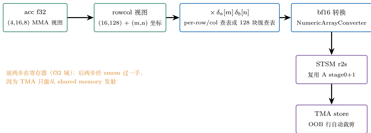
图 31.3: epilogue 数据流。整个反量化只在「scale 查表乘回」一步发生——这是式 30.4 把全部 scale 从主循环赶出去的直接回报：MMA 循环跑的是纯 e4m3 语义，epilogue 每元素额外开销只有一次乘法加一次查表（per-block 时查表索引是一次 128 整除，由编译器强度削减成移位）。
