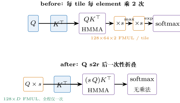
图 28.1: softmax scale 融合的数据流对照。上: 传统路径, S 从 QK GEMM 出来后在 softmax 的 max/exp 两个 pass 各乘一次 s = \text{scale} \cdot \log_2 e ; 下: 融合路径, s 在 Q s2r 后一次性乘进 A-fragment (persist-D 使 Q 对整个 KV 循环不变), HMMA 直接输出 log2 域分数, softmax 循环体内零 FMUL。等价性由式 (28.7)/(28.8) 保证; 代价是 s \odot Q 的一次 fp16 重舍入。
