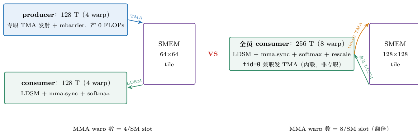
图 29.1: WS 与 non-WS 执行模型对照。左（第 二十七章 WS 教学版）：128 线程专职 producer 与 128 线程 consumer 分工，smem 为交接面——搬运与计算解耦的代价是 SM 上做 MMA 的 warp 只剩一半。右（本章）：256 线程全员 consumer， tid=0 在消费循环内联发射 TMA（发射指令本身不占独立 warp 的时间片，只占少量指令槽）；tile 同步升到 128 \times 128 ，MMA warp 数翻倍、算术强度上一档。大 D 下 O 累加器吃满寄存器预算， setmaxnreg 让渡不动，WS 的收益侧消失——non-WS 成为唯一选择。
