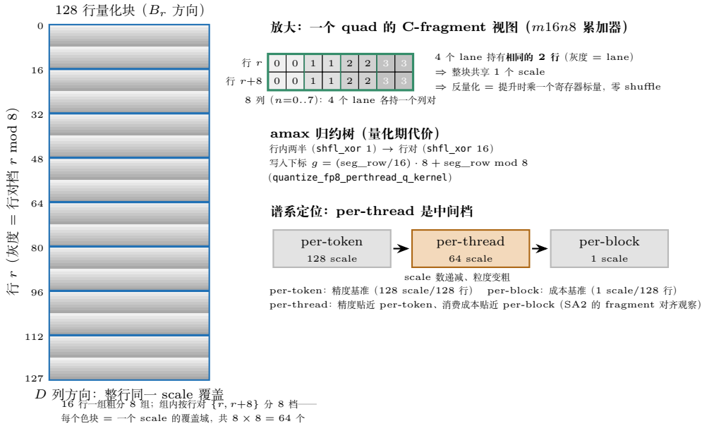
图 35.1: per-thread Q 量化的 64 槽位表与 quad 消费视角 ( quantize_fp8_perthread_q_kernel , 28.3.2 节)。左: 128 行量化块铺 8 \times 8 = 64 个 scale——行维按 16 行一组粗分 8 组 (粗边界), 组内按行对 \{r, r+8\} 分 8 档灰度 (行 r 与 r+8 同色), 每个色块就是一个 scale 的覆盖域; 写入下标 g = (\text{seg\_row}/16) \cdot 8 + \text{seg\_row} \bmod 8 。右上: 放大一个 quad 的 m16n8 C-fragment——4 个 lane 持有相同的 2 行、各占一个列对, 因此整块共享一个 scale, 反量化变成「fragment 提升时顺手乘一个寄存器标量」, 零 shuffle; 代价是 amax 归约树跨行对组合 (行内两半 shfl_xor 1 、行对 shfl_xor 16 )。下: 谱系定位——per-thread 是 per-token (128) 与 per-block (1) 之间的工程甜点。
