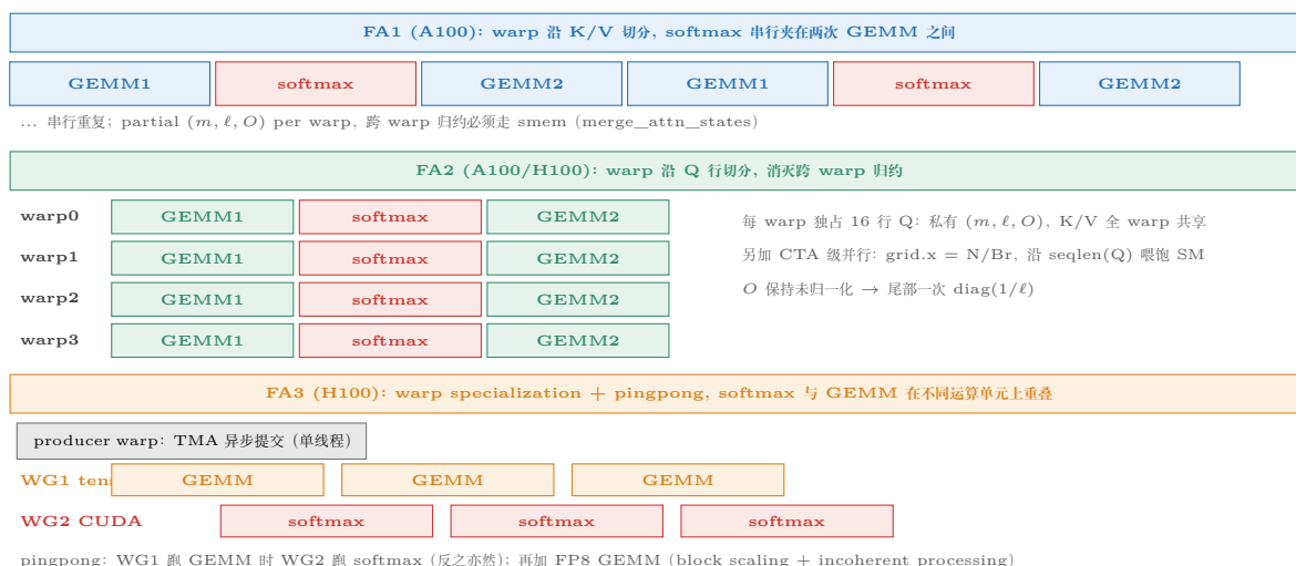
FA1 → FA2 → FA3: 时间去哪了 (时间结构示意图)
