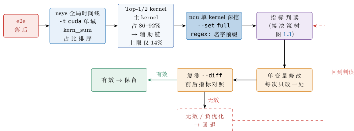
图 1.1: nsys → ncu → 单变量修改 → 复测 --diff 的闭环工作流：nsys 先给全局占比与优化预算（主 kernel 占 86–92%，辅助链上限仅 14%，对应 §1.8 例一）；ncu 只深挖 Top-1/2 kernel；每次只改一处，复测后无效立即回退、回到指标判读。配色：红 = 告警起点，蓝 = 采集/分析链，紫 = 判读决策点，橙 = 修改/复测动作，绿 = 有效保留，红虚线 = 无效回退。
