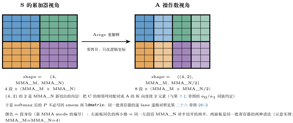
图 20.3: 零拷贝的寄存器重解释 (19.4.3 节 quote 块中 convert_layout_acc_Aregs 的模式级示意)。左: S 的累加器 layout 是 (MMA=4, MMA\_M, MMA\_N) ——4 个 MMA 重复段, 每段 MMA\_M \times MMA\_N ; 右: 同一批寄存器被读成 ((4, 2), MMA\_M, MMA\_N/2) ——沿 MMA\_N 切一刀得到 (2, MMA\_N/2) , 切出的 2 与原来的 4 配对成新的 8 段 MMA mode, 正是 PV 的 A 操作数所需的「K 向连续 2 元素」(与第 十七 章旗舰图的 a_0/a_1 配对同族)。数据一个比特都没动: 只是坐标重排, softmax 后的 P 因此不需要写回 smem 再 ldmatrix 。
