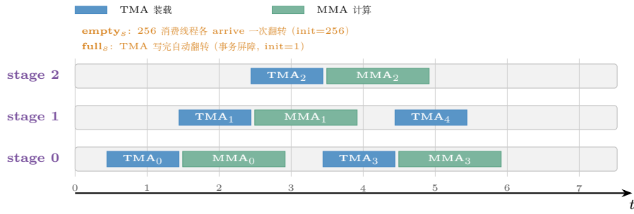
图 31.2: 三级流水的时序示意 (横轴时间、纵轴 stage 的矩阵视图)。TMA i 装载第 i 个 K-tile 到 stage i \bmod 3 , MMA i 消费之; 装载 i+3 要等 MMA i 的全体 arrive (empty 翻转), 消费 i 要等 TMA i 的事务完成 (full 翻转)。稳态下三条 TMA 与三条 MMA 在时间上错峰重叠——装载带宽与 tensor core 吞吐互不等待, 这正是 96 KB smem 买来的东西。
