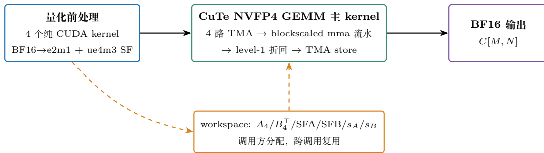
图 33.1: fp4_gemm_bf16 全链路。与第三十一章 (图 31.1) 同构, 唯一的结构差异是 workspace 里多出两份 SF: A 侧的 SFA 是 \lceil M/128 \rceil \cdot (K/64) 个 512B 原子, B 侧的 SFB 同理。SF 不是「辅助数据」, 它是 MMA 指令的操作数——主 kernel 必须为它单独开一条 TMA 通道、一块 smem、一个寄存器 fragment (33.4 与 33.5 节)。
