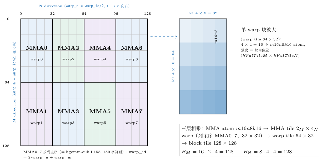
图 12.6: MMA warp 2 \times 4 排布 (左, 128 \times 128 block tile, 浅色 = warp 身份): MMA0–7 按列主序——N 向 MMA0/2/4/6、M 向 MMA1/3/5/7 ( \text{warp\_m} = \text{warp\_id} \% 2 变化快); 每 warp 块内 4 \times 4 个 m16n8 atom 小格。右: 单 warp 块放大 (warp tile 64 \times 32 , 蓝深 = atom 块内位置); 侧栏三层记号 B_M = 16 \cdot 2 \cdot 4 、 B_N = 8 \cdot 4 \cdot 4 。
