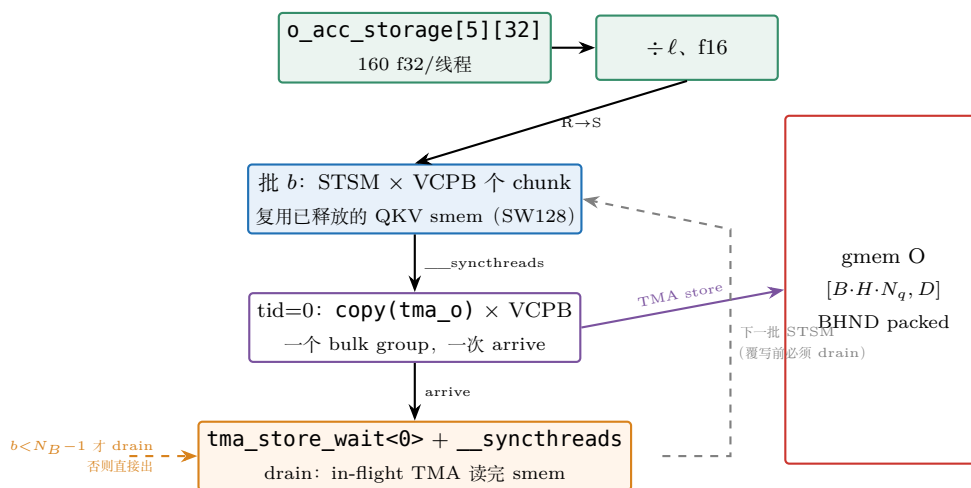
图 29.3: epilogue 的批量写出协议 ( D=320 : 5 个 v\_chunk 一批, VCPB = k_V ChunksPerBatch )。O 累加器除以 \ell 转 f16 后, STSM 把每 chunk 的 128 \times 64 分量暂存进复用的 QKV smem; tid=0 对批内所有 chunk 发 TMA store 并提交一个 bulk group。灰色回边是 drain race 的约束: 下一批的 STSM 要覆写同一段 smem, 必须等 in-flight TMA 读完 ( tma\_store\_wait<0> 只对发线程有意义, 配套 __syncthreads 让全 CTA 对齐; 末批免等直接收尾)。对比 WS 教学版的逐元素寄存器直写 gmem: 指令数从每线程 32C 次标量 store 降到 VCPB 次 STSM + 一次 bulk 提交。
