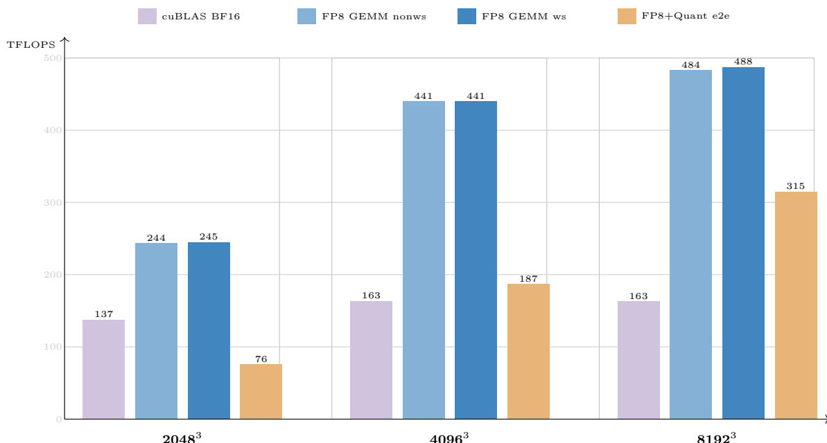
图 31.4: FP8 GEMM vs cuBLAS BF16 (PRO 5000, 越高越好; 默认档 128 \times 256/s2 )。三个规律: kernel-only 随 shape 增大从 1.77\times 爬到 2.99\times ——宽 tile 需要足够多的 tile 填满 110 个 SM, 2048^3 的 128 \times 256 grid 只有 128 个 CTA (35.8.4 节末的波次量化); e2e 的形状敏感度更陡: 2048^3 反而亏 ( 0.55\times ), 因为量化是 O(MK+NK) 的带宽型工序, GEMM 变小时它的占比线性放大 (35.8.2 节); WS 全程略优于 non-WS (寄存器有余量、setmaxnreg 有让渡空间, 35.6 节), 但差距远小于 attention 大 D 场景。图中 e2e 柱是「全链路量化」的保守口径; 权重 B 离线量化后 e2e 回到 226/411/429 T (35.8.3 节)。
