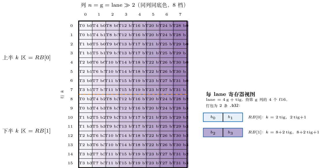
图 12.2: B fragment ( k16 \times n8 ) 寄存器布局, 式 12.2 的网格化 (图 12.1 的 B 侧姊妹图): 列 n = g = \text{lane} \gg 2 (同列同底色 8 档), 行 k 按 b_0 \rightarrow 2\text{tig} , b_1 \rightarrow 2\text{tig}+1 , b_2/b_3 再 +8 分布。右: 每 lane 4 个 f16 打包为 RB[0]/RB[1] 两条 .b32 。与 A 对照: A 按行分、B 按列分。
