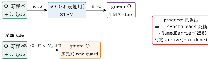
图 28.6: Epilogue 双路径。整 tile 走 R \rightarrow S \rightarrow G : STSM 把 O fragment 写进 (已完成使命的) Q smem 段, NamedBarrier 后由一个线程发射 TMA store——与装载对称的「反向 TMA 全链」。尾部 tile 行数不足 128, STSM/TMA 的整块写会越界, 退化为带行 guard 的 R \rightarrow G 。
