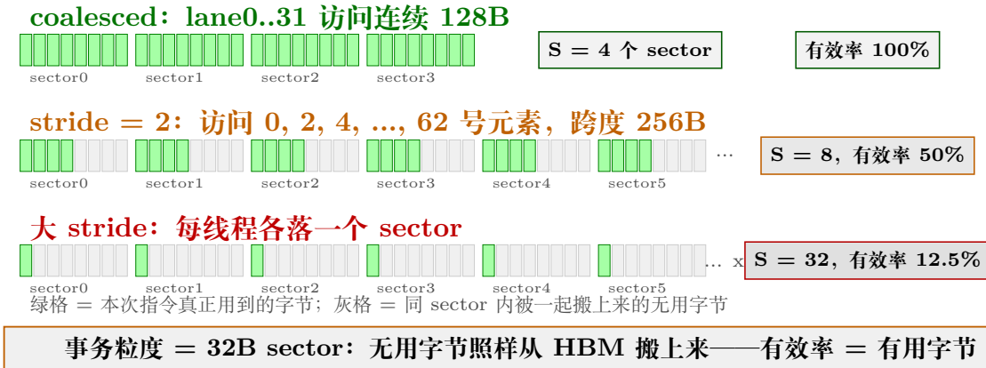
图 4.1: coalescing 与非合并访存对比 (fp32, 每格 4B, 一个 sector 8 格 32B): coalesced 一条指令落 4 个 sector 有效率 100%; stride=2 落 8 个、50%; 大 stride 每线程各占一个 sector、仅 12.5%——事务粒度是 32B sector, 无用字节照样从 HBM 搬上来。
