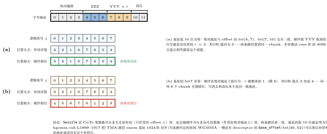
图 24.2: 位置无关与位置相关: 为什么 TMA 路径要求 smem 基址 1024 B 对齐 (3.5 节)。上方把字节地址的位段摆开: bit[4,7) 的 ZZZ 是 XOR 目标 (16B 块号), bit[7,10) 的 YYY 是源 (行号 r )。 (a) 基址低 10 位为零时, 绝对地址与 offset 的这两个字段一致, 布局求值与硬件相位给出同一个物理 chunk; (b) 基址一旦带 bit7, 硬件看到的行号整体抬 1, XOR 值随之改变, 写/读两条路径错位。
