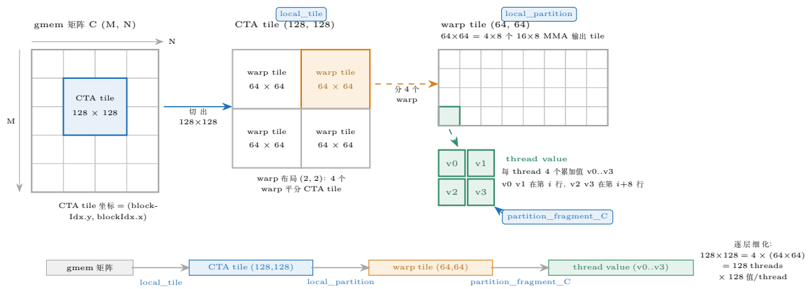
图 25.5: CuTe GEMM 的三层 partition: local_tile 以 (blockIdx.y, blockIdx.x) 为坐标从 gmeme 切出 CTA tile (128,128); warp 布局 (2,2) 下 local_partition 平分给 4 个 warp 得 (64,64); warp tile 由 4 \times 8 个 16 \times 8 atom 铺满, partition_fragment_C 为每 thread 生成累加器片段 (单 MMA tile 内 2 \times 2 四值, v0/v1 在第 i 行、v2/v3 在第 i+8 行)。层级换算 128 \times 128 = 4 \times (64 \times 64) = 128 \text{ threads} \times 128 \text{ 值/thread} 。重建自 @reed 《cute 之简单 GEMM 实现》(示意图为经典 4-warp/64 × 64 配置; 本章 kernel 实为 tile 32 × 32、warp 16 × 16, 层级方法相同)。
