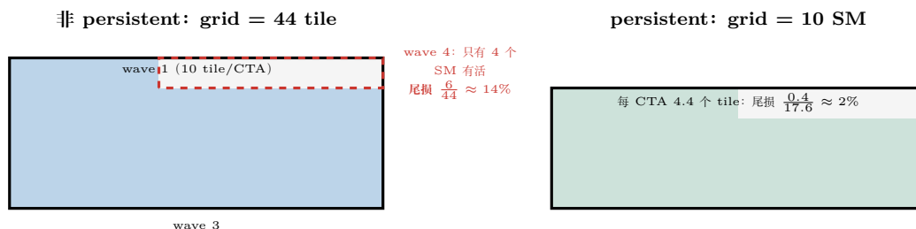
图 28.5: wave 量化尾损示意 (10 个 SM、44 个 tile 的缩小模型)。左：非 persistent launch 按整 wave 调度，最后一个 wave 只有 4 个 SM 在算，其余空转满一个 tile 时长；右：persistent CTA 把 grid 收缩到 SM 数，每个 CTA 串行吃 \lceil 44/10 \rceil 或 \lfloor 44/10 \rfloor 个 tile，不均衡被压缩到最后一个 tile 的零头。真实场景 (110 SM, H=32/N=8192 ) dense 收益 +2%~6%； causal 反向 ——tile 负载前轻后重，线性分配会把重 tile 锁死在同一批 CTA 上（实测 -9% ~ -21%），此时必须回退全量 grid 让硬件调度器自然均衡。
