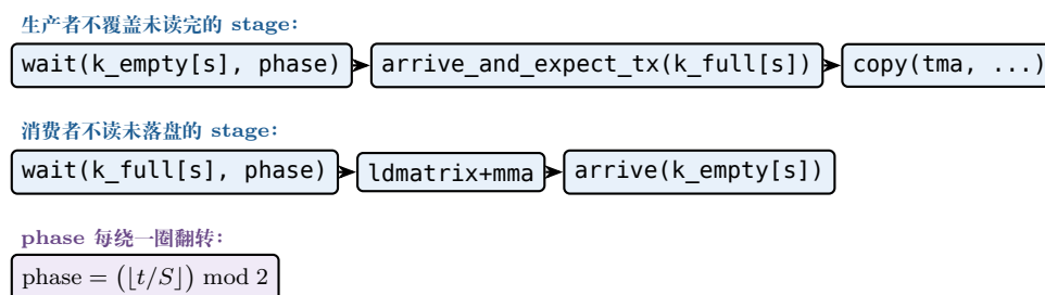
图 26.3: TMA 事务计数协议的两条不变量 (26.3.5 节)：生产者 wait 到空 stage 才覆盖写入、消费者 wait 到满 stage 才读、phase 每绕 S 个 stage 翻转一次。
