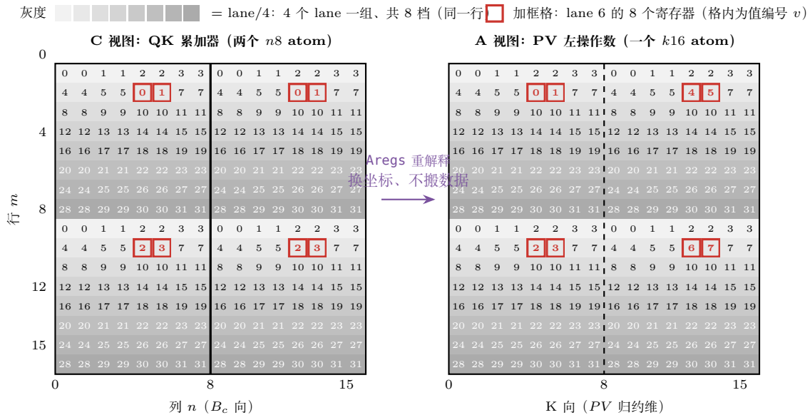
图 26.2: C fragment \rightarrow A fragment 的零拷贝重解释 (convert_layout_acc_Aregs)。左右两图是同一批寄存器的两套坐标读法: 每格标注持有它的 lane, 灰度按 lane/4 分 8 档 (4 个 lane 一组, 与第 17 章 fragment 图的分组语义一致), 两图的格子位置与 lane 归属逐格恒等——这正是「数据一个比特都不用改」的几何形态。差别只在分组与编号: 左图按 n8 累加器约定, 值编号 v = d_0 + 2d_1 在每个 atom 内各自循环 0..3 ( (c_0, c_1) 同行相邻两列、 (c_2, c_3) 行偏移 +8, 即 bit0= 列、bit1= 行); 右图按 k16 A 操作数约定读同一批格子, 值编号变 v = d_0 + 2d_1 + 4d_2 连续 0..7——第二个 n8 atom 的列对成为 K 向的 k \in [8, 16) (虚线半块, d_2=1 )。加框示例 lane 6 的 8 格在两图位置完全相同、编号从「两轮 0..3」变「一轮 0..7」, 即式 (26.8) 的「列拆半 + 重新配对」。
