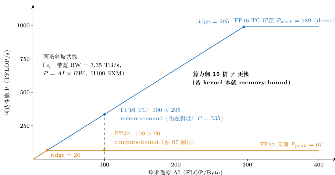
图 2.4: 同一 GPU 的两条屋顶线 (H100 SXM): FP32 ( P_{\text{peak}} = 67 TFLOP/s, ridge = 20) 与 FP16 TC dense ( P_{\text{peak}} = 989 , ridge = 295) 共用同一条带宽斜坡 ( BW = 3.35 TB/s), 脊点相差约 15 倍。AI=100 的竖虚线在两条线上落点相反: FP32 侧已 compute-bound ( 100 > 20 ), FP16 TC 侧仍 memory-bound ( 100 < 295 ) —— 把 kernel 迁到 Tensor Core 未必变快; ridge 口径算错 (如 sparse 当 dense) 会把 bound 类别判反。
