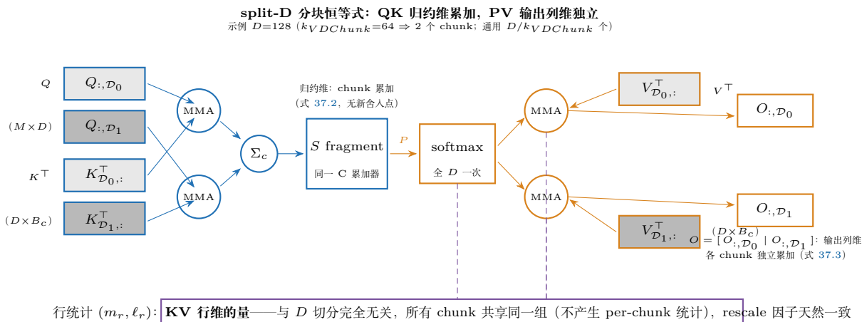
图 37.1: split-D 分块恒等式的数据流 (30.3.1 节)。QK 侧: D 是归约维, 各 chunk 的 Q_{:,D_c} K_{D_c,:}^\top 累加进同一个 S fragment (式 37.2, f32/s32 累加, 不引入新舍入点); PV 侧: D 是输出列维, 各 chunk 独立累加出 O_{:,D_c} 列段 (式 37.3), 无任何合并。softmax 的行统计 ( m_r, \ell_r ) 是 KV 行维的量——与 D 切分完全无关, 所有 chunk 共享同一组 (灰色 = chunk 身份, 两图同语义)。
