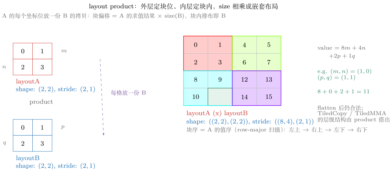
图 21.10: layout product: A 的每个坐标位放一份 B 的拷贝 (块偏移 = A 的线性序号 \times size(B)), 得到嵌套布局 ((2,2),(2,2)):((8,4),(2,1))。行值 0,1,4,5/2,3,6,7/... 的「块拷贝拼接」排布即 product 的几何签名——它不是 row-major。重建自 @ 竹熙佳处《写给大家看的 CuTe 教程: Layout Product & Divide》。
