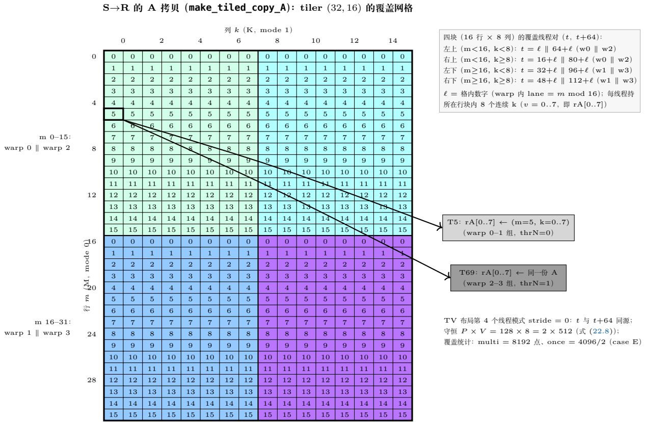
图 22.3: S→R A 拷贝的 2 倍重复因子 (式 (22.9)、测试 case D/E): tiler (32, 16) 的 A tile ( M \times K ) 上, 每格标 warp 内 lane 号 \ell = m \bmod 16 , 格子的实际覆盖线程对为 (基址 +\ell , 基址 +64+\ell ), 四块的基址见右上表 (w0-w3 即 warp 0-3)。每个元素恰被 2 个 (thread, value) 对覆盖: t 与 t+64 (两个 N 方向 warp, thrN = 0/1) 各持同一行块 8 个连续 k 的一份寄存器拷贝——TV 布局第 4 个线程模式 stride 为 0 的几何含义, 守恒 128 \times 8 = 2 \times 512 。对照图 22.5 的 G→S 双射网格 (每格恰一线程)。
