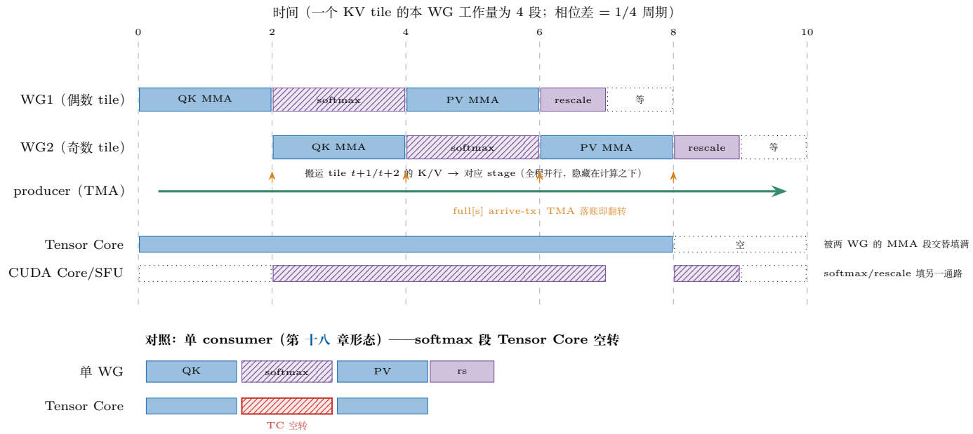
图 19.4: 双 consumer 的相位交错时序 (18.4.6 节统计性交错的图形化)。上: WG1/WG2 各按「QK MMA → softmax → PV MMA → rescale」四段推进自己的 KV tile 子序列, 两 WG 相位差 1/4 周期——WG1 处于 MMA 段时 WG2 大概率处于 softmax/rescale 段; producer 的 TMA 全程并行, 落账即 arrive-tx 翻转 full[s] 。中: Tensor Core 与 CUDA Core/SFU 两条资源条被两路计算交替填满 (同步 mma.sync 做不到 WG 内重叠, 靠两路独立流在硬件调度器上统计性交错)。下: 单 consumer (第 十八 章形态) 的对照——softmax 段 Tensor Core 只能空转, 这正是第二个 consumer 要填的洞。
