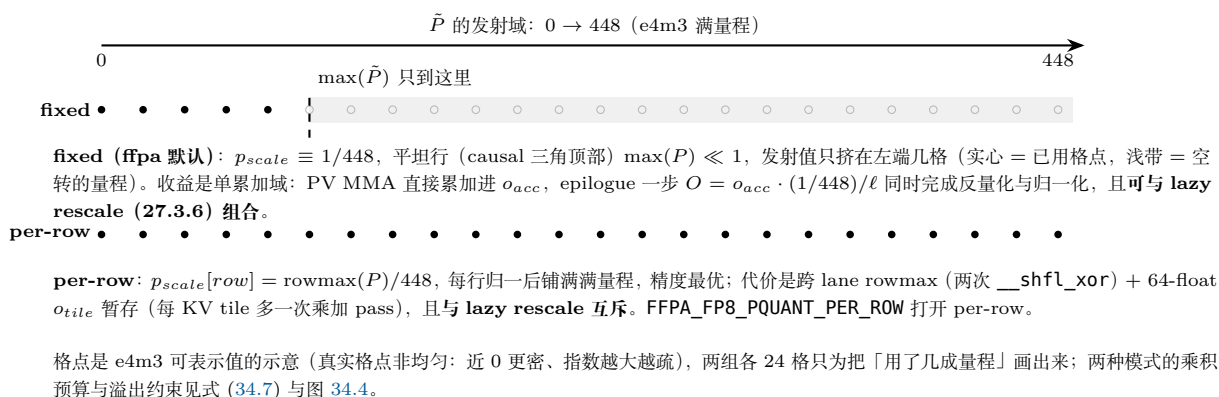
图 34.2: fixed 与 per-row 两种 p_{scale} 策略的发射域利用率 (27.3.5 节)。上: fixed 的 p_{scale} \equiv 1/448 是编译期常数, 平坦行的 \max(P) \ll 1 使发射值只占量程左端一小段, 其余量程空转——换来的是单累加域与「可与 lazy rescale 组合」; 下: per-row 用 \text{rowmax}(P)/448 把每一行拉满, 精度最优, 代价是跨 lane rowmax 归约与 64-float 的 o_{tile} 暂存, 且与 lazy rescale 互斥。
