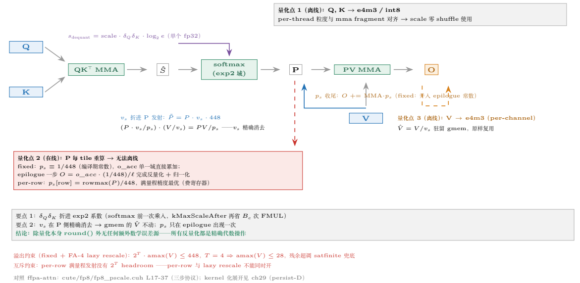
图 34.6: attention 的三个量化点与 scale 流向: \delta_Q \delta_K 折进 exp2 系数 (式 34.4)、 v_s 在 P 侧精确消去 (式 34.5)、 p_{scale} 在 epilogue 一步收尾。
