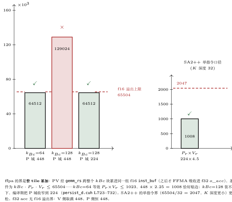
图 36.1: f16 PV 累加器的整 tile 域预算 (式 36.4)。条形为 kBc \times P_r \times V_r : kBc=64 与「 kBc=128 + P 域自动收窄到 224」都恰为 64512, 贴住 65504 上限; kBc=128 且 P 仍 448 则 129024 约 2 倍超限。右: SA2++ 按单条 MMA ( K=32 ) 核算的界 2047 更松 ( P_r=224, V_r=4.5 双侧收窄)。f32 acc 路径无此约束。
