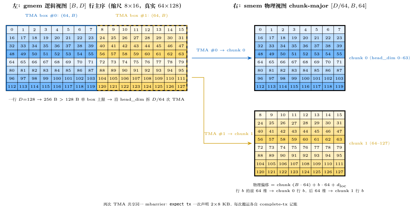
图 18.2: chunk-major 布局与双 TMA 拆分 (17.4.3 节, 缩尺示意: 8 \times 16 代表真实 64 \times 128 )。左: gmem 里 K/V 的逻辑视图 [B, D] 行主序, cell 填逻辑线性 idx ( = b \cdot D + d 的缩尺版本); D=128 时一行 256 B 超出 128B swizzle box 的维上限, 两个 box (head_dim 0-63 / 64-127) 各搬一半。右: smem 物理视图写成 chunk-major [D/64, B, 64] ——同一批数据 (idx 一一对应) 被拆成两个连续的 64 \times 64 chunk 面板, 行 b 的前后 64 维分别落在 chunk 0/1 的行 b 。两次 TMA 共享同一个 mbarrier, expect_tx 一次声明总字节、两次 complete_tx 各自记账, 协议数学不变。
