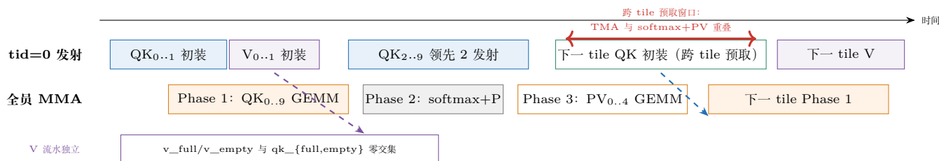
图 29.2: 单 kv_tile 内的相位时间线与跨 tile 预取 ( S_K=S_V=2 , D=320 的 10+5 chunk 结构示意)。上线是 tid=0 的发射序列: 初始预取填满两条流水, 主循环内每个 QK chunk 消费完领先 S_K 发下一个, V 预取每 tile 开头补一批; 本 tile QK 相位一结束 (stage 池整体空闲), 立刻发射下一 tile 的初始 QK chunk。下线是全员 MMA 的计算序列。红色双箭头是本章协议的核心红利: 下一 tile 的 QK 装载与本 tile 的 softmax (纯寄存器 + shfl) 和 PV GEMM 完全重叠——QK/V 两套 barrier 集不相交保证这段发射不会与后续相位互相等待。
