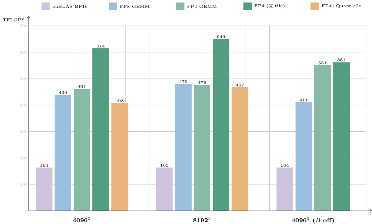
图 33.6: NVFP4 GEMM vs cuBLAS BF16 (PRO 5000, 越高越好)。三条读法: 其一, kernel-only 口径下 FP4 只比 FP8 快 6 ~ 40%——库默认档 (128 2 /s4, 柱取口径: 4096 3 取扫描表 461 T, 8192 3 取默认档实测 476 T) 只快 6%, 宽 tile 档才快 40%, 远不是比特数暗示的 2×; 原因是本 kernel 走 bf16 输出、f32 累加, 且 BK=64 让 K 方向的算术强度下降 (表 33.1 的两条「钉死」); 其二, 宽 tile (128×256) 是本章最大的单项收益 (+31%, 33.9.4 节), 也是 --bench 标准行在 MNK \geq 4096 上的自适应选择; 其三, e2e 口径下 FP4 反超 FP8 (4096 3 : 408 vs 187 T; 8192 3 : 467 vs 315 T)——量化的写出字节数只有 FP8 的一半, B 侧重重构后这个差距被彻底拉开 (33.9.3 节); 第三组 ( B 离线) 把 FP4 的 e2e 拉回 551~561 T (FP8 为 411 T), 是各自 kernel 的 91 ~ 93%。
