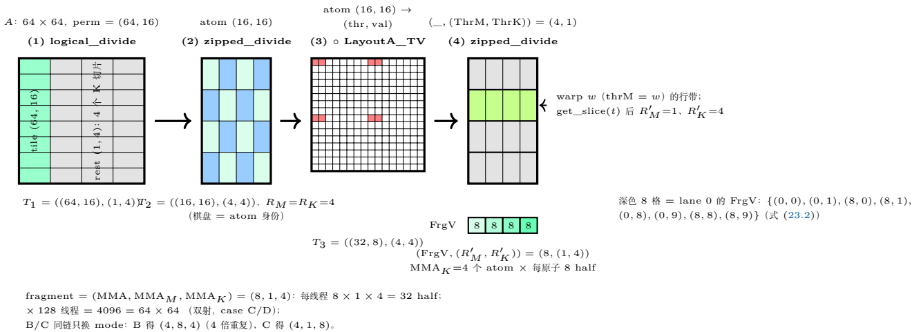
图 23.1: thrfrg_A 四步推导链 (式 (23.7)–(23.10)) 在 FFPA QK (tile 64 \times 64 \times 16 、AtomLayout (4, 1, 1)、Q 为 64 \times 64 ) 上的 shape 演化: (1) logical_divide 按 tile 切出 (64, 16) 与 4 个 K 切片; (2) zipped_divide 按 atom (16, 16) 切成 4 \times 4 个原子块; (3) 复合 LayoutA_TV 把原子内坐标换成 (线程, 值)，深色 8 格即 lane 0 的 FrgV; (4) 按 (ThrM, ThrK) = (4, 1) 剥出 warp 行带，get_slice( t ) 后每线程 fragment = (8, (1, 4)) = 32 half (右下: FrgV = 8 \times \text{MMA}_K = 4 )。
