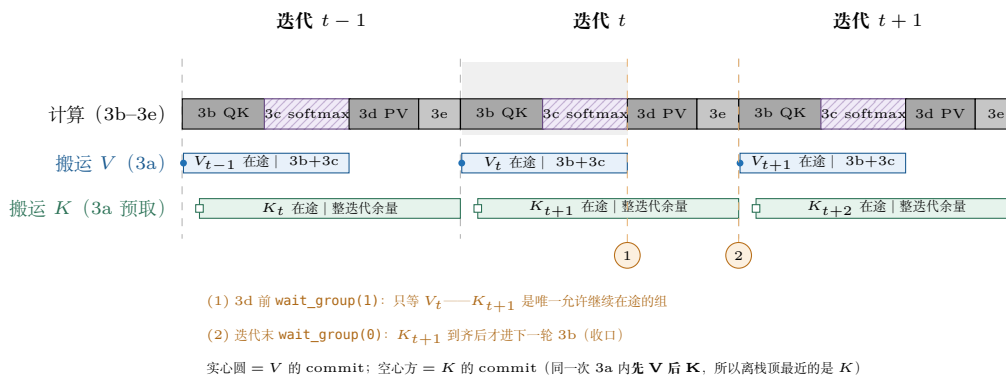
图 17.4: K 双缓冲、 V 单级的流水时序 (16.4.5 节 3a 步)。三个稳态迭代 t-1/t/t+1 : 每个迭代内 3a 依次提交两组搬运—— V_t (实心圆, 写当前 V buffer) 与 K_{t+1} (空心方, 写 smem_sel_next )。 V_t 的在途窗口 (蓝条) 恰好覆盖同迭代的 3b (QK mma) 与 3c (softmax)——softmax 全在 CUDA Core/SFU 上跑, 正好填满 V 的搬运延迟; K_{t+1} 则有整整一个迭代的余量。两处等待: (1) 3d 前的 wait_group(1) 只等 V_t , 把 K_{t+1} 留在途; (2) 迭代末 (3e 之后) 的 wait_group(0) 收口 K_{t+1} 才进下一轮 3b。与第 12 章 GEMM 的「kStages 全操作数统一多级」不同——attention 两段 mma 之间夹着一段非 mma 计算, 天然提供了第二级的隐藏窗口, 所以 kStagesK=2 就够 (「one stage is enough for V 」)。
