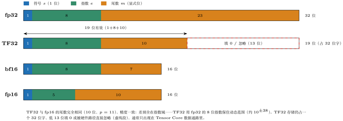
图 11.1: 四种浮点格式的位域条 (与表 11.1 同序, 按位宽比例绘制): 蓝 = 符号位、绿 = 指数、橙 = 显式尾数。TF32 砍掉 fp32 尾数低 13 位 (红色虚线框: 填 0 / 忽略), 保留 1+8+10 共 19 位; bf16/fp16 只有 16 位, 指数域分别为 8 与 5。
