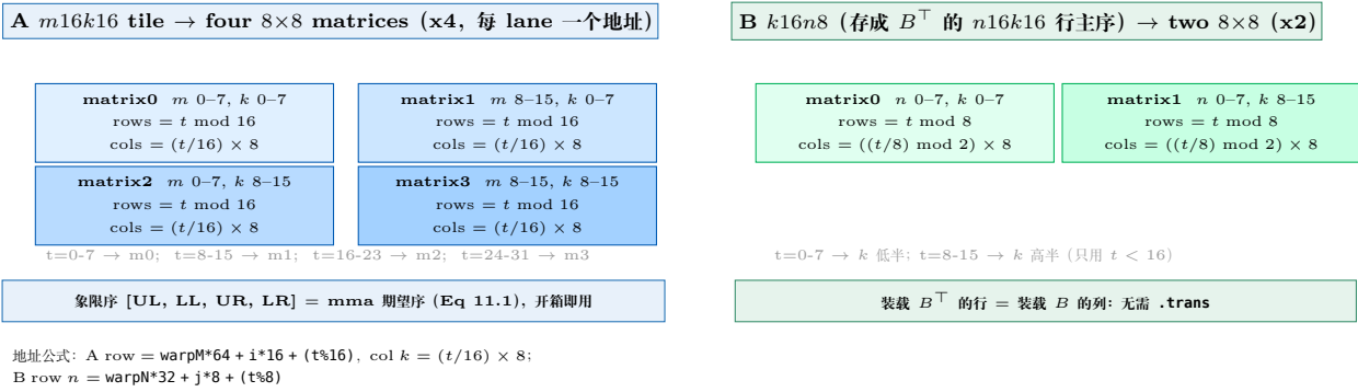
图 12.4: 本章 kernel 的 ldmatrix 寻址映射: A 用 x4 一次装载 m16 \times k16 的四象限 (象限序恰为 mma 期望序); B 用 x2 装载 k16 \times n8 (借 B^T 行主序存储, 无需.trans)。
