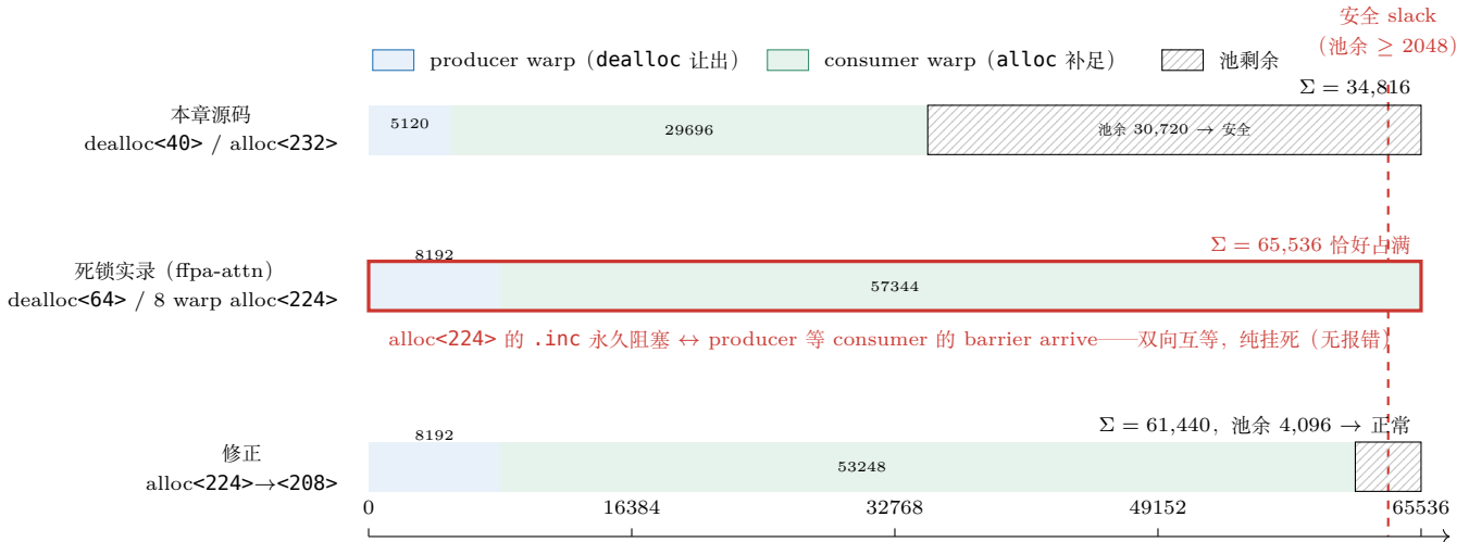
图 15.1: setmaxnreg 的 CTA 寄存器池三配置对照 (式 15.4, 每 SM 寄存器文件共 65,536 个 32-bit 寄存器): 条形按 \sum_w 32r_w 堆叠 producer ( dealloc 让出) 与 consumer ( alloc 补足) 两段, 红色虚线为工程安全界 (池余 \geq 2048 )。① 本章源码 dealloc<40>/alloc<232> : 5120 + 29696 = 34816 , 池余 30720, 安全; ② ffpa-attn 调优实录的死锁配置 dealloc<64> + 8 warp \times alloc<224> : 8192 + 57344 = 65536 恰好占满——有效池 < 65536 , .inc 永远凑不齐而阻塞在 setmaxnreg 上, 与 producer 等 barrier arrive 形成双向互等, 纯挂死; ③ alloc 降到 208: 总 61440、池余 4096, 恢复正常。
