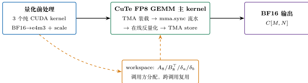
图 31.1: fp8_gemm_bf16 全链路: 一次调用在给定 stream 上先发射量化 kernel (第 三十 章), 再发射主 kernel, 同步语义与 cuBLAS 一致 (入队即返回, 调用方在 stream 上同步)。所有中间张量都住在 workspace 里, 主 kernel 通过模板参数拿到量化输出的 e4m3 指针与 scale 指针——两级之间没有额外的拷贝或布局变换。
