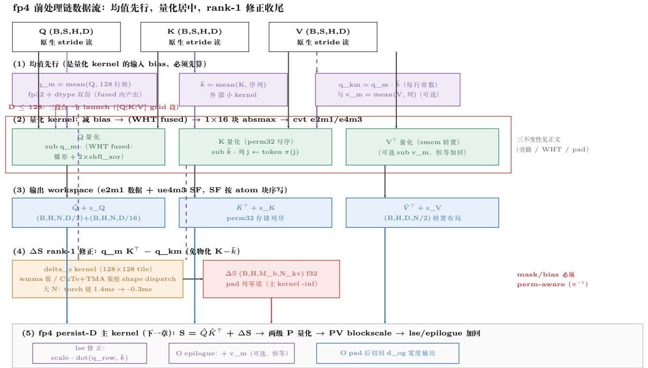
图 38.6: fp4 前处理链数据流 ( D \leq 128 走 fused 单 launch 路径): \bar{k}/q_m 均值先行的原因是它们是量化 kernel 的输入 bias; hadamard 下 q_m^{rot} 在 fused kernel 内顺带产出。
