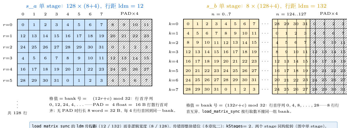
图 11.3: s\_a / s\_b 的 padded 行距布局 (单 stage, 格值为该 word 的 bank 号 = 行距 \times r + 列 \bmod 32 , 斜线格为 PAD)。左 s\_a : 128 \times (8+4) , ldm=12 , 行首 bank 序列 0, 12, 24, 4, ...; 右 s\_b : 8 \times (128+4) , ldm=132 , 行首 bank 序列 0, 4, ..., 28。补 4 float (16 B) PAD 打散行首对齐、消除 load_matrix_sync 按行取数的 bank conflict——ldm 取行距而非逻辑宽度。
