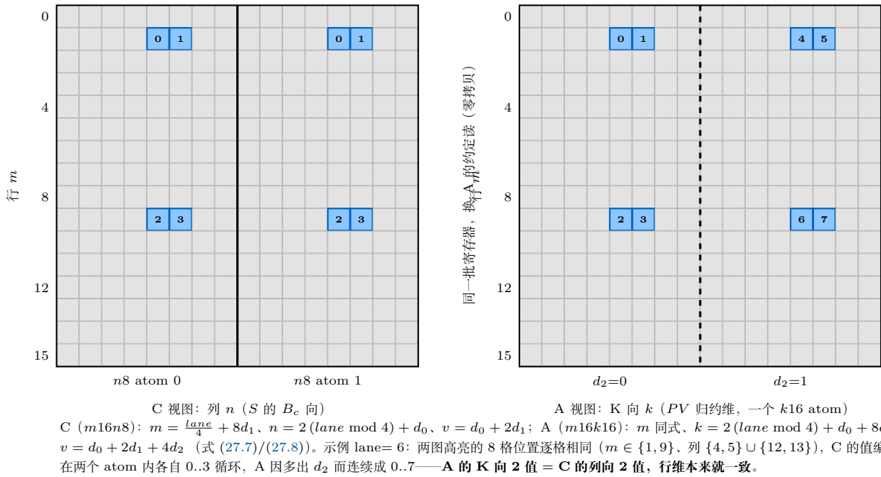
图 27.2: C 与 A fragment 的线程-值映射逐位对照 (式 (27.7)/(27.8))。左: S 的 C 视图——两个 n8 atom 拼成 16 列, 格内数字是 lane 6 所持值的编号 v = d_0 + 2d_1 (在每个 atom 内循环 0..3); 右: P 的 A 视图——同一个 k16 atom, lane 6 持有同样的 8 个格, 值编号变成 v = d_0 + 2d_1 + 4d_2 连续 0..7, 其中 d_2=1 的 4 格来自 C 的第二个 n8 atom (虚线半块)。两图高亮位置逐格相同、数据指针不换: 重解释只把「列向相邻 2 值」的约定换成「K 向相邻 2 值」, 行维 ( m ) 的映射本来就一致。
