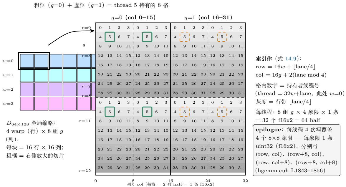
图 14.2: WGMMMA m64n128k16 输出 D 的寄存器分布 (13.3.4 节, 式 14.9): 左为 64 \times 128 全局缩略 (4 warp \times 8 组 g , 每块 16 行 \times 16 列); 右侧放大 warp w=0 的 16 行切片 ( g=0, 1 两组, 每格一条 f16x2 = 相邻 2 列), 格内数字为持有该输出的线程号、灰度按行带 \lfloor \text{lane}/4 \rfloor 区分。索引律 \text{row} = 16w + \lfloor \text{lane}/4 \rfloor 、 \text{col} = 16g + 2(\text{lane} \bmod 4) 使每个线程在每组 g 内恰好持有 4 个 8 \times 8 象限里各一条寄存器 (粗框/虚框标出 thread 5 的 8 格), epilogue 据此用 4 次写覆盖 4 个象限。
