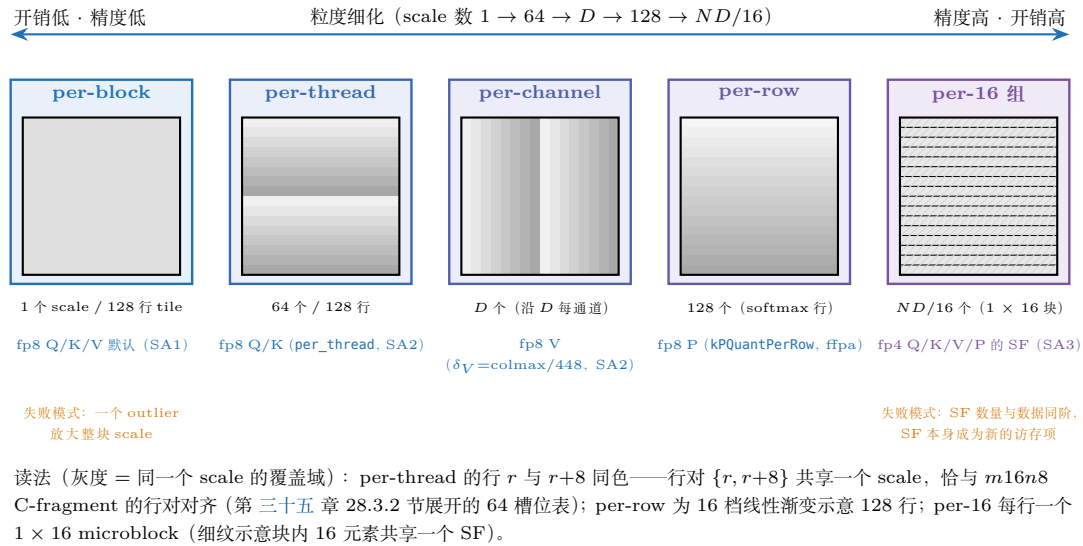
图 34.1: 量化粒度谱系五列网格 (表 34.2 的可视化, 缩略网格为 16 行 \times 16 列)。从左到右: per-block 整块共享 1 个 scale; per-thread 按 C-fragment 行对 \{r, r+8\} 分档 (128 行块共 8 \times 8 = 64 个, 零 shuffle 消费); per-channel 沿 D 每通道一个; per-row 每 softmax 行一个 (128 个); per-16 每行一个 1 \times 16 microblock (NVFP4 的 SF)。顶部双向轴是整条谱系的 trade-off: 粒度越细精度越高, 但 scale 的存储、传递与消去开销同步上涨, 且必须与 MMA 的 fragment 布局对齐——谱系两端的失败模式分别是对 outlier 的脆弱性与 SF 自身的访存开销。
