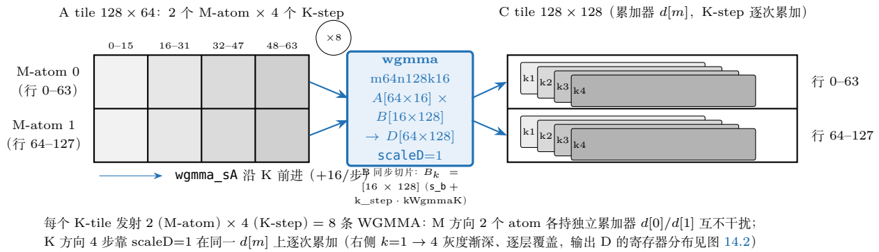
图 14.1: 一个 K-tile 的 8 条 WGMMMA 拼出 C tile (C2 双层循环): A tile 128 \times 64 按 M 方向切 2 个 64 行 M-atom、K 方向切 4 个 kWgmmaK=16 的 K-step，对每个 (M-atom, K-step) 发射一条 wgmma.m64n128k16 ——A 指针 wgmma_sA 沿 K 每步前进 16 (本 kernel 即 m 循环 \times k\_step 循环)，B 从 s_b 同步切 [16 \times 128] 片；4 次 K-step 靠 scaleD=1 在同一累加器 d[m] 上逐次累加 (C tile 内 k=1 \rightarrow 4 灰度渐深)，2 个 M-atom 各持独立累加器 d[0]/d[1] 。
