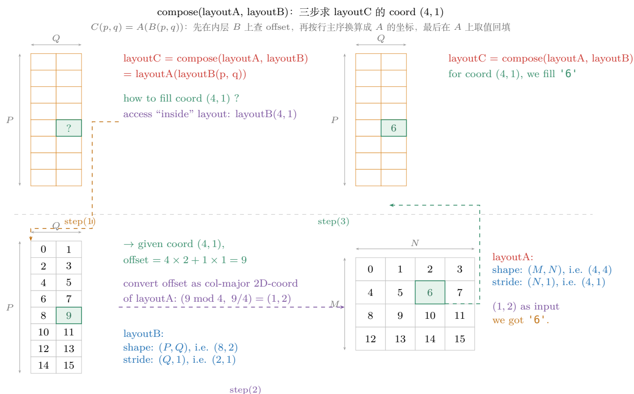
图 21.7: compose(A, B) 的三步求值: 先查内层 B 得 offset, 再按外层 A 的 shape 把 offset 换算回坐标, 最后查 A 得最终值。例: C(4, 1) \rightarrow B(4, 1) = 9 \rightarrow (9 \bmod 4, 9/4) = (1, 2) \rightarrow A(1, 2) = 6 回填 C。重建自同上文。
