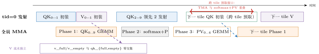
图 29.2: 单 kv_tile 内的相位时间线与跨 tile 预取 ( S_K=S_V=2 , D=320 的 10+5 chunk 结构示意图)。上排是 tid=0 的发射序列: 初始预取填满两条流水, 主循环内每个 QK chunk 消费完领先 S_K 发下一个, V 预取每 tile 开头补一批; 本 tile QK 相位一结束 (stage 池整体空闲), 立刻发射下一 tile 的初始 QK chunk。下排是全员 MMA 的计算序列。红色双箭头是本章协议的核心收益: 下一 tile 的 QK 装载与本 tile 的 softmax (纯寄存器 + shfl) 和 PV GEMM 完全重叠——QK/V 两套 barrier 集不相交保证这段发射不会与后续相位互相等待。
