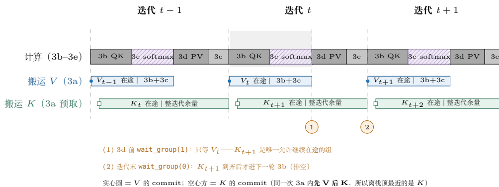
图 17.4: K 双缓冲、 V 单级的流水时序 (16.4.5 节 3a 步)。三个稳态迭代 t-1/t/t+1 : 每个迭代内 3a 依次提交两组搬运—— V_t (实心圆, 写当前 V buffer) 与 K_{t+1} (空心方, 写 smem_sel_next )。 V_t 的在途窗口 (蓝条) 恰好覆盖同迭代的 3b (QK mma) 与 3c (softmax) ——softmax 全在 CUDA Core/SFU 上跑, 恰好掩盖 V 的搬运延迟; K_{t+1} 则有整整一个迭代的余量。两处等待: (1) 3d 前的 wait_group(1) 只等 V_t , 把 K_{t+1} 留在途; (2) 迭代末 (3e 之后) 的 wait_group(0) 等 K_{t+1} 到齐才进下一轮 3b。与第 12 章 GEMM 的「kStages 全操作数统一多级」不同——attention 两段 mma 之间夹着一段非 mma 计算, 天然提供了第二级的隐藏窗口, 所以 kStagesK=2 就够 (「one stage is enough for V 」)。
