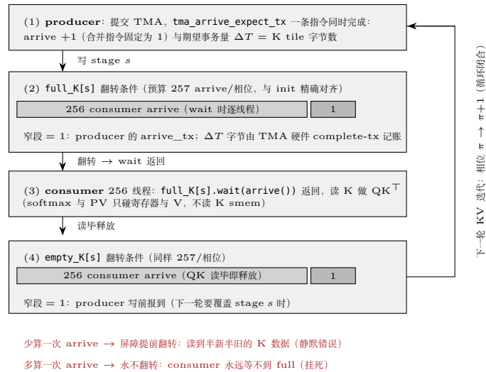
图 18.1: 固定 stage s 上 full/empty 两张屏障的相位收支循环 (式 18.5 与式 18.6 的图形化)。每轮 KV 迭代: producer 提交 TMA 时用 tma_arrive_expect_tx 一条指令完成「arrive +1」与「声明 \Delta T 」两件事, TMA 硬件搬完后自动 complete-tx 记账; consumer 256 线程在 full_K[s].wait() 时各贡献一份 arrive (256 + 1 + tx 构成翻转条件), 读毕 K 再各 arrive 一次释放 empty_K[s] , producer 下一轮写前补上第 257 份。两边的 arrive 预算都是 257/轮, 与 init 值精确对齐——多算一次挂死、少算一次静默错。窄段为可读放大, 实际只占 1/257。
