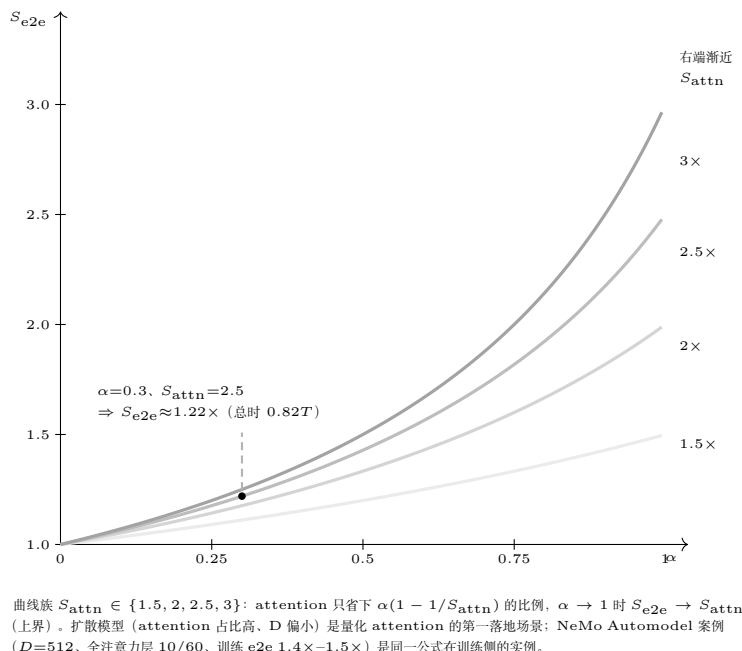
图 35.2：端到端摊销曲线族（式 35.3）：单算子 S_{\text{attn}} 换算到管线收益由 attention 占比 \alpha 封顶。 \alpha=0.3 、 S_{\text{attn}}=2.5\times 时只剩 1.22x； \alpha \rightarrow 1 的渐近线即 S_{\text{attn}} 。
