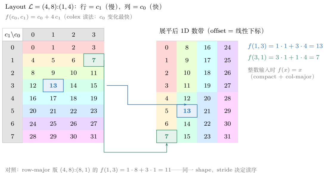
图 21.3: colex 线性化: 坐标 (c_0, c_1) 与 offset 的对应表 (左), 同一布局展开后的 1D 数带 (右)。 c_0 沿行方向变化最快, 故 \text{idx} = c_0 + 4c_1 ; 整数输入时 CuTe 用式 (21.2) 先把 x 分解回坐标。compact 且 col-major 时 f(x) = x (本章测试 128 点核对)。对照 row-major 版 (4, 8):(8, 1) : f(1, 3) = 11 ——同一 shape, stride 决定读序。
