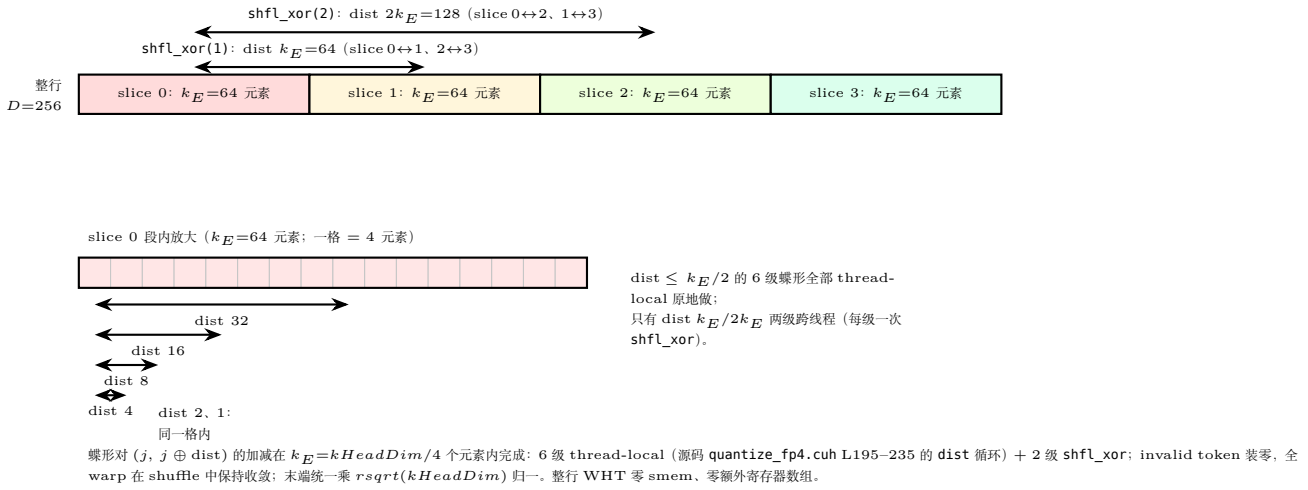
图 33.4: fused WHT 的蝶形距离分层 ( D=256 , 4 线程一 token、每线程 k_E=64 连续元素)。距离 < k_E 的 6 级蝶形全在 thread-local 数组内; dist k_E 与 2k_E 两级各用一次 shfl_xor(1)/shfl_xor(2) 跨 slice 交换——零 smem、零额外寄存器数组。
