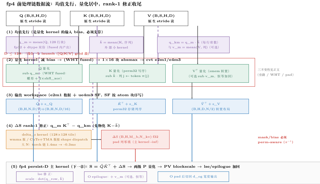
图 33.6: fp4 前处理链数据流 ( D \leq 128 走 fused 单 launch 路径): \bar{k}/q_m 均值先行的原因是它们是量化 kernel 的输入 bias; hadamard 下 q_m^{rot} 在 fused kernel 内顺带产出。
