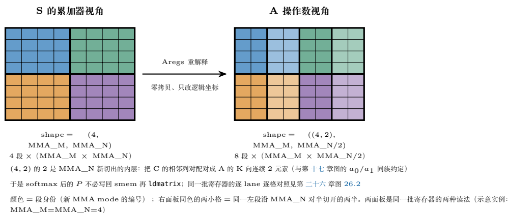
图 20.3: 零拷贝的寄存器重解释 (19.4.3 节 quote 块中 convert_layout_acc_Aregs (L300–305) 的模式级示意)。左: S 的累加器 layout 是 (MMA=4, MMA\_M, MMA\_N) ——4 个 MMA 重复段, 每段 MMA\_M \times MMA\_N ; 右: 同一批寄存器被读成 ((4, 2), MMA\_M, MMA\_N/2) ——沿 MMA\_N 切一刀得到 (2, MMA\_N/2) , 切出的 2 与原来的 4 配对成新的 8 段 MMA mode, 正是 PV 的 A 操作数所需的「K 向连续 2 元素」(与第 十七 章旗舰图的 a_0/a_1 配对同族)。数据一个比特都没动: 只是坐标重排, softmax 后的 P 因此不需要写回 smem 再 ldmatrix 。
