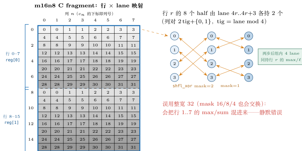
图 17.2: m16n8 C fragment 的行 × lane 映射与 warp_reduce<4> 的宽度依据 (源码注释 L458-474 的图形化)。左: 行 r 与 r+8 的 8 个列元素同由 lane 4r..4r+3 持有 ( \text{tig} = 0..3 各一对), 行 0-7 走 reg[0] 、行 8-15 走 reg[1] ; 右: 组内两步 XOR 蝶形 ( \text{mask } 2 \rightarrow \text{mask } 1 ) 后 4 个 lane 同持该行归约值。若误用整宽 32, \text{mask } 16/8/4 的交换会把别的行的值混进来——这是 3c 步最典型的静默错误。
