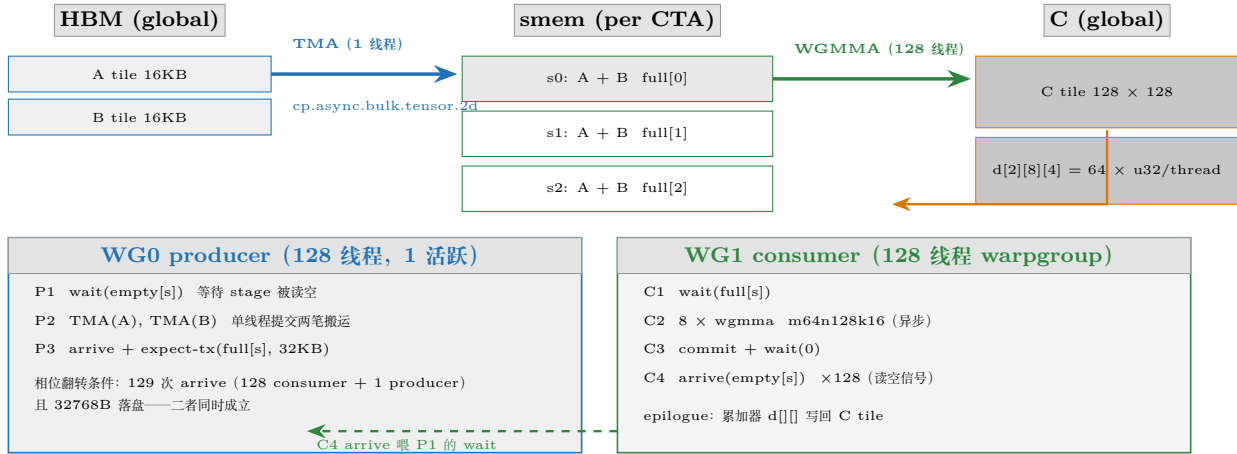
图 14.5: producer/consumer 双 warp group 数据流: TMA 单线程提交搬运, WGMMA 全 warp group 计算, full[]/empty[] 双屏障阵列按 stage 解耦两支执行流, kStages=3 使计算与搬运最多重叠 2 个 tile。
