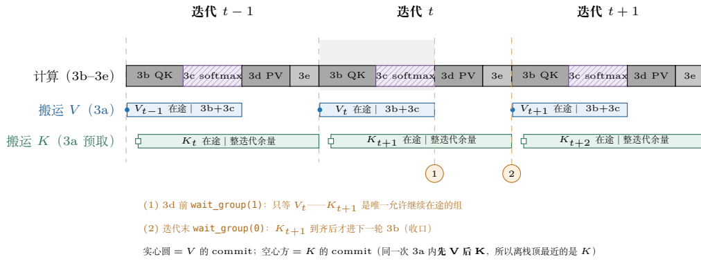
图 17.4: K 双缓冲、V 单级的流水时序 (16.4.5 节 3a 步, 源码 L273-340 与 L563-569、L710-714 的图形化)。三个稳态迭代 t-1/t/t+1 : 每个迭代内 3a 依次提交两组搬运—— V_t (实心圆, 写当前 V buffer) 与 K_{t+1} (空心方, 写 smem_sel_next )。 V_t 的在途窗口 (蓝条) 恰好覆盖同迭代的 3b (QK mma) 与 3c (softmax)——softmax 全在 CUDA Core/SFU 上跑, 正好填掉 V 的搬运延迟; K_{t+1} 则有整整一个迭代的余量。两处等待: (1) 3d 前的 wait_group(1) 只等 V_t , 把 K_{t+1} 留在途; (2) 迭代末 (3e 之后) 的 wait_group(0) 收口 K_{t+1} 才进下一轮 3b。与第 12 章 GEMM 的「kStages 全操作数统一多级」不同——attention 两段 mma 之间夹着一段非 mma 计算, 天然提供了第二级的隐藏窗口, 所以 kStagesK=2 就够 (源码注释 L281 「one stage is enough for V」)。
