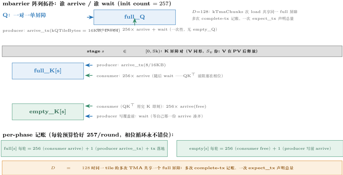
图 18.4: 本章 kernel 的 mbarrier 阵列拓扑: Q 一对一单屏障、K/V 各 S_k/S_v 对 full/empty 屏障, 全部 init 257。D = 128 时同一 tile 的多次 TMA 共享一个 full 屏障 (多次 complete-tx 记账、一次 expect_tx 声明总量)。
