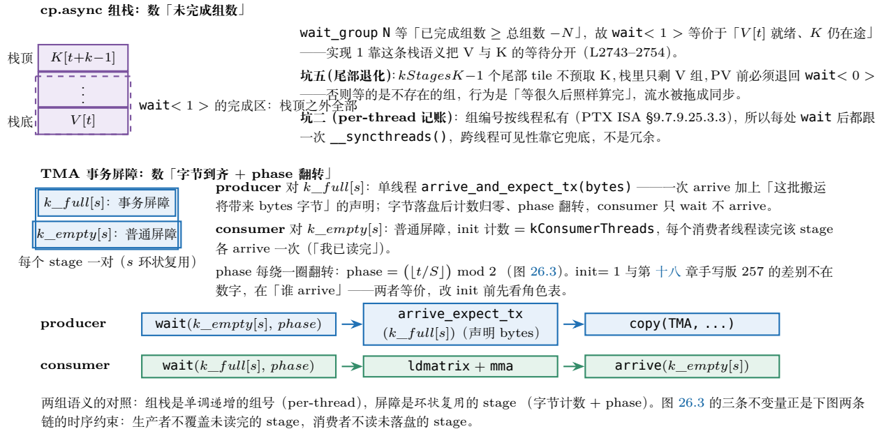
图 26.4: 两种异步等待语义的时间线对照 (flash_attn.cuh L2743–2754 与 ffpa_attn.cuh 的 TMA 版)。上: cp.async 组栈——提交顺序 V[t] (栈底) \rightarrow K[t+k-1] (栈顶), \text{wait} < 1 > 停在「除栈顶 K 之外全部完成」, 尾部 k\text{Stages}K-1 个 tile 必须退回 \text{wait} < 0 > (坑五); 每处 \text{wait} 后跟一次 __syncthreads() (坑二: 组计数按线程私有)。中下: TMA 的事务计数——每个 stage 一对 k\_full[s] (事务屏障, producer 单线程 arrive_and_expect_tx ) 与 k\_empty[s] (普通屏障, init = kConsumerThreads ), \text{phase} 由 [t/S] \bmod 2 现算; 最下一行是两条流水链的时序。
