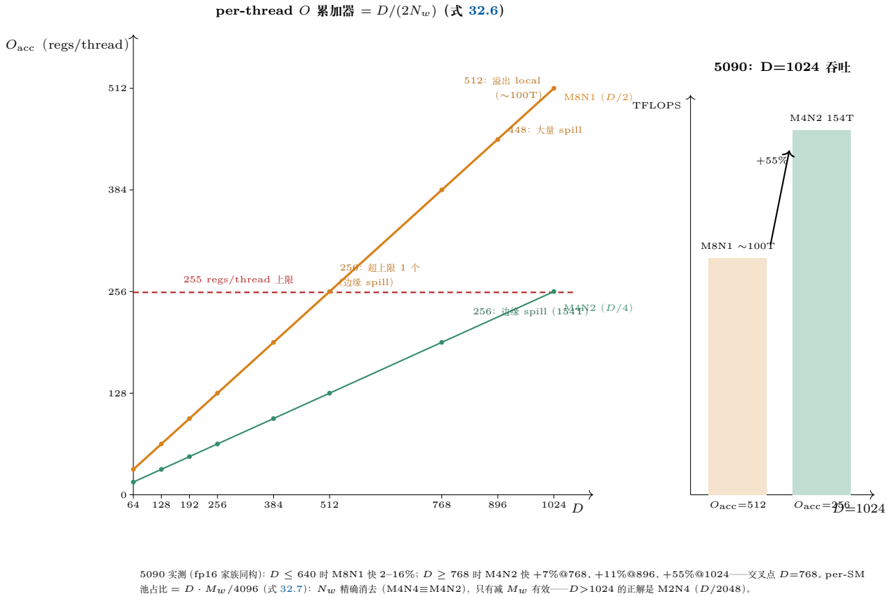
图 32.2: 寄存器墙的定量视图。左: per-thread O 累加器 = D/(2N_w) (式 32.6) ——M8N1 的 D/2 在 D=512 达 256 (超 255 上限 1 个, 边缘 spill)、 D \geq 896 大量 spill、 D=1024 溢出 local memory (~100T); M4N2 的 D/4 同点仅 256 (154T)。右: 5090 实测 D=1024 吞吐对比 (+55%)。下: per-SM 池占比 D \cdot M_w / 4096 (式 32.7) 中 N_w 精确消去——加 N-warp 不降总量, D > 1024 只能走 M2N4。
