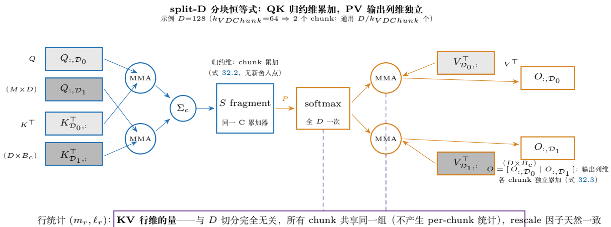
图 32.1: split-D 分块恒等式的数据流 (30.3.1 节)。QK 侧: D 是归约维, 各 chunk 的 Q_{:,D_c} K_{D_c,:}^\top 累加进同一个 S fragment (式 32.2, f32/s32 累加, 不引入新舍入点); PV 侧: D 是输出列维, 各 chunk 独立累加出 O_{:,D_c} 列段 (式 32.3), 无任何合并。softmax 的行统计 ( m_r, \ell_r ) 是 KV 行维的量——与 D 切分完全无关, 所有 chunk 共享同一组 (灰色 = chunk 身份, 两图同语义)。
