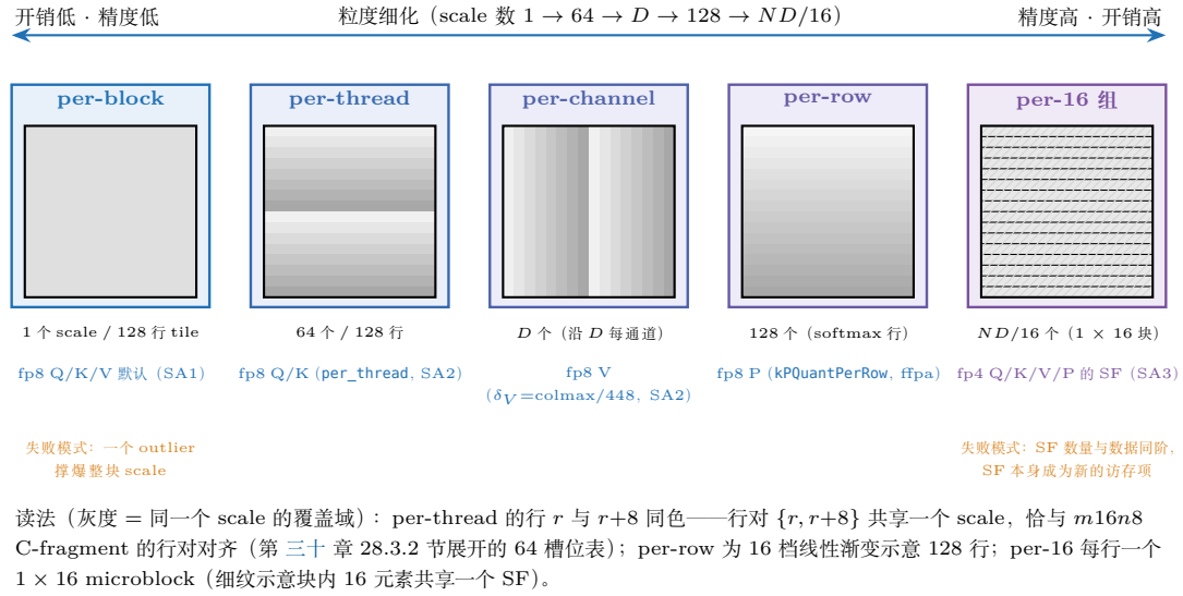
图 29.1: 量化粒度谱系五联网络 (表 29.2 的可视化, 缩略网格为 16 行 \times 16 列)。从左到右: per-block 整块共享 1 个 scale; per-thread 按 C-fragment 行对 \{r, r+8\} 分档 (128 行块共 8 \times 8 = 64 个, 零 shuffle 消费); per-channel 沿 D 每通道一个; per-row 每 softmax 行一个 (128 个); per-16 每行一个 1 \times 16 microblock (NVFP4 的 SF)。顶部双向轴是整条谱系的 trade-off: 粒度越细精度越高, 但 scale 的存储、传递与消去开销同步上涨, 且必须与 MMA 的 fragment 布局对齐——谱系两端的失败模式分别是对 outlier 的脆弱性与 SF 自身的访存账。
