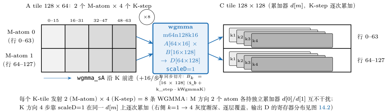
图 14.1: 一个 K-tile 的 8 条 WGMMA 拼出 C tile (hgemm.cuh L1744–1761 的 C2 双层循环): A tile 128 \times 64 按 M 方向切 2 个 64 行 M-atom、K 方向切 4 个 kWgmmaK=16 的 K-step，对每个 (M-atom, K-step) 发射一条 wgmma.m64n128k16 ——A 指针 wgmma_sA 沿 K 每步前进 16 (本 kernel 即 m 循环 \times k\_step 循环)，B 从 s_b 同步切 [16 \times 128] 片；4 次 K-step 靠 scaleD=1 在同一累加器 d[m] 上逐次累加 (C tile 内 k=1 \rightarrow 4 灰度渐深)，2 个 M-atom 各持独立累加器 d[0]/d[1] 。
