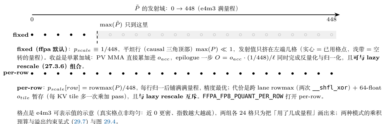
图 29.2: fixed 与 per-row 两种 p_{scale} 策略的发射域利用率 (27.3.5 节)。上: fixed 的 p_{scale} \equiv 1/448 是编译期常数, 平坦行的 \max(P) \ll 1 使发射值只占量程左端一小段, 其余量程空转——换来的是单累加域与「可与 lazy rescale 组合」; 下: per-row 用 \text{rowmax}(P)/448 把每一行拉满, 精度最优, 代价是跨 lane rowmax 归约与 64-float 的 o_{tile} 暂存, 且与 lazy rescale 互斥。
