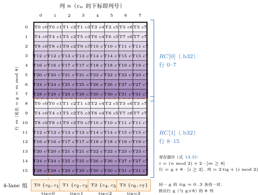
图 12.3: C fragment ( m16 \times n8 ) 寄存器布局——hgemm.cuh L311-333 字符画的 TikZ 版, 与式 12.3 逐格一致: 行 m = g = \text{lane} \gg 2 (底色 8 档, 行 0-7 与 8-15 由同批 lane 重复覆盖), 列对由 \text{tig} = \text{lane} \% 4 决定; RC[0] 装行 0-7、RC[1] 装行 8-15。底部: 4-lane 组内 \text{tig} = 0..3 各持一对 \{c_{2t}, c_{2t+1}\} , 拼齐一行 8 个 half——11.4.6 节 epilogue shuffle 的出发点。
