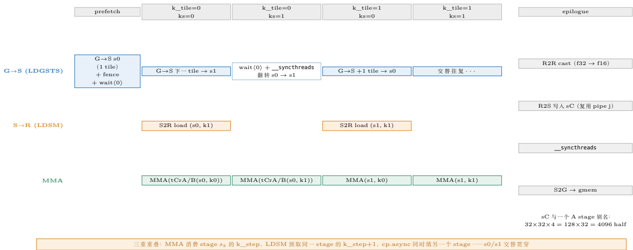
图 25.4: CuTe HGEMM 的 k_{\text{stage}} = 2 流水时序（含寄存器双缓冲）。上：G→S（LDGSTS）；中：S→R（LDSM）；下：MMA。MMA 消费 stage s_k 的 k_{\text{step}} 时，LDSM 预取同一 stage 的 k_{\text{step}}+1 ，cp.async 同时填另一个 stage——三重重叠；左端 prefetch 一个 tile，右端 epilogue（ R2R \rightarrow R2S \rightarrow S2G ，sC 与一个 A stage 别名： 32 \times 32 \times 4 = 128 \times 32 = 4096 half）。
