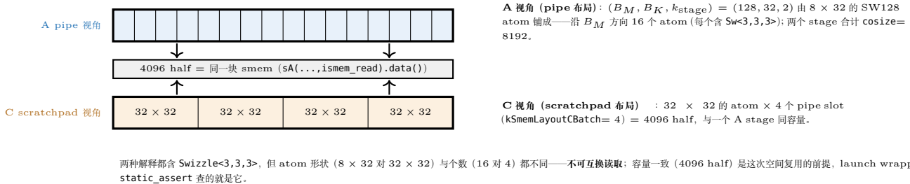
图 22.4: epilogue scratchpad: 同一块 4096 half 的 smem、两种布局视图 (hgemm.cuh L1001)。上条带是 A 的 pipe 解释——(128,32) 的 stage 按 8 \times 32 的 SW128 atom 沿 B_M 切成 16 段；下条带是 C 的 scratchpad 解释—— 32 \times 32 的 atom \times 4 个 pipe slot ( kSmemLayoutCBatch=4 )。中间那条带是两者共用的地址带： sC 拿到的只是 sA(_,_,ismem_read).data() 这个裸指针，没有 Tensor 类型转换，重复的只是「同一段地址的两种读法」。
