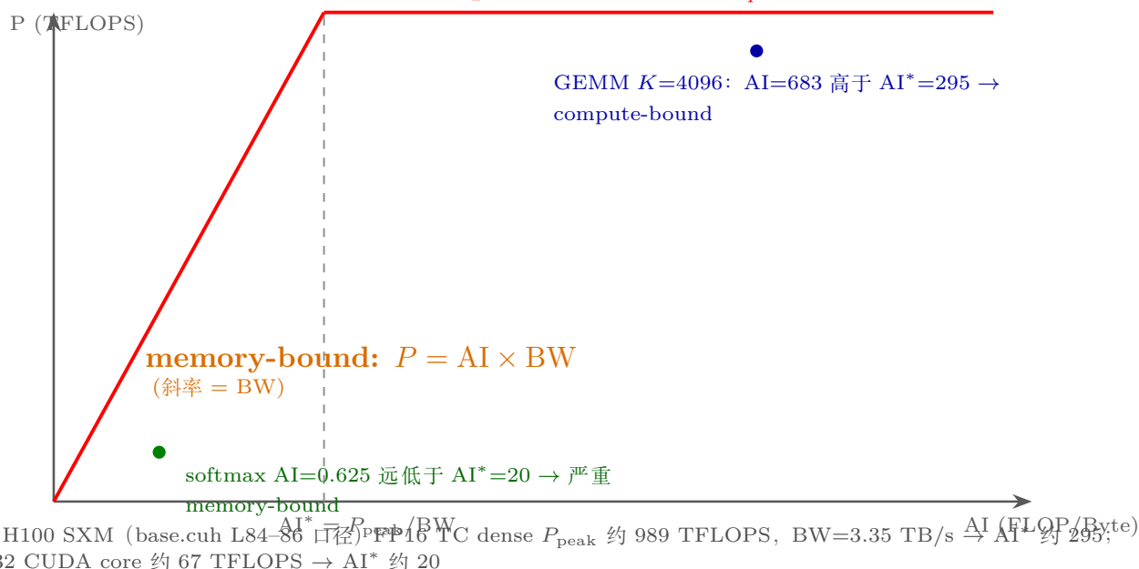
图 2.3: Roofline 模型: P = \min(P_{\text{peak}}, AI \times BW) , 脊点 AI^* = P_{\text{peak}}/BW 。GEMM K=4096 (AI= 683) 落在计算屋顶, softmax (AI= 0.625) 落在带宽斜线区。
