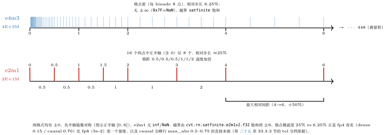
图 33.1: e2m1 vs e4m3 的格点数轴 (同一 [0, 6] 区间)。上: e4m3 每个 binade 8 个格点、相对步长 6.25%，满量程 \pm 448 ；下: e2m1 正半轴全部格点仅 \{0, 0.5, 1, 1.5, 2, 3, 4, 6\} 、相对步长约 25%，[4, 6] 段相对间距最大 (+50%)。fp4 的容差天然比 fp8 宽一个量级的格式层根源。
