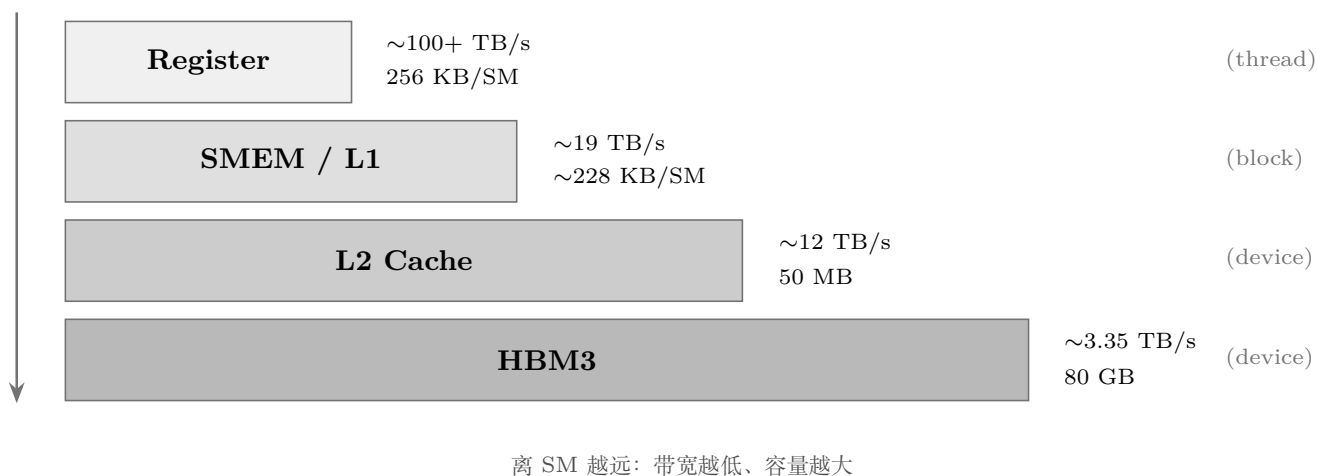
图 2.2: GPU 内存层级金字塔: 离 SM 越远带宽越低、容量越大 (H100 数量级, base.cuh L16–21 口径)。
