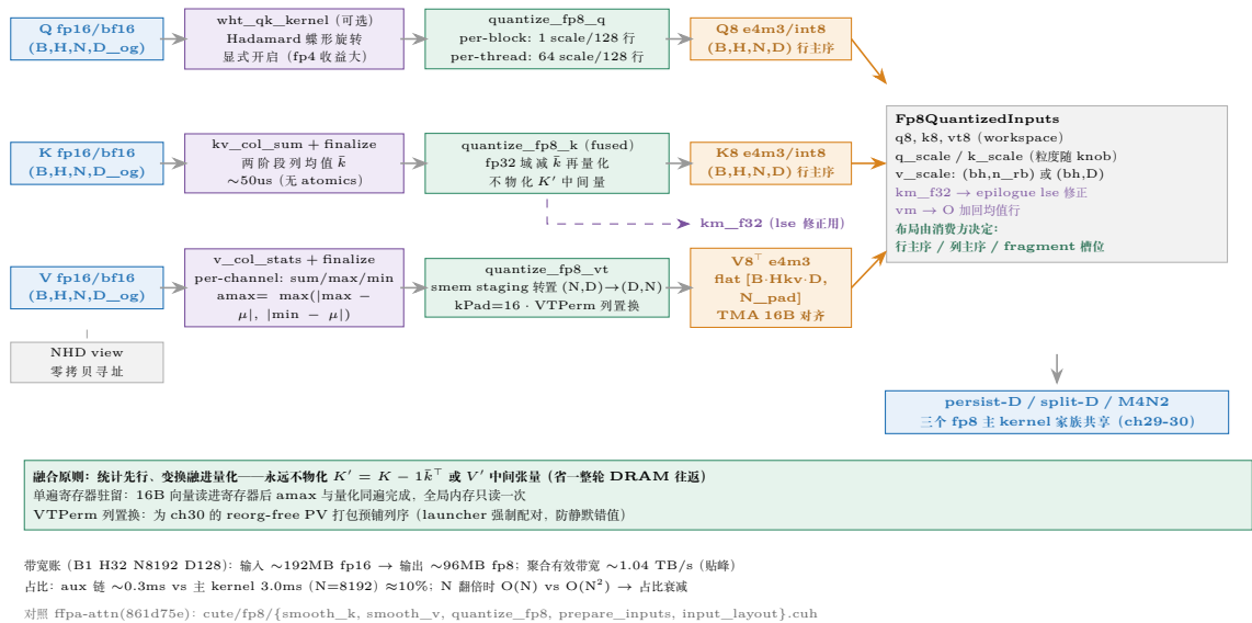
图 30.5: fp8 前处理链全景: 三泳道 (Q/K/V) 各自的统计 \rightarrow 变换 \rightarrow 量化 kernel 与输出 workspace 布局。smoothing 与量化融合在同一 kernel 内 (无中间落盘); V^T 的列 pad 兼顾 TMA 16B 对齐与置换写。
