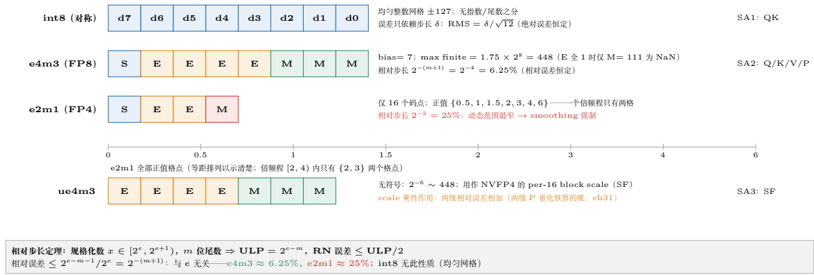
图 29.5: 四种量化格式的位域与值域对照 (int8 / e4m3 / e2m1 / ue4m3)。e4m3 的指数全 1 时仅 M=111 编码 NaN, 故满量程 448; e2m1 全部 16 个码点在数轴上标出, 直观呈现「一个倍频程内只有两格」。
