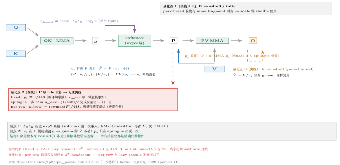
图 29.6: attention 的三个量化点与 scale 流向: \delta_Q \delta_K 折进 exp2 系数 (式 29.4)、 v_s 在 P 侧精确消去 (式 29.5)、 p_{scale} 在 epilogue 一步收尾。
