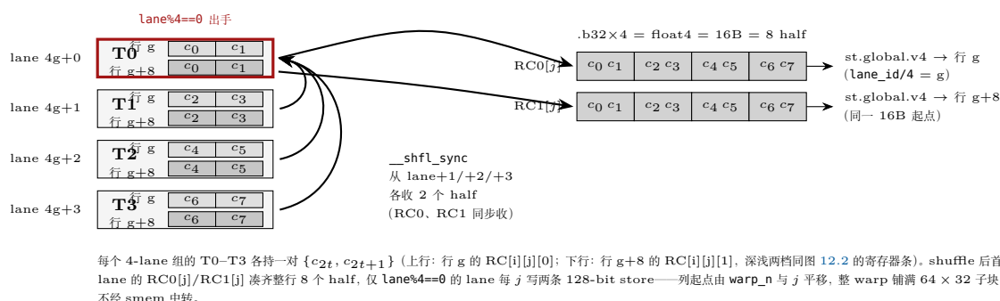
图 12.7: Epilogue shuffle 收拢与写回 (hgemm.cuh L336-382): 4-lane 组内 T0-T3 各持一对 \{c_{2t}, c_{2t+1}\} (上行 = 行 g , 下行 = 行 g+8 的寄存器对), _shfl_sync 从 \text{lane}+1/+2/+3 各收 2 个 half, 把 \text{RC0}[j] (行 g ) 与 \text{RC1}[j] (行 g+8 ) 各凑成 4 条 .b32 = 一条 16B float4; 随后仅 \text{lane}\%4==0 的 lane 出手, 行号 = \text{lane\_id}/4 = g , 两条 128-bit store 分别写行 g 与 g+8 。
