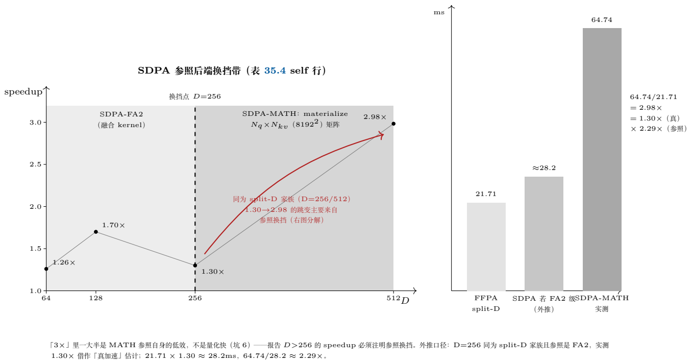
图 35.1: 参照系视角看表 35.4 的 self 行。左: SDPA 参照随 D 换挡——FA2 只覆盖 D \leq 256 , 更大 D 静默落到 MATH (materialize N_q \times N_{kv} 矩阵); 四个 speedup 点 (1.26/1.70/1.30/2.98×) 落在换挡带上, D=512 的跳变与 kernel 无关。右: D=512 的 2.98× 归因——以 D=256 同家族 (split-D、FA2 参照) 实测 1.30× 为真加速估计, MATH 参照自身再慢 \times 2.29 : 「3×」的大头是参照低效 (坑 6)。
