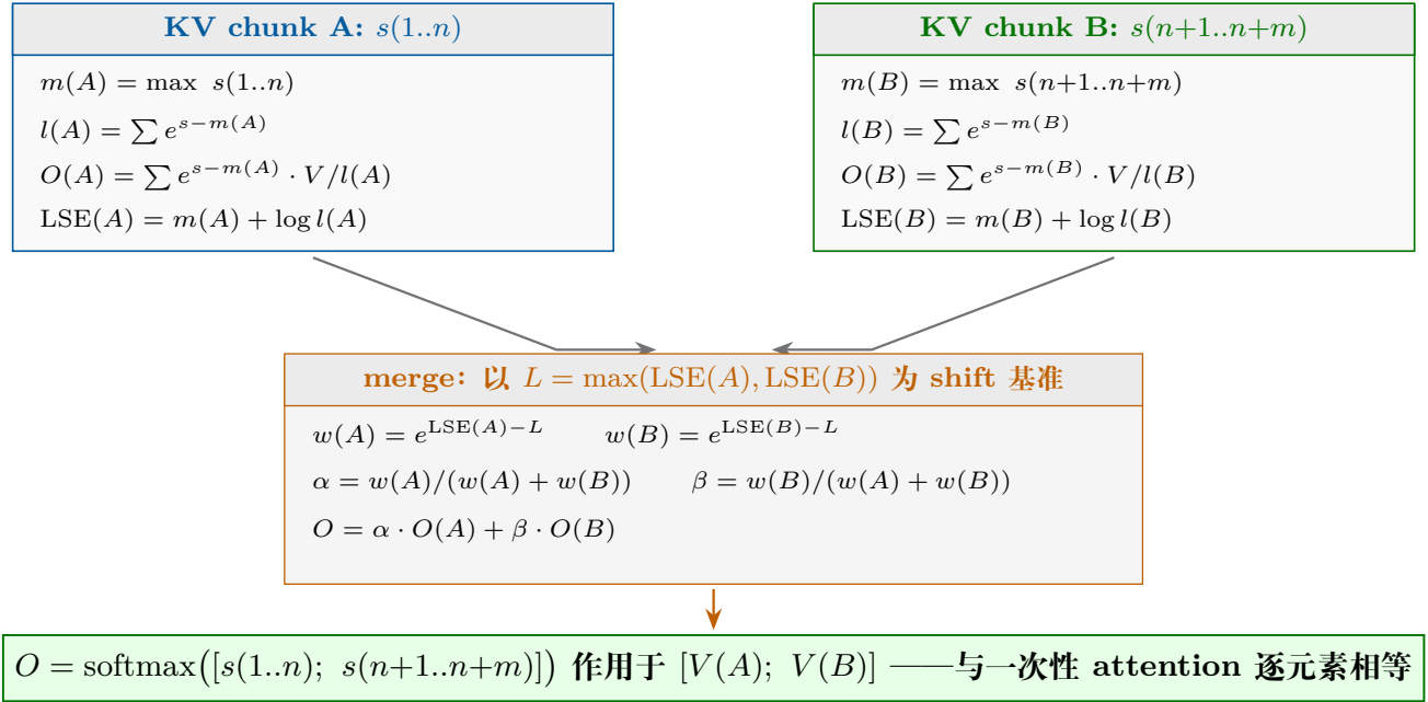
图 6.3: 两个分块 attention 状态的合并: 块内各自输出 (已归一化 O 与单标量 \text{LSE} ), 块间以 L = \max(\text{LSE}) 为 shift 基准计算凸组合系数 \alpha, \beta , 合并结果与整体 softmax 直接加权逐元素相等 (定理 6.2)。
