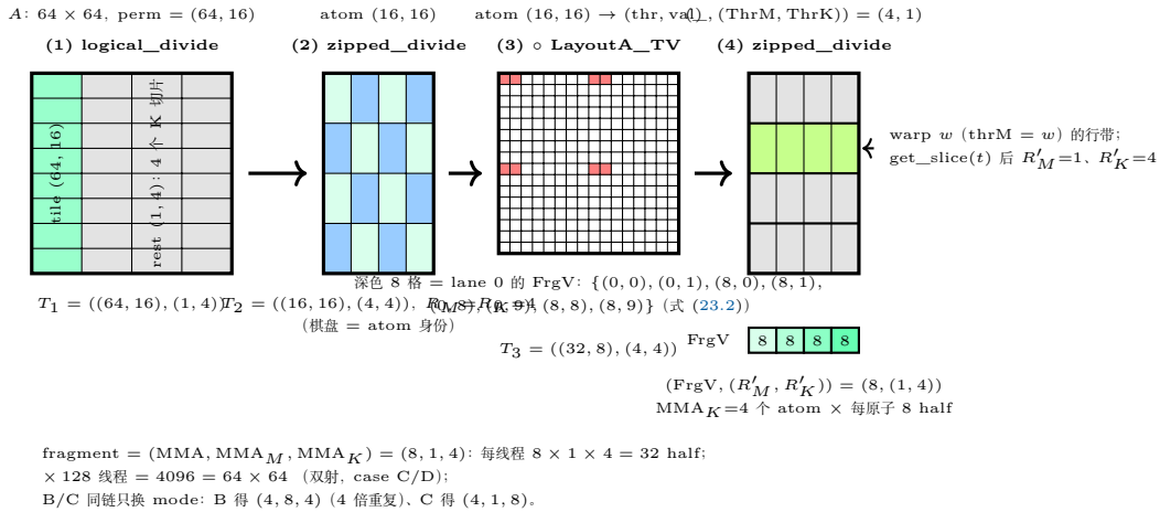
图 23.1: thrfrg_A 四步推导链 (式 (23.7)–(23.10)) 在 FFPA QK (tile 64 \times 64 \times 16 、AtomLayout (4, 1, 1)、Q 为 64 \times 64 ) 上的 shape 演化: (1) logical_divide 按 tile 切出 (64, 16) 与 4 个 K 切片; (2) zipped_divide 按 atom (16, 16) 切成 4 \times 4 个原子块; (3) 复合 LayoutA_TV 把原子内坐标换成 (线程, 值), 深色 8 格即 lane 0 的 FrgV; (4) 按 (ThrM, ThrK) = (4, 1) 剥出 warp 行带, get_slice( t ) 后每线程 fragment = (8, (1, 4)) = 32 half (右下: FrgV = 8 \times \text{MMA}_K = 4 )。
