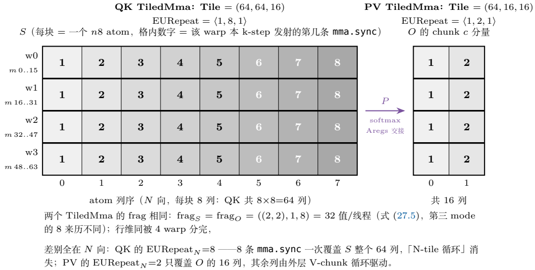
图 27.1: 双 TiledMma 的 Tile 分工 ( ffpa_attn_.cu L52–58, 式 (27.2)–(27.3))。左: QK 的输出 S[64, 64] ——4 个 warp 各占 16 行 ( \text{AtomLayout} 的 M 分量 4), 列向 8 个 n8 atom 由同一线程在一个 k-step 里连发 8 条 mma.sync 覆盖 (灰度 8 档标识 atom 身份, 格内数字为发射序); 右: PV 的输出 O 只有一个 chunk 分量 [64, 16] (2 个 atom、2 条 mma.sync )。中间箭头是 26.3.3 节的交接: S 经 softmax 与 Aregs 零拷贝重解释成 P , 作为 PV 的 A 操作数——共享的正是左侧那批 S 寄存器。
