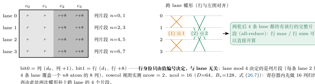
图 26.1: convert_layout_acc_rowcol 的两层拆解 (式 (26.6)–(26.7))。左: quad 内 4 条 lane 的 4 个寄存器 c_0..c_3 —— 两档灰度标出「行身份」: c_0, c_1 属行 r 、 c_2, c_3 属行 r+8 ; 右侧标出该 lane 覆盖的列片段 (由 \text{lane} \bmod 4 决定)。值编号的 bit0 是列偏移、bit1 是行 +8, 所以同一行的 8 列散落在 quad 的 4 条 lane 上。右: 两次 __shfl_xor_sync 的蝶形——第一轮并 (0,1) 与 (2,3) (步长 1), 第二轮并 (0,2) 与 (1,3) (步长 2), 两轮后每条 lane 都持有该行的完整片段, 行 max / 行 sum 可以就地开算。
