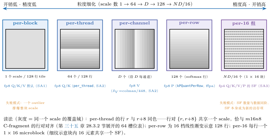
图 34.1: 量化粒度谱系五联网格 (表 34.2 的可视化, 缩略网格为 16 行 \times 16 列)。从左到右: per-block 整块共享 1 个 scale; per-thread 按 C-fragment 行对 \{r, r+8\} 分档 (128 行块共 8 \times 8 = 64 个, 零 shuffle 消费); per-channel 沿 D 每通道一个; per-row 每 softmax 行一个 (128 个); per-16 每行一个 1 \times 16 microblock (NVFP4 的 SF)。顶部双向轴是整条谱系的 trade-off: 粒度越细精度越高, 但 scale 的存储、传递与消去开销同步上涨, 且必须与 MMA 的 fragment 布局对齐——谱系两端的失败模式分别是对 outlier 的脆弱性与 SF 自身的访存账。
