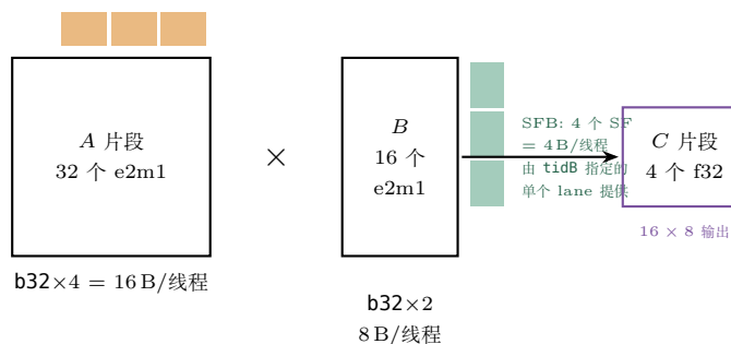
图 33.2: SM120_16x8x64_TN_VS 一条指令的操作数账。数据侧共 16 + 8 = 24 B/线程, SF 侧 8 B/线程——SF 的字节数达到数据的 1/3。注意 SF 的「字节数/线程」与「SF 数/线程」是一回事 (ue4m3 是 1 字节), 但哪些 lane 的字节作数由指令的 tidA/tidB 选择器决定, 这就是 SF 的寄存器 fragment 必须由 CuTe 的 partition_fragment_sfa 从权威布局推导、而不能手写的原因。
