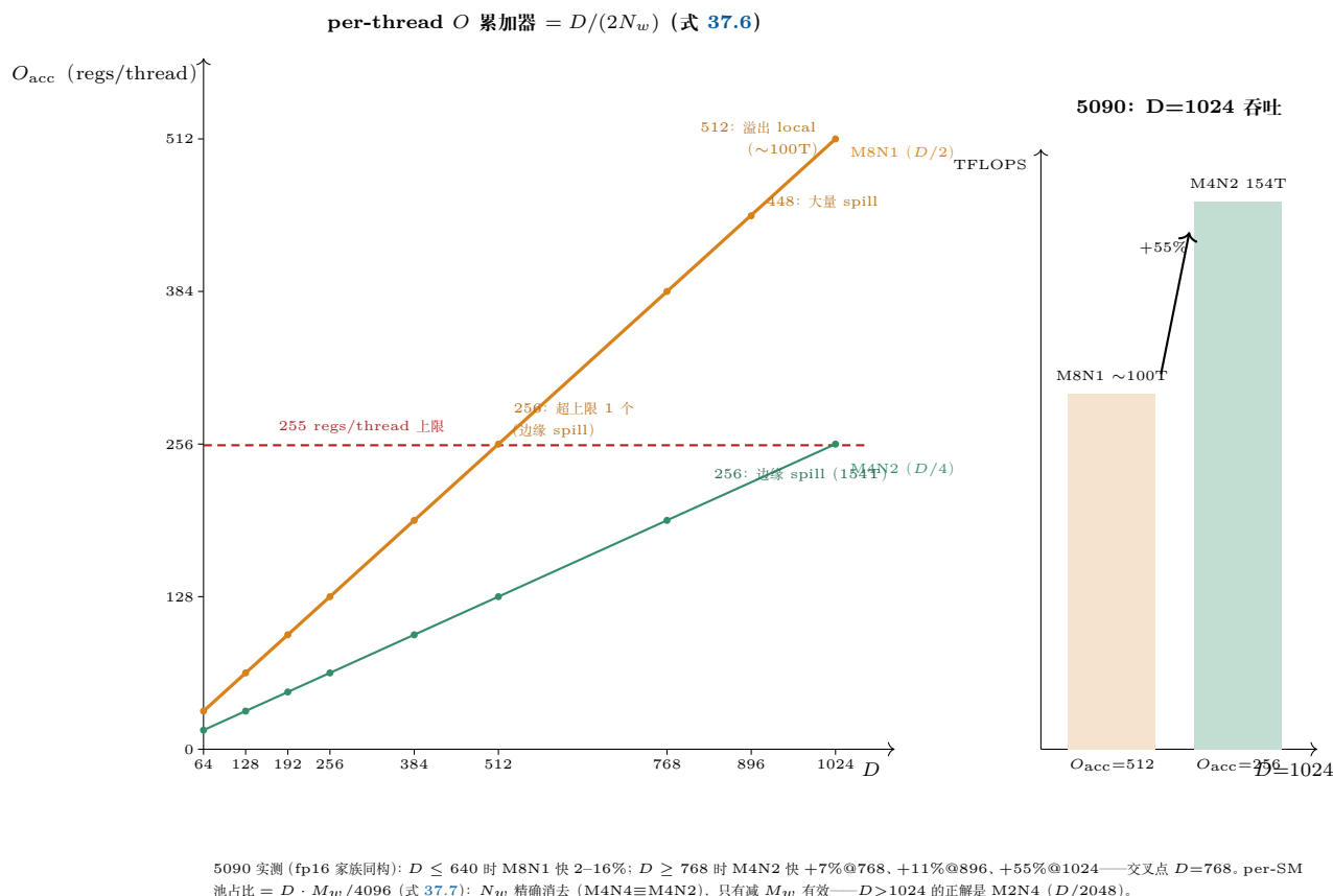
图 37.2: 寄存器墙的定量视图。左: per-thread O 累加器 = D/(2N_w) (式 37.6) —— M8N1 的 D/2 在 D=512 达 256 (超 255 上限 1 个, 边缘 spill)、 D \geq 896 大量 spill、 D=1024 溢出 local memory (~100T); M4N2 的 D/4 同点仅 256 (154T)。右: 5090 实测 D=1024 吞吐对比 (+55%)。下: per-SM 池占比 D \cdot M_w / 4096 (式 37.7) 中 N_w 精确消去——加 N-warp 不降总量, D > 1024 只能走 M2N4。
