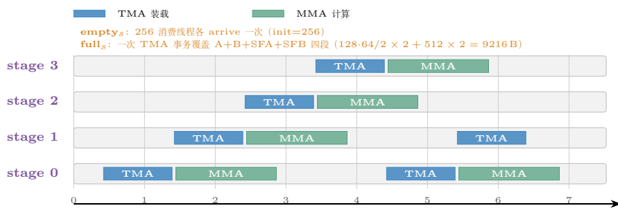
图 33.4: 四级流水的时序示意 (BN 取 128 的默认档；本卡 k_{Stages} 可用到 8~10 级，见 33.9.4 节扫描表)。与第三十一章图 31.2 的结构差别在 MMA 块的宽度：FP4 的一个 stage 只有一跳原子 (BK=64)，K 方向不再有内层循环，MMA 块相对 TMA 块更窄——这意味着流水线对 TMA 延迟的容忍度更低，是 BN 翻倍的收益来源之一 (BN 翻倍 = MMA 块宽翻倍，而 TMA 字节数只涨 B 与 SFB 的部分)。
