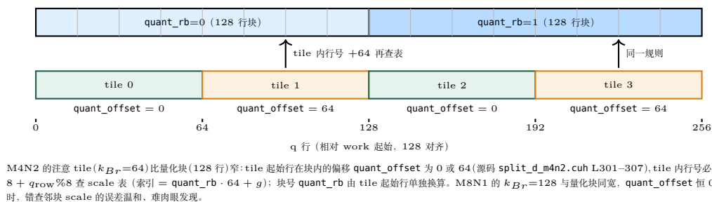
图 37.3: 量化 128 行块与 M4N2 注意 tile ( k_{Br}=64 ) 的错位对齐。tile 1/3 的起始行落在量化块内的偏移 64 处, 其行号需先加 quant_offset 再查 per-thread scale 表; tile 0/2 偏移为 0。M8N1 的 k_{Br}=128 与量化块同宽, 不存在该映射。
