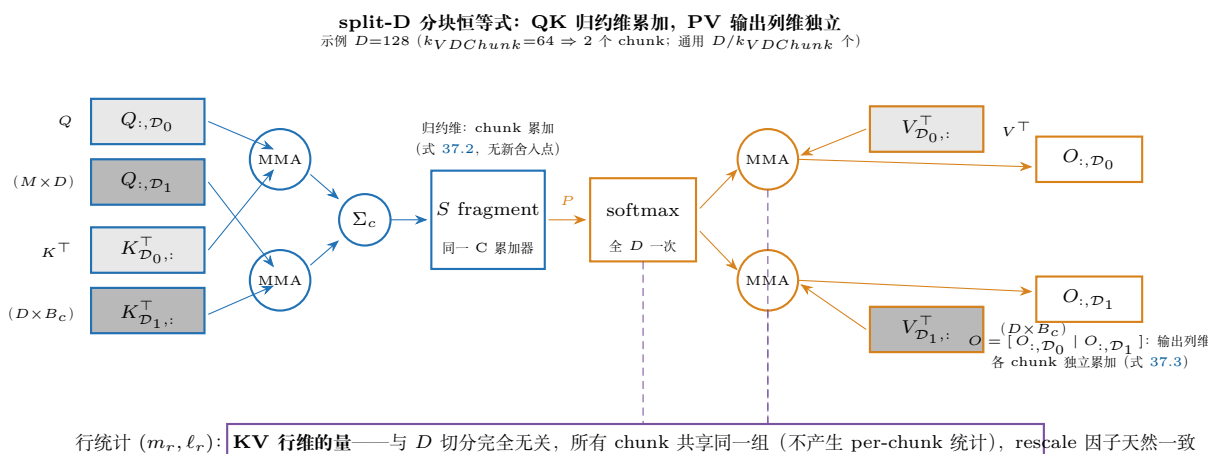
图 37.1: split-D 分块恒等式的数据流 (30.3.1 节)。QK 侧： D 是归约维，各 chunk 的 Q_{:,D_c} K_{D_c,:}^\top 累加进同一个 S fragment (式 37.2, f32/s32 累加，不引入新舍入点)；PV 侧： D 是输出列维，各 chunk 独立累加出 O_{:,D_c} 列段 (式 37.3)，无任何合并。softmax 的行统计 ( m_r, \ell_r ) 是 KV 行维的量——与 D 切分完全无关，所有 chunk 共享同一组 (灰色 = chunk 身份，两图同语义)。
