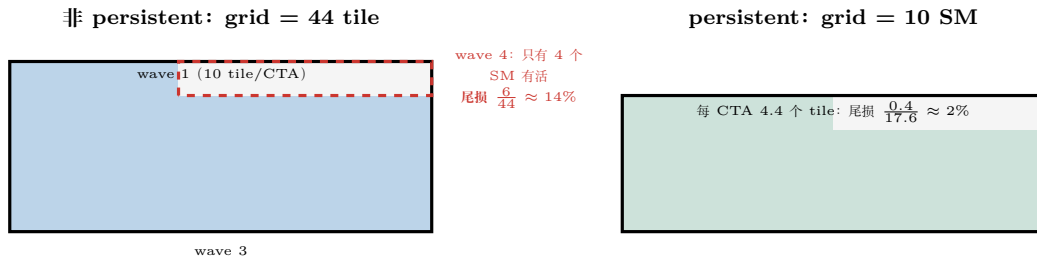
图 28.5: wave 量化尾损示意 (10 个 SM、44 个 tile 的缩小模型)。左: 非 persistent launch 按整 wave 调度, 最后一个 wave 只有 4 个 SM 在算, 其余空转满一个 tile 时长; 右: persistent CTA 把 grid 收缩到 SM 数, 每个 CTA 串行吃 \lceil 44/10 \rceil 或 \lfloor 44/10 \rfloor 个 tile, 不均衡被压缩到最后一个 tile 的零头。真实场景 (110 SM, H=32/N=8192 ) dense 收益 +2%~6%; causal 反向 ——tile 负载前轻后重, 线性分配会把重 tile 锁死在同一批 CTA 上 (实测 -9% ~ -21%), 此时必须回退全量 grid 让硬件调度器自然均衡。
