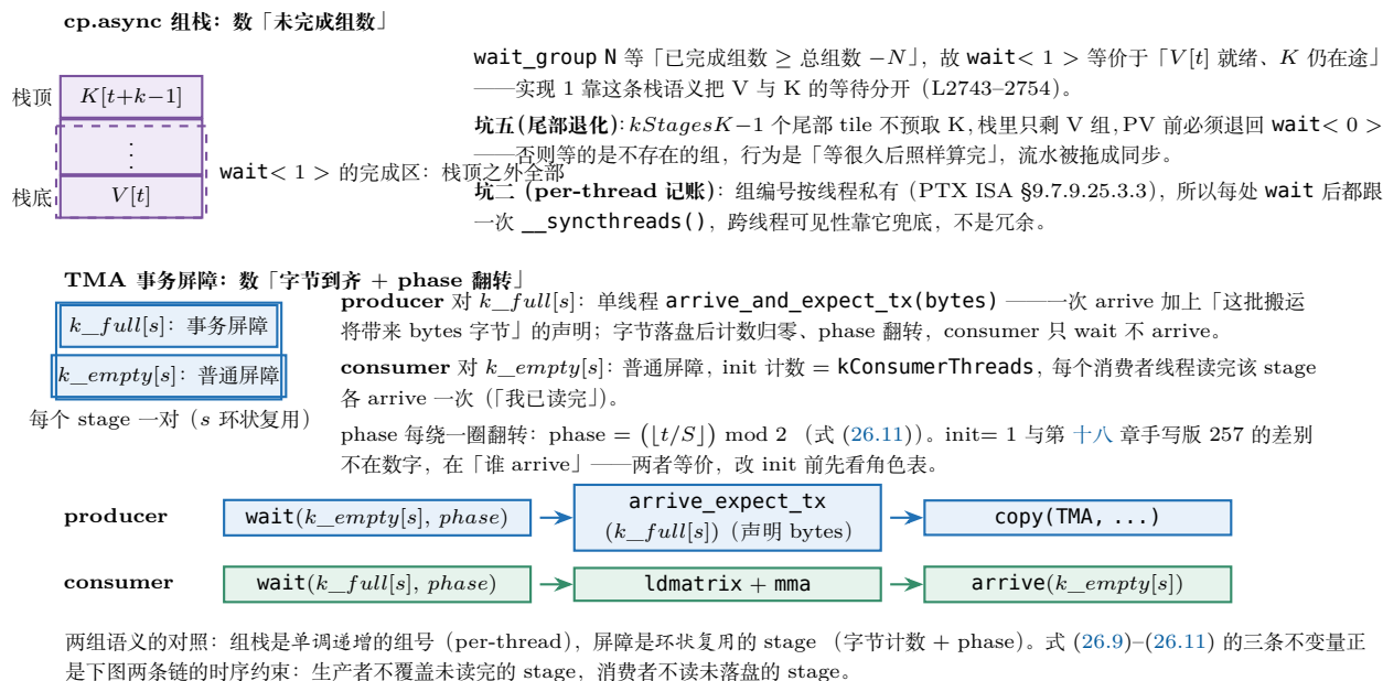
图 26.3: 两种异步等待语义的时间线对照 (flash_attn.cuh L2743–2754 与 ffpa_attn.cuh 的 TMA 版)。上: \text{cp.async} 组栈——提交顺序 V[t] (栈底) \rightarrow K[t+k-1] (栈顶)， \text{wait} < 1 > 停在「除栈顶 K 之外全部完成」，尾部 kStagesK-1 个 tile 必须退回 \text{wait} < 0 > (坑五)；每处 \text{wait} 后跟一次 \_\text{syncthreads}() (坑二：组计数按线程私有)。中下: TMA 的事务计数——每个 \text{stage} 一对 k\_full[s] (事务屏障， \text{producer} 单线程 \text{arrive\_and\_expect\_tx} ) 与 k\_empty[s] (普通屏障， \text{init} = \text{kConsumerThreads} )， \text{phase} 由 \lfloor t/S \rfloor \bmod 2 现算；最下一行是两条流水链的时序。
