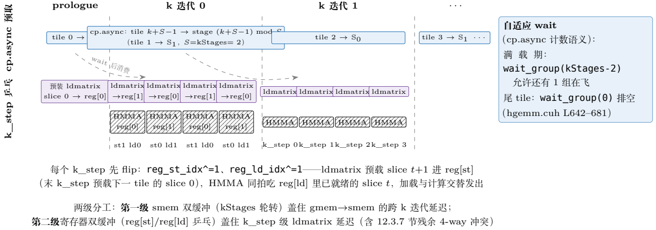
图 13.3: 两级双缓冲叠加的流水时间线 (12.4.4 节, hgemm.cuh L514-681): 上泳道是第一级——cp.async 按 stage (k+S-1) \bmod S 预取下一 K-tile ( S=kStages=2 时 k 迭代 0 预取 tile 1 进 S 1 、 迭代 1 预取 tile 2 回 S 0 )；下泳道是第二级——每个 k 迭代 内 4 个 k_step 逐个过: 先 flip ( reg_st_idx/reg_ld_idx 各异或 1)，ldmatrix 把 slice t+1 写进 reg[st] ，同拍 HMMA 吃 reg[ld] 里已就绪的 slice t ，tensor core 不必等 ldmatrix。右侧为自适应等待: 满载期 wait_group(kStages-2) 允许 1 组在飞、尾 tile 退化为 wait_group(0) 排空。
