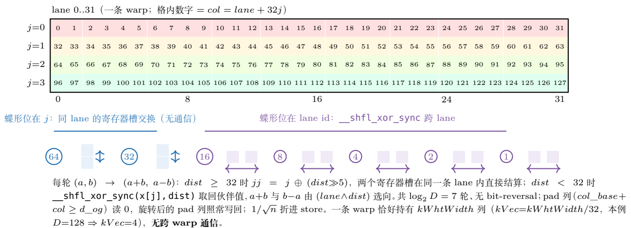
图 30.4: radix-2 蝶形的距离二分 ( hadamard.cuh L40-92, 本例 D=128 、 kWhtWidth=D )。上: 列归属—— j 是寄存器槽、lane 是 warp 内线程, 格内数字 col = lane + 32j 满足索引律, 右下角 127 = size - 1 ; 一条 warp 覆盖整行 128 列。下: 七轮的「距离阶梯」—— dist \geq 32 的 bit 落在 j 上 (同 lane 两个寄存器槽直接加减, 无通信), dist < 32 的 bit 落在 lane id 上 ( __shfl_xor_sync 跨 lane); 每轮一个 bit, 1/\sqrt{n} 折进 store。
