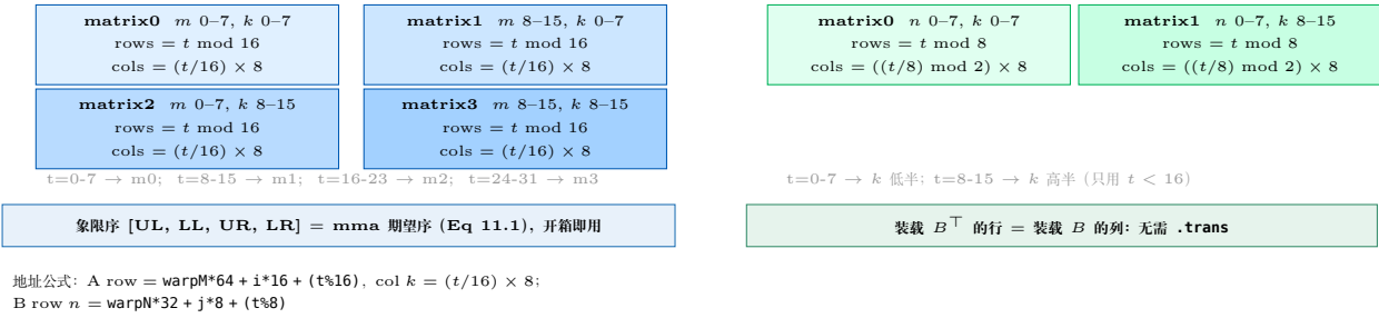
图 12.4: 本章 kernel 的 ldmatrix 寻址映射: A 用 x4 一次装载 m16 \times k16 的四象限 (象限序恰为 mma 期望序); B 用 x2 装载 k16 \times n8 (借 B^T 行主序存储, 无需.trans)。
