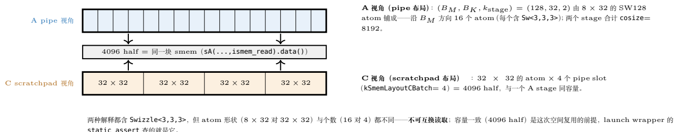
图 22.4: epilogue scratchpad：同一块 4096 half 的 smem、两种布局视图（ hgemm.cuh L1001）。上条带是 A 的 pipe 解释—— (128, 32) 的 stage 按 8 \times 32 的 SW128 atom 沿 B_M 切成 16 段；下条带是 C 的 scratchpad 解释—— 32 \times 32 的 atom \times 4 个 pipe slot（ kSmemLayoutCBatch=4 ）。中间那条带是两者共用的地址带： sC 拿到的只是 sA(_,_,ismem_read).data() 这个裸指针，没有 Tensor 类型转换，重复的只是「同一段地址的两种读法」。
