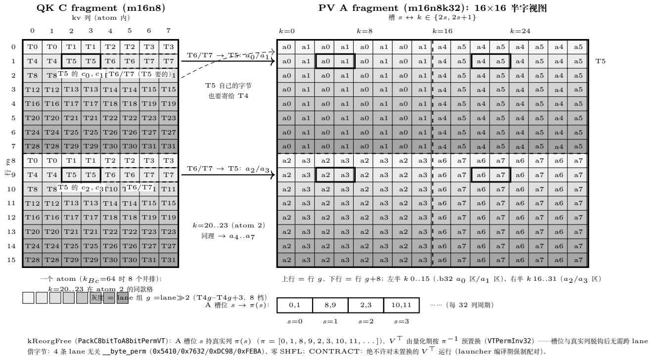
图 31.2: C→A fragment 的 lane→值映射 (lst:29-reorg-bg 的网格化)。左: QK C fragment (m16n8), 每 lane 4 值 c_0-c_3 落在行 g/g+8 的列对 \{2t, 2t+1\} ; 右: PV A fragment (m16n8k32) 的 16×16 半字视图, 格值 a_0-a_7 为 e4m3x2 半字寄存器, 四象限对应源码.b32 a_0-a_3 ; 两面板灰度同语义 (lane 组 g = \text{lane} \gg 2 , 8 档)。中: t=1 (T5) 的自然 A 需要 k \in \{4..7\} \cup \{20..23\} (行 g 与 g+8 ), 在 C 视图里属 T6/T7——纯 lane 内置换凑不齐, 即 16 SHFL + 32 PRMT (ReorgC8bitToA8bit) 的根源。下: kReorgFree 的出路——槽位持 \pi(s) 、 V^T 预置换, 4 条 lane 无关 __byte_perm、零 SHFL。
