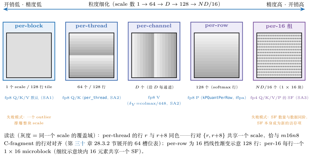
图 29.1: 量化粒度谱系五联网格 (表 29.2 的可视化, 缩略网格为 16 行 \times 16 列)。从左到右: per-block 整块共享 1 个 scale; per-thread 按 C-fragment 行对 \{r, r+8\} 分档 (128 行块共 8 \times 8 = 64 个, 零 shuffle 消费); per-channel 沿 D 每通道一个; per-row 每 softmax 行一个 (128 个); per-16 每行一个 1 \times 16 microblock (NVFP4 的 SF)。顶部双向轴是整条谱系的 trade-off: 粒度越细精度越高, 但 scale 的存储、传递与消去开销同步上涨, 且必须与 MMA 的 fragment 布局对齐——谱系两端的失败模式分别是对 outlier 的脆弱性与 SF 自身的访存账。
