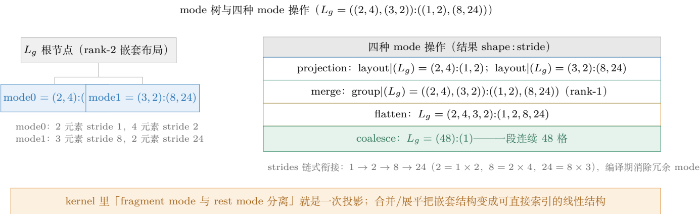
图 21.4: mode 树与四种 mode 操作的结果 (本章测试逐一核对了 shape/stride)。投影用于取子布局, 合并/展平用于把嵌套结构变成可直接索引的线性结构, 化简 (coalesce) 在编译期消除冗余 mode——kernel 里「fragment mode 与 rest mode 分离」就是一次投影。
