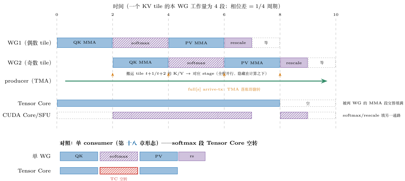
图 19.4: 双 consumer 的相位交错时序 (18.4.6 节统计性交错的图形化)。上：WG1/WG2 各按「QK MMA \rightarrow softmax \rightarrow PV MMA \rightarrow rescale」四段推进自己的 KV tile 子序列，两 WG 相位差 1/4 周期——WG1 处于 MMA 段时 WG2 大概率处于 softmax/rescale 段；producer 的 TMA 全程并行，落账即 arrive-tx 翻转 full[s] 。中：Tensor Core 与 CUDA Core/SFU 两条资源条被两路计算交替填满（同步 mma.sync 做不到 WG 内重叠，靠两路独立流在硬件调度器上统计性交错）。下：单 consumer (第 十八 章形态) 的对照——softmax 段 Tensor Core 只能空转，这正是第二个 consumer 要填的洞。
