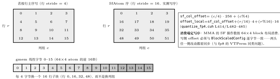
图 33.3: SF 字节的写序由消费端决定 ( V^\top 量化链)。同一 (r, c) 单元格在行主序假设下偏移 4r + c , 在 SfAtom 序下偏移 16r + c : 每 4 个列组构成 64 \times 4 的 256B atom, atom 内按 16 行子块交错。写侧 (sf_col_offset/offset_local) 与 MMA 的 BlockScaledConfig 必须逐字节一致。
