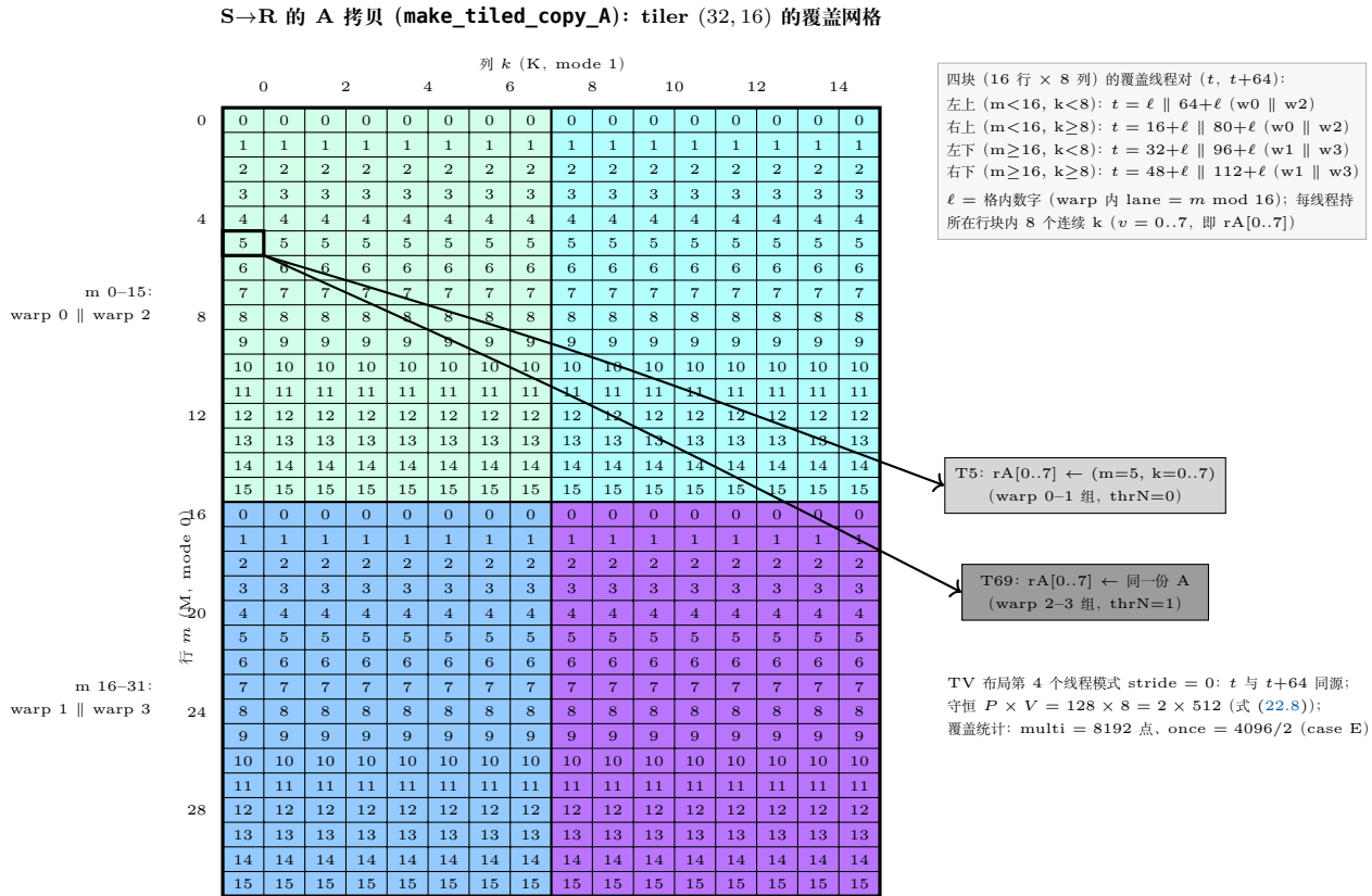
图 22.3: S→R A 拷贝的 2 倍重复因子 (式 (22.9)、测试 case D/E): tiler (32, 16) 的 A tile ( M \times K ) 上, 每格标 warp 内 lane 号 \ell = m \bmod 16 , 格子的实际覆盖线程对为 (基址 + \ell , 基址 + 64 + \ell ), 四块的基址见右上表 (w0-w3 即 warp 0-3)。每个元素恰被 2 个 (thread, value) 对覆盖: t 与 t+64 (两个 N 方向 warp, thrN = 0/1 ) 各持同一行块 8 个连续 k 的一份寄存器拷贝——TV 布局第 4 个线程模式 stride 为 0 的几何含义, 守恒 128 \times 8 = 2 \times 512 。对照图 22.5 的 G→S 双射网格 (每格恰一线程)。
