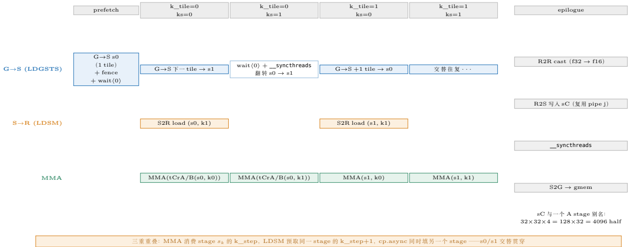
图 25.4: CuTe HGEMM 的 k_{\text{stage}} = 2 流水时序（含寄存器双缓冲）。上：G \rightarrow S (LDGSTS)；中：S \rightarrow R (LDSM)；下：MMA。MMA 消费 stage s_k 的 k_step 时，LDSM 预取同一 stage 的 k_step+1 ， cp.async 同时填另一个 stage——三重重叠；左端 prefetch 一个 tile，右端 epilogue ( R2R \rightarrow R2S \rightarrow S2G ， sC 与一个 A stage 别名： 32 \times 32 \times 4 = 128 \times 32 = 4096 half)。
