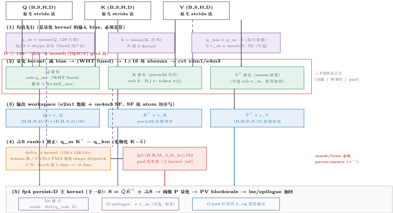
图 33.6: fp4 前处理链数据流 ( D \leq 128 走 fused 单 launch 路径): \bar{k}/q_m 均值先行的原因是它们是量化 kernel 的输入 bias; hadamard 下 q_m^{rot} 在 fused kernel 内顺带产出。
