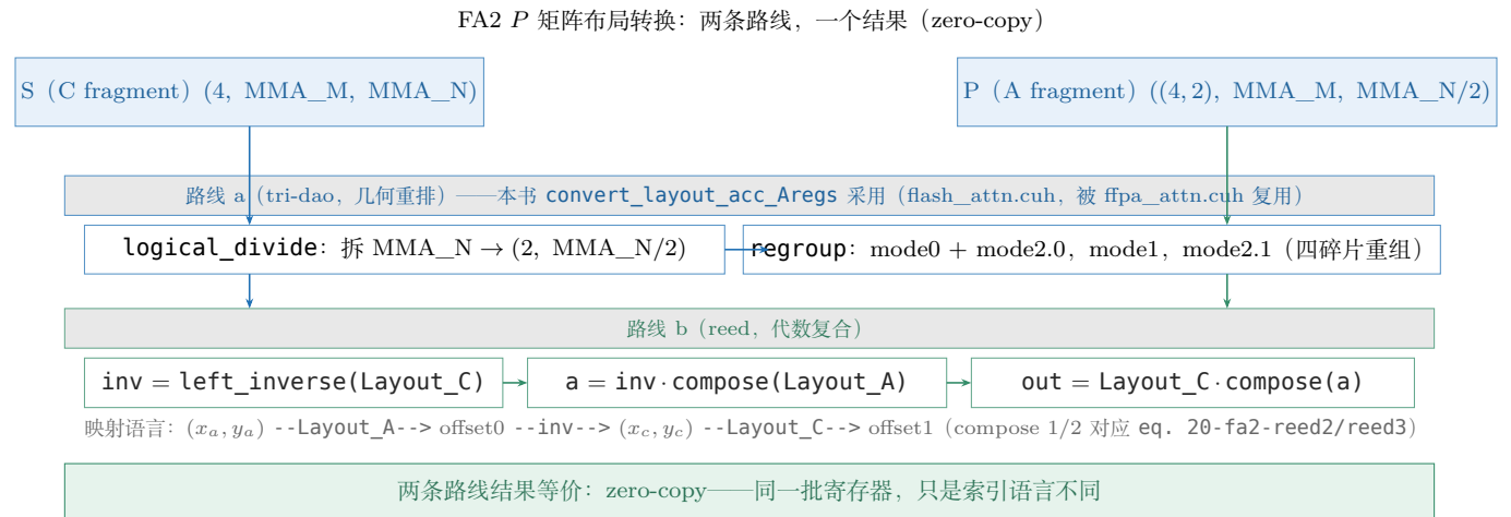
图 21.5: FA2 的 P 矩阵布局转换: tri-dao 的几何重排与 reed 的代数复合两条路线, 结果等价。本书 flash_attn.cuh 的 convert_layout_acc_Aregs (被 ffpa_attn.cuh 复用) 采用的是几何路线。
