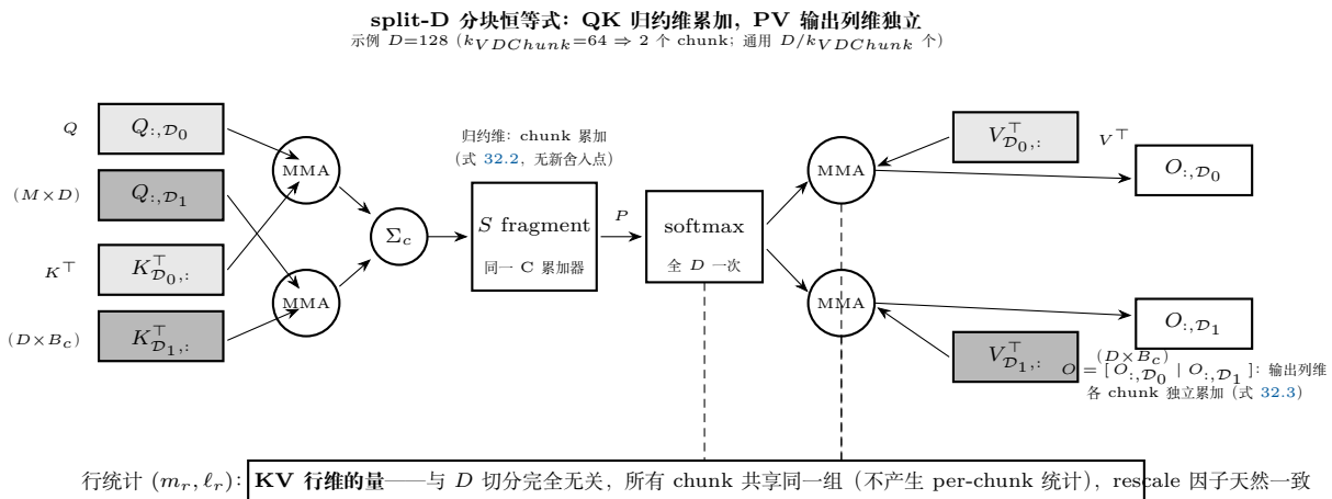
图 32.1: split-D 分块恒等式的数据流 (30.3.1 节)。QK 侧： D 是归约维，各 chunk 的 Q_{:,D_c} K_{D_c,:}^\top 累加进同一个 S fragment (式 32.2, f32/s32 累加，不引入新舍入点)；PV 侧： D 是输出列维，各 chunk 独立累加出 O_{:,D_c} 列段 (式 32.3)，无任何合并。softmax 的行统计 ( m_r, \ell_r ) 是 KV 行维的量——与 D 切分完全无关，所有 chunk 共享同一组 (灰色 = chunk 身份，两图同语义)。
