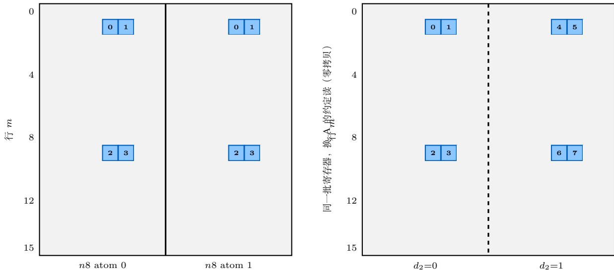
C 视图：列 n ( S 的 B_c 向) C ( m16n8 ): m = \frac{lane}{4} + 8d_1 , n = 2(lane \bmod 4) + d_0 , v = d_0 + 2d_1 ; A ( m16k16 ): m 同式, k = 2(lane \bmod 4) + d_0 + 8d_2 , v = d_0 + 2d_1 + 4d_2 (式 (27.7)/(27.8))。示例 lane=6: 两图高亮的 8 格位置逐格相同 ( m \in \{1, 9\} , 列 \{4, 5\} \cup \{12, 13\} ), C 的值编号 在两个 atom 内各自 0..3 循环, A 因多出 d_2 而连续成 0..7——A 的 K 向 2 值 = C 的列向 2 值, 行维 (m) 的映射本来就一致。
