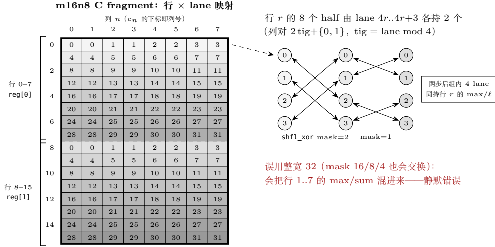
图 17.2: m16n8 C fragment 的行 × lane 映射与 warp_reduce<4> 的宽度依据 (源码注释 L458–474 的图形化)。左: 行 r 与 r+8 的 8 个列元素同由 lane 4r..4r+3 持有 ( \text{tig} = 0..3 各一对), 行 0–7 走 reg[0] 、行 8–15 走 reg[1] ; 右: 组内两步 XOR 蝶形 (mask 2 → mask 1) 后 4 个 lane 同持该行归约值。若误用整宽 32, mask 16/8/4 的交换会把别的行的值混进来——这是 3c 步最典型的静默错误。
