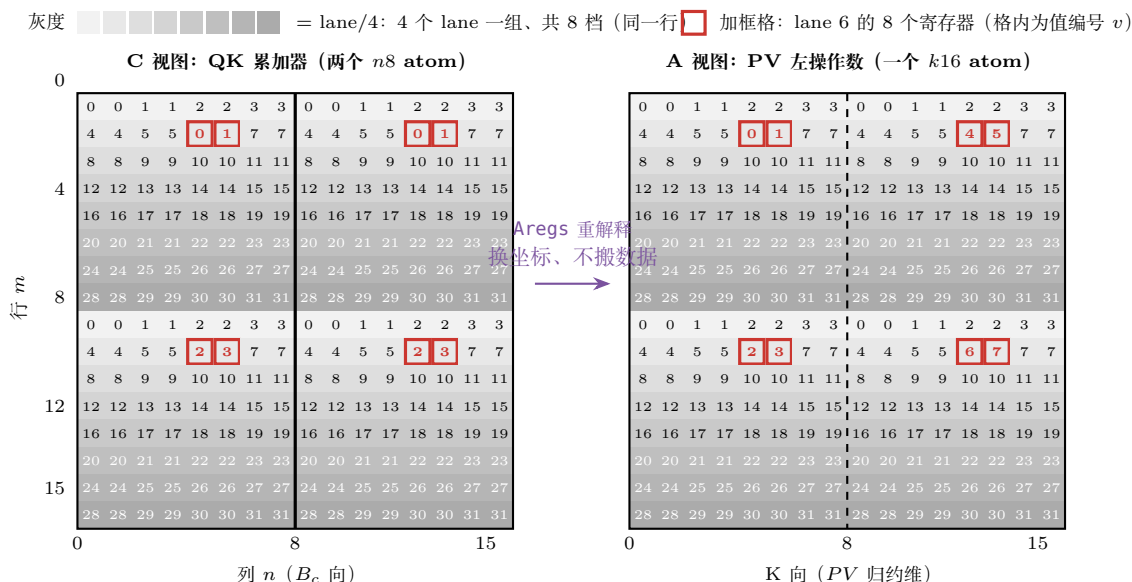
图 26.2: C fragment \rightarrow A fragment 的零拷贝重解释 (convert_layout_acc_Aregs, L2341–2372)。左右两图是同一批寄存器的两套坐标读法: 每格标注持有它的 lane, 灰度按 lane/4 分 8 档 (4 个 lane 一组, 与第十七章 fragment 图的分组语义一致), 两图的格子位置与 lane 归属逐格恒等——这正是「数据一个比特都不用改」的几何形态。差别只在分组与编号: 左图按 n8 累加器约定, 值编号 v = d_0 + 2d_1 在每个 atom 内各自循环 0..3 ( (c_0, c_1) 同行相邻两列、 (c_2, c_3) 行偏移 +8, 即 bit0= 列、bit1= 行); 右图按 k16 A 操作数约定读同一批格子, 值编号变 v = d_0 + 2d_1 + 4d_2 连续 0..7——第二个 n8 atom 的列对成为 K 向的 k \in [8, 16) (虚线半块, d_2=1 )。加框示例 lane 6 的 8 格在两图位置完全相同, 编号从「两轮 0..3」变「一轮 0..7」, 即式 (26.8) 的「列拆半 + 重新配对」。
