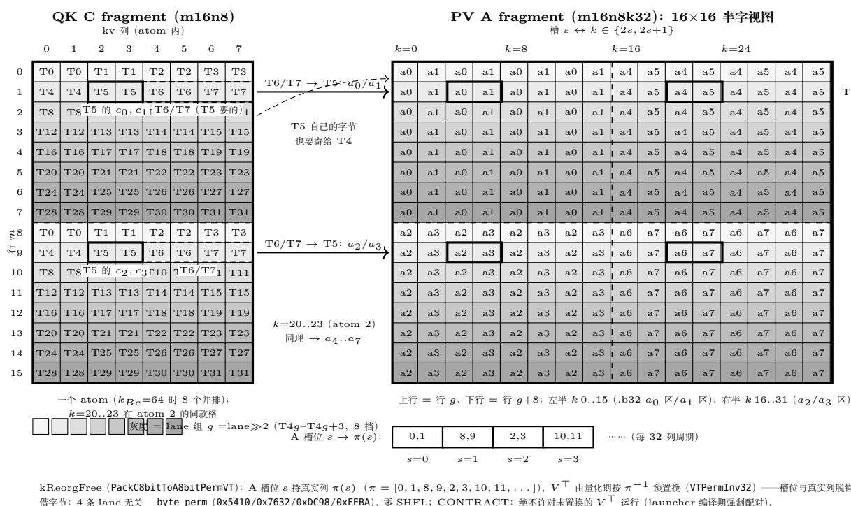
图 31.2: C→A fragment 的 lane→值映射 (lst:29-reorg-bg 的网格化)。左: QK C fragment (m16n8), 每 lane 4 值 c_0 – c_3 落在行 g/g+8 的列对 \{2t, 2t+1\} ; 右: PV A fragment (m16n8k32) 的 16×16 半字视图, 格值 a_0 – a_7 为 e4m3x2 半字寄存器, 四象限对应源码.b32 a_0 – a_3 ; 两面板灰度同语义 (lane 组 g = \text{lane} \gg 2 , 8 档)。中: t=1 (T5) 的自然 A 需要 k \in \{4..7\} \cup \{20..23\} (行 g 与 g+8 ), 在 C 视图里属 T6/T7——纯 lane 内置换凑不齐, 即 16 SHFL + 32 PRMT (ReorgC8bitToA8bit) 的根源。下: kReorgFree 的出路——槽位持 \pi(s) 、 V^\top 预置换, 4 条 lane 无关 __byte_perm、零 SHFL。
