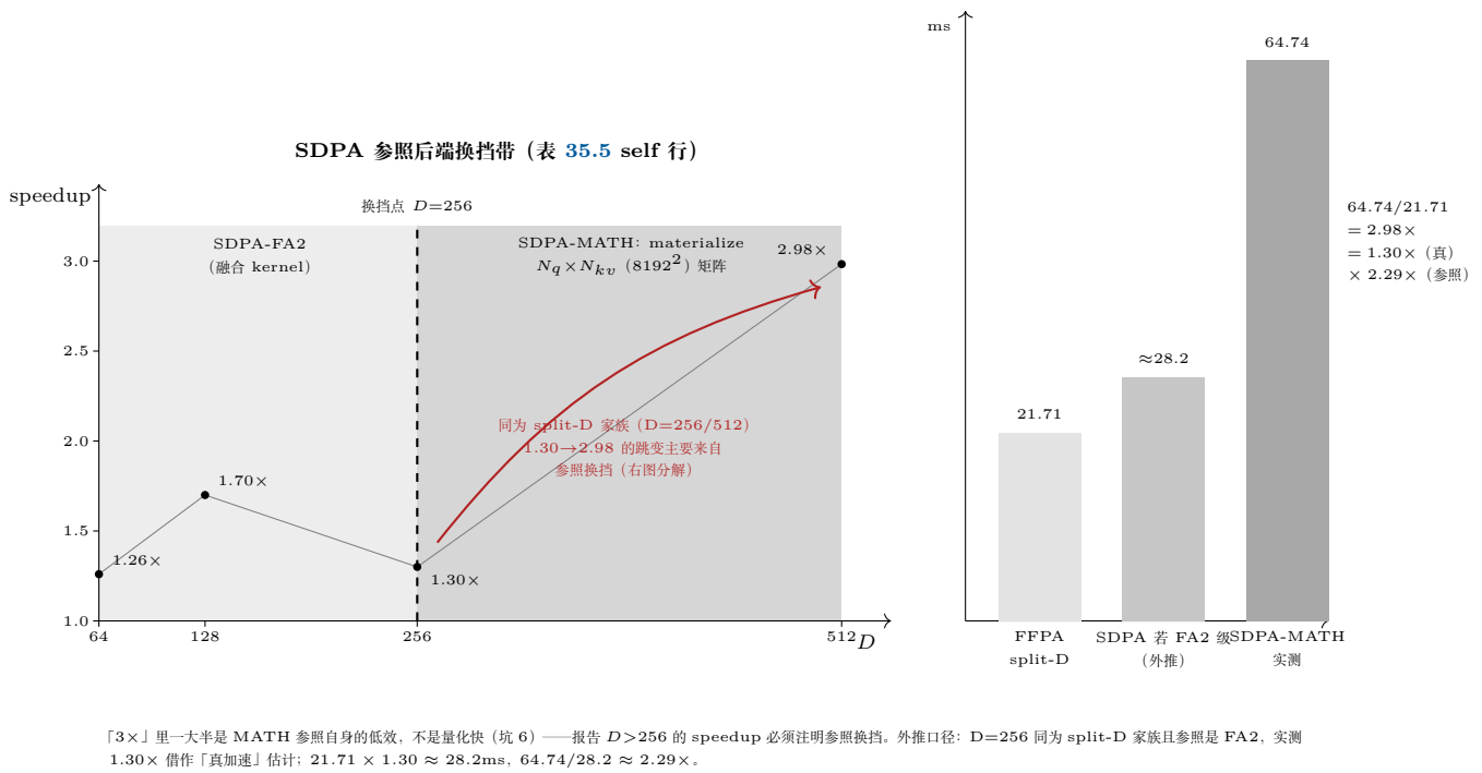
图 35.1: 参照系视角看表 35.5 的 self 行。左: SDPA 参照随 D 换挡——FA2 只覆盖 D \leq 256 , 更大 D 静默落到 MATH (materialize N_q \times N_{kv} 矩阵); 四个 speedup 点 (1.26/1.70/1.30/2.98×) 落在换挡带上, D=512 的跳变与 kernel 无关。右: D=512 的 2.98× 归因——以 D=256 同家族 (split-D、FA2 参照) 实测 1.30× 为真加速估计, MATH 参照自身再慢 \times 2.29 : 「3×」的大头是参照低效 (坑 6)。
