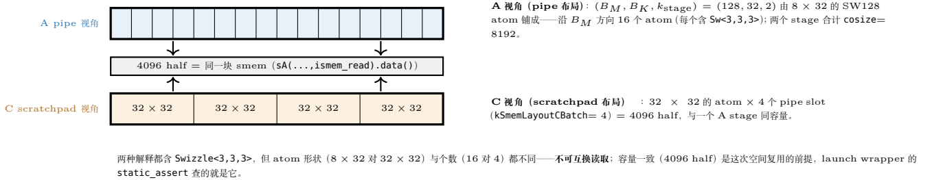
图 22.4: epilogue scratchpad: 同一块 4096 half 的 smem、两种布局视图 (hgemm.cuh L1001)。上条带是 A 的 pipe 解释——(128,32) 的 stage 按 8 \times 32 的 SW128 atom 沿 B_M 切成 16 段；下条带是 C 的 scratchpad 解释—— 32 \times 32 的 atom \times 4 个 pipe slot ( kSmemLayoutCBatch=4 )。中间那条带是两者共用的地址带： sC 拿到的只是 sA(_,_,ismem_read).data() 这个裸指针，没有 Tensor 类型转换，重复的只是「同一段地址的两种读法」。
