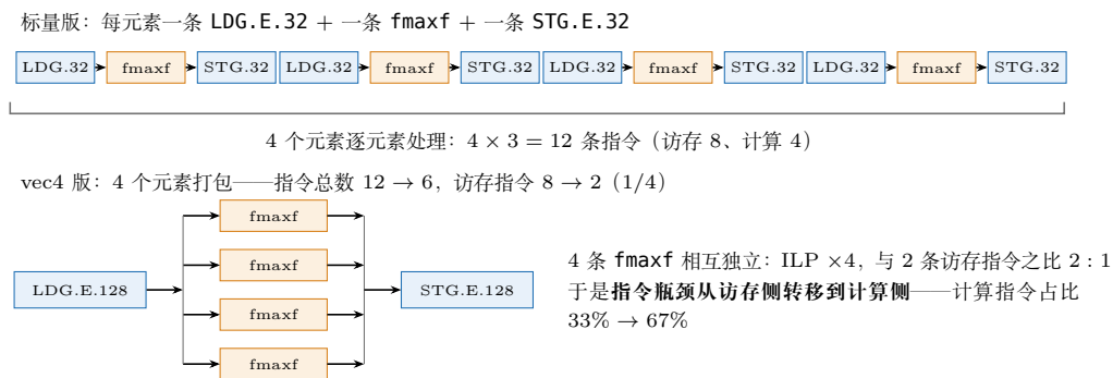
图 4.3: 标量与 vec4 的指令流对照(relu, 以 4 个元素为例): 标量版每元素 3 条指令 ( LDG.E.32 \rightarrow fmaxf \rightarrow STG.E.32 ), 4 元素共 12 条、其中访存 8 条; vec4 版用一条 LDG.E.128 取回 4 个元素, 4 条 fmaxf 互不依赖 ( \text{ILP} \times 4 ) 后由一条 STG.E.128 写回, 总数降到 6 条、访存只剩 2 条。访存: 计算从 8:4 变为 2:4, 指令瓶颈因此从访存侧移到计算侧。
