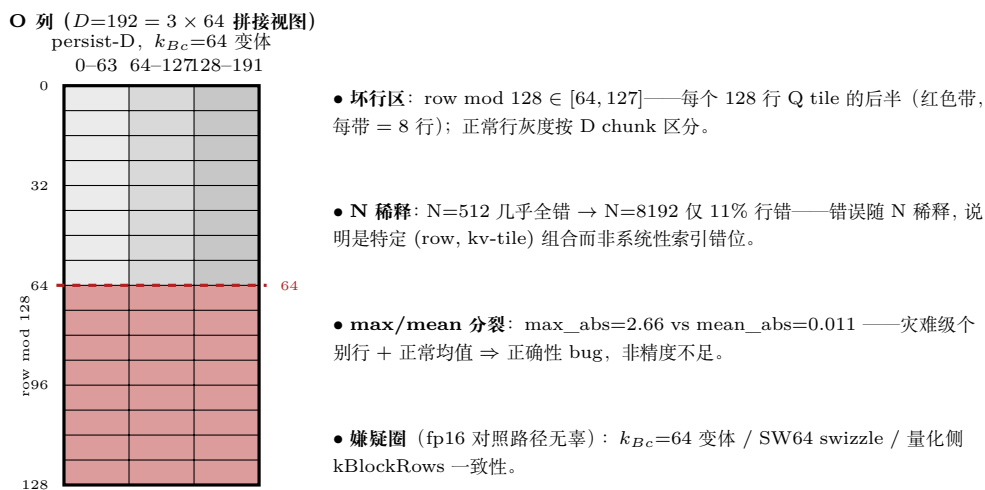
图 31.6: D=192 正确性 bug 的坏行定位 (29.7.1 节五步法的可视化): 把 O 视为 3 \times 64 列拼接, 坏行集中在 \text{row mod } 128 \in [64, 127] (每个 128 行 Q tile 的后半); N=512 几乎全错而 N=8192 仅 11% 行错 (N 稀释 \Rightarrow 特定 (row, kv-tile) 组合); \max\_abs=2.66 对 \text{mean\_abs}=0.011 的分裂是「个别行灾难」的强信号。
