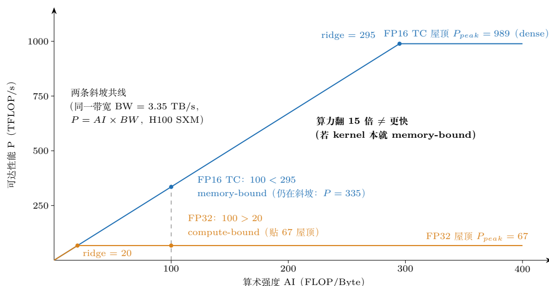
图 2.4: 同一 GPU 的两条屋顶线 (H100 SXM): FP32 ( P_{\text{peak}} = 67 TFLOP/s, ridge = 20) 与 FP16 TC dense ( P_{\text{peak}} = 989 , ridge = 295) 共用同一条带宽斜坡 (BW = 3.35 TB/s), 脊点相差约 15 倍。AI=100 的竖虚线在两条线上落点相反: FP32 侧已 compute-bound ( 100 > 20 ), FP16 TC 侧仍 memory-bound ( 100 < 295 ) ——把 kernel 迁到 Tensor Core 未必变快; ridge 口径算错 (如 sparse 当 dense) 会把 bound 类别判反。
