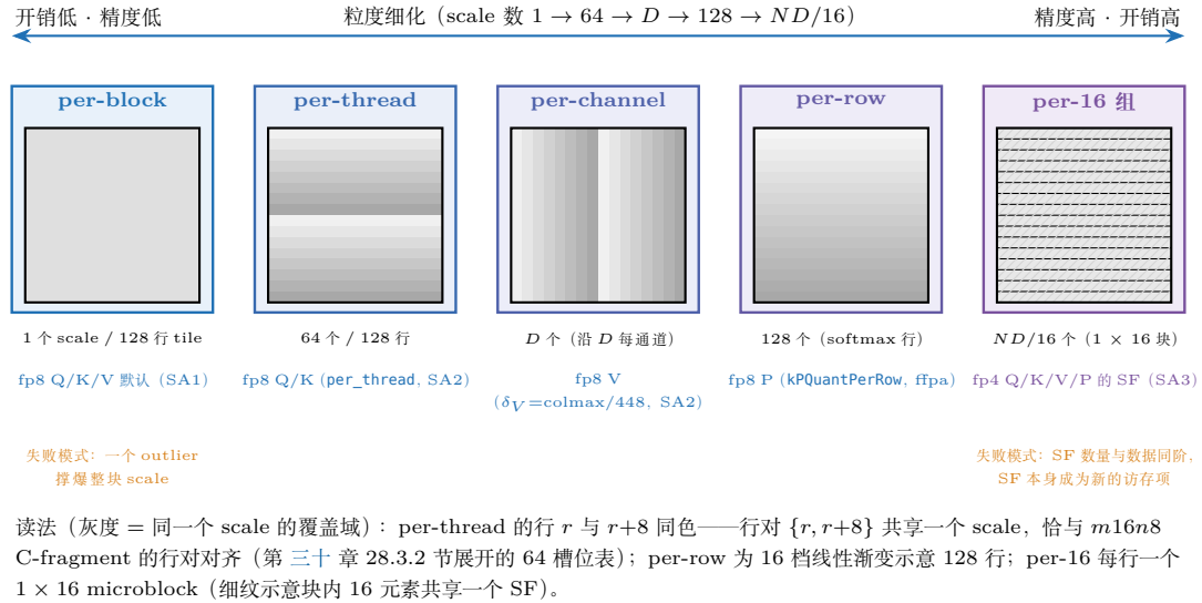
图 29.1: 量化粒度谱系五联网络 (表 29.2 的可视化, 缩略网络为 16 行 \times 16 列)。从左到右: per-block 整块共享 1 个 scale; per-thread 按 C-fragment 行对 \{r, r+8\} 分档 (128 行块共 8 \times 8 = 64 个, 零 shuffle 消费); per-channel 沿 D 每通道一个; per-row 每 softmax 行一个 (128 个); per-16 每行一个 1 \times 16 microblock (NVFP4 的 SF)。顶部双向轴是整条谱系的 trade-off: 粒度越细精度越高, 但 scale 的存储、传递与消去开销同步上涨, 且必须与 MMA 的 fragment 布局对齐——谱系两端的失败模式分别是对 outlier 的脆弱性与 SF 自身的访存账。
