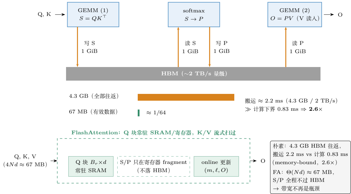
图 16.2: 朴素 attention 的 HBM 往返账 vs FlashAttention (15.3.3 节, B=1, H=32, N=4096, d=64 ): 上行三个 kernel 之间, S 与 P (各 \approx 1 \text{ GiB} ) 必须经 HBM 往返——写 S 、读 S 、写 P 、读 P 共 4 \times 1 \text{ GiB} \approx 4.3 \text{ GB} , 而有效数据 ( Q, K, V 读入 + O 写出) 只有 \approx 67 \text{ MB} , 占全部流量的 1/64 ; 按 2 \text{ TB/s} 乐观带宽, 仅搬运就要 \approx 2.2 \text{ ms} , 已是 0.83 \text{ ms} 计算下界的 2.6 倍——kernel 被钉死在 memory-bound 区。下行 FlashAttention 把 S, P 困在 SRAM/寄存器 fragment 里 (虚线框), HBM 只见 Q, K, V 进、 O 出 ( \Theta(Nd) , 式 16.9 的另一端), 中间量全程不过 HBM。
