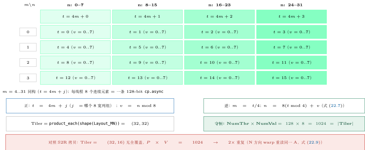
图 22.5: thread×value 网格: G \rightarrow S 拷贝把 32 \times 32 的 tile 划成 t = 4m + j 的网格, 每个线程搬 8 个连续元素 (一条 128-bit cp.async )。同一划分用 MN 语言或 TV 语言描述是等价的 (式 (22.6) 与式 (22.7)); 本章测试 case A/B 对 1024 个 (t, v) 对与 4096 个坐标逐一核对了这两组公式。
