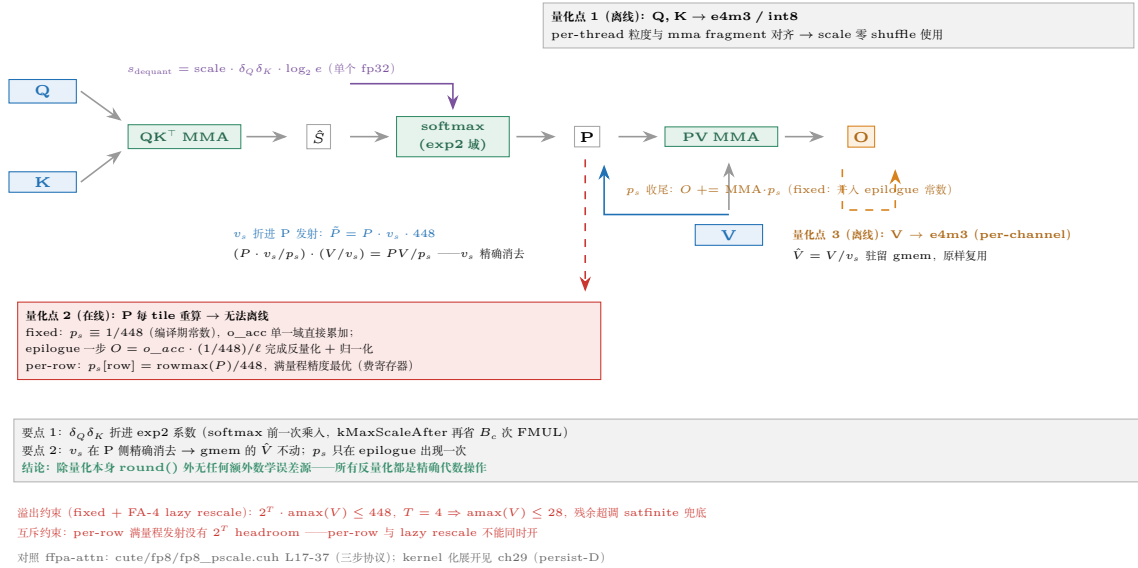
图 29.6: attention 的三个量化点与 scale 流向： \delta_Q \delta_K 折进 exp2 系数 (式 29.4)、 v_s 在 P 侧精确消去 (式 29.5)、 p_{\text{scale}} 在 epilogue 一步收尾。
