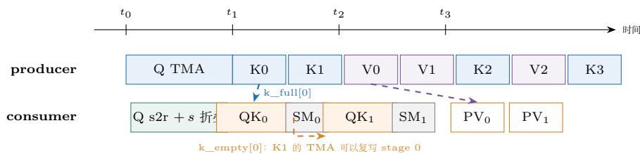
图 28.4: producer/consumer 流水时序 ( S_K=S_V=2 示意)。producer 每个 KV tile 领先 S-1 发射下一个 tile 的 TMA, 且 V 先于 K 发射 (V 的消费点更晚, K 的传输得以填进 QK 计算窗口)。虚线箭头是 mbarrier 握手: k\_full[s] (事务屏障, TMA 完成 + expect_tx 校验) 放行 consumer 读取; k\_empty[s] (consumer 每线程 arrive) 放行 producer 复写该 stage。S tile 的 softmax ( SM_i ) 与下一 tile 的 QK 在 consumer 侧串行, 但与 producer 侧的 TMA 完全重叠。
