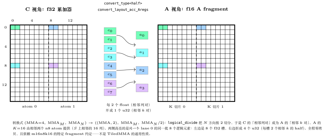
图 23.2: QK→PV 的寄存器原地复用 (ffpa_attn.cuh L300–305、源码注释 flash_attn.cuh L2341–2372): 两侧网格是同一个 16 \times 16 坐标空间 ( S 的列 = P 的 K ), 高亮的是 lane 0 在同一批元素上的两套坐标。左 (C 视角): 每个 n8 atom 给 lane 0 留下 4 个 f32 累加器 (2 行 \times 2 相邻列), 两个相邻 atom 共 8 个; 右 (A 视角): 同样 8 个逻辑元素被解释成 4 个 u32, 每槽 2 个相邻 k 的 half, 可直接作为 gemm_rs 的 tCrA。convert_type<half> (fp32→fp16, 寄存器减半) + convert_layout_acc_Aregs ( N 方向按 2 切分的重索引) 就是这条「P 不写回 smem」路径的全部代价。
