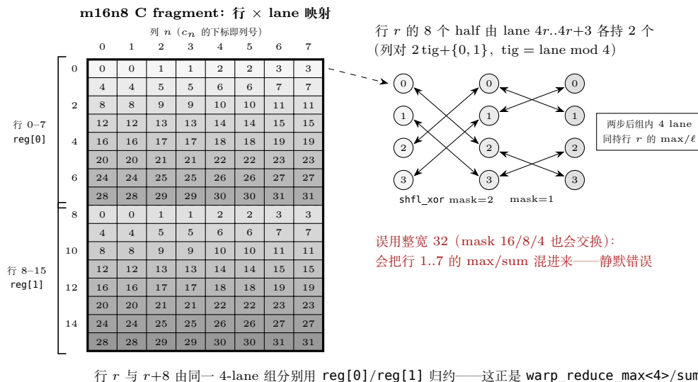
图 17.2: m16n8 C fragment 的行 × lane 映射与 \text{warp\_reduce}<4> 的宽度依据 (源码注释 L458–474 的图形化)。左: 行 r 与 r+8 的 8 个列元素同由 lane 4r..4r+3 持有 ( \text{tig} = 0..3 各一对), 行 0–7 走 \text{reg}[0] 、行 8–15 走 \text{reg}[1] ; 右: 组内两步 XOR 蝶形 (mask 2 → mask 1) 后 4 个 lane 同持该行归约值。若误用整宽 32, mask 16/8/4 的交换会把别的行的值混进来——这是 3c 步最典型的静默错误。
