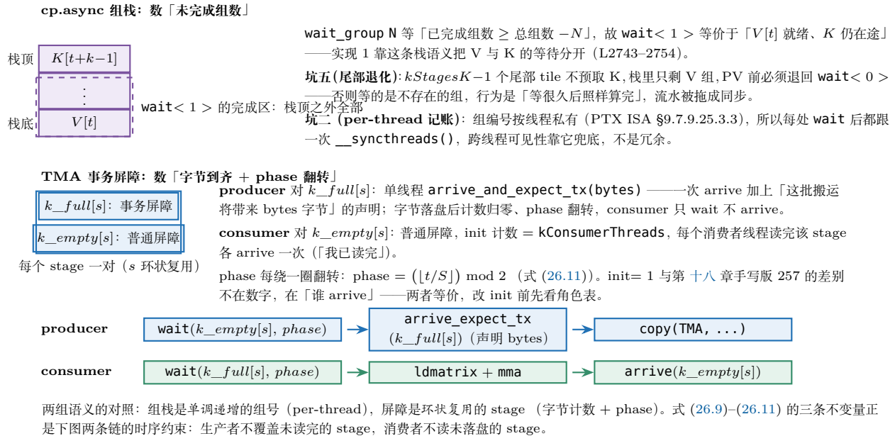
图 26.3: 两种异步等待语义的时间线对照 (flash_attn.cuh L2743–2754 与 ffpa_attn.cuh 的 TMA 版)。上: cp.async 组栈——提交顺序 V[t] (栈底) \rightarrow K[t+k-1] (栈顶), \text{wait} < 1 > 停在「除栈顶 K 之外全部完成」, 尾部 k\text{Stages}K-1 个 tile 必须退回 \text{wait} < 0 > (坑五); 每处 \text{wait} 后跟一次 \_\_\text{syncthreads}() (坑二: 组计数按线程私有)。中下: TMA 的事务计数——每个 stage 一对 k\_full[s] (事务屏障, producer 单线程 \text{arrive\_and\_expect\_tx} ) 与 k\_empty[s] (普通屏障, \text{init} = k\text{ConsumerThreads} ), phase 由 [t/S] \bmod 2 现算; 最下一行是两条流水链的时序。
