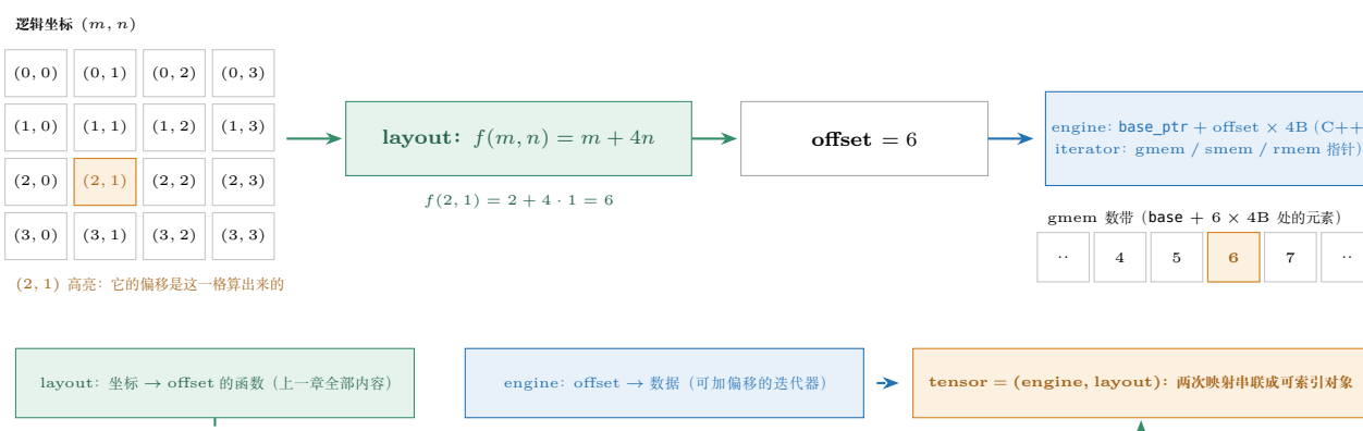
图 22.1: Tensor 的两段结构: layout 把坐标映成偏移, engine 把偏移映成数据。同一个 layout 换不同 engine (gmem/smem/rmem/identity) 就得到服务不同内存的 Tensor——这是第 二十一 章「布局与内存解耦」的落地方式。
