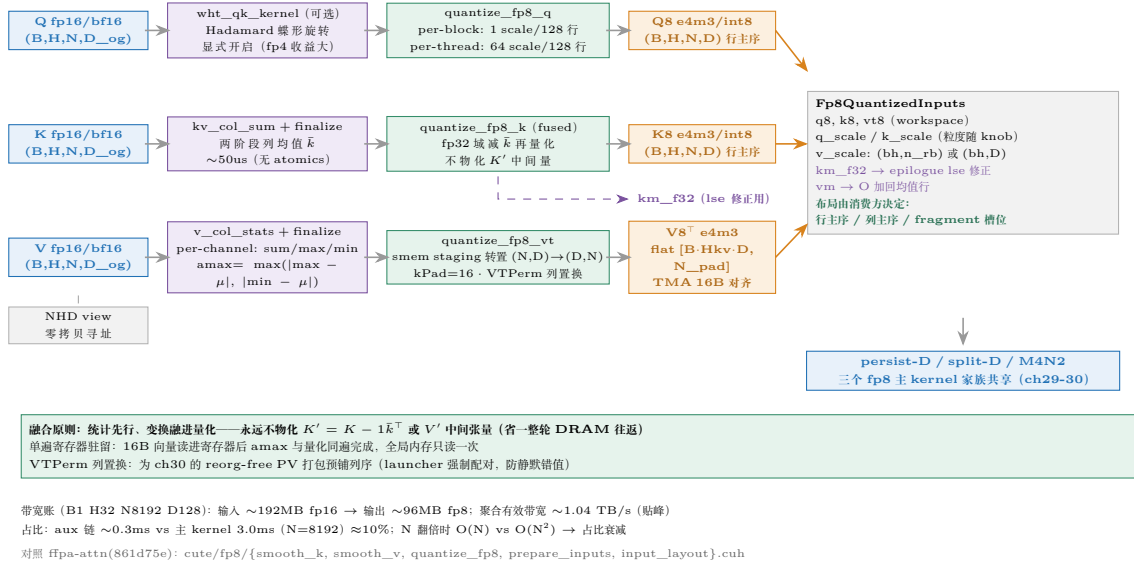
图 30.5: fp8 前处理链全景：三泳道 (Q/K/V) 各自的统计 → 变换 → 量化 kernel 与输出 workspace 布局。smoothing 与量化融合在同一 kernel 内 (无中间落盘)； V^T 的列 pad 兼顾 TMA 16B 对齐与置换写。
