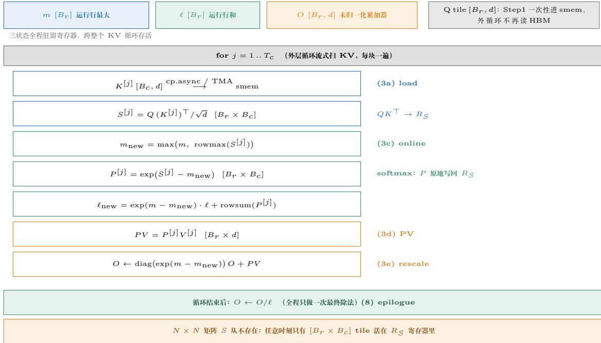
图 16.3: Attention 分块计算: 单个 Q 块 ( B_r 行) 流式扫过全部 T_c 个 KV 块 ( B_c \times d ), 每块依次执行 S^{[j]} \rightarrow P^{[j]} \rightarrow P^{[j]} V^{[j]} , 并把 (m, \ell, O) 三状态按式 16.12–16.17 联动更新, 循环结束后统一除 \ell 。步骤编号对齐 flash_attn.cuh L48–59 的执行流程。
