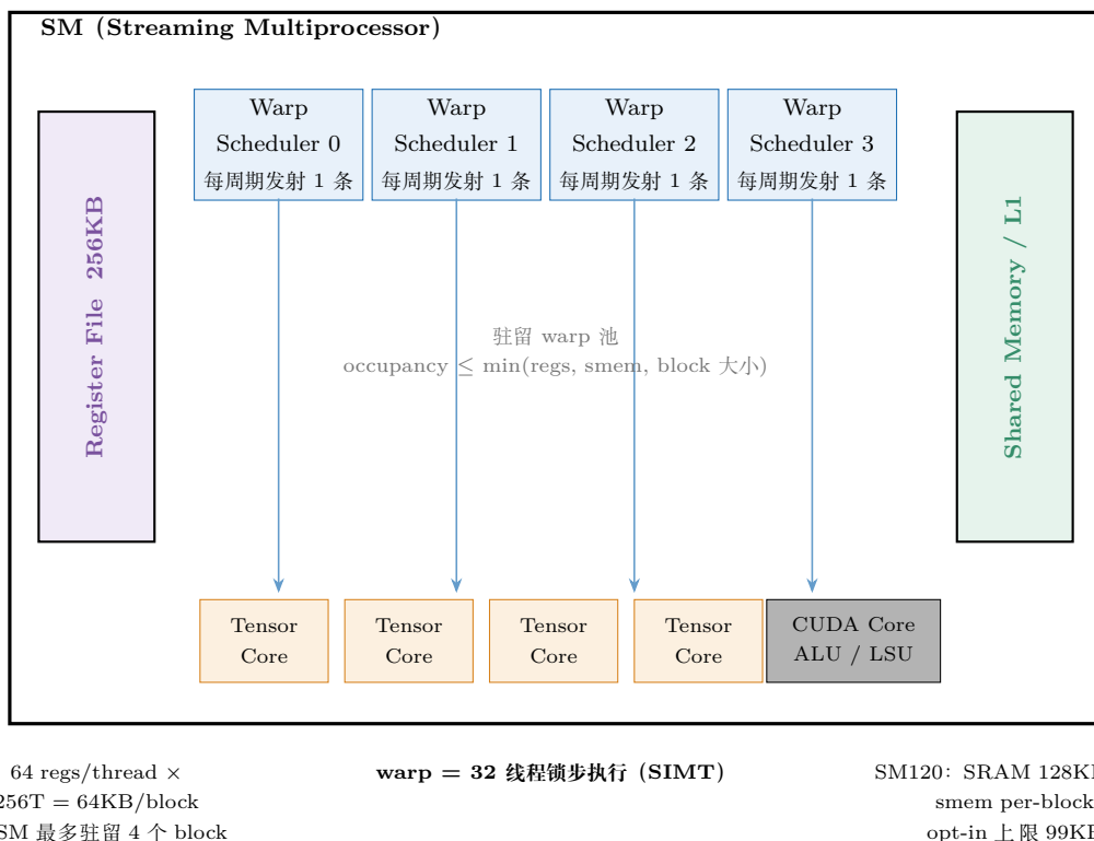
图 2.1: SM 内部结构示意图 (Blackwell sm_120 口径): 顶部 4 个 warp scheduler (各每周期发射 1 条指令), 左侧 256KB 寄存器文件与右侧 smem/L1 共池 SRAM 共同钳制驻留 block 数, 底部 4 个 Tensor Core 与 CUDA Core 阵列执行发射来的指令。
