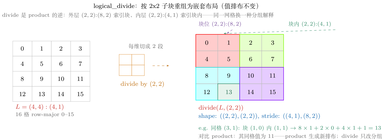
图 21.11: logical_divide: 按 2 \times 2 子块把 (4, 4):(4, 1) 重组为 ((2, 2), (2, 2)):((4, 1), (8, 2)) (CuTe 实测的 zipped 形式: 块内 mode 在前、块位 mode 在后)——值排布不变 (仍 row-major), 改变的只是索引方式 (一组 (4, 1) 索引块内、一组 (8, 2) 索引块位)。与上图对比: 同物理格 (3, 1) 的 product 值为 11 (新排布), divide 后仍为 13 (原排布)。重建自同上文。
