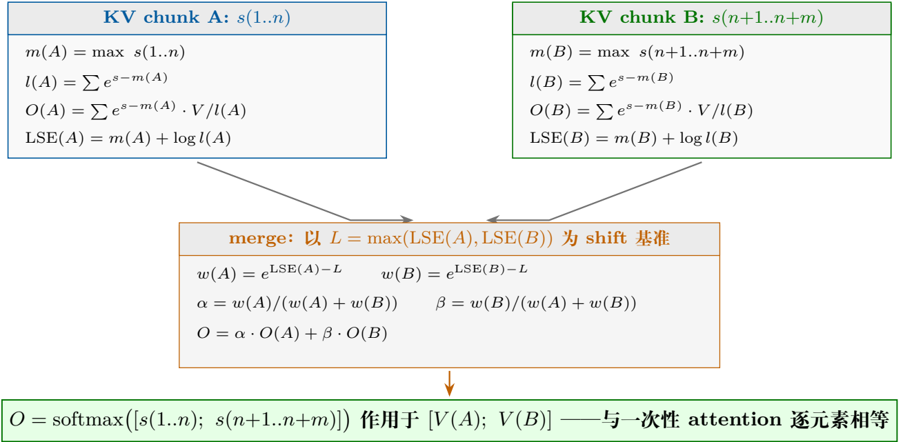
图 6.3: 两个分块 attention 状态的合并: 块内各自输出 (已归一化 O 与单标量 LSE), 块间以 L = \max(\text{LSE}) 为 shift 基准计算凸组合系数 \alpha, \beta , 合并结果与整体 softmax 直接加权逐元素相等 (定理 6.2)。
