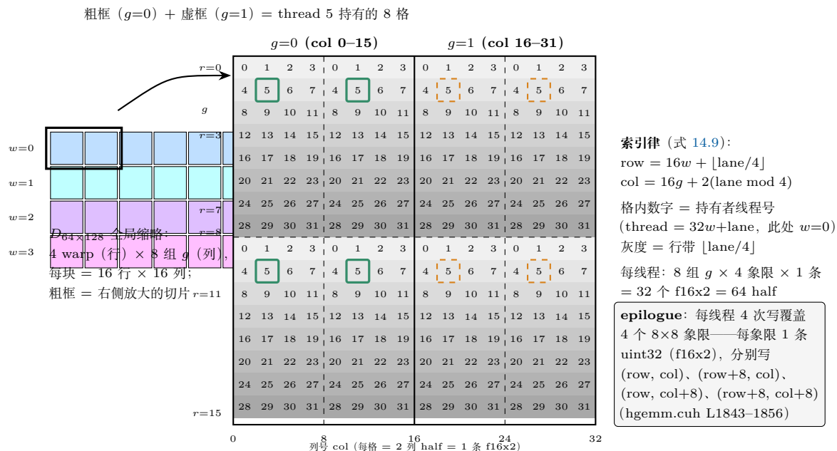
图 14.2: WGMMA m64n128k16 输出 D 的寄存器分布 (13.3.4 节, 式 14.9): 左为 64 \times 128 全局缩略 (4 warp \times 8 组 g , 每块 16 行 \times 16 列); 右侧放大 warp w=0 的 16 行切片 ( g=0,1 两组, 每格一条 f16 \times 2 = 相邻 2 列), 格内数字为持有该输出的线程号、灰度按行带 \lfloor \text{lane}/4 \rfloor 区分。索引律 \text{row} = 16w + \lfloor \text{lane}/4 \rfloor 、 \text{col} = 16g + 2(\text{lane} \bmod 4) 使每个线程在每组 g 内恰好持有 4 个 8 \times 8 象限里各一条寄存器 (粗框/虚框标出 thread 5 的 8 格), epilogue 据此用 4 次写覆盖 4 个象限。
