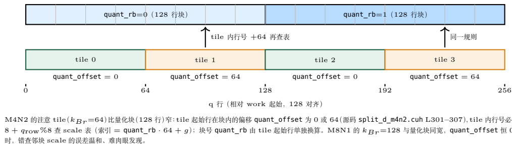
图 35.3: 量化 128 行块与 M4N2 注意 tile ( k_{Br}=64 ) 的错位对齐。tile 1/3 的起始行落在量化块内的偏移 64 处, 其行号需先加 quant_offset 再查 per-thread scale 表; tile 0/2 偏移为 0。M8N1 的 k_{Br}=128 与量化块同宽, 不存在该映射。
