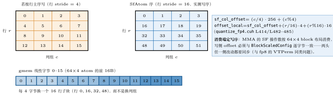
图 36.3: SF 字节的写序由消费端决定 ( V^T 量化链)。同一 (r, c) 单元格在行主序假设下偏移 4r + c , 在 SfAtom 序下偏移 16r + c : 每 4 个列组构成 64 \times 4 的 256B atom, atom 内按 16 行子块交错。写侧 (sf_col_offset/offset_local) 与 MMA 的 BlockScaledConfig 必须逐字节一致。
