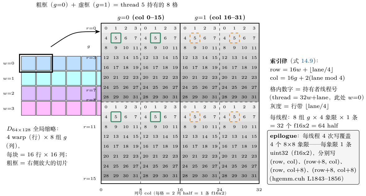
图 14.2: WGMMMA m64n128k16 输出 D 的寄存器分布 (13.3.4 节, 式 14.9): 左为 64 \times 128 全局缩略 (4 warp \times 8 组 g , 每块 16 行 \times 16 列); 右侧放大 warp w=0 的 16 行切片 ( g=0,1 两组, 每格一条 \text{f16x2} = 相邻 2 列), 格内数字为持有该输出的线程号、灰度按行带 \lfloor \text{lane}/4 \rfloor 区分。索引律 row = 16w + \lfloor \text{lane}/4 \rfloor 、col = 16g + 2(\text{lane mod } 4) 使每个线程在每组 g 内恰好持有 4 个 8 \times 8 象限里各一条寄存器 (粗框/虚框标出 thread 5 的 8 格), epilogue 据此用 4 次写覆盖 4 个象限。
