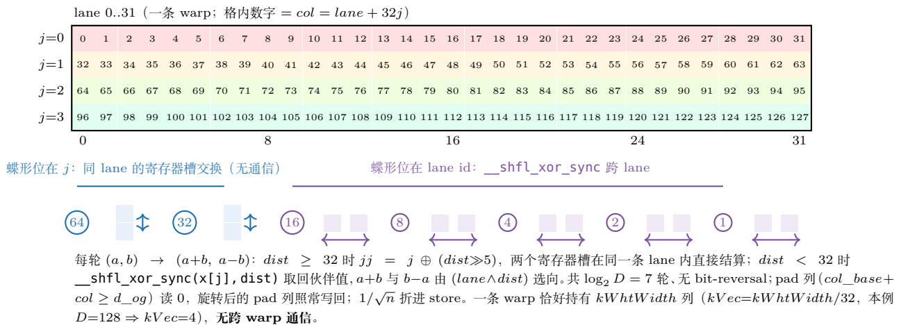
图 33.4: radix-2 蝶形的距离二分 (hadamard.cuh L40-92, 本例 D=128 、 kWhWidth=D )。上: 列归属—— j 是寄存器槽、lane 是 warp 内线程, 格内数字 col = lane + 32j 满足索引律, 右下角 127 = \text{size} - 1 ; 一条 warp 覆盖整行 128 列。下: 七轮的「距离阶梯」—— dist \geq 32 的 bit 落在 j 上 (同 lane 两个寄存器槽直接加减, 无通信), dist < 32 的 bit 落在 lane id 上 ( __shfl_xor_sync 跨 lane); 每轮一个 bit, 1/\sqrt{n} 折进 store。
