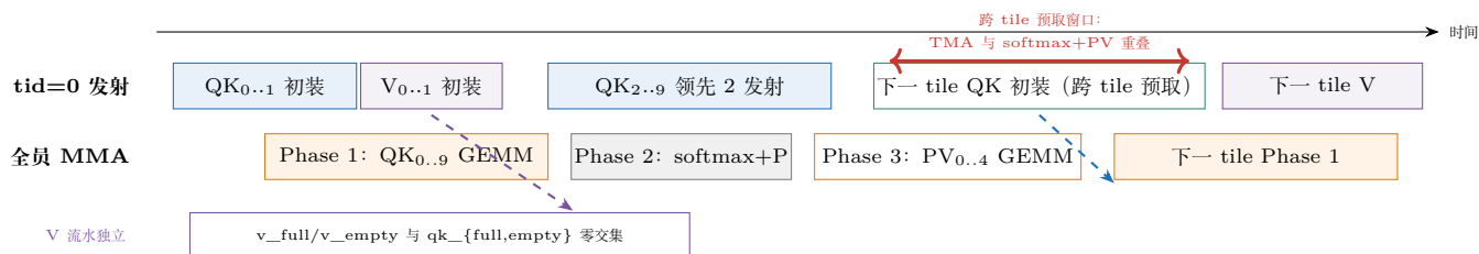
图 29.2: 单 kv_tile 内的相位时间线与跨 tile 预取 ( S_K=S_V=2 , D=320 的 10+5 chunk 结构示意图)。上线是 tid=0 的发射序列: 初始预取填满两条流水, 主循环内每个 QK chunk 消费完领先 S_K 发下一个, V 预取每 tile 开头补一批; 本 tile QK 相位一结束 (stage 池整体空闲), 立刻发射下一 tile 的初始 QK chunk。下线是全员 MMA 的计算序列。红色双箭头是本章协议的核心红利: 下一 tile 的 QK 装载与本 tile 的 softmax (纯寄存器 + shfl) 和 PV GEMM 完全重叠——QK/V 两套 barrier 集不相交保证这段发射不会与后续相位互相等待。
