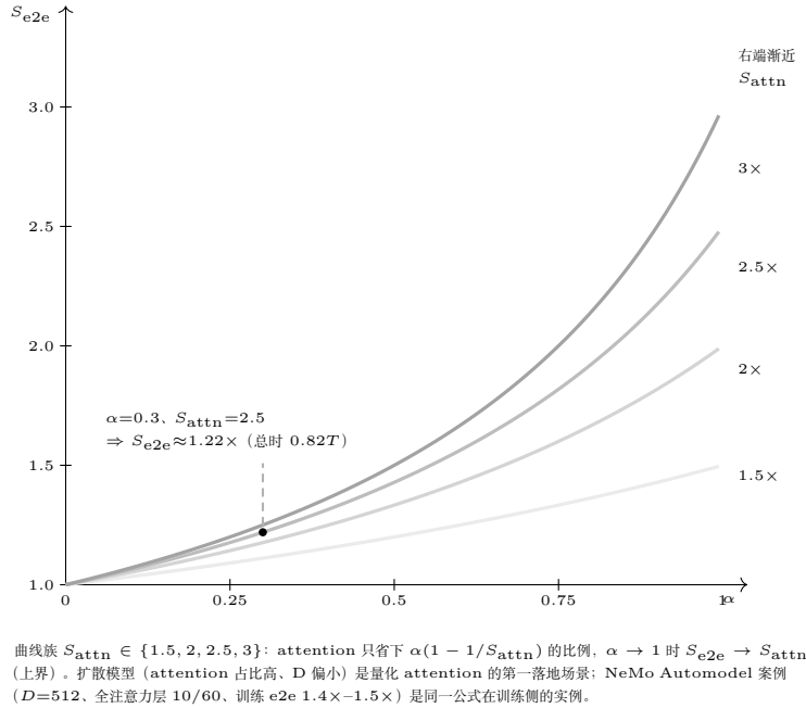
图 38.2: 端到端摊销曲线族（式 38.3）：单算子 S_{\text{attn}} 换算到管线收益由 attention 占比 \alpha 封顶。 \alpha=0.3 、 S_{\text{attn}}=2.5\times 时只剩 1.22\times ； \alpha \rightarrow 1 的渐近线即 S_{\text{attn}} 。
