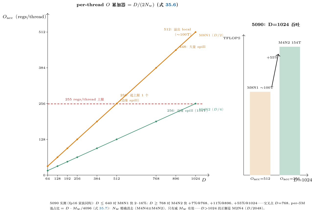
图 35.2: 寄存器墙的定量视图。左: per-thread O 累加器 = D/(2N_w) (式 35.6) —— M8N1 的 D/2 在 D=512 达 256 (超 255 上限 1 个, 边缘 spill)、 D \geq 896 大量 spill、 D=1024 溢出 local memory ( \sim 100T ); M4N2 的 D/4 同点仅 256 (154T)。右: 5090 实测 D=1024 吞吐对比 (+55%)。下: per-SM 池占比 D \cdot M_w / 4096 (式 35.7) 中 N_w 精确消去——加 N-warp 不降总量, D > 1024 只能走 M2N4。
