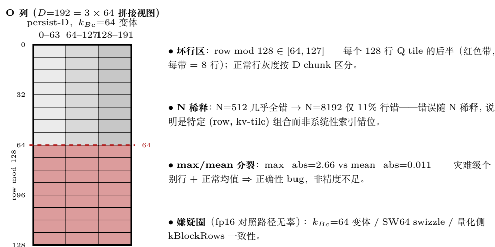
图 34.6: D=192 正确性 bug 的坏行定位（29.7.1 节五步法的可视化）：把 O 视为 3×64 列拼接，坏行集中在 \text{row mod } 128 \in [64, 127] （每个 128 行 Q tile 的后半）；N=512 几乎全错而 N=8192 仅 11% 行错（N 稀释 ⇒ 特定 (row, kv-tile) 组合）；max_abs=2.66 对 mean_abs=0.011 的分裂是「个别行灾难」的强信号。
