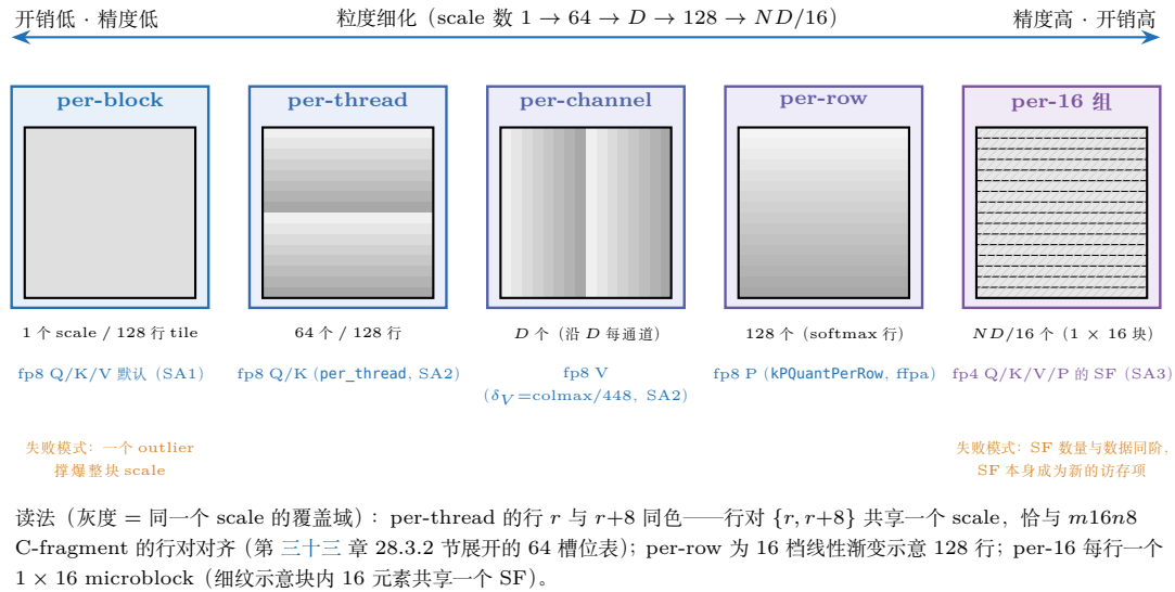
图 32.1: 量化粒度谱系五联网格 (表 32.2 的可视化, 缩略网格为 16 行 \times 16 列)。从左到右: per-block 整块共享 1 个 scale; per-thread 按 C-fragment 行对 \{r, r+8\} 分档 (128 行块共 8 \times 8 = 64 个, 零 shuffle 消费); per-channel 沿 D 每通道一个; per-row 每 softmax 行一个 (128 个); per-16 每行一个 1 \times 16 microblock (NVFP4 的 SF)。顶部双向轴是整条谱系的 trade-off: 粒度越细精度越高, 但 scale 的存储、传递与消去开销同步上涨, 且必须与 MMA 的 fragment 布局对齐——谱系两端的失败模式分别是对 outlier 的脆弱性与 SF 自身的访存账。
