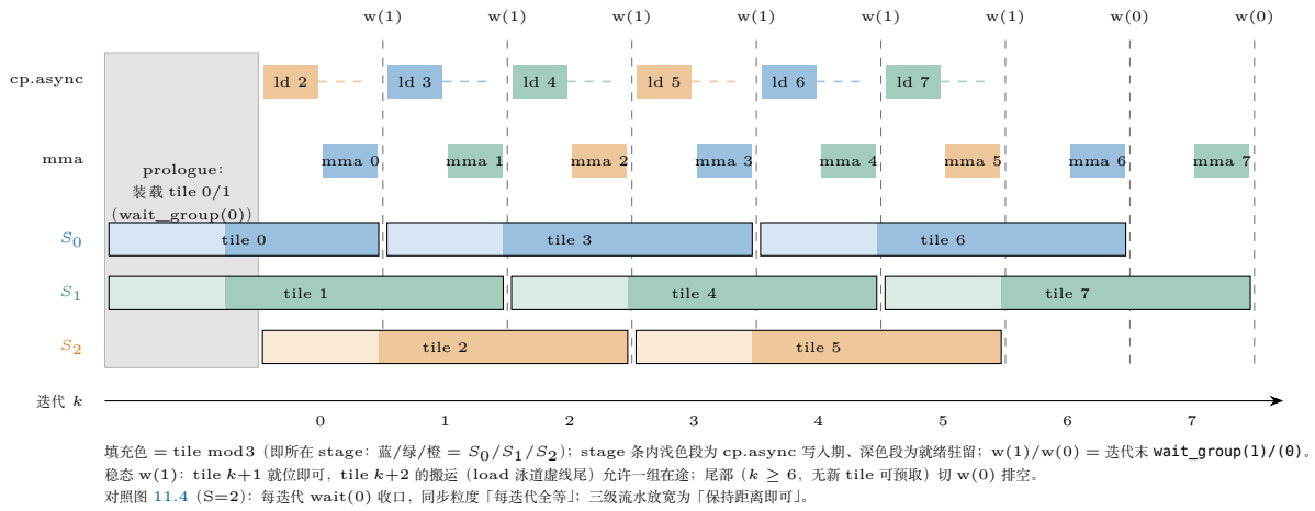
图 12.5: k\text{Stages}=3 三级流水时序: 迭代 k 读 S_{k \bmod 3} (tile k )、同时预取 (k+2) \bmod 3 (tile k+2 ), 三个 stage 按 tile mod 3 轮转。稳态迭代末 wait_group(1) 允许一组搬运在途; 尾部无 tile 可预取时切 wait_group(0) 排空。与图 11.4 的两级流水 (每迭代 wait(0)) 相比, 同步粒度从「每迭代全等」放松为「保持距离即可」。
