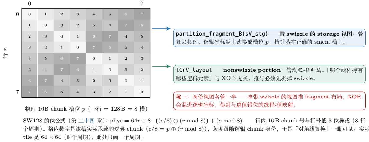
图 27.4: V 的双视图分工 (ffpa_attn.cuh L136–141)。同一张 SW128 smem tile: sV_stg (带 swizzle 的 storage 视图) 负责把逻辑坐标换算成物理槽位、给数据指针用; tCrV_layout (由 nonswizzle portion 推导) 负责回答「哪个线程持有 哪些逻辑元素」。SW128 的 XOR 只改地址、不改归属, 所以推 fragment 布局时必须先剥掉 swizzle——两份视图各管一半, 混用即错 (坑一)。
