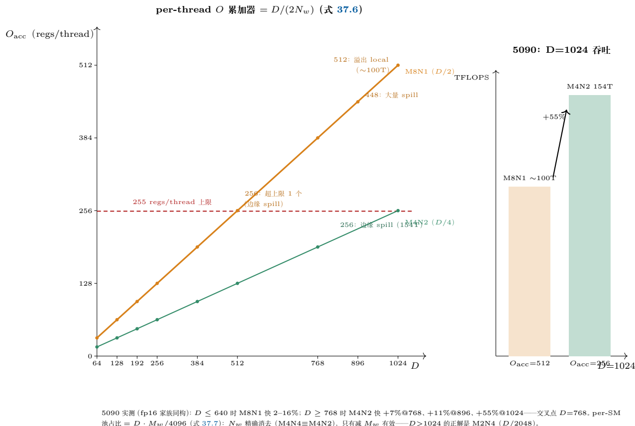
图 37.2: 寄存器瓶颈的定量视图。左: per-thread O 累加器 = D/(2N_w) (式 37.6) ——M8N1 的 D/2 在 D=512 达 256 (超 255 上限 1 个, 边缘 spill)、 D \geq 896 大量 spill、 D=1024 溢出 local memory (~100T); M4N2 的 D/4 同点仅 256 (154T)。右: 5090 实测 D=1024 吞吐对比 (+55%)。下: per-SM 池占比 D \cdot M_w / 4096 (式 37.7) 中 N_w 精确消去——加 N-warp 不降总量, D > 1024 只能走 M2N4。
