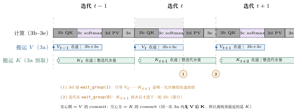
图 17.4: K 双缓冲、V 单级的流水时序（16.4.5 节 3a 步）。三个稳态迭代 t-1/t/t+1 ：每个迭代内 3a 依次提交两组搬运—— V_t （实心圆，写当前 V buffer）与 K_{t+1} （空心方，写 smem_sel_next）。 V_t 的在途窗口（蓝条）恰好覆盖同迭代的 3b (QK mma) 与 3c (softmax) ——softmax 全在 CUDA Core/SFU 上跑，恰好掩盖 V 的搬运延迟； K_{t+1} 则有整整一个迭代的余量。两处等待：(1) 3d 前的 wait_group(1) 只等 V_t ，把 K_{t+1} 留在途；(2) 迭代末 (3e 之后) 的 wait_group(0) 等 K_{t+1} 到齐才进下一轮 3b。与第十二章 GEMM 的「kStages 全操作数统一多级」不同——attention 两段 mma 之间夹着一段非 mma 计算，天然提供了第二级的隐藏窗口，所以 kStagesK=2 就够（「one stage is enough for V」）。
