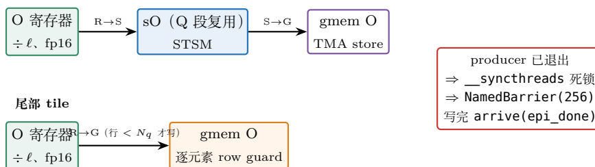
图 28.6: Epilogue 双路径。整 tile 走 R \rightarrow S \rightarrow G : STSM 把 O fragment 写进 (已闲置的) Q smem 段, NamedBarrier 后由一个线程发射 TMA store——与装载对称的「反向 TMA 全链」。尾部 tile 行数不足 128, STSM/TMA 的整块写会越界, 退化为带行 guard 的 R \rightarrow G 。
