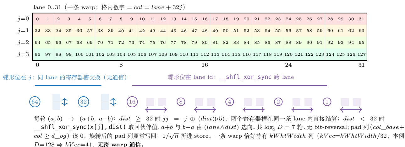
图 35.4: radix-2 蝶形的距离二分 (本例 D=128 、 kWhtWidth=D )。上: 列归属—— j 是寄存器槽、lane 是 warp 内线程, 格内数字 col = lane + 32j 满足索引律, 右下角 127 = size - 1 ; 一条 warp 覆盖整行 128 列。下: 七轮的距 离二分—— dist \geq 32 的 bit 落在 j 上 (同 lane 两个寄存器槽直接加减, 无通信), dist < 32 的 bit 落在 lane id 上 ( shfl xor sync 跨 lane); 每轮一个 bit, 1/\sqrt{n} 折进 store。
