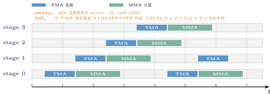
图 33.4: 四级流水的时序示意 ( BN 取 128 的默认档; 本卡 k_{Stages} 可用到 8~10 级, 见 33.9.4 节扫描表)。与第三十一章图 31.2 的结构差别在 MMA 块的宽度: FP4 的一个 stage 只有一跳原子 ( BK=64 ), K 方向不再有内层循环, MMA 块相对 TMA 块更窄——这意味着流水线对 TMA 延迟的容忍度更低, 是 BN 翻倍的收益来源之一 ( BN 翻倍 = MMA 块宽翻倍, 而 TMA 字节数只增加 B 与 SFB 的部分)。
