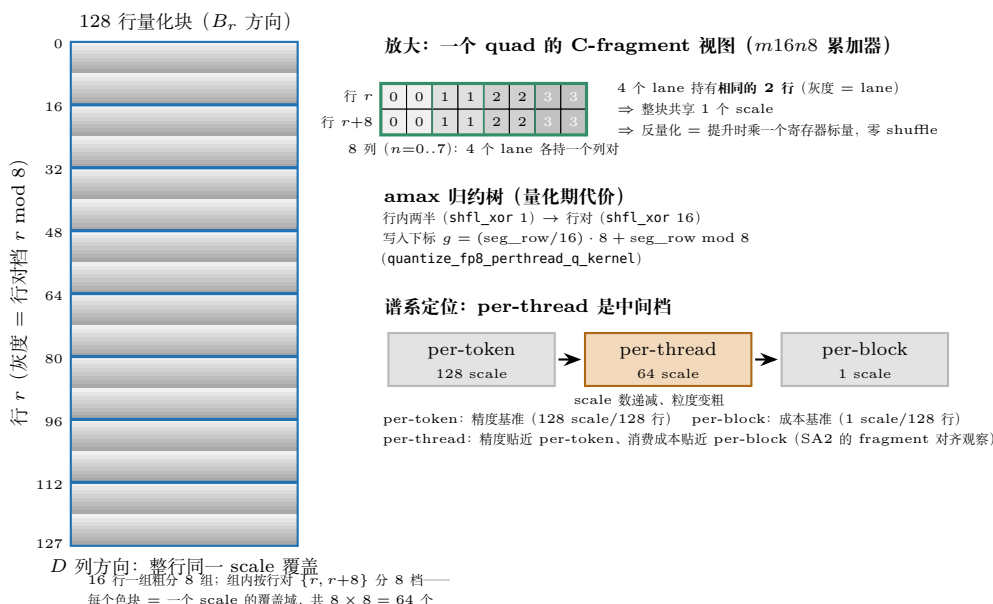
图 33.1: per-thread Q 量化的 64 槽位表与 quad 消费视角 ( \text{quantize\_fp8\_perthread\_q\_kernel} , 28.3.2 节)。左: 128 行量化块铺 8 \times 8 = 64 个 scale——行维按 16 行一组粗分 8 组 (粗边界), 组内按行对 \{r, r+8\} 分 8 档灰度 (行 r 与 r+8 同色), 每个色块就是一个 scale 的覆盖域; 写入下标 g = (\text{seg\_row}/16) \cdot 8 + \text{seg\_row} \bmod 8 。右上: 放大一个 quad 的 m16n8 C-fragment——4 个 lane 持有相同的 2 行、各占一个列对, 因此整块共享一个 scale, 反量化变成「fragment 提升时顺手乘一个寄存器标量」, 零 shuffle; 代价是 amax 归约树跨行对组合 (行内两半 \text{shfl\_xor } 1 、行对 \text{shfl\_xor } 16 )。下: 谱系定位——per-thread 是 per-token (128) 与 per-block (1) 之间的工程甜点。
