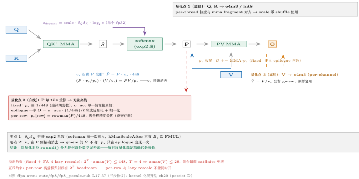
图 32.6: attention 的三个量化点与 scale 流向: \delta_Q \delta_K 折进 exp2 系数 (式 32.4)、 v_s 在 P 侧精确消去 (式 32.5)、 p_{\text{scale}} 在 epilogue 一步收尾。
