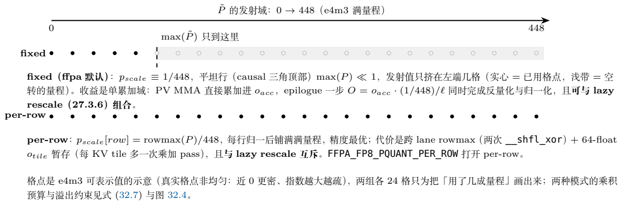
图 32.2: fixed 与 per-row 两种 p_{scale} 策略的发射域利用率 (27.3.5 节)。上: fixed 的 p_{scale} \equiv 1/448 是编译期常数, 平坦行的 \max(P) \ll 1 使发射值只占量程左端一小段, 其余量程空转——换来的是单累加域与「可与 lazy rescale 组合」; 下: per-row 用 \text{rowmax}(P)/448 把每一行拉满, 精度最优, 代价是跨 lane rowmax 归约与 64-float 的 o_{tile} 暂存, 且与 lazy rescale 互斥。
