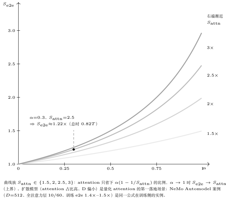
图 38.2: 端到端摊销曲线族（式 38.3）：单算子 S_{\text{attn}} 换算到管线收益由 attention 占比 \alpha 封顶。 \alpha=0.3 、 S_{\text{attn}}=2.5\times 时只剩 1.22x； \alpha \rightarrow 1 的渐近线即 S_{\text{attn}} 。
