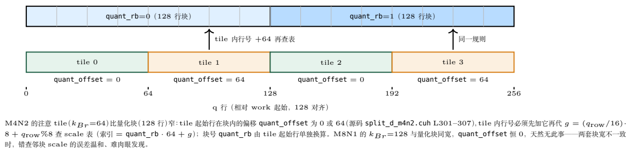
图 35.3: 量化 128 行块与 M4N2 注意 tile ( k_{Br}=64 ) 的错位对齐。tile 1/3 的起始行落在量化块内的偏移 64 处, 其行号需先加 quant_offset 再查 per-thread scale 表; tile 0/2 偏移为 0。M8N1 的 k_{Br}=128 与量化块同宽, 不存在该映射。
