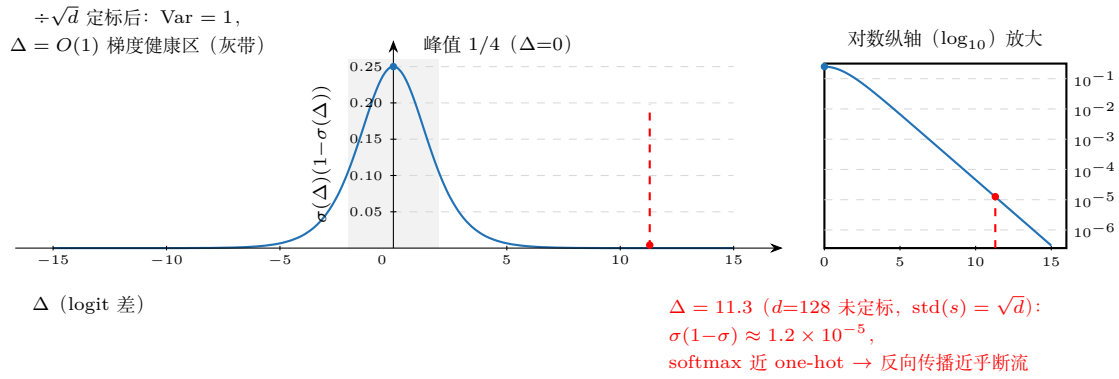
图 16.1: 1/\sqrt{d} 定标的饱和论证 (15.3.2 节, 式 16.6): sigmoid 梯度 \sigma(\Delta)(1-\sigma(\Delta)) 的峰值 1/4 在 \Delta=0 ; 除以 \sqrt{d} 后 \text{Var} = 1 、 \Delta = O(1) (灰带), 梯度处于健康敏感区。不定标时 \text{std}(s) = \sqrt{d} (式 16.5), d = 128 即 \Delta \approx 11.3 , 梯度跌到 \approx 1.2 \times 10^{-5} ——线性纵轴上贴地, 右侧对数纵轴面板可见其仍在 10^{-5} 量级 (红点, 恰在 10^{-5} 网格线上方), softmax 近 one-hot、反向传播近乎断流。曲线偶对称, \Delta = -11.3 同理。
