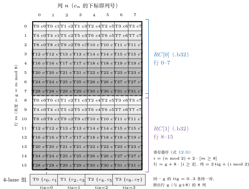
图 12.3: C fragment ( m16 \times n8 ) 寄存器布局——hgemm.cuh L311–333 字符画的 TikZ 版，与式 12.3 逐格一致：行 m = g = \text{lane} \gg 2 (灰度 8 档，行 0–7 与 8–15 由同批 lane 重复覆盖)，列对由 \text{tig} = \text{lane} \% 4 决定； RC[0] 装行 0–7、 RC[1] 装行 8–15。底部：4-lane 组内 \text{tig} = 0..3 各持一对 \{c_{2t}, c_{2t+1}\} ，拼齐一行 8 个 half——11.4.6 节 epilogue shuffle 的出发点。
