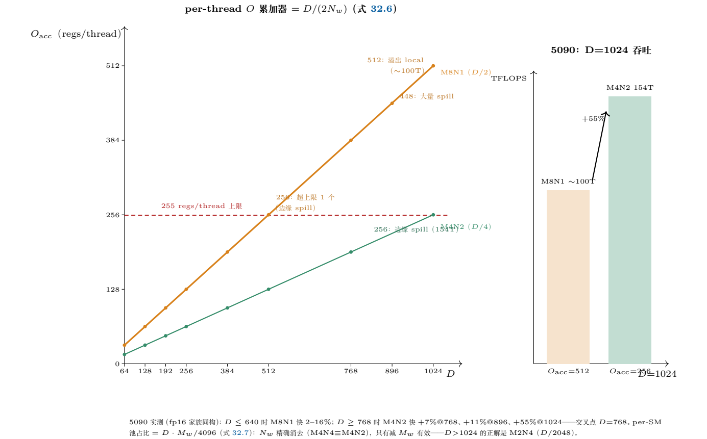
图 32.2: 寄存器墙的定量视图。左: per-thread O 累加器 = D/(2N_w) (式 32.6) ——M8N1 的 D/2 在 D=512 达 256 (超 255 上限 1 个, 边缘 spill)、 D \geq 896 大量 spill、 D=1024 溢出 local memory ( \sim 100T ); M4N2 的 D/4 同点仅 256 (154T)。右: 5090 实测 D=1024 吞吐对比 (+55%)。下: per-SM 池占比 D \cdot M_w / 4096 (式 32.7) 中 N_w 精确消去——加 N-warp 不降总量, D > 1024 只能走 M2N4。
