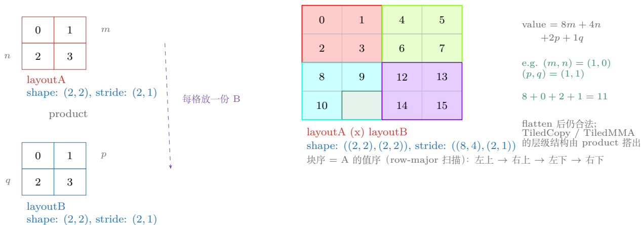
图 21.10: layout product: A 的每个坐标位放一份 B 的拷贝 (块偏移 = A 的线性序号 \times size(B)), 得到嵌套布局 ((2, 2), (2, 2)) : ((8, 4), (2, 1)) 。行值 0, 1, 4, 5 / 2, 3, 6, 7 / ... 的「块拷贝拼接」排布即 product 的几何特征——它不是 row-major。重建自 @ 竹熙佳处《写给大家看的 CuTe 教程: Layout Product & Divide》。
