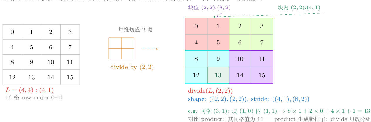
图 21.11: logical_divide: 按 2 \times 2 子块把 (4, 4) : (4, 1) 重组为 ((2, 2), (2, 2)) : ((4, 1), (8, 2)) (CuTe 实测的 zipped 形式: 块内 mode 在前、块位 mode 在后)——值排布不变 (仍 row-major), 改变的只是索引方式 (一组 (4, 1) 索引块内、一组 (8, 2) 索引块位)。与上图对比: 同物理格 (3, 1) 的 product 值为 11 (新排布), divide 后仍为 13 (原排布)。重建自同上文。
