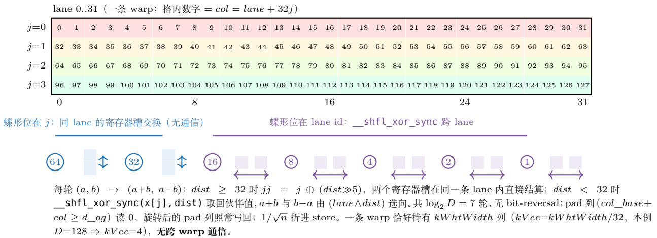
图 35.4: radix-2 蝶形的距离二分 (本例 D=128 、 kWhWidth=D )。上: 列归属—— j 是寄存器槽、lane 是 warp 内线程, 格内数字 col = lane + 32j 满足索引律, 右下角 127 = \text{size} - 1 ; 一条 warp 覆盖整行 128 列。下: 七轮的距离二分—— dist \geq 32 的 bit 落在 j 上 (同 lane 两个寄存器槽直接加减, 无通信), dist < 32 的 bit 落在 lane id 上 ( __shfl_xor_sync 跨 lane); 每轮一个 bit, 1/\sqrt{n} 折进 store。
