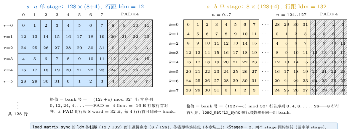
图 11.3: s_a / s_b 的 padded 行距布局 (单 stage, 格值为该 word 的 bank 号 = 行距 \times r + 列 \bmod 32 , 斜线格为 PAD)。左 s_a : 128 \times (8+4) , ldm=12 , 行首 bank 序列 0, 12, 24, 4, ...; 右 s_b : 8 \times (128+4) , ldm=132 , 行首 bank 序列 0, 4, ..., 28。补 4 float (16 B) PAD 打散行首对齐、消除 load_matrix_sync 按行取数的 bank conflict——ldm 取行距而非逻辑宽度。
