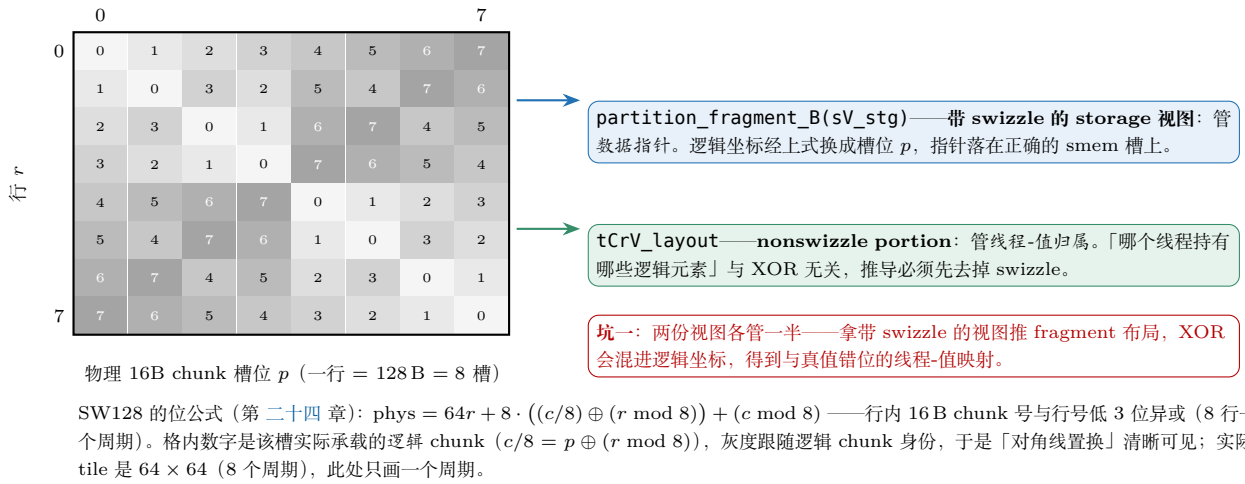
图 27.4: V 的双视图分工。同一张 SW128 smem tile: sV_stg (带 swizzle 的 storage 视图) 负责把逻辑坐标换算成物理槽位、给数据指针用; tCrV_layout (由 nonswizzle portion 推导) 负责回答「哪个线程持有哪些逻辑元素」。SW128 的 XOR 只改地址、不改归属, 所以推 fragment 布局时必须先去掉 swizzle——两份视图各管一半, 混用即错 (坑一)。
