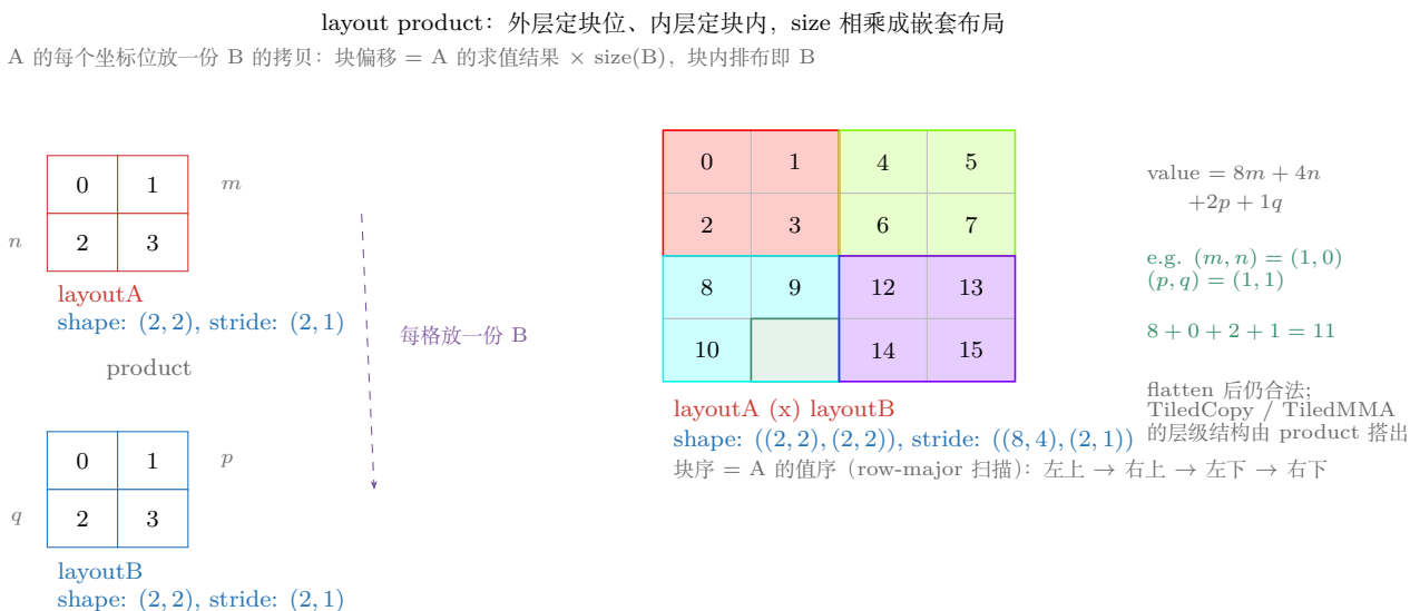
图 21.10: layout product: A 的每个坐标位放一份 B 的拷贝 (块偏移 = A 的线性序号 \times size(B)), 得到嵌套布局 ((2,2),(2,2)):(8,4),(2,1)。行值 0,1,4,5/2,3,6,7/... 的「块拷贝拼接」排布即 product 的几何签名——它不是 row-major。重建自 @ 竹熙佳处《写给大家看的 CuTe 教程: Layout Product & Divide》。
