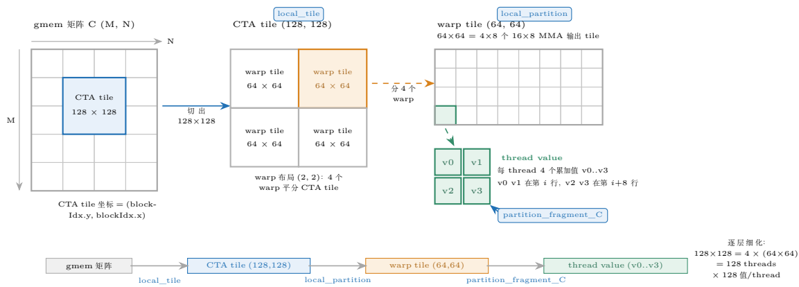
图 25.5: CuTe GEMM 的三层 partition: local_tile 以 (blockIdx.y, blockIdx.x) 为坐标从 gmemb 切出 CTA tile (128,128); warp 布局 (2,2) 下 local_partition 平分给 4 个 warp 得 (64,64); warp tile 由 4 \times 8 个 16 \times 8 atom 铺满, partition_fragment_C 为每 thread 生成累加器片段 (单 MMA tile 内 2 \times 2 四值, v0/v1 在第 i 行、 v2/v3 在第 i+8 行)。层级换算 128 \times 128 = 4 \times (64 \times 64) = 128 \text{ threads} \times 128 \text{ 值/thread} 。重建自 @reed 《cute 之简单 GEMM 实现》(示意图为经典 4-warp/64 × 64 配置; 本章 kernel 实为 tile 32 × 32、warp 16 × 16, 层级方法相同)。
