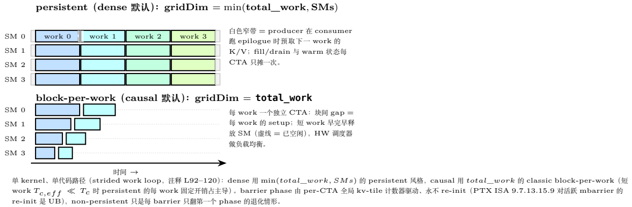
图 39.1: dense persistent 与 causal block-per-work 的 grid 调度对比 (同一 kernel、同一代码路径, runtime grid 定风格)。上: \min(\text{total\_work}, SMs) 个 CTA 按 strided work loop 认领, fill/drain 每 CTA 摊一次, producer 在 epilogue 期间预取下一 work 的 K/V; 下: 每 work 一个 CTA, 短 work 早完早释放 SM。
