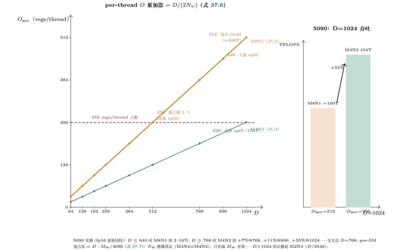
图 37.2: 寄存器墙的定量视图。左: per-thread O 累加器 = D/(2N_w) (式 37.6) ——M8N1 的 D/2 在 D=512 达 256 (超 255 上限 1 个, 边缘 spill)、 D \geq 896 大量 spill、 D=1024 溢出 local memory ( \sim 100T ); M4N2 的 D/4 同点仅 256 (154T)。右: 5090 实测 D=1024 吞吐对比 (+55%)。下: per-SM 池占比 D \cdot M_w / 4096 (式 37.7) 中 N_w 精确消去——加 N-warp 不降总量, D > 1024 只能走 M2N4。
