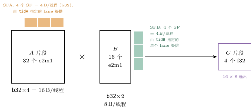
图 33.2: SM120_16x8x64_TN_VS 一条指令的操作数账。数据侧共 16 + 8 = 24 B/线程，SF 侧 8 B/线程——SF 的字节数达到数据的 1/3。注意 SF 的「字节数/线程」与「SF 数/线程」是一回事（ue4m3 是 1 字节），但哪些 lane 的字节作数由指令的 tidA/tidB 选择器决定，这就是 SF 的寄存器 fragment 必须由 CuTe 的 partition_fragment_sfa 从权威布局推导、而不能手写的原因。
