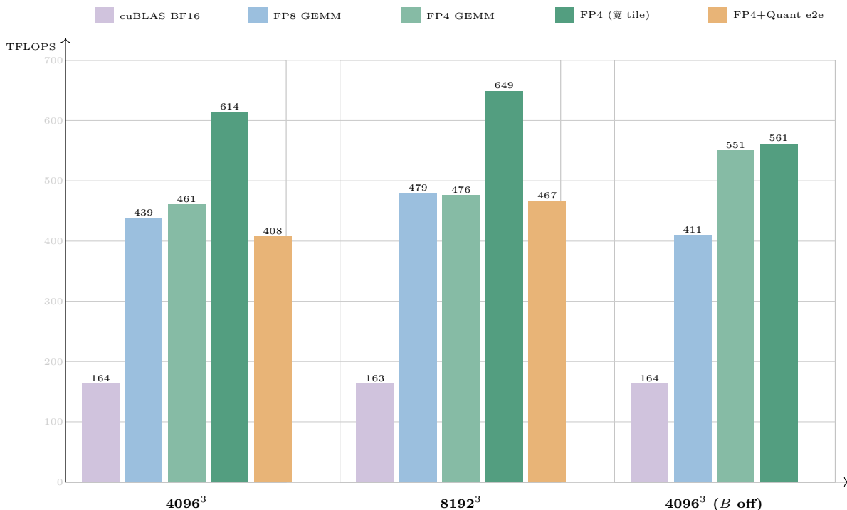
图 33.6: NVFP4 GEMM vs cuBLAS BF16 (PRO 5000, 越高越好)。三条读法: 其一, kernel-only 口径下 FP4 只比 FP8 快 6 ~ 40%——库默认档 ( 128^2/s4 , 柱取口径: 4096^3 取扫描表 461 T, 8192^3 取默认档实测 476 T) 只快 6%, 宽 tile 档才快 40%, 远不是比特数暗示的 2\times ; 原因是本 kernel 走 bf16 输出、f32 累加, 且 BK=64 让 K 方向的算术强度下降 (表 33.1 的两条「钉死」); 其二, 宽 tile ( 128\times 256 ) 是本章最大的单项收益 (+31%, 33.9.4 节), 也是 --bench 标准行在 MNK \geq 4096 上的自适应选择; 其三, e2e 口径下 FP4 反超 FP8 ( 4096^3 : 408 vs 187 T; 8192^3 : 467 vs 315 T)——量化的写出字节数只有 FP8 的一半, B 侧重构后这个差距被彻底拉开 (33.9.3 节); 第三组 (B 离线) 把 FP4 的 e2e 拉回 551~561 T (FP8 为 411 T), 是各自 kernel 的 91 ~ 93%。
