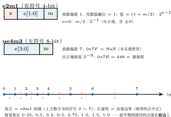
图 32.2: NVFP4 的两个 4-bit 类型。上：e2m1 位域与数轴（格宽随量级翻倍，最外侧两格「码点在格边」是误差模型里最大的一项贡献，见 32.5 节）；下：ue4m3 位域（scale 专用，量程 [2^{-9}, 448] ， 0x7F 是 NaN）。
