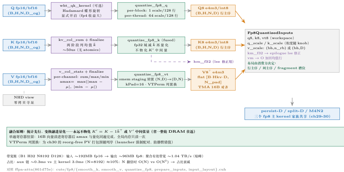
图 35.5: fp8 前处理链全景: 三泳道 (Q/K/V) 各自的统计 \rightarrow 变换 \rightarrow 量化 kernel 与输出 workspace 布局。smoothing 与量化融合在同一 kernel 内 (无中间落盘); V^\top 的列 pad 兼顾 TMA 16B 对齐与置换写。
