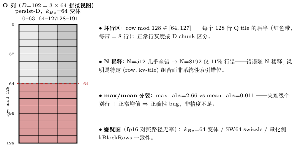
图 31.6: D=192 正确性 bug 的坏行定位 (29.7.1 节五步法的可视化)：把 O 视为 3 \times 64 列拼接，坏行集中在 \text{row mod } 128 \in [64, 127] (每个 128 行 Q tile 的后半)；N=512 几乎全错而 N=8192 仅 11% 行错 (N 稀释 \Rightarrow 特定 (row, kv-tile) 组合)；max_abs=2.66 对 mean_abs=0.011 的分裂是「个别行灾难」的强信号。
