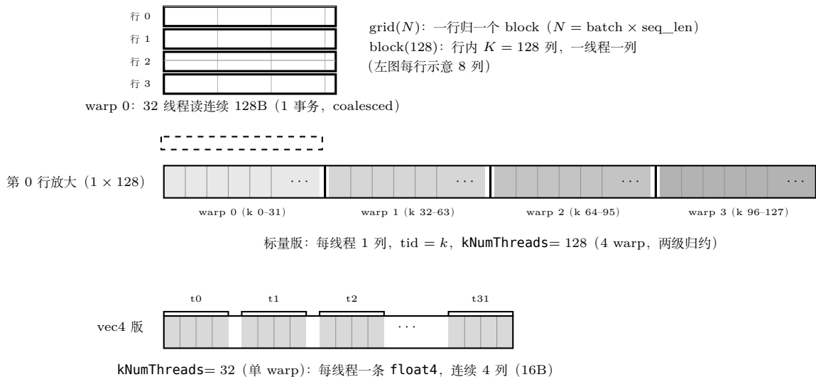
图 7.2: one-row-one-block 行划分: 上, N \times K 矩阵每行归一个 block ( \text{grid}(N) ); 中, 单行放大为 1 \times 128 条带, 4 个 warp 各占 32 列 (各一档灰度), warp 0 的 32 线程读连续 128B, 单事务合并; 下, vec4 版改为 32 线程、每线程一条 float4 (连续 4 列), 指令数降为 1/4。
